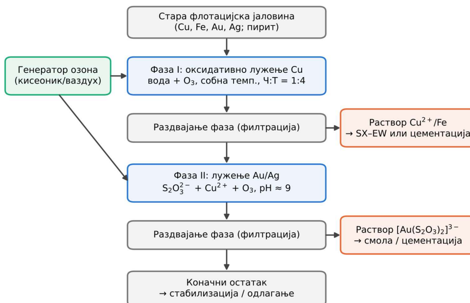
Слика 5.2. Концептуална шема двостепене прераде старе флотацијске јаловине озонским и озонско-тиосулфатним лужењем (предлог аутора)
