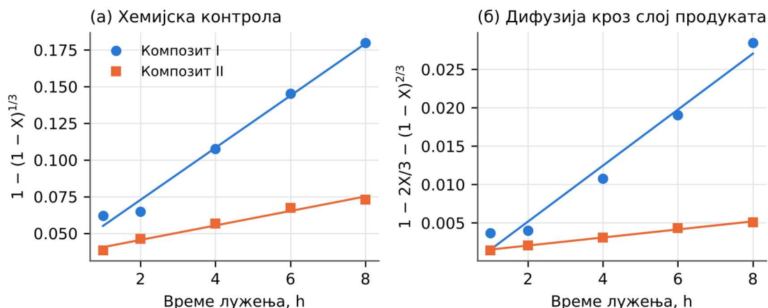
Слика 4.6. Линеаризација података о лужењу гвожђа у Експерименту 2 према моделу смањујућег језгра: (а) хемијска контрола, (б) дифузиона контрола (обрада аутора)
