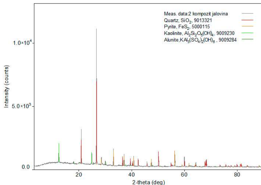
Слика 4.16. Дифрактограм полазног узорка Композит II [17]
