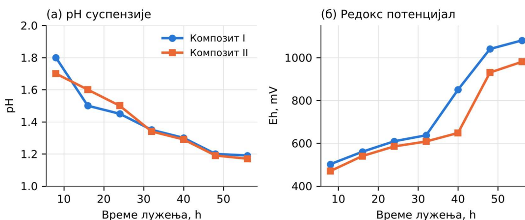
Слика 4.3. Промена (а) pH вредности и (б) редокс потенцијала током лужења у Експерименту I (подаци из [17], обрада аутора)
