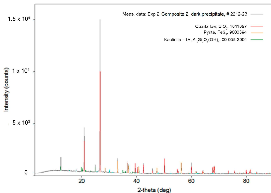
Слика 4.9а. Дифрактограм тамне фазе Композита II из Експеримента 2 [17]
