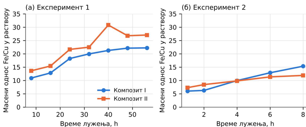
Слика 4.5. Масени однос Fe/Cu у раствору током лужења: (а) Експеримент 1, (б) Експеримент 2 (обработка аутора)
