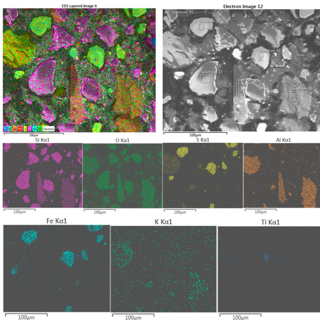
Слика 4.12. (а) EDS мапа и (б) SEM слика тамне фазе Композита II (увећање 500×); (в) расподела елемената [17]
