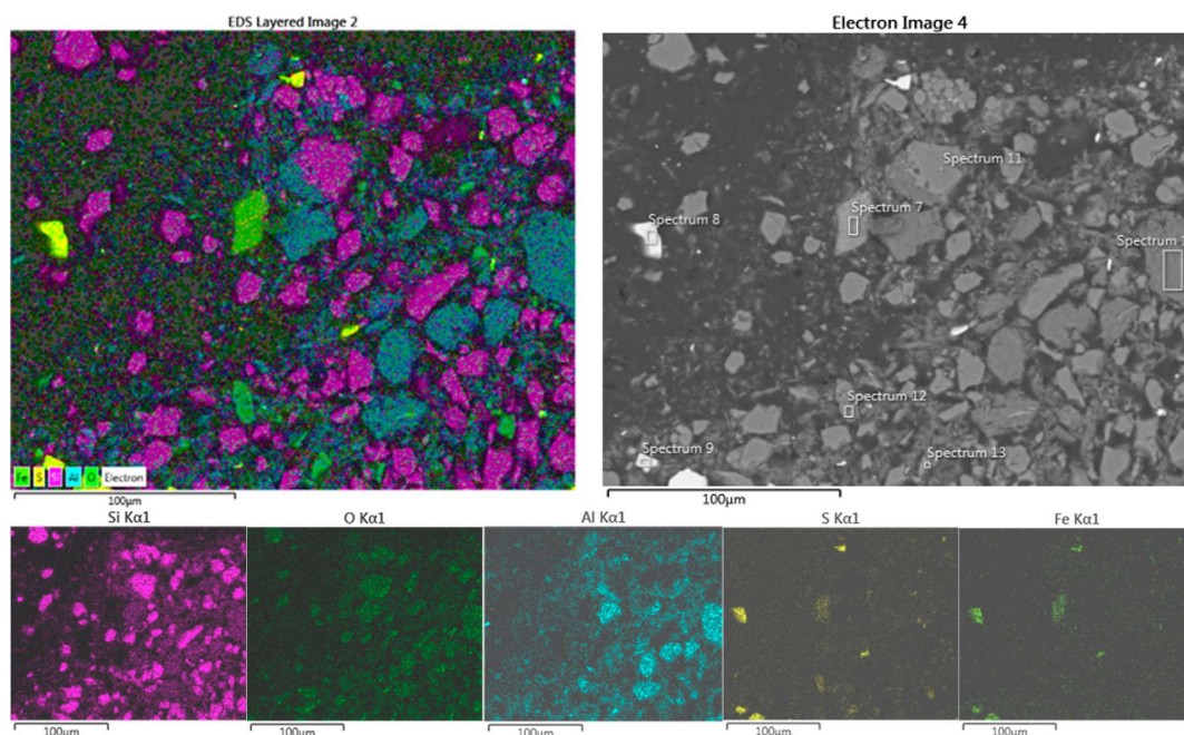
Слика 4.13. (а) EDS мапа и (б) SEM слика светле фазе Композита II (увећање 500×); (в) расподела елемената [17]
