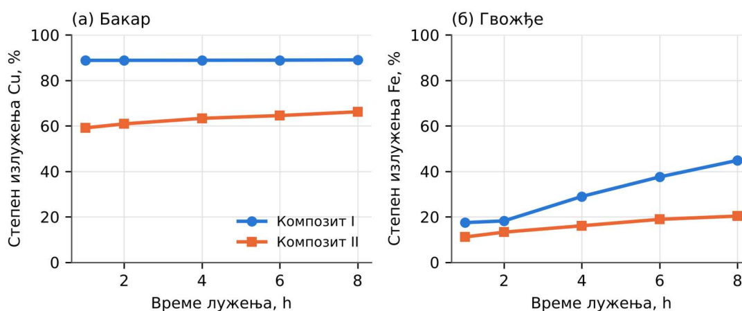
Слика 4.4. Кинетика лужења (а) бакра и (б) гвожђа у Експерименту 2 (подаци из [17], обрада аутора)
