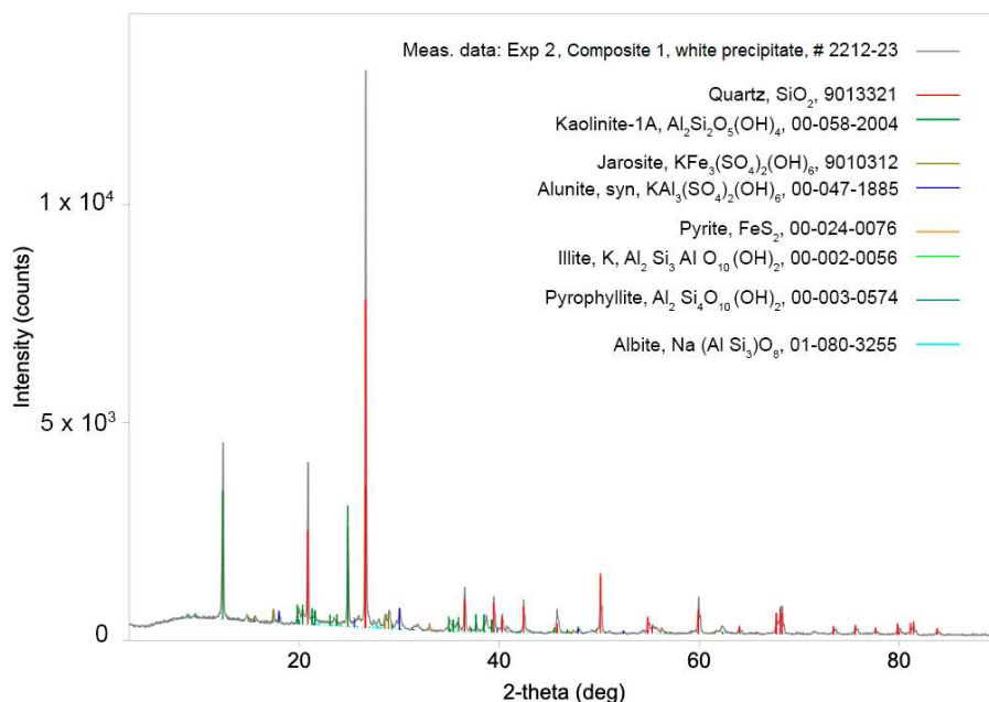
Слика 4.8б. Дифрактограм светле фазе Композита I из Експеримента 2 [17]
