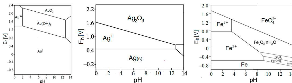
Слика 5.1. Pourbaix ( E_h - pH ) дијаграми на 25 °C за системе: (а) \text{Au-O} , (б) \text{Ag-O} и (в) \text{Fe-O} (претпостављена концентрација растворених врста 10^{-4} \text{ mol/L} ) [17,132]
