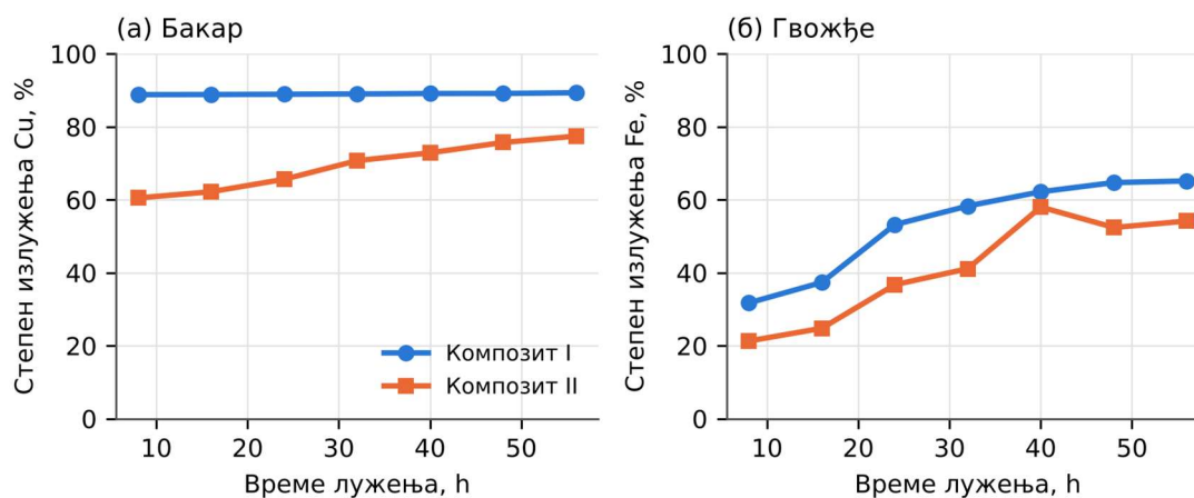
Слика 4.2. Кинетика лужења (а) бакра и (б) гвожђа у Експерименту 1 (подаци из [17], обрада аутора)
