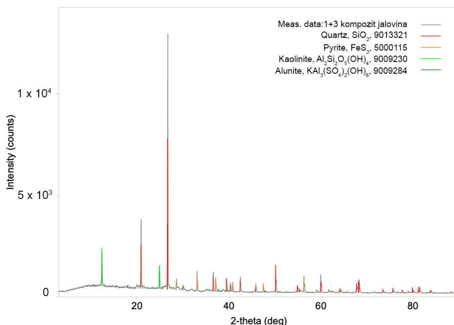
Слика 4.1а. Дифрактограм полазног узорка Композит I [17]
