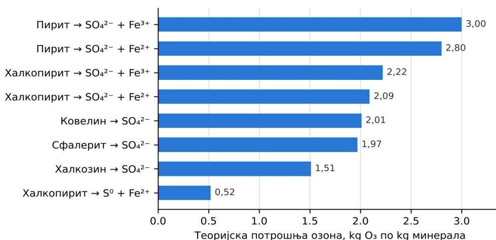
Слика 6.8. Теоријска стехиометријска потрошња озона за оксидацију сулфидних минерала у зависности од крајњих производа оксидације (прорачун аутора)
