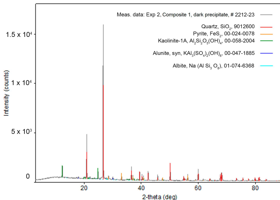
Слика 4.8а. Дифрактограм тамне фазе Композита I из Експеримента 2 [17]
