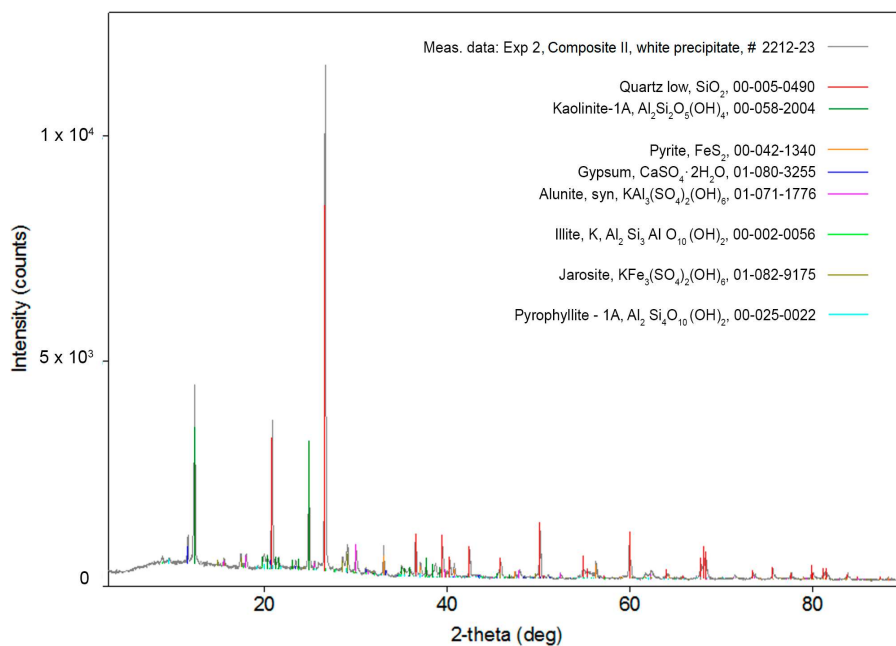
Слика 4.96. Дифрактограм светле фазе Композита II из Експеримента 2 [17]
