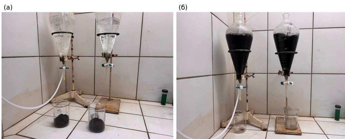
Слика 6.2. Лабораторијска апаратура за озонско лужење концентрата бакра: (а) одмерени узорци концентрата у стакленим чашама и реакциони судови са раствором кроз који се уводи озон, пре додавања концентрата; (б) пулна концентрата у реакционим судовима током лужења озоном (фотографије аутора)
