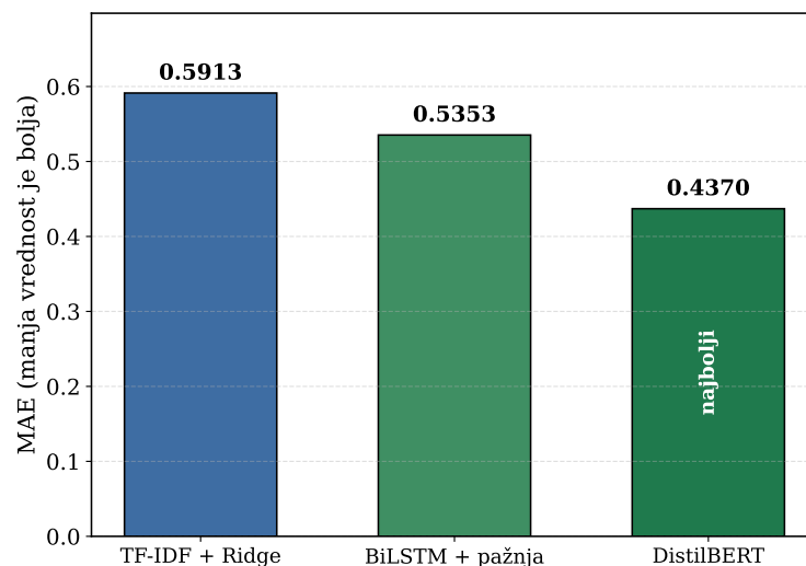
Slika 4.2: Poređenje performansi modela za predikciju hotelskih ocena.
