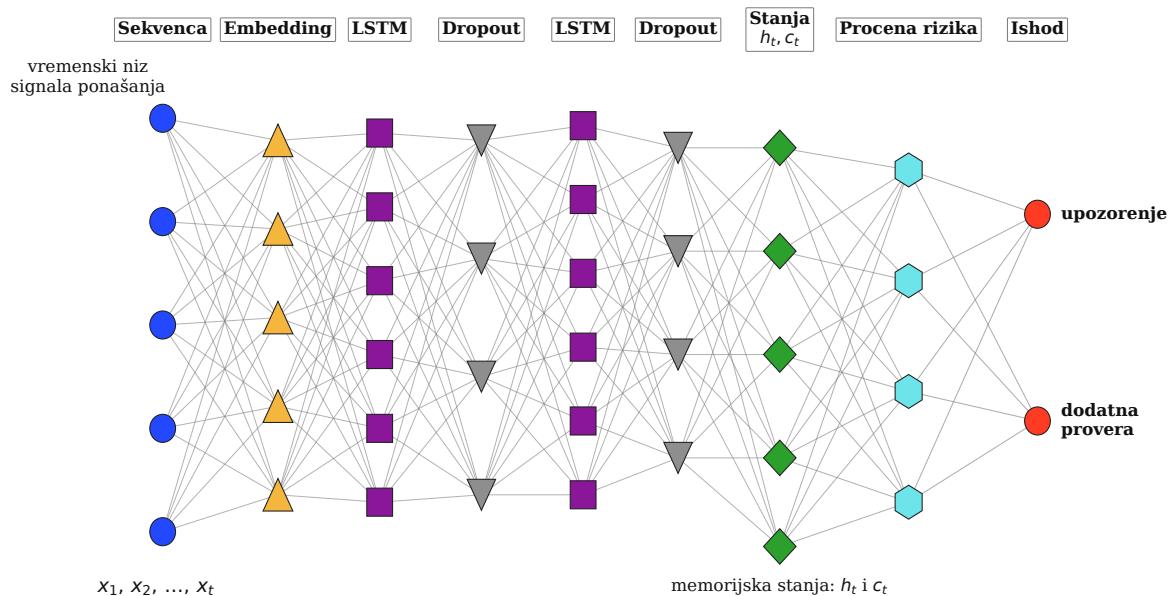
Slika 5.3: LSTM tok za ranu detekciju agresivne vožnje kroz sekvencu ponašajnih i kontekstualnih signala.
