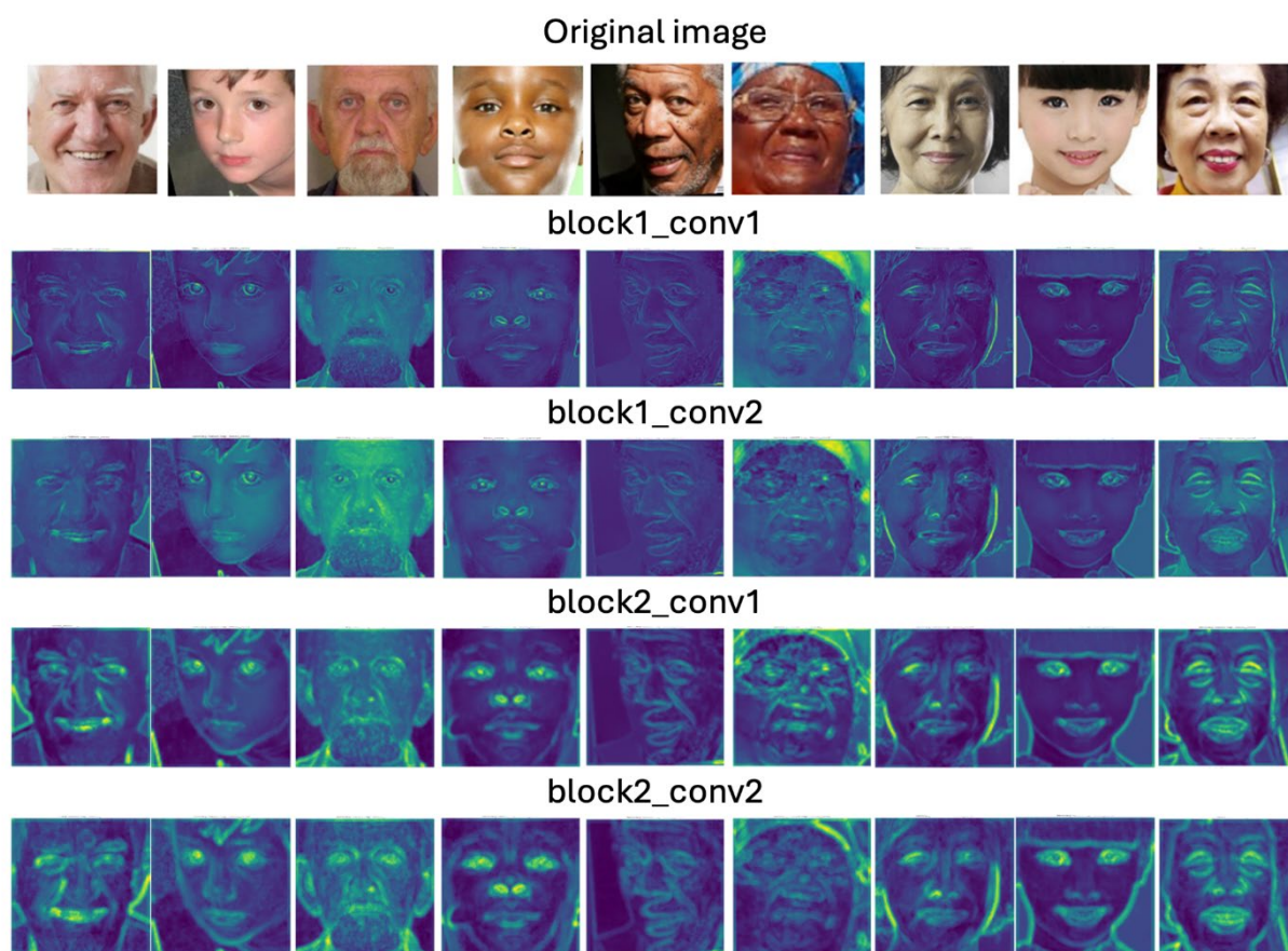
Slika 26. Primeri slika iz UTKFace skupa podataka i njihove mape karakteristika kroz slojeve.
