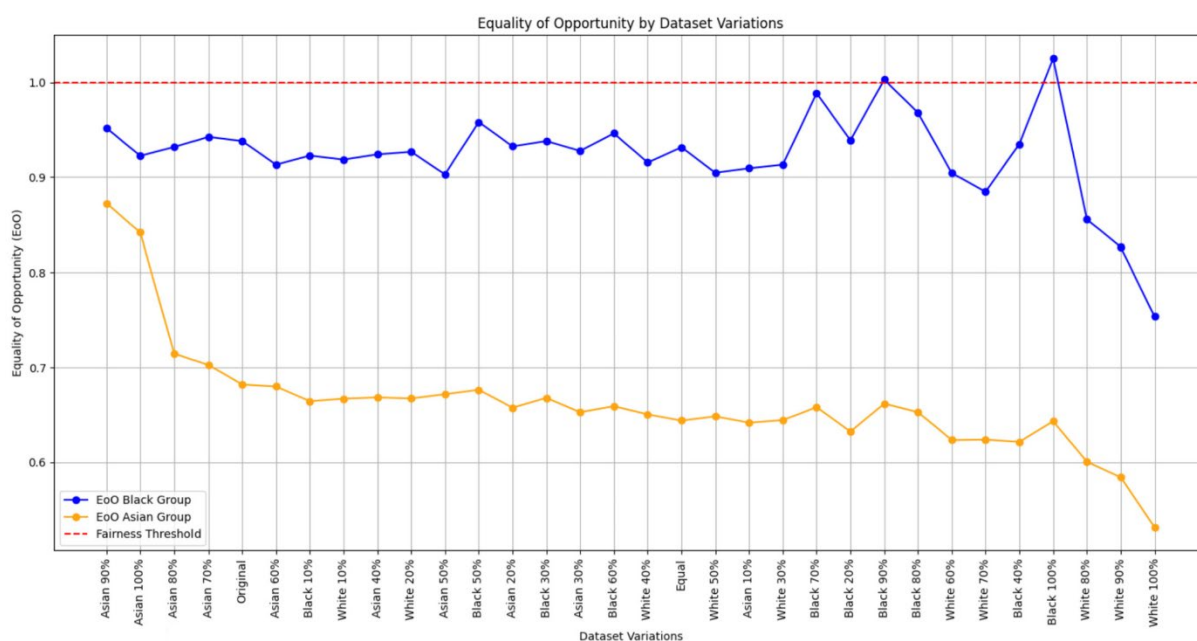
Slika 24. Nejednaki uticaj prema varijacijama UTK Face skupa podataka.
