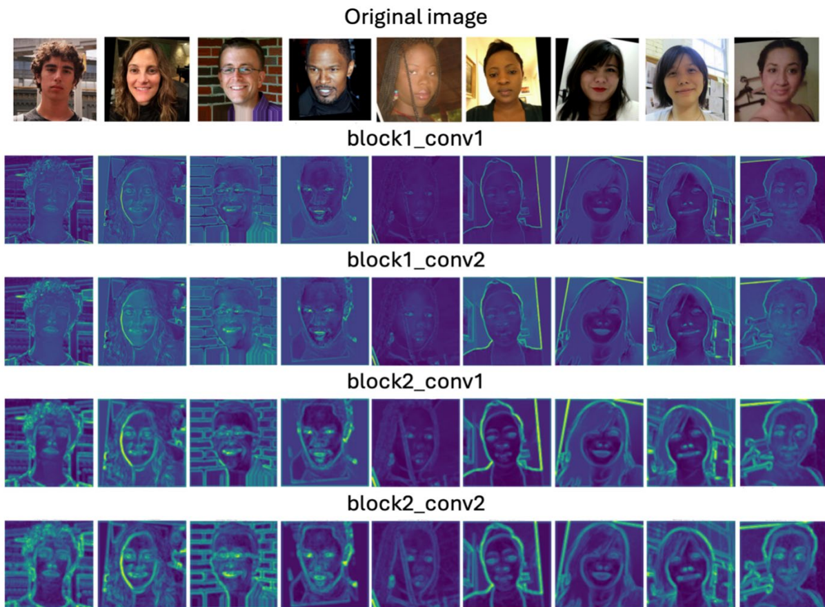
Slika 27. Primeri slika iz APPA-REAL skupa podataka i njihove mape karakteristika kroz slojeve.
