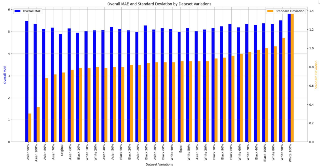
Slika 22. Ukupni MAE i standardna devijacija za varijacije skupa podataka UTK Face
