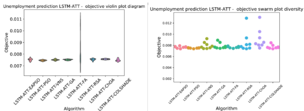
Slika 14 Dijagrami raspodele vrednosti funkcije cilja u LSTM-ATT simulacijama prognožiranja nezaposlenosti
