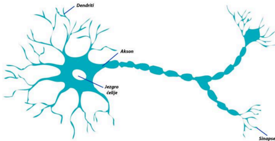
Slika 1 Biološki neuron
