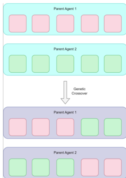
Slika 5 Cross-over mehanizam
