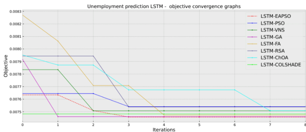
Slika 11. Dijagrami konvergencije vrednosti funkcije cilja u LSTM simulaciji prognožiranja nezaposlenosti
