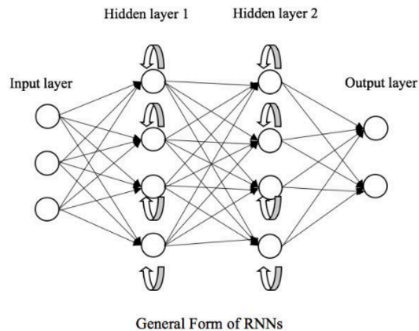
Slika 4 Arhitektura rekurentnih neuronskih mreža RRN
