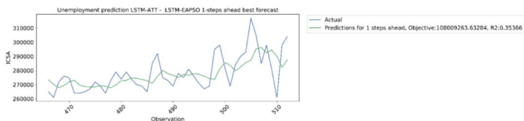
Slika 18. Najbolje pokazani model LSTM-ATT-EAPSO za predviđanje nezaposlenosti
