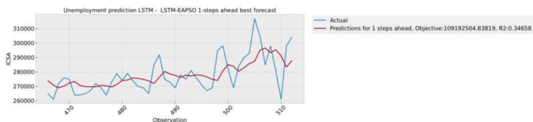
Slika 13 Prognoze modela LSTM-EAPSO sa najboljim performansama
