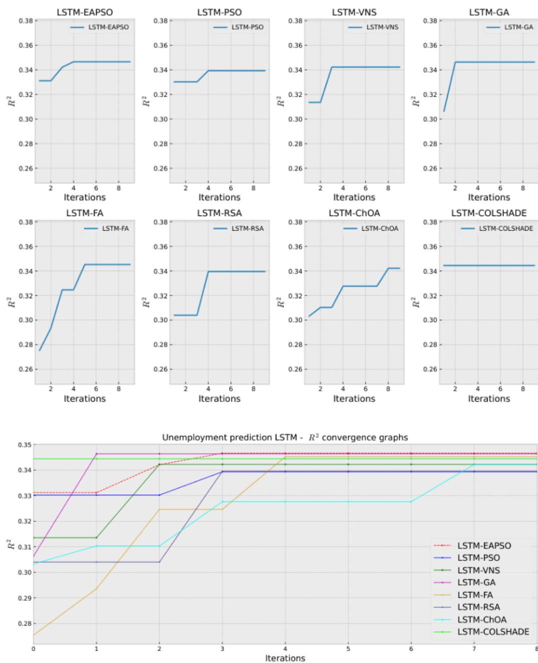
Slika12. Dijagrami konvergencije vrednosti indikatorske funkcije u LSTM simulacijama prognožiranja nezaposlenosti
