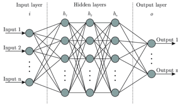
Slika 2 Arhitektura neuronske mreže
