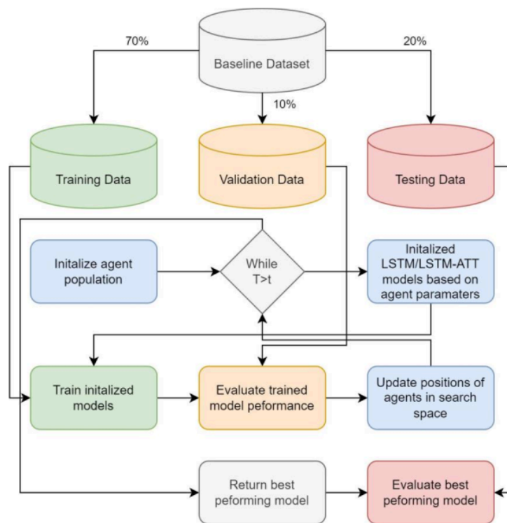
Slika 7 Dijagram toka predloženog optimizacionog okvira
