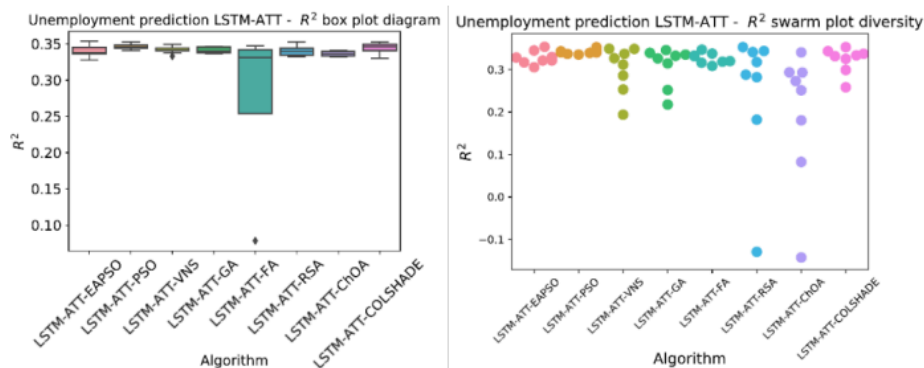
Slika 15. LSTM-ATT dijagrami raspodele vrednosti indikatorske funkcije u simulacijama prognožiranja nezaposlenosti
