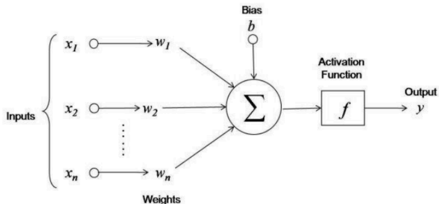
Slika 3 Arhitektura neurona
