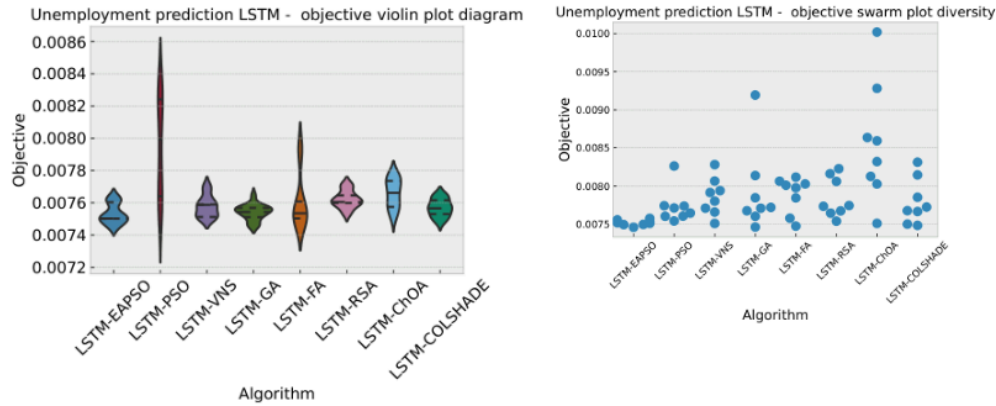
Slika 9. Dijagram raspodele ishoda funkcije cilja u LSTM simulacijama prognožiranja nezaposlenosti
