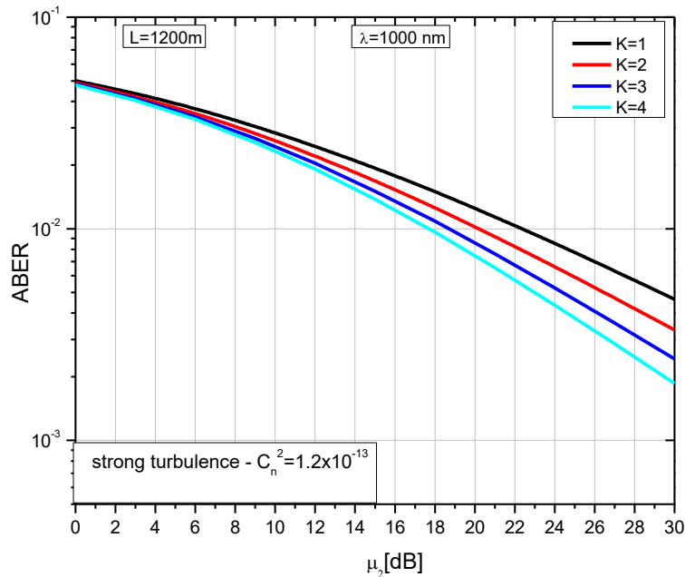
Slika 6.4.2. ABER za FSO sistem u uslovima jake turbulencije za različite vrednosti K-faktora kada se primenjuje CBPSK tehnika modulacije.
