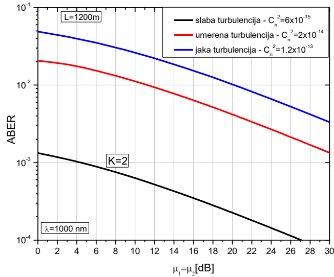
Slika 6.4.4. ABER za FSO sistem u uslovima slabe, umerene i jake turbulencije za K=2 pri primeni CBPSK tehnike modulacije.
