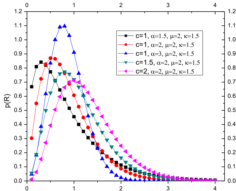
Slika 5.3.1. PDF nove kompozitne distribucije za različite vrednosti odgovarajućih parametara
