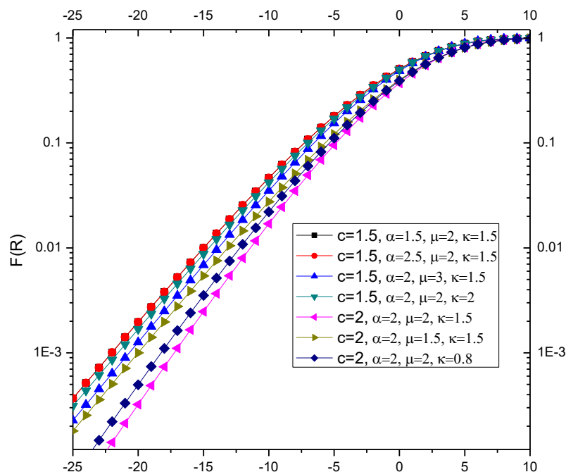
Slika 5.3.2. CDF funkcija kompozitnog procesa za različite vrednosti odgovarajućih parametara.
