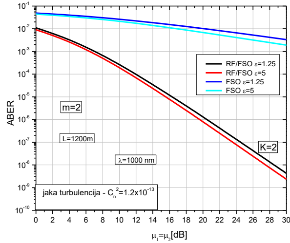
Slika 6.4.5. ABER za hibridne One-Hop RF/FSO i FSO sisteme kao funkcija greške pokazivanja.
