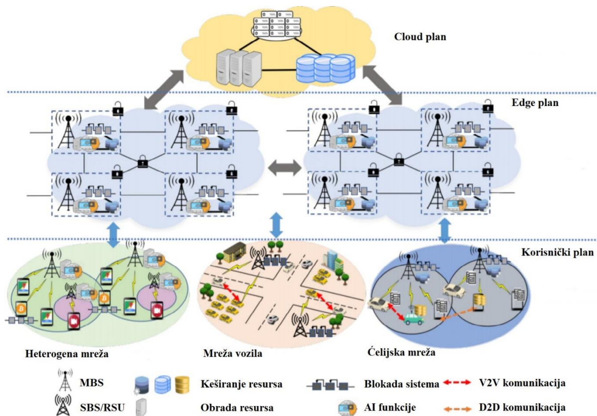
Slika 2.19.1. Bezbedna i inteligentna arhitektura 6G.
