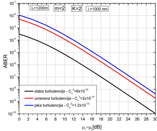
Slika 6.4.3. ABER za hibridni One-Hop RF/FSO sistem u uslovima slabe, umerene i jake turbulencije za vrednosti K=2 , K=2 i m=2 pri primeni CBPSK tehnike modulacije.
