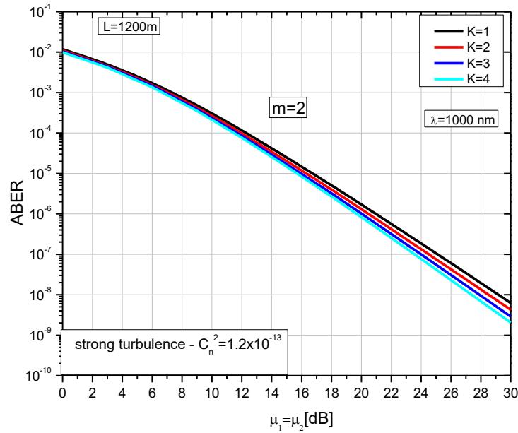
Slika 6.4.1. ABER za hibridni One-Hop RF/FSO sistem u uslovima jake turbulencije za različite vrednosti K-faktora kada se primenjuje CBPSK tehnika modulacije.
