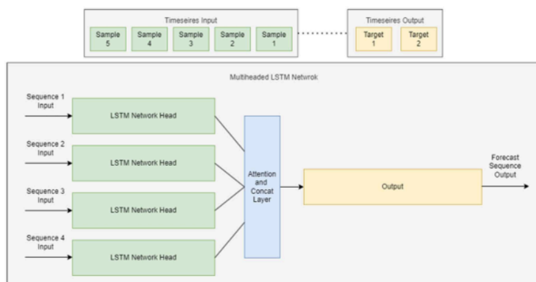
Ilustracija 11 MHLSTM mreža
