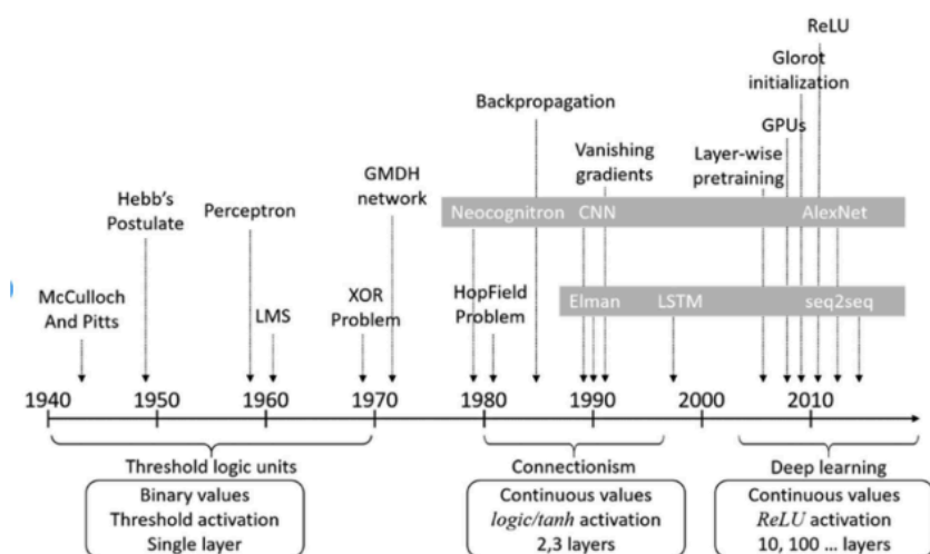
Ilustracija 4 Istorijat razvoja modela mašinskog učenja
