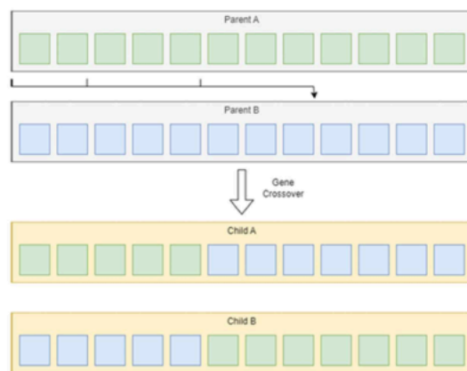
Ilustracija 9 Cross-over mehanizam
