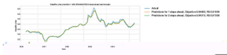
Ilustracija 24 Modeli sa najboljim predikcijama
