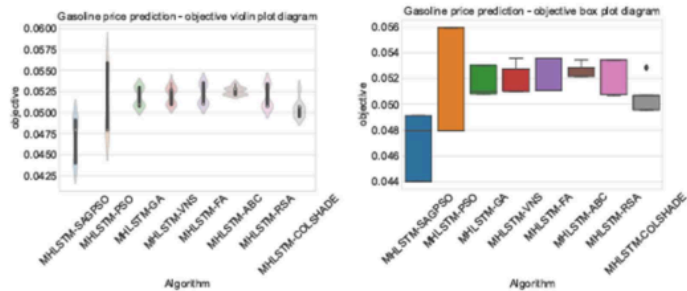
Ilustracija 16 Distribucija rezultata funkcije cilja
