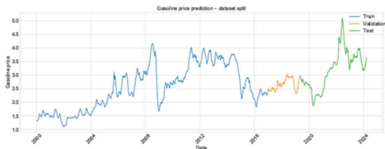
Ilustracija 14 Vizuelni prikaz skupa podataka
