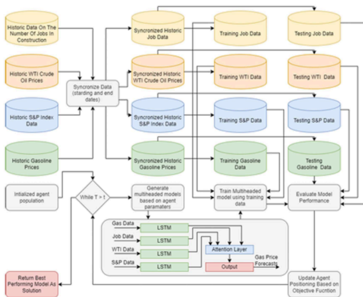
Ilustracija 12 Predloženi okvir
