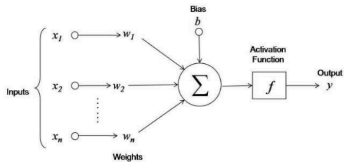
Ilustracija 6 Arhitektura neurona
