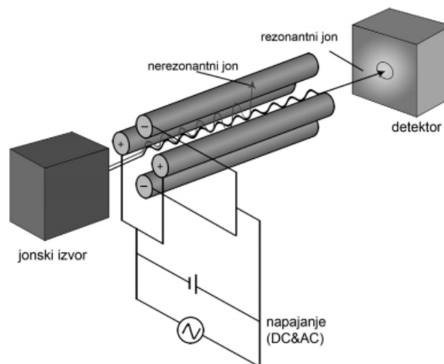
Slika 8. Kvadrupolni maseni analizator
