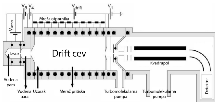
Slika 7. Drift cev PTR-MS uređaja (izvor slike: Blake i koautori, 2009)
