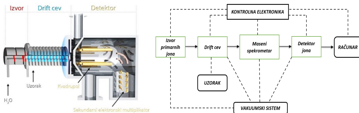
Slika 6. Prikaz osnovnih delova uređaja PTR-MS
