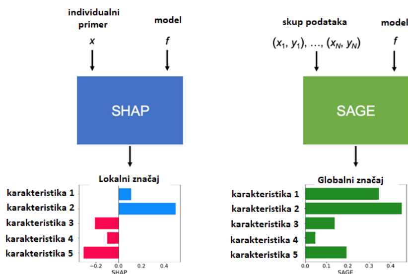
Slika 17. Primer lokalne (SHAP, levo) i globalne (SAGE, desno) interpretacije uticaja varijabli (Ian Covert, 2020)
