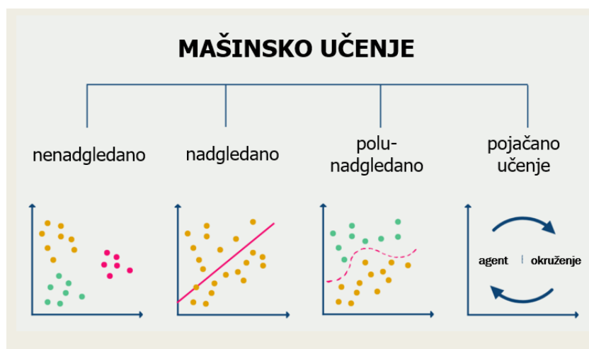
Slika 12: Vrste mašinskog učenja (izvor: https://databasecamp.de/en/ml/semi-supervised-learning-en pristupljeno 22.1.2025. godine)
