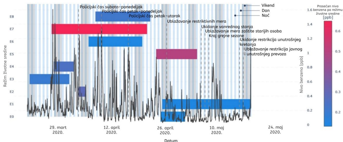
Slika 22. Vremenske serije nivoa benzena i režima životne sredine
