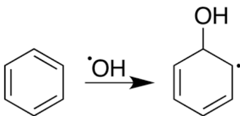
Slika 3. Reakcija benzena sa \cdot\text{OH}
