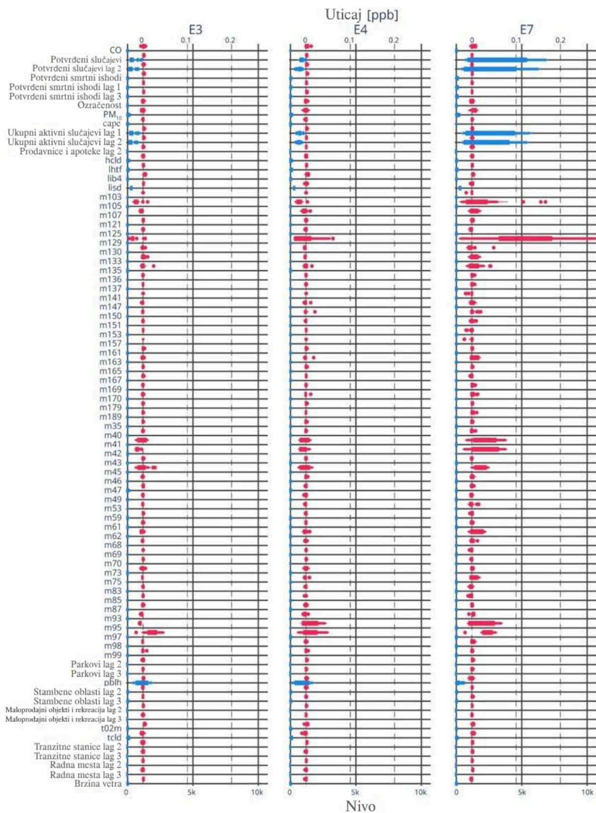
Slika 23. Distribucija najvažnijih nivoa (plavo) i uticaja (crveno) za režime E3, E4 i E7
