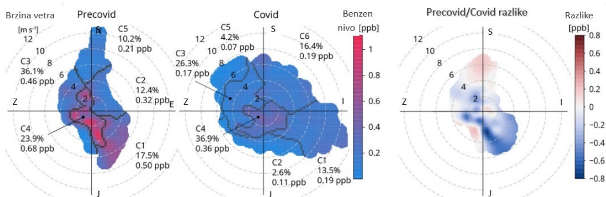
Slika 18. Indikacija prostorne raspodele i razlika u nivoima benzena pre i tokom pandemije (Radić i koautori, 2025)
