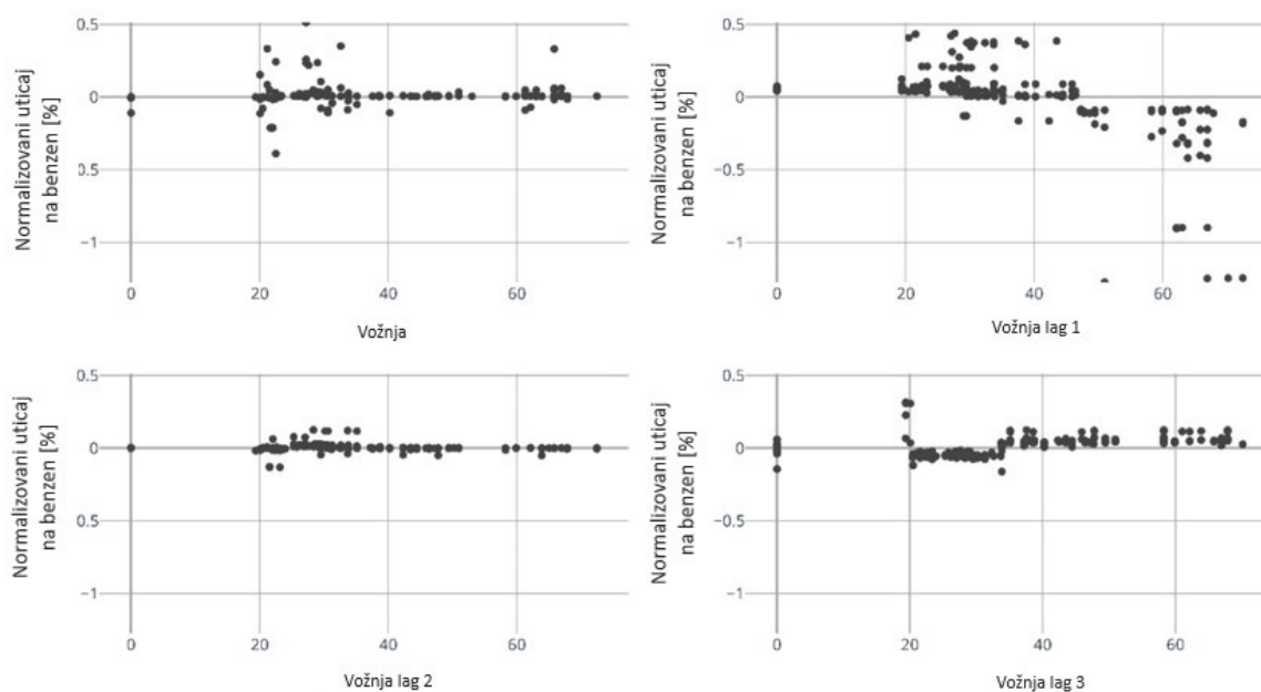
Slika 26. Normalizovani uticaj smanjene vožnje na dinamiku benzena (u realnom vremenu i sa zakašnjenjem od jednog, dva i tri dana)
