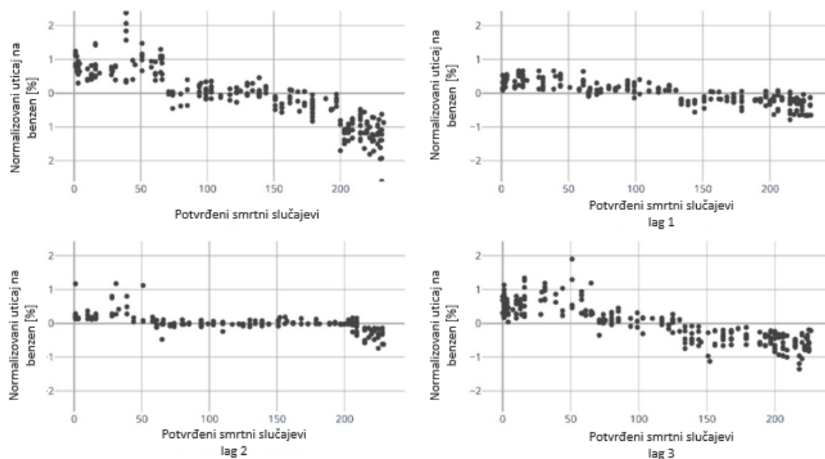
Slika 25. Normalizovani uticaj potvrđenih smrtnih slučajeva na dinamiku benzena (u realnom vremenu i sa zakašnjenjem od jednog, dva i tri dana)
