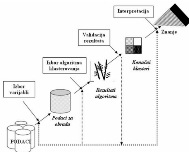
Slika 11. Koraci u postupku klaster analize (Dragnić, 2016)
