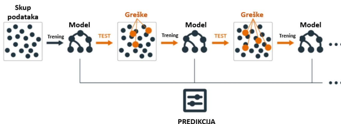
Slika 14. Glavni koraci rada u Boosting-a (izvor: https://mlvu.github.io/lecture10/ pristupljeno 22.1.2025. godine)
