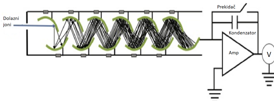
Slika 9. Sekundarni elektronski multiplikator (izvor slike: Carlson, 2025)
