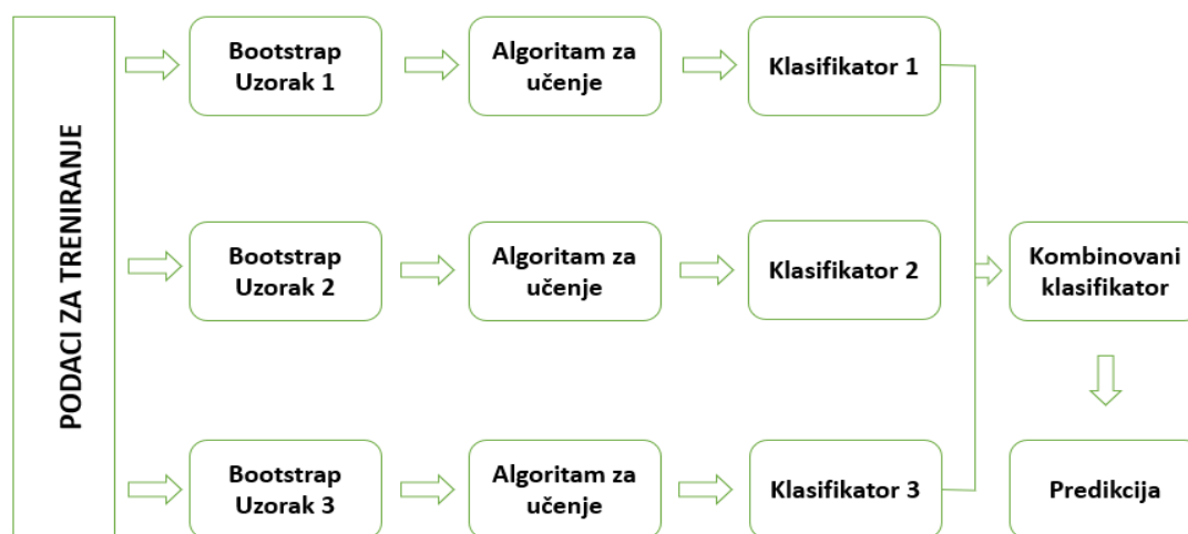
Slika 13. Glavni koraci rada koncepta Bagging (CFI, 2025)
