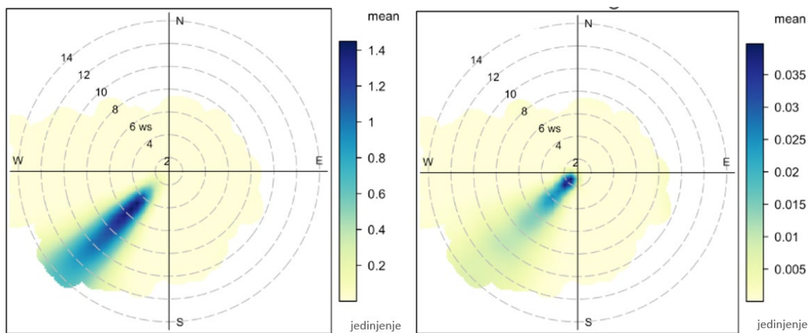
Slika 10. Primer emisija iz visoko (levo) i nisko (desno) pozicioniranih izvora
