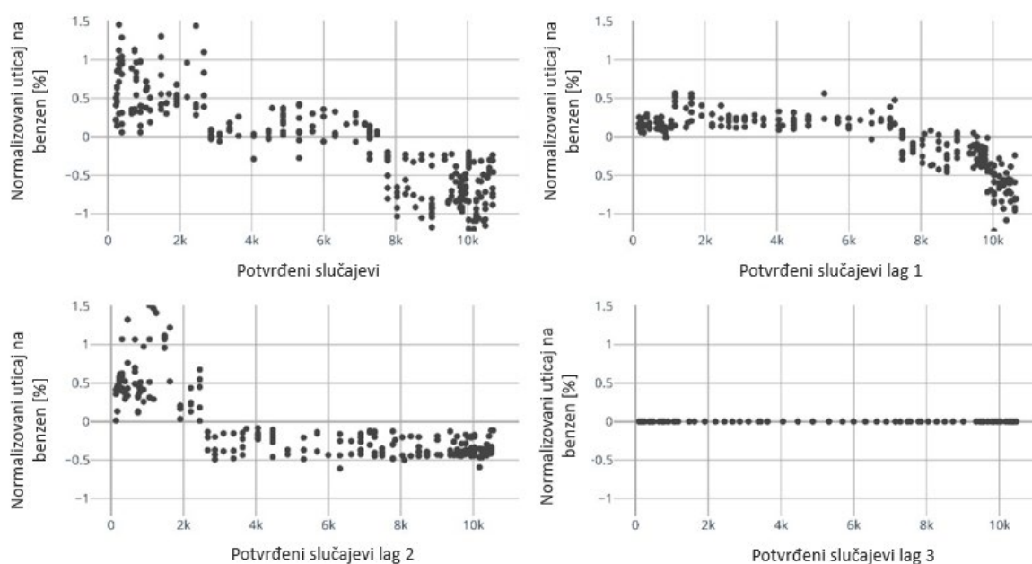
Slika 24. Normalizovani uticaj potvrđenih slučajeva na dinamiku benzena (u realnom vremenu i sa zakašnjenjem od jednog, dva i tri dana)
