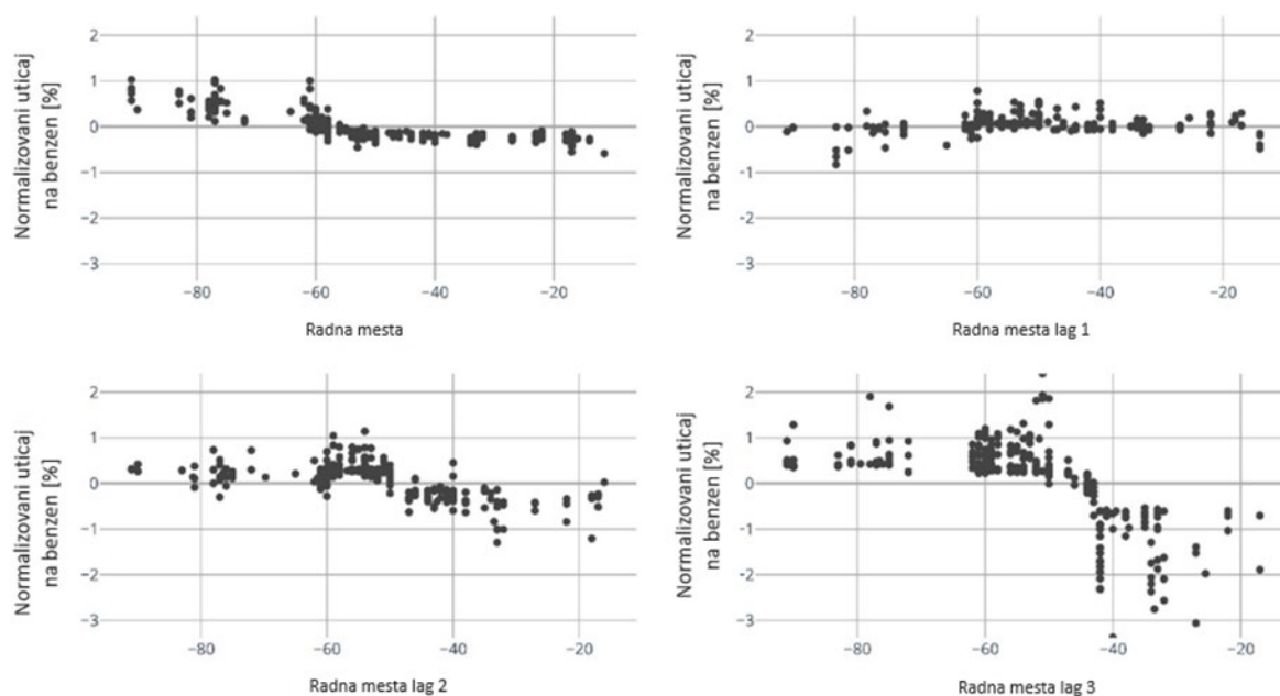
Slika 27. Normalizovani uticaj promene prisustva zaposlenih na radnim mestima na dinamiku benzena (u realnom vremenu i sa zakašnjenjem od jednog, dva i tri dana)
