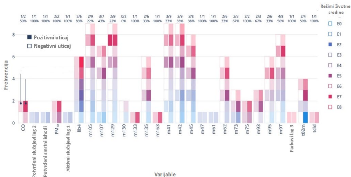
Slika 21. Normalizovani nivoi i normalizovani lokalni uticaji varijabli u različitim režimima životne sredine (Radić i koautori, 2025).
