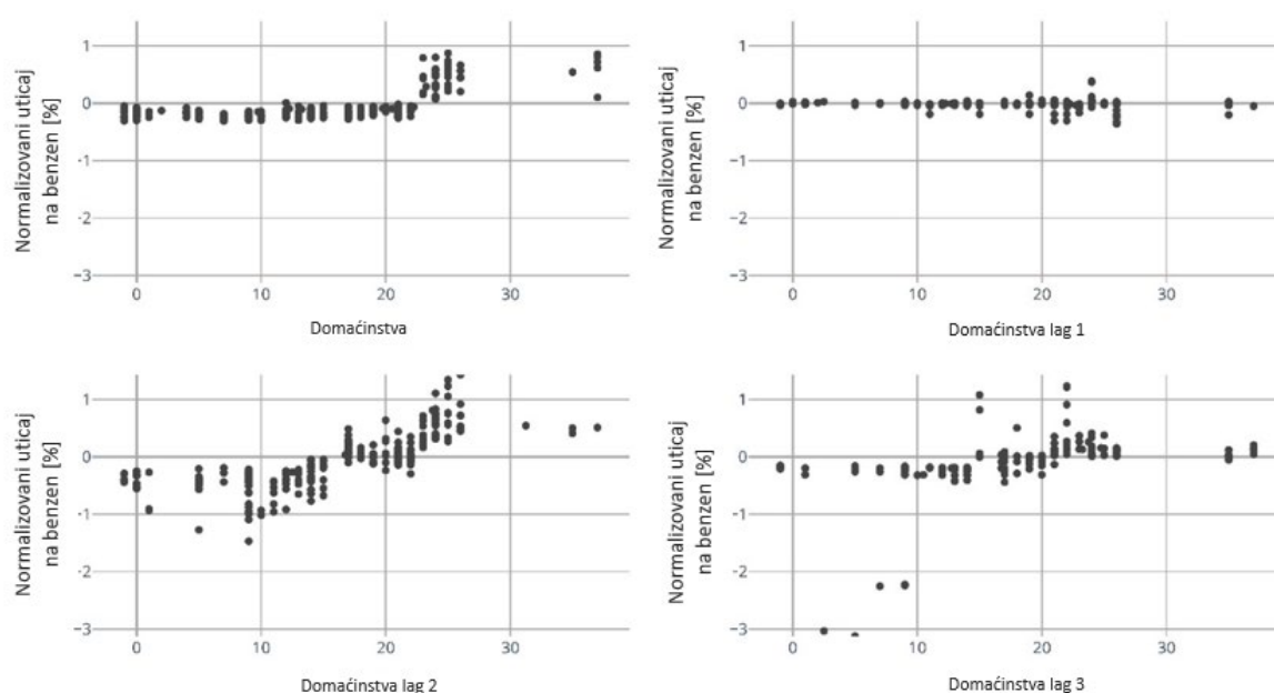
Slika 28. Normalizovani uticaj promene vremena provedenog kod kuće na dinamiku benzena (u realnom vremenu i sa zakašnjenjem od jednog, dva i tri dana)
