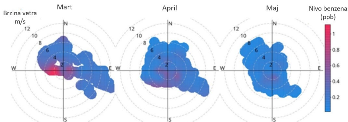
Slika 19. Indikacija mesečne prostorne raspodele nivoa benzena tokom pandemije (Radić i koautori, 2025)
