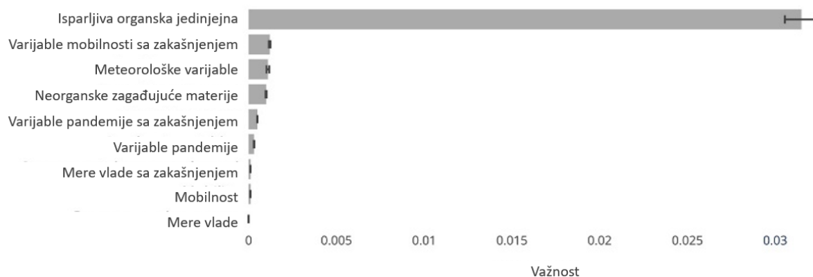
Slika 20. Globalna važnost grupa varijabli na koncentracije benzene tokom vanrednog stanja izazvanog pandemijom COVID-19
