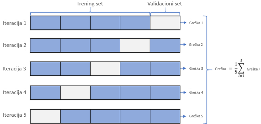
Slika 15: 5-fold cross-validacija (Rebecca Patro, 2021)
