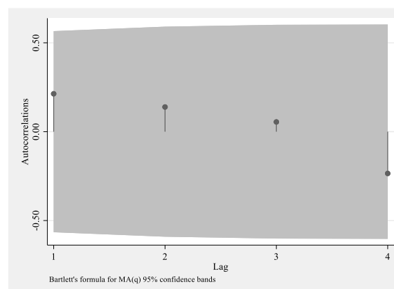
Графикон 54. ACF за проценат војне потрошње у извршењу буџета Републике србије
