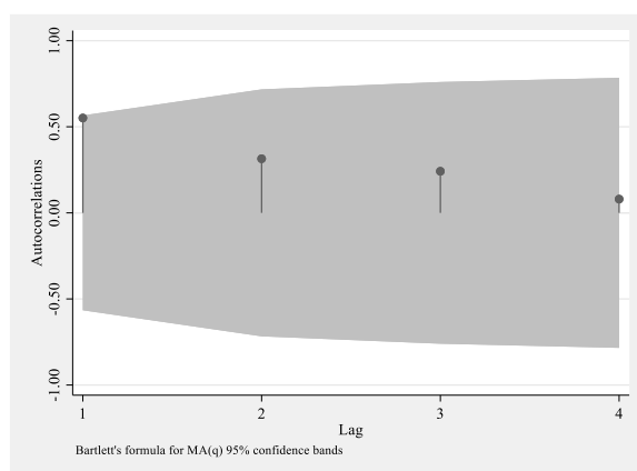
Графикон 36. ACF за извоз роба и услуга у Републици Србији
