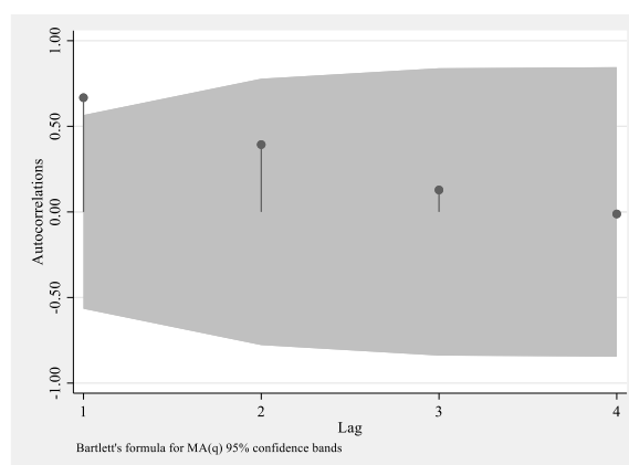
Графикон 26. ACF за консолидоване јавне расходе у буџету Републике Србије
