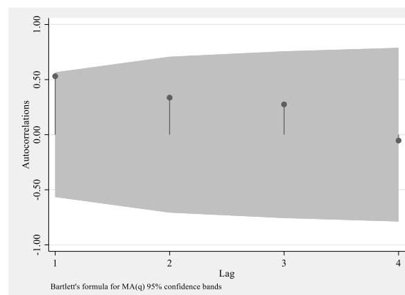
Графикон 59. ACF за планиране инвестиције у буџету Министарства одбране
