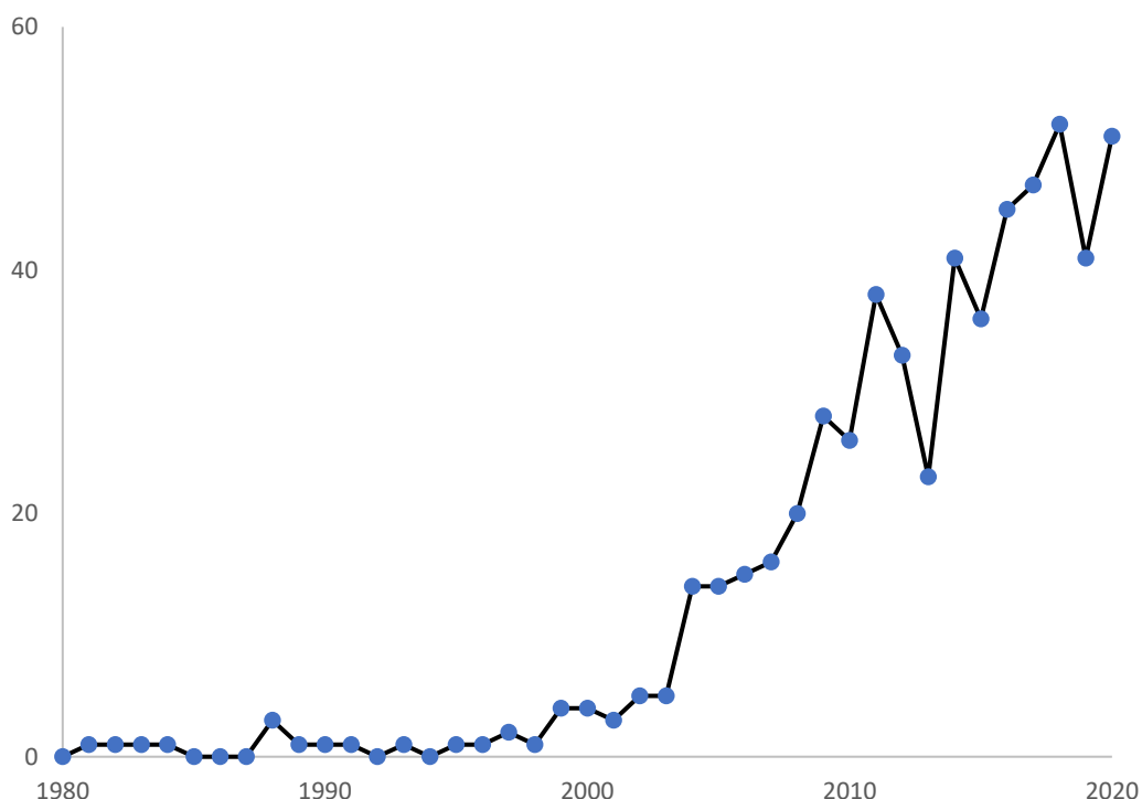
Графикон 10. Временске серије броја радова (по години) у Скопусу са цитираним низом "Бенфордов закон" у наслову чланка, или/и сажетку, или/и кључним речима
