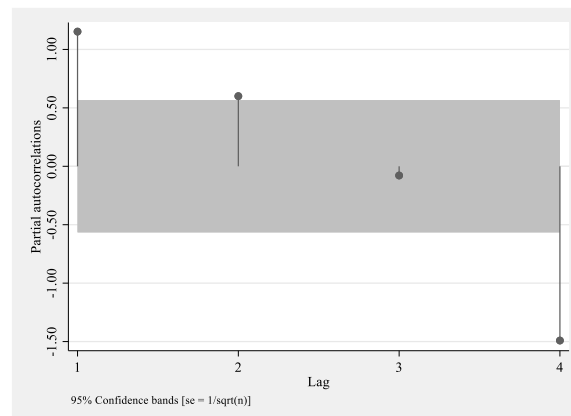
Графикон 29. PACF за бруто домаћи производ (БДП) Републике Србије
