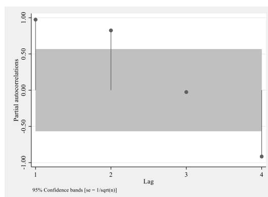
Графикон 51. PACF за извршење буџета Министарства одбране
