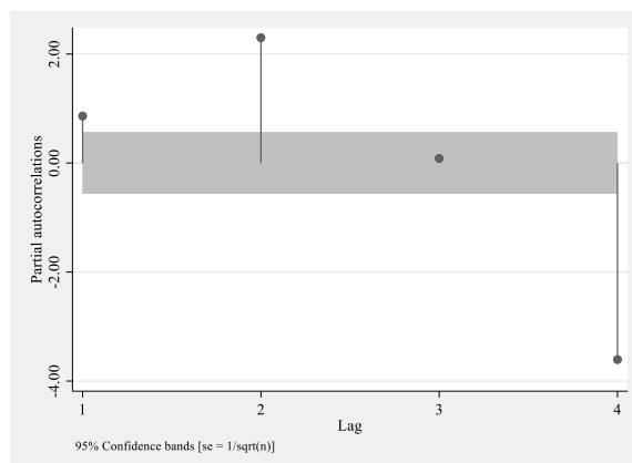
Графикон 63. PACF за извршене инвестиције у МО и ВС
