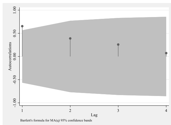
Графикон 24. ACF за консолидоване јавне приходе у буџету Републике Србије
