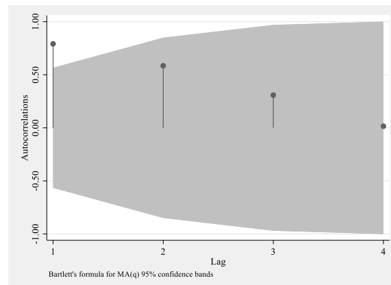
Графикон 44. ACF за број незапослених у Републици Србији
