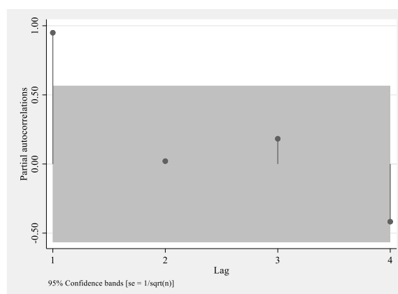
Графикон 47. PACF за стопу незапослености у Републици Србији
