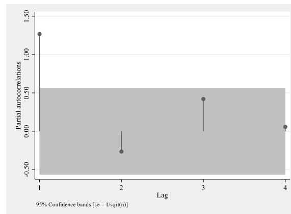
Графикон 39. PACF за просечне бруто зараде у Републици Србији
