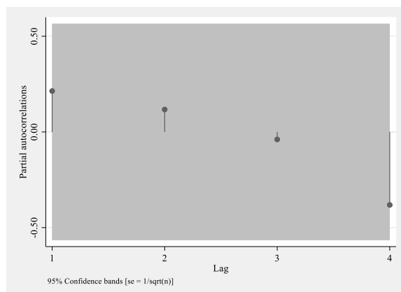
Графикон 55. PACF за проценат војне потрошње у извршењу буџета Републике Србије
