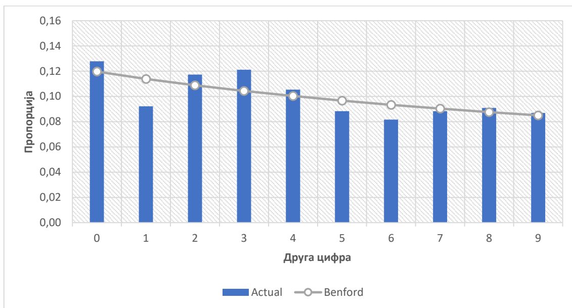
Графикон 12. Расподела друге цифре у односу на Бенфордов закон из извештаја о извршењу буџета МО и ВС
