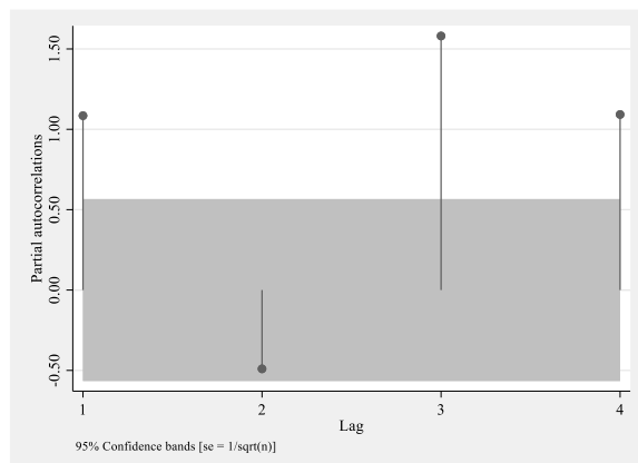
Графикон 45. PACF за број незапослених у Републици Србији
