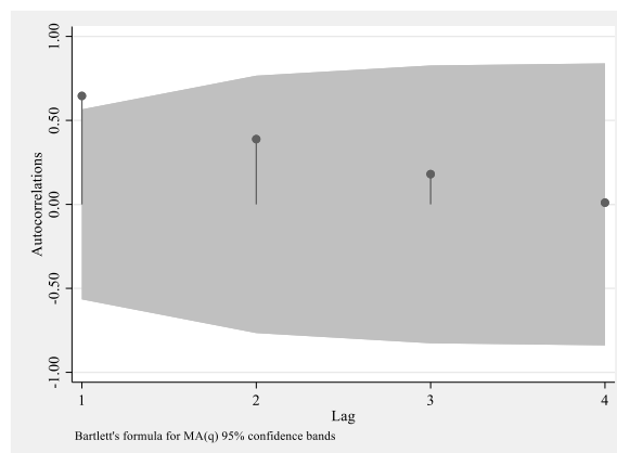
Графикон 38. ACF за просечне бруто зараде у Републици Србији
