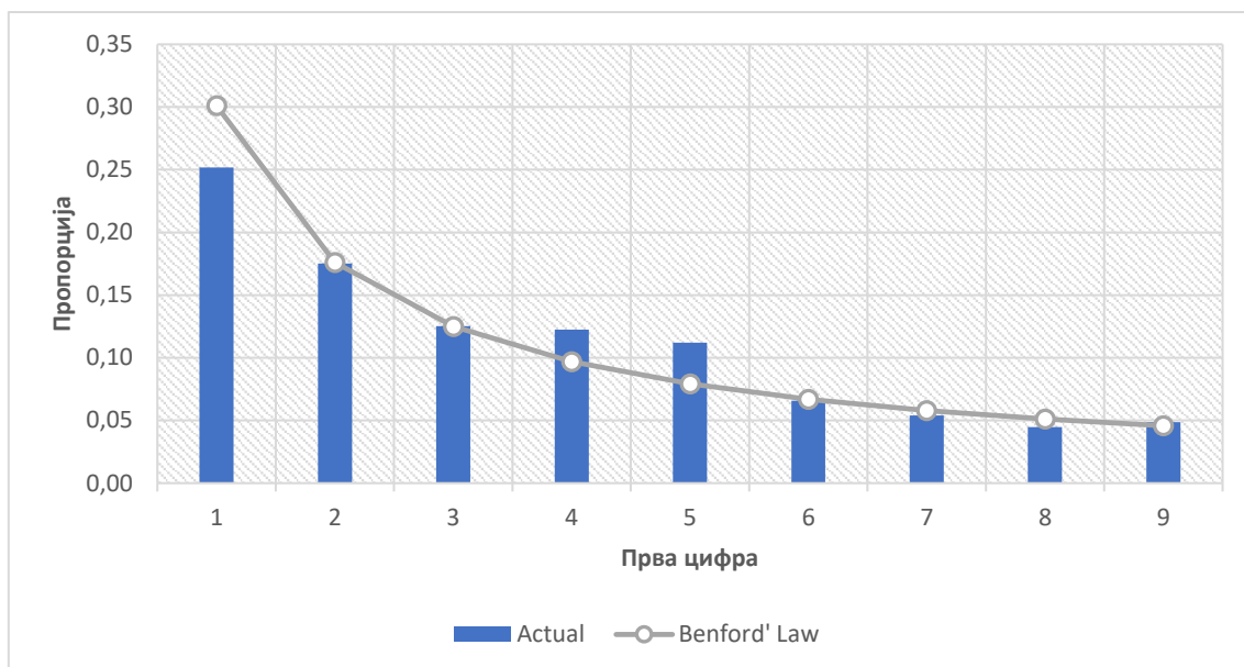
Графикон 11. Расподела прве цифре у односу на Бенфордов закон из извештаја о извршењу буџета МО и ВС
