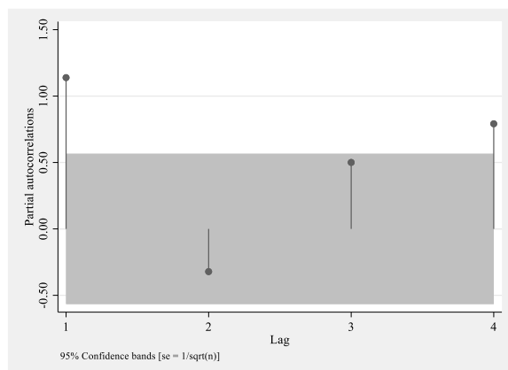
Графикон 57. PACF за планирана издвајања за плате и примања запослених у МО и ВС
