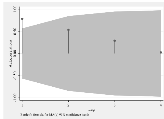
Графикон 42. ACF за број запослених у Републици Србији
