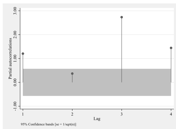
Графикон 25. PACF за консолидоване јавне приходе у буџету Републике Србије
