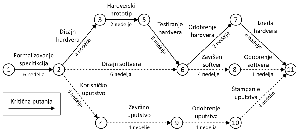
Slika 8.3. Primena PERT/CPM za projekat izrade PC ploče
