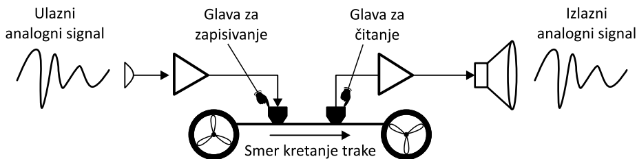
Slika 5.6. Snimanje analognog signala
