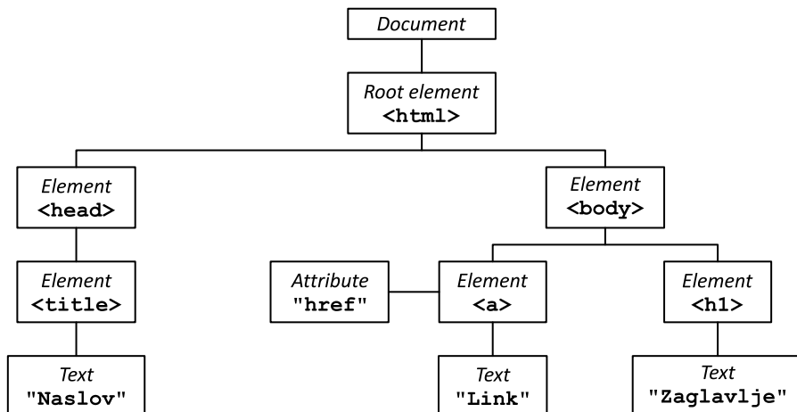
Slika 12.2. HTML DOM stablo objekata
