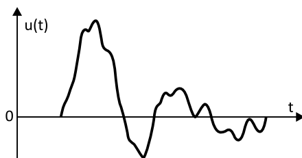
Slika 5.4. Analogni signal
