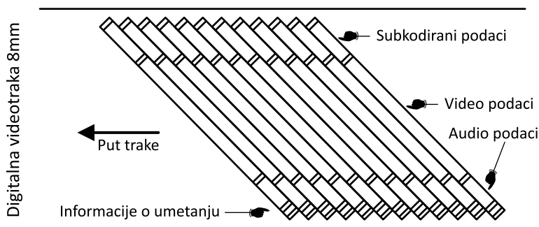
Slika 5.2. Putanja trake preko video glave za digitalno snimanje
