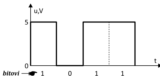
Slika 5.5. Digitalni signal
