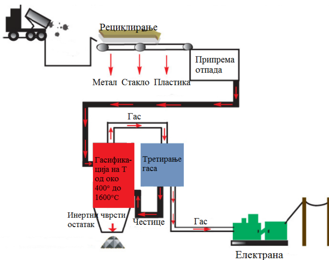
Слика 10: Шематски приказ гасификације чврстог комуналног отпада и коришћење гаса за потребе електране (197)
