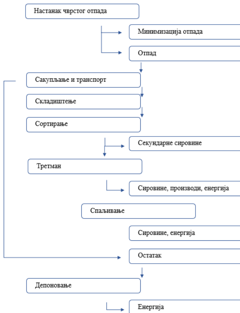
Слика 6. Систем управљања чврстим отпадом (262)
