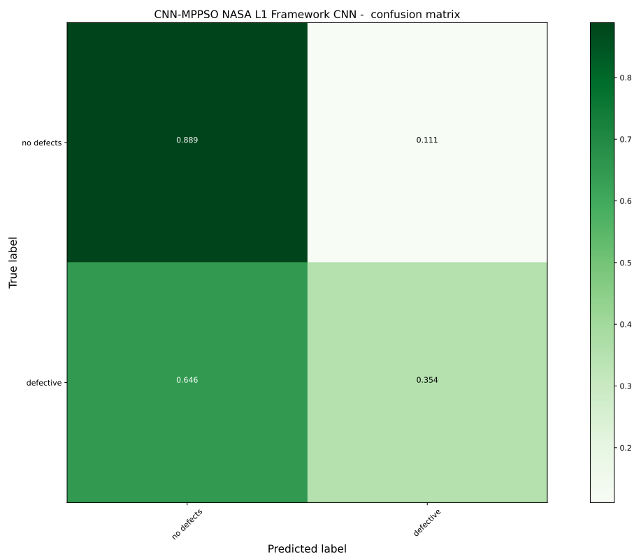
Слика 6.16: Матрица конфузије L1 CNN-MPPSO оптимизованог модела.
