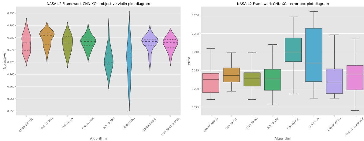
Слика 6.23: Дистрибуције циљне и индикаторске функције L2 XGBoost модела.
