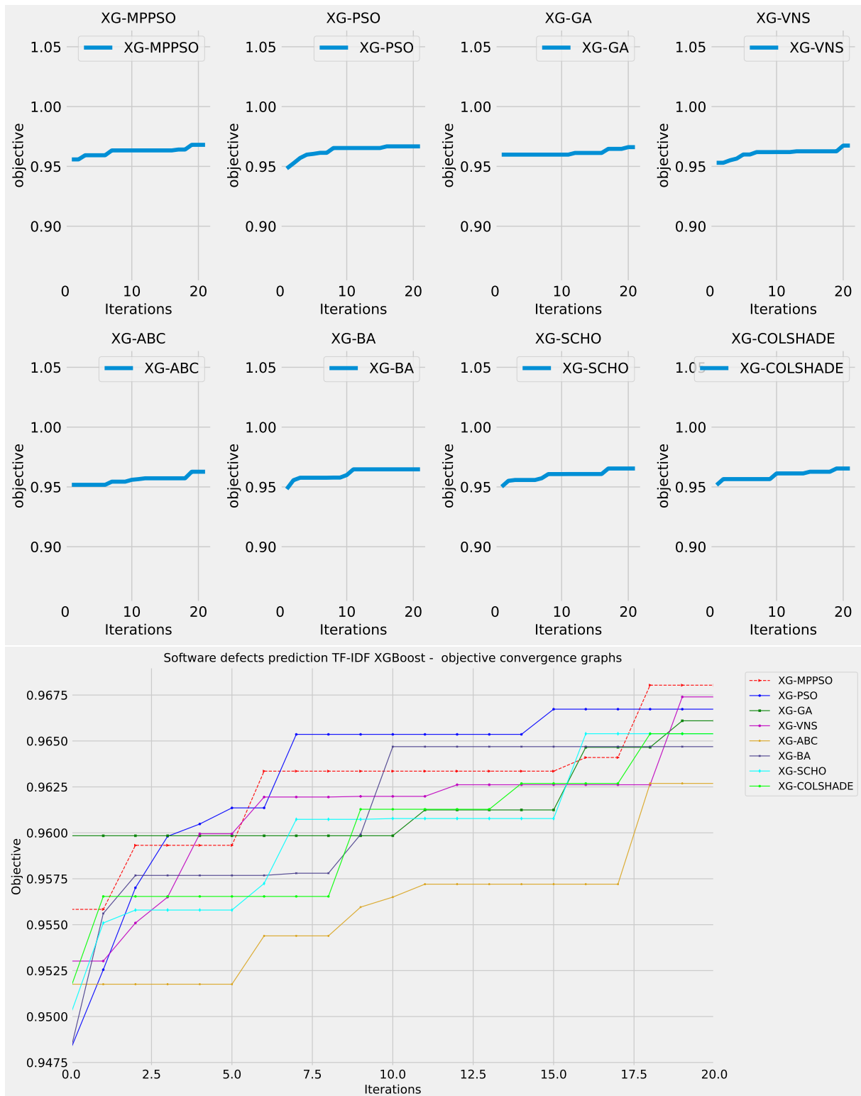
Слика 6.34: Конвергенција циљне функције NLP L2 XGBoost модела.
