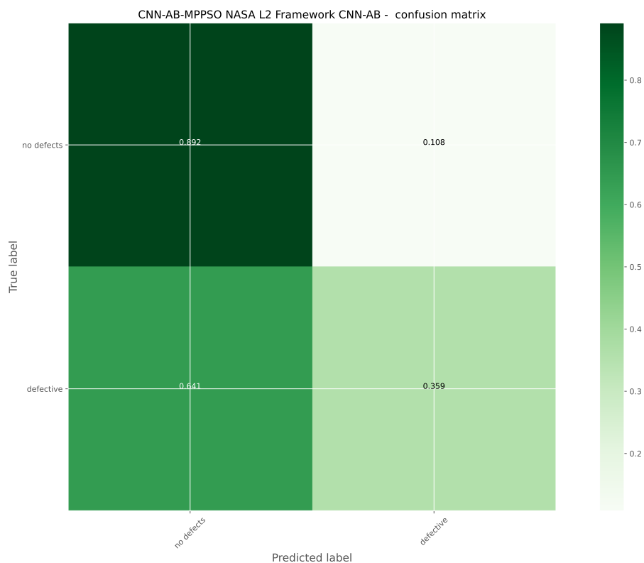
Слика 6.22: Матрица конфузије L2 AdaBoost оптимизованог L1 модела.
