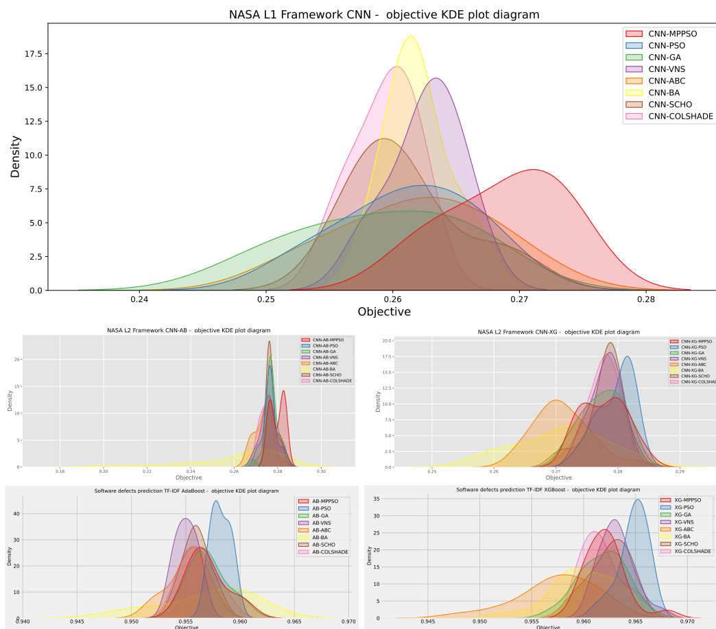
Слика 6.38: KDE дијаграми пет експеримената предвиђања софтверске грешке.
