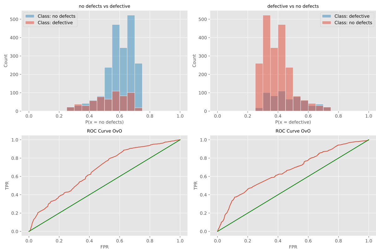
Слика 6.26: ROC крива L2 XGBoost оптимизованог L1 модела.
