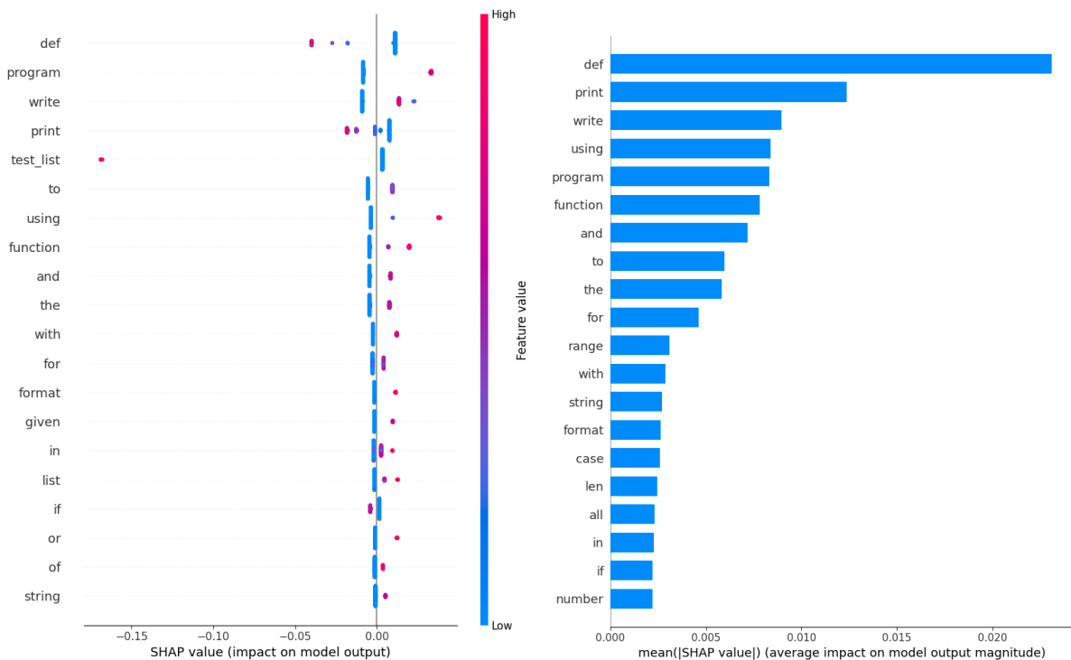
Слика 6.40: Важност обележја за најбоље modele AdaBoost на NLP скупу података.
