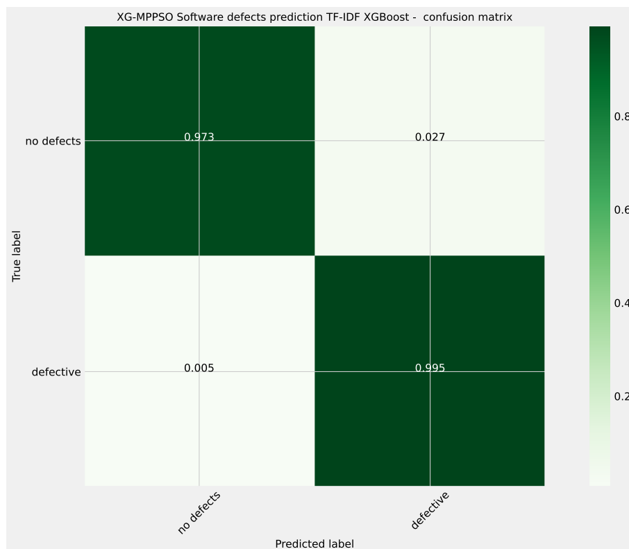
Слика 6.37: Матрица конфузије NLP L2 XGBoost оптимизованог L1 модела.
