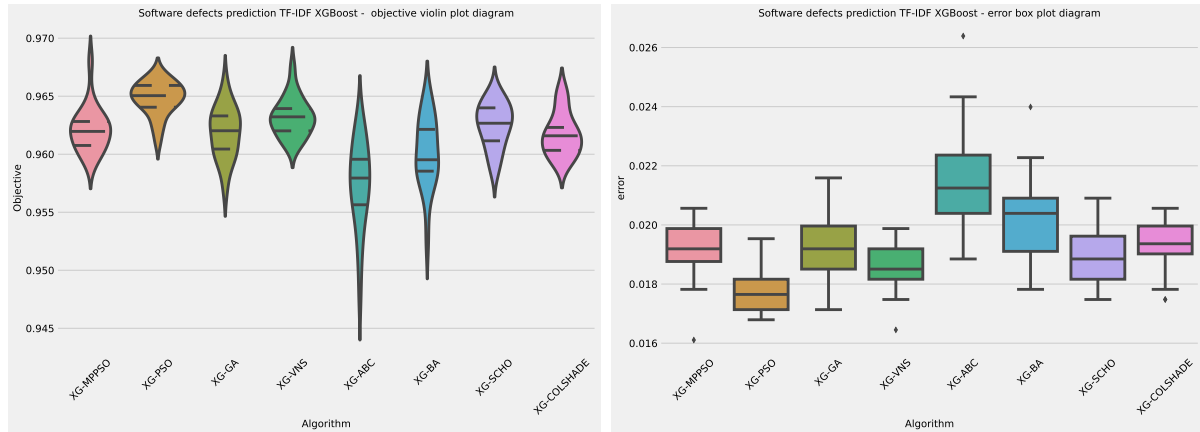
Слика 6.33: Дистрибуција циљне и индикаторске функције NLP L2 XGBoost модела.
