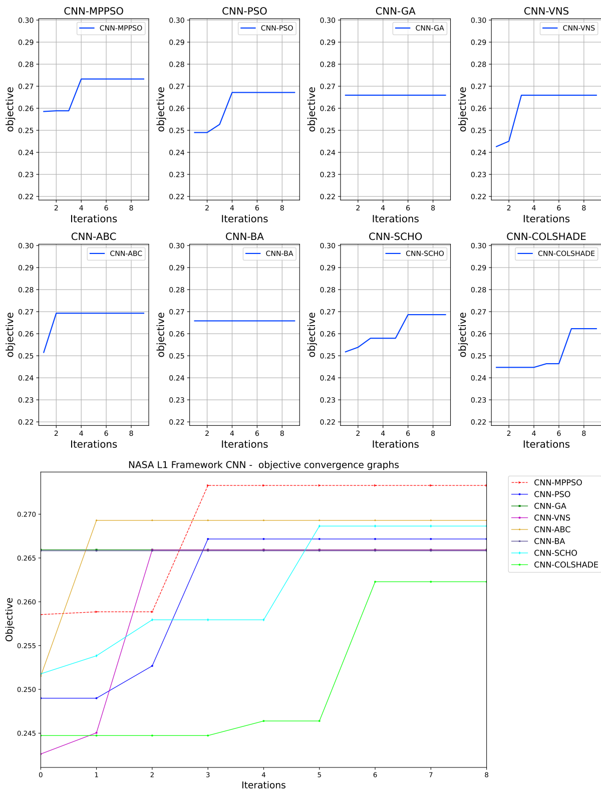
Слика 6.13: Конвергенција циљне функције L1 CNN модела.
