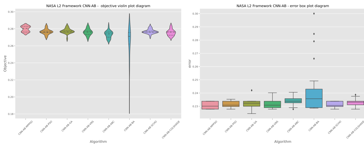
Слика 6.19: Дистрибуције циљне и индикаторске функције L2 AdaBoost модела.
