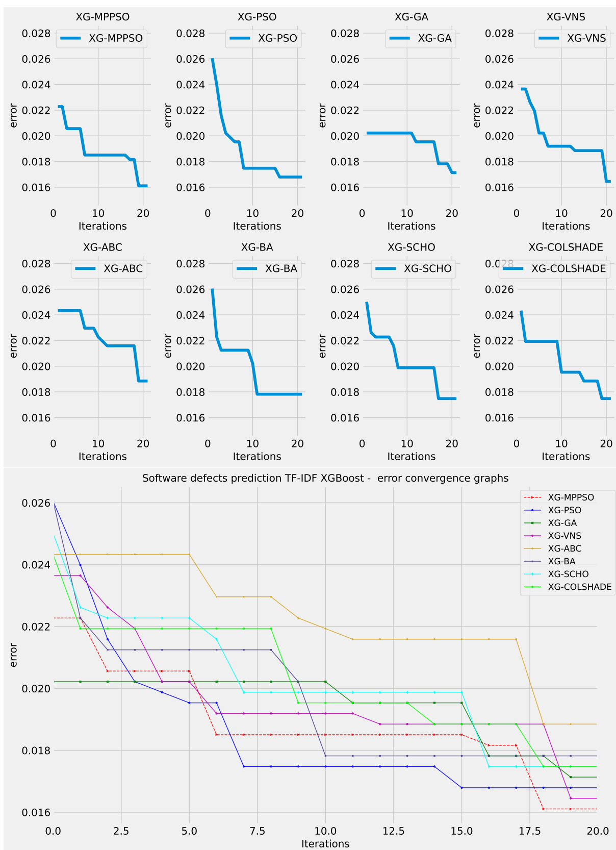
Слика 6.35: Конвергенција индикаторске функције NLP L2 XGBoost модела.
