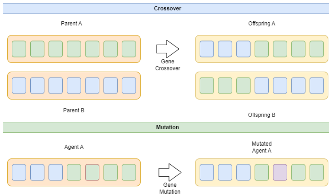
Слика 5.1: Механизми укрштања и мутације.
