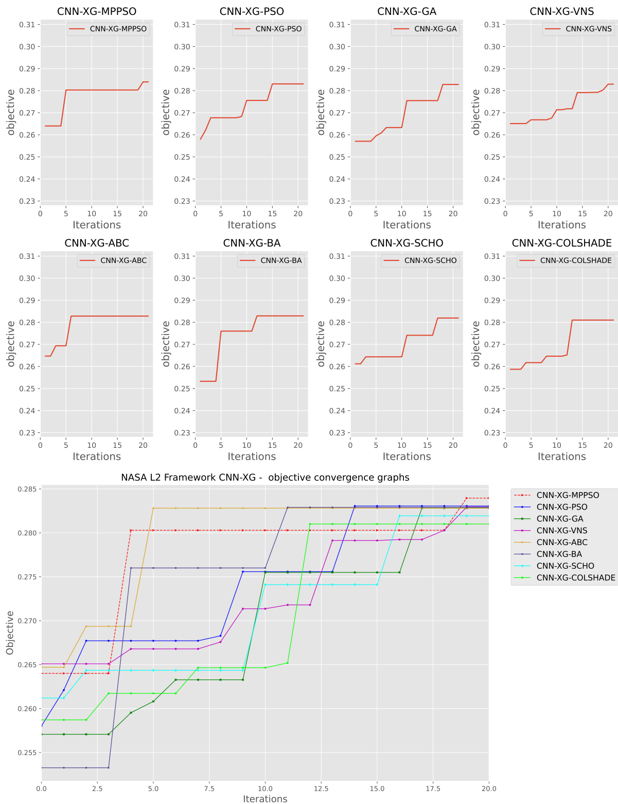
Слика 6.24: Конвергенција циљне функције L2 XGBoost модела.
