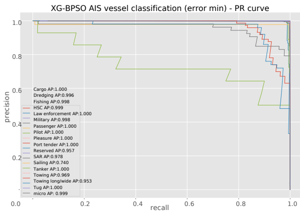
(в) Крива прецизности и одзива
