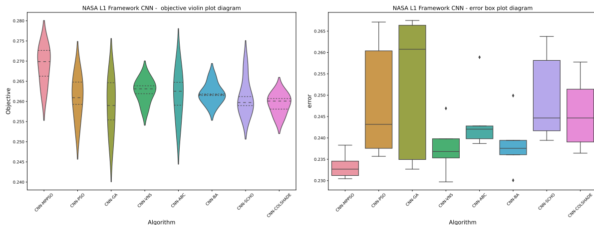
Слика 6.12: Дистрибуције циљне и индикаторске функције L1 CNN модела.
