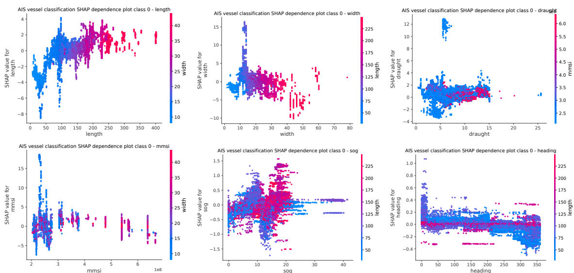
Слика 6.8: Графикони важности обележја за теретна пловила.
