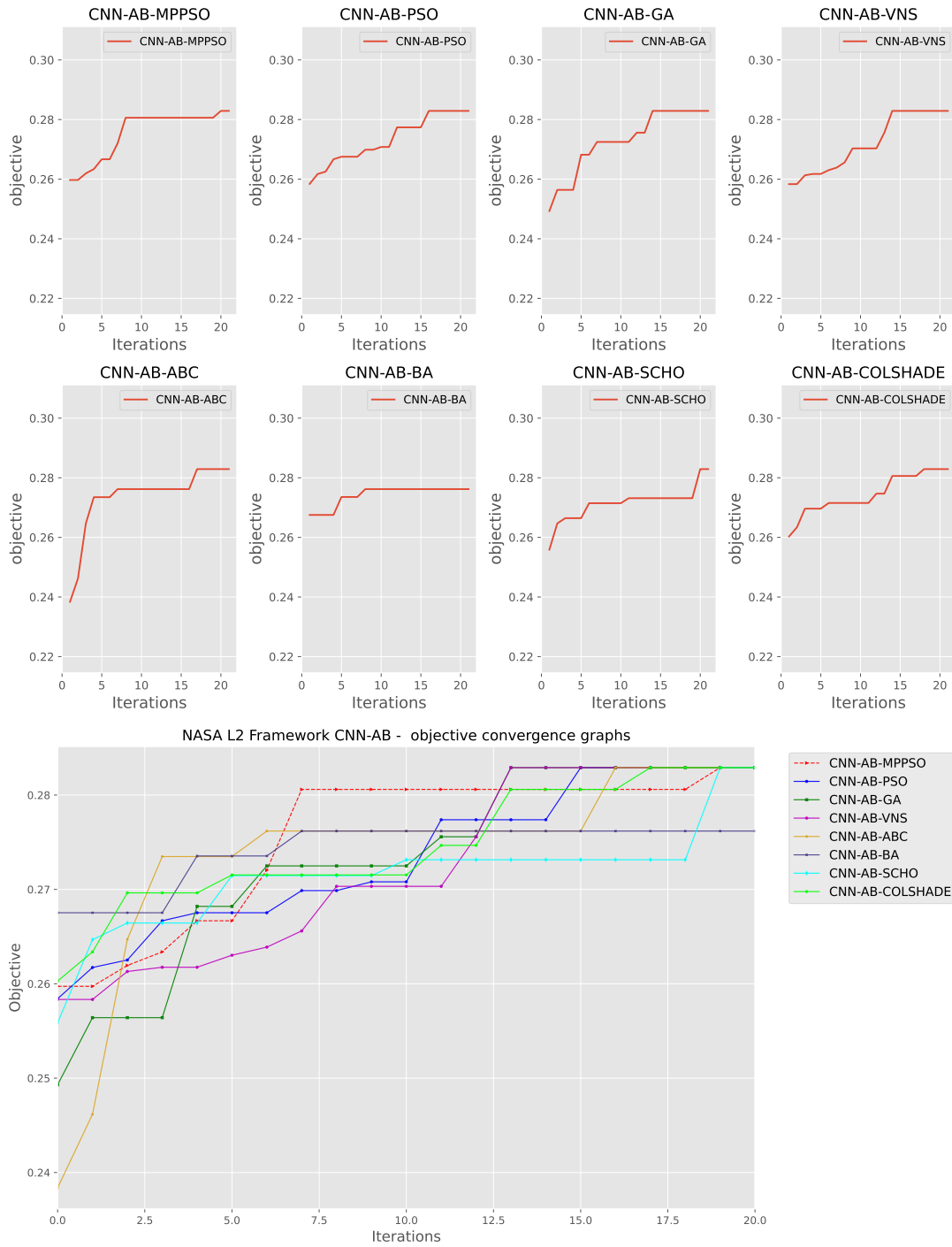
Слика 6.18: Конвергенција циљне функције L2 Adaboost модела.
