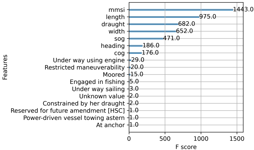
Слика 6.7: Важност обележја одређена путем XGBoost и SHAP .
