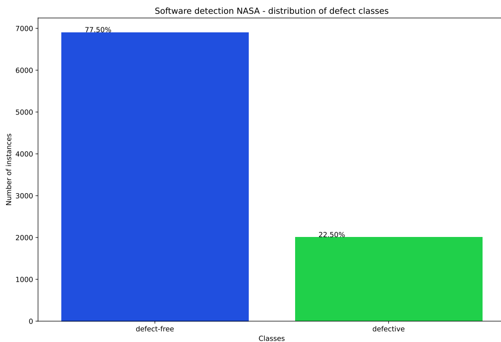
Слика 6.10: Дистрибуција класа у НАСА скупу података.
