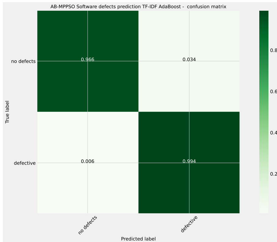
Слика 6.32: Матрица конфузије NLP L2 AdaBoost оптимизованог L1 модела.
