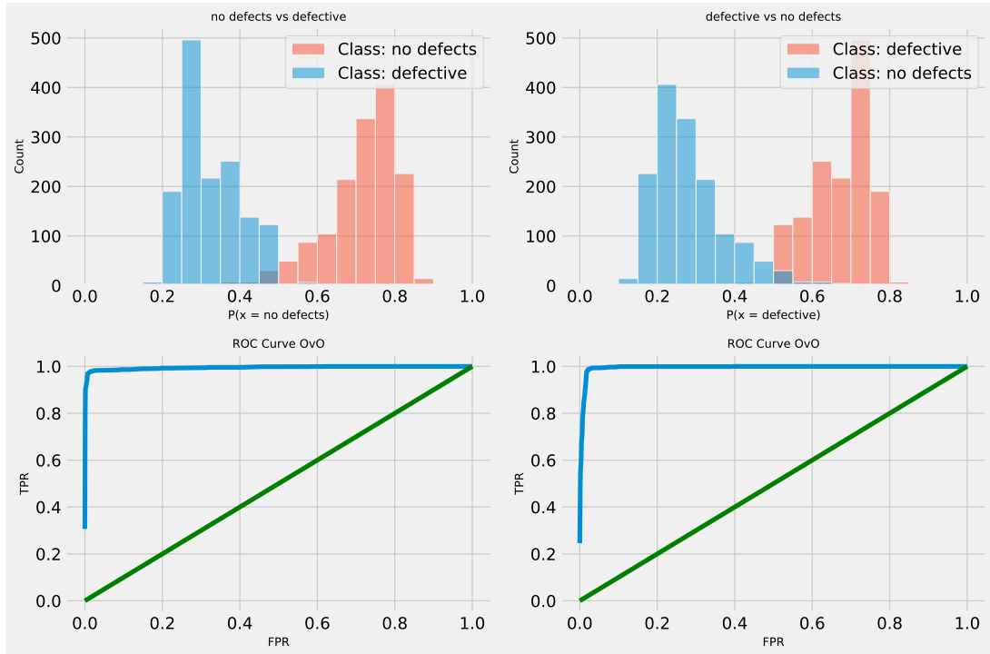
Слика 6.31: ROC крива NLP L2 AdaBoost оптимизованог L1 модела.
