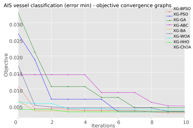
(б) Конвергенција циљне функције
