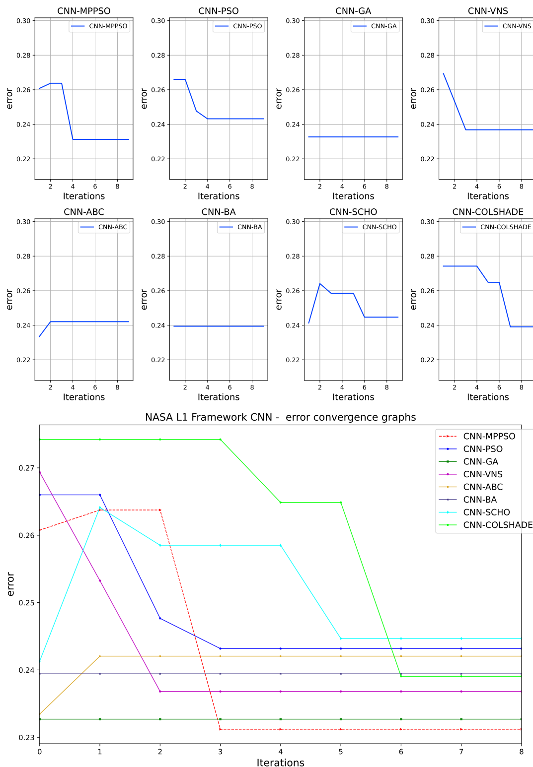
Слика 6.14: Конвергенција индикаторске функције L1 CNN модела.
