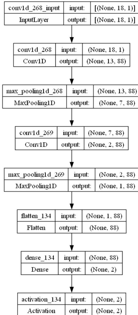
Слика 6.17: Визуелизација CNN-MPPSO оптимизованог L1 модела.
