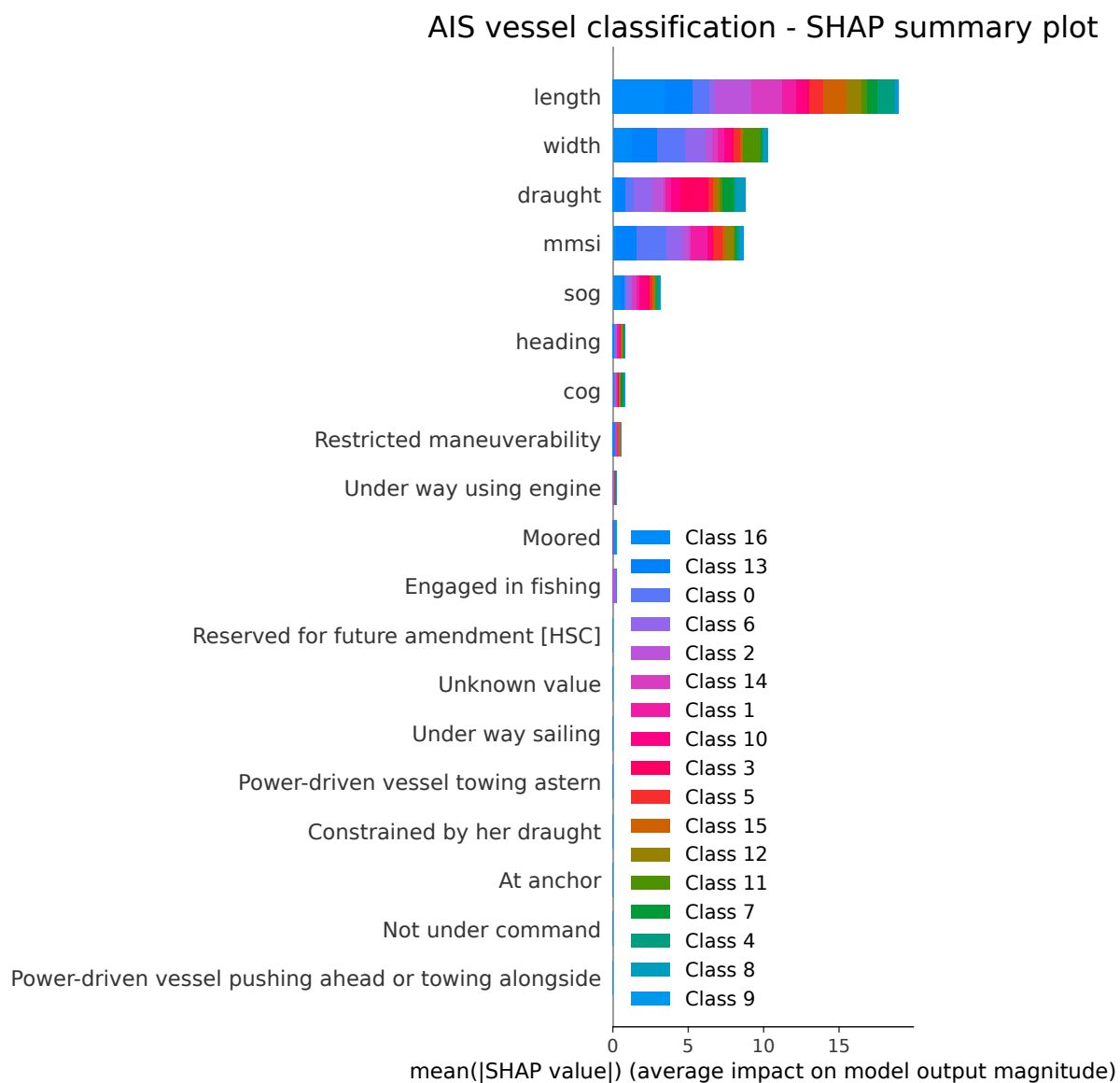
Слика 6.6: Сумарна важност обележја одређена путем XGBoost и SHAP .
