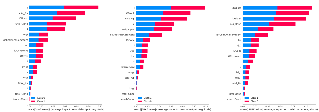
Слика 6.39: Важност обележја за најбоље modele CNN , XGBoost и AdaBoost на НАСА скупу података.
