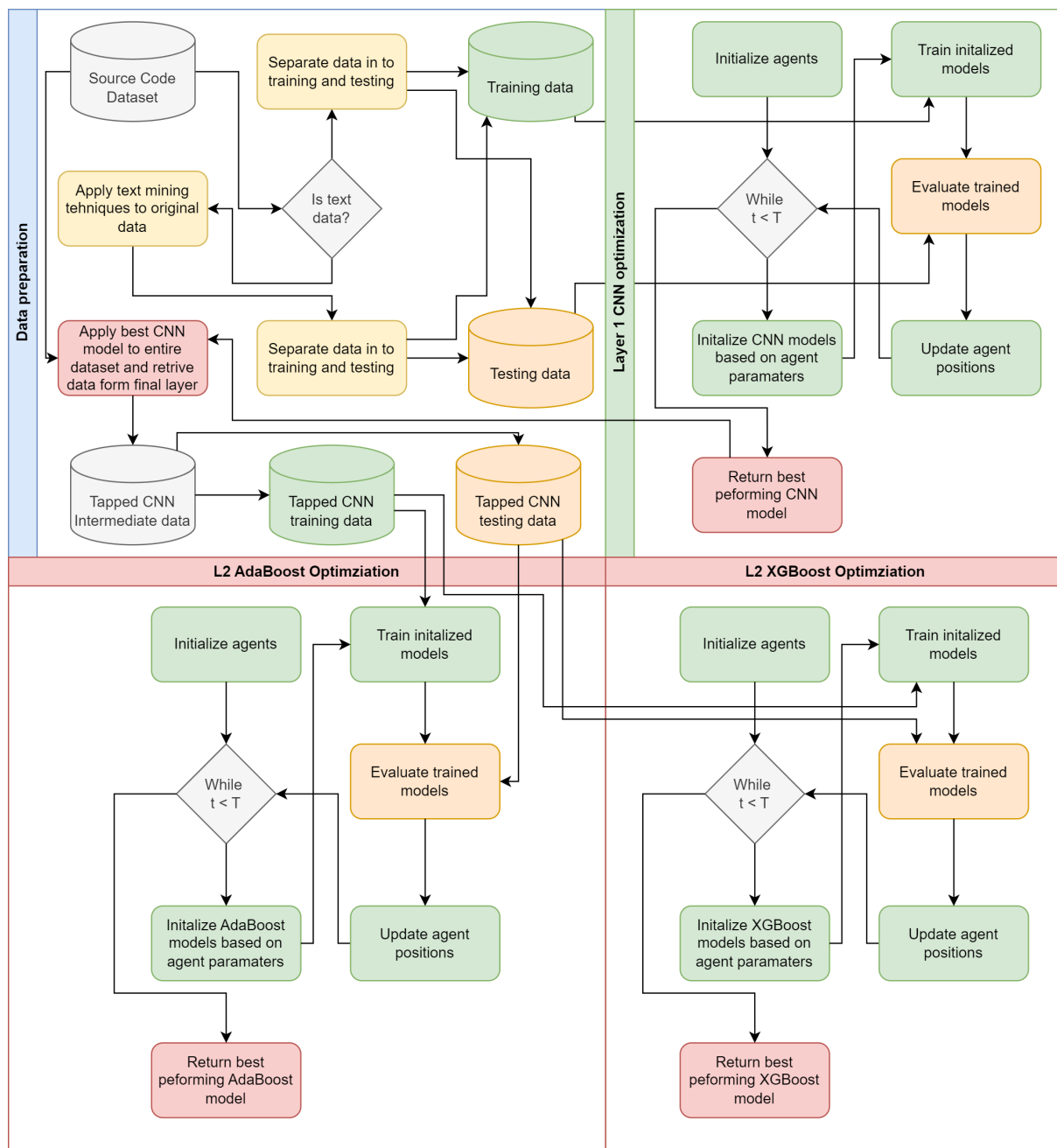
Слика 2.2: Дијаграм тока предложеног радног оквира за експерименте грешке у програмском коду.
