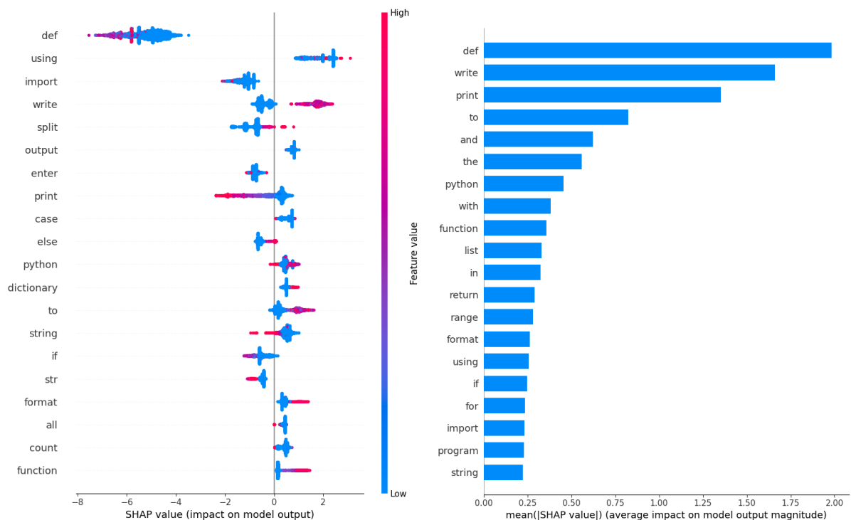
Слика 6.41: Важност обележја за најбоље моделе XGBoost на NLP скупу података.
