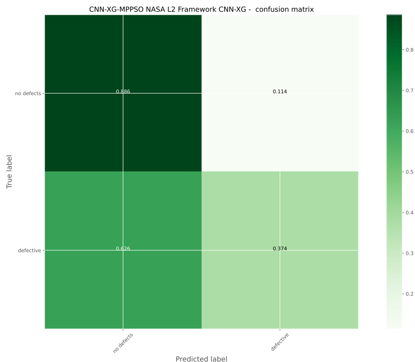
Слика 6.27: Матрица конфузије L2 XGBoost оптимизованог L1 модела.
