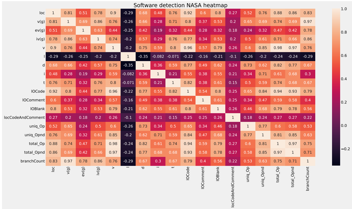
Слика 6.11: Корелација обележја у НАСА скупу података.
