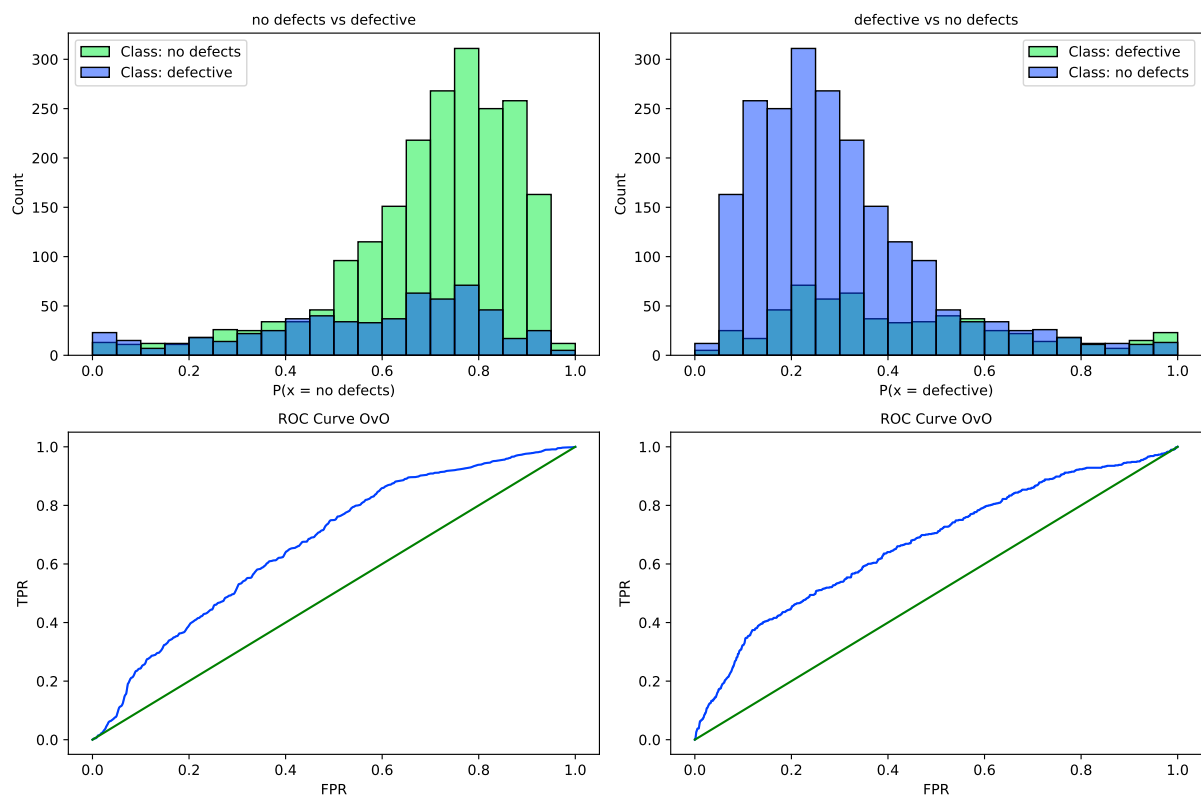
Слика 6.15: ROC крива L1 CNN-MPPSO оптимизованог модела.
