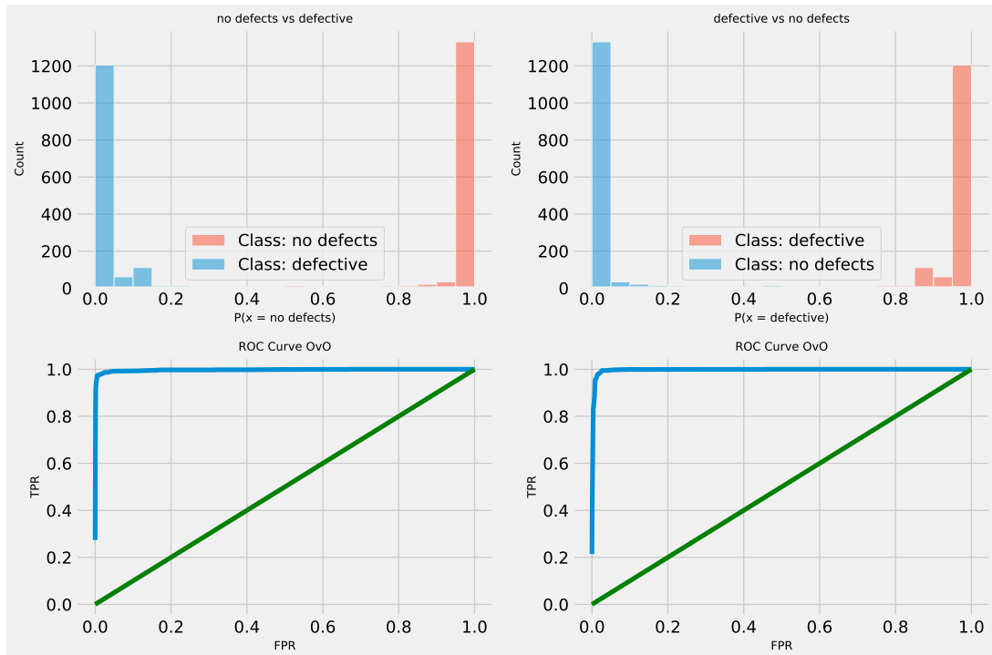
Слика 6.36: ROC крива NLP L2 XGBoost оптимизованог L1 модела.
