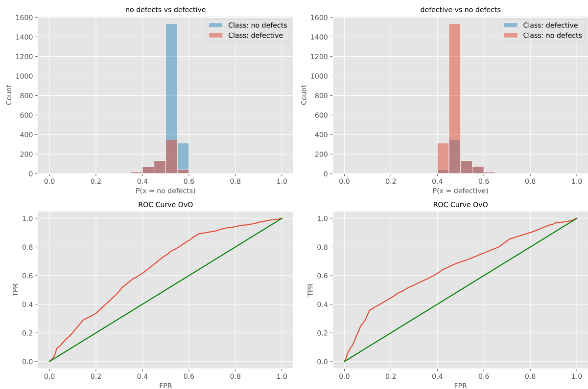
Слика 6.21: ROC крива L2 AdaBoost оптимизованог модела.
