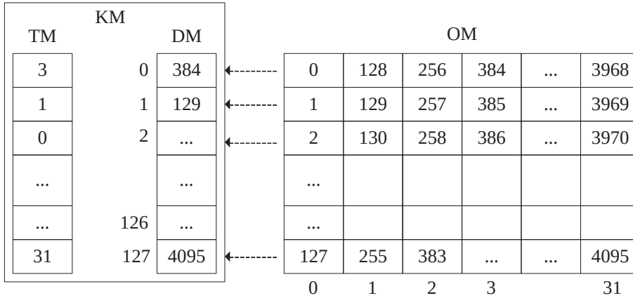
Slika 12.3 Primer direktnog preslikavanja
