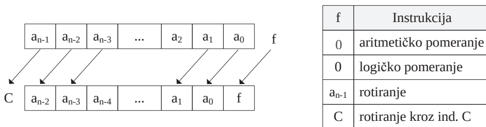
Slika 10.2 Pomeranje binarne reči ulevo
