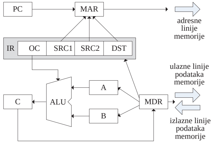
Slika 5.3 Struktura procesora
