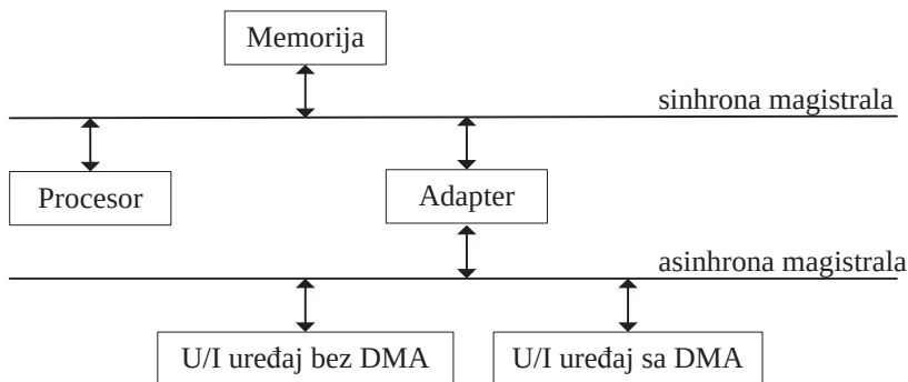
Slika 14.8 Sistem sa asinhronom i sinhronom magistralom
