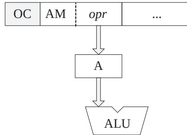
Slika 9.1 Neposredno adresiranje
