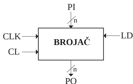
Slika 4.31 Brojač
