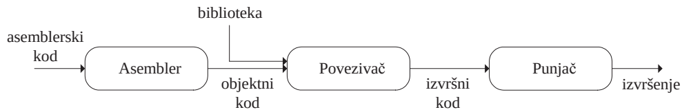
Slika 11.3 Proces pripreme asemblerskog programa za izvršenje
