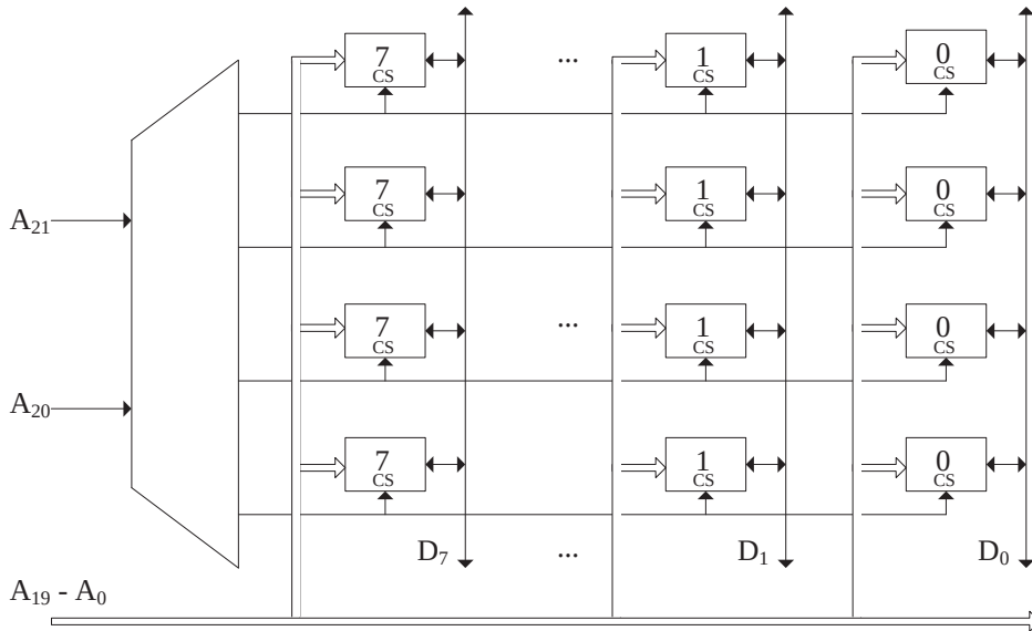
Slika 12.14 Realizacija memorijskog podsistema - primer
