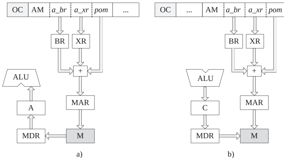
Slika 9.8 Bazno-indeksno adresiranje sa pomerajem (a) izvorišnog i (b) odredišnog operandata
