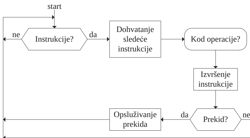
Slika 8.1 Instrukcijski ciklus
