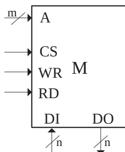
Slika 4.33 RAM memorija
