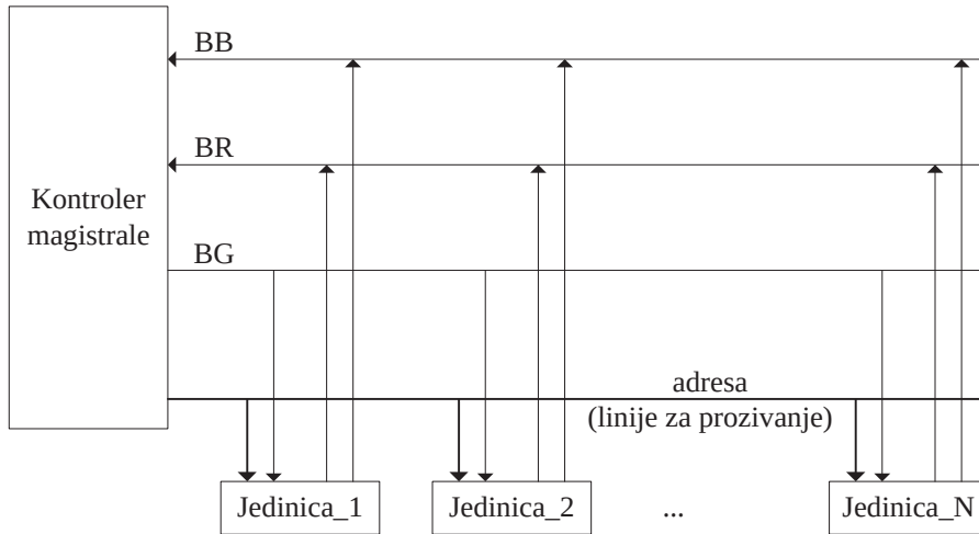
Slika 14.4 Tehnika prozivanja
