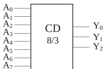
Slika 4.2 Koder 8/3
