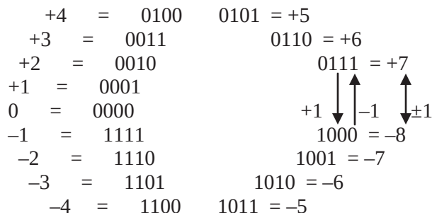
Slika 1.1 Kružna povezanost brojeva predstavljenih u komplementu dvojke
