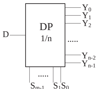
Slika 4.17 Demultiplekser 1/n
