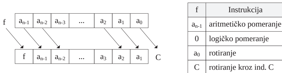
Slika 10.1 Pomeranje binarne reči udesno
