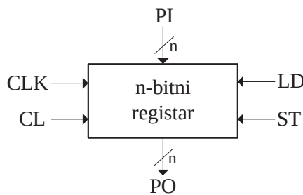
Slika 4.29 Paralelni registar
