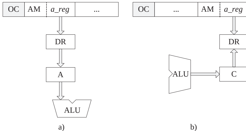
Slika 9.3 Registarsko direktno adresiranje (a) izvorišnog i (b) odredišnog operanda
