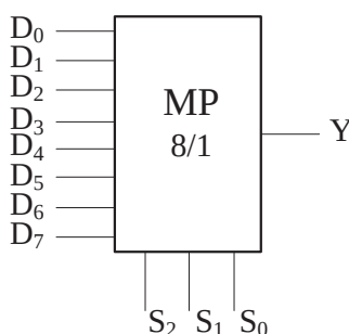
Slika 4.12 Multiplekser 8/1
