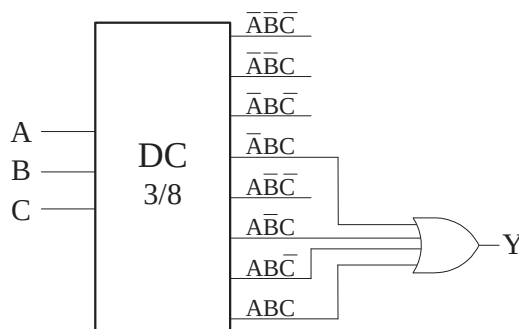
Slika 4.9 Realizacija logičke funkcije primenom dekodera 3/8
