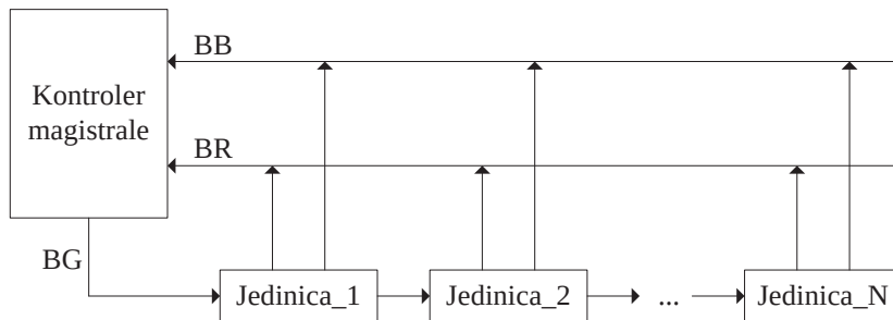
Slika 14.3 Tehnika ulančavnja
