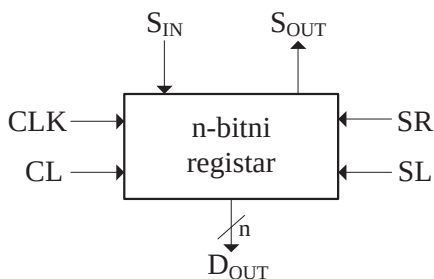
Slika 4.30 Serijski registar
