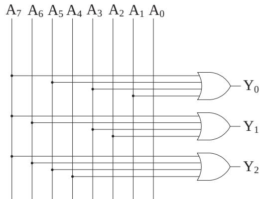
Slika 4.4 Prekidačka mreža koja realizuje koder 8/3
