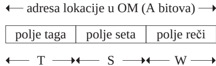
Slika 12.8 Interpretacija adrese kod set-asocijativnog preslikavanja
