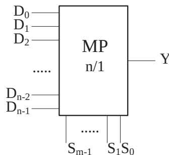
Slika 4.11 Multiplekser n/1
