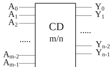
Slika 4.1 Koder m/n
