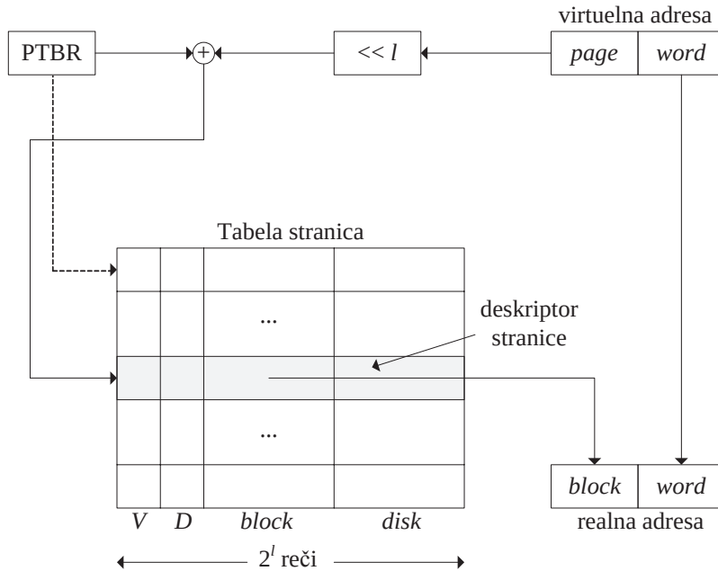
Slika 12.15 Preslikavanje virtuelne u realnu adresu
