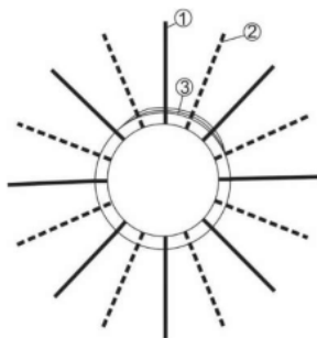
Slika I.17. Raspored injehtionih bušotina za naponsko injehtiranje (1-parni profil, 2-neparni profil, 3- kontaktno injehtiranje)
