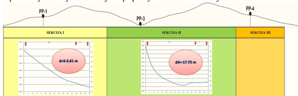
Slika IV.63. Sniženja nivoa podzemnih voda u reprezentativnom piježometru, kroz Sekcije za ceo period (21/9/2016 – 21/10/2016)
