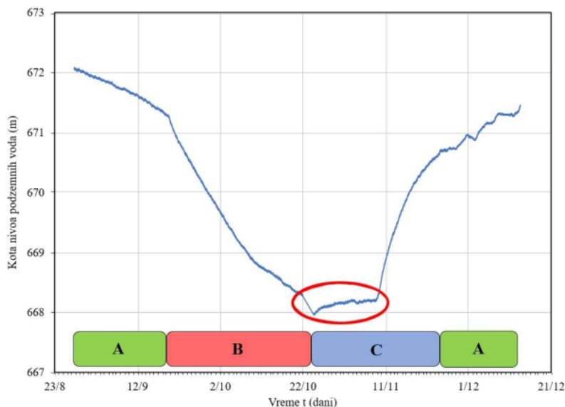
Slika IV.41. Oscilacije nivoa podzemnih voda u piježometru PP-1 (interval osmatranja na 2 minuta) kroz različite režime rada tunela: A, B i C (crveni krug označava blagi porast nivoa u toku faze C)
