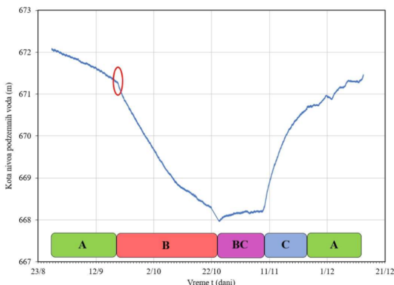
Slika IV.50. Segment merenja sumarnih gubitaka u odnosu na ceo osmatrački period promene nivoa podzemnih voda u pijeziometru PP-1 označen crvenom bojom
