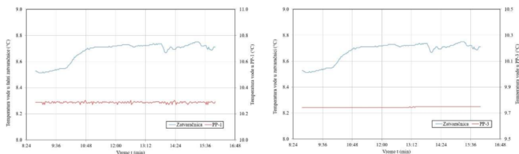
Slika IV.35. Promena temperature voda u tunelskoj zatvaračnici i pijeziometrima PP-1 i PP-3, na stepenicama držanja nivoa u toku merenja sumarnih gubitaka na 2 minuta
