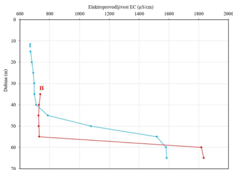
Slika IV.71. Promena vrednosti EC podzemnih voda po dubini u pijezometaru PP-3 (I - pre merenja sumarnih gubitaka, II - nakon merenja sumarnih gubitaka)
