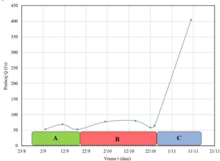
Slika IV.9. Hidrogram Dobrodolske reka na mernom profilu 1
