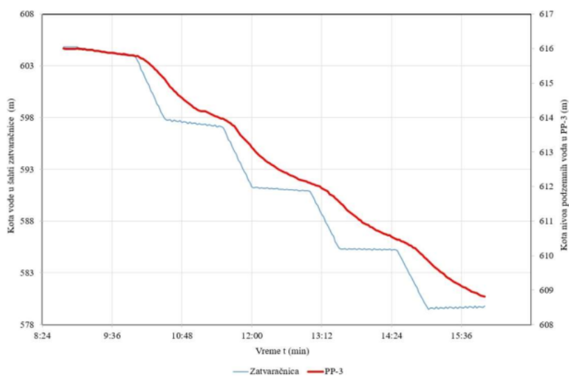
Slika IV.53. Promena nivoa vode u zatvaračnici i pijeziometru PP-3 za vreme merenja sumarnih gubitaka [17]
