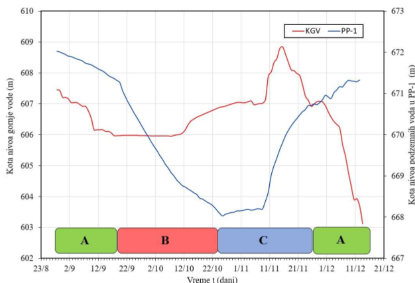
Slika IV.40. Uporedni dijagram promene nivoa podzemnih voda u PP-1 i koti gornje vode akumulacionog jezera (interval osmatranja na 6 časova) kroz različite režime rada tunela: A, B i C [17], [40]
