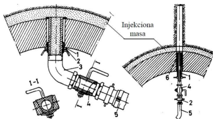
Slika I.16. Sema injehtiranja: (1) – otvor u oblozi, (2) – muf, (3) – cev, (4) – ventil, (5) – crevo, (6) – gumeni zaptivač (2,3,4 ima naziv „paker“) [88]
