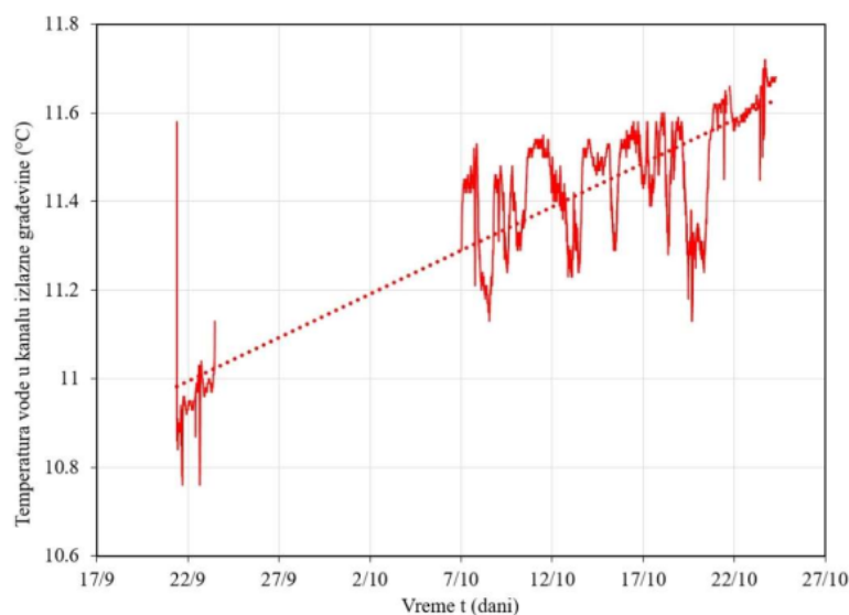
Slika IV.36. Promena temperature vode na kanalu izlazne građevine (interval osmatranja 2 minuta)
