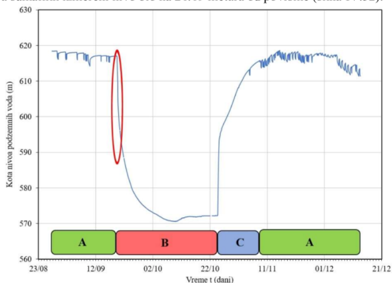
Slika IV.52. Segment merenja sumarnih gubitaka u odnosu na ceo osmatrački period promene nivoa podzemnih voda u pijeozmetru PP-3 označen crvenom bojom
