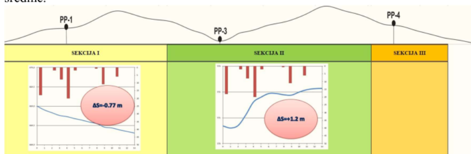
Slika IV.67. Snižjenja nivoa podzemnih voda u reprezentativnom pijeziometru, kroz Sekcije za II period (7/10/2016 – 21/10/2016)
