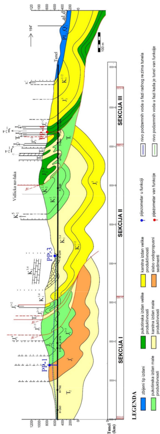
Slika IV.60. Geološki profil tunela sa prikazom sekcija merenja dotoka i osmatračkim piježometrima [17]
