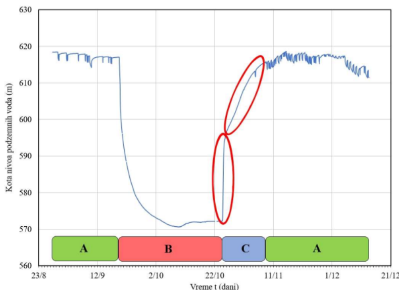
Slika IV.47. Oscilacije nivoa podzemnih voda u pijezometru PP-3 (interval osmatranja na 2 minuta) kroz različite režime rada tunela: A, B i C, sa posebnim akcentom na fazu C
