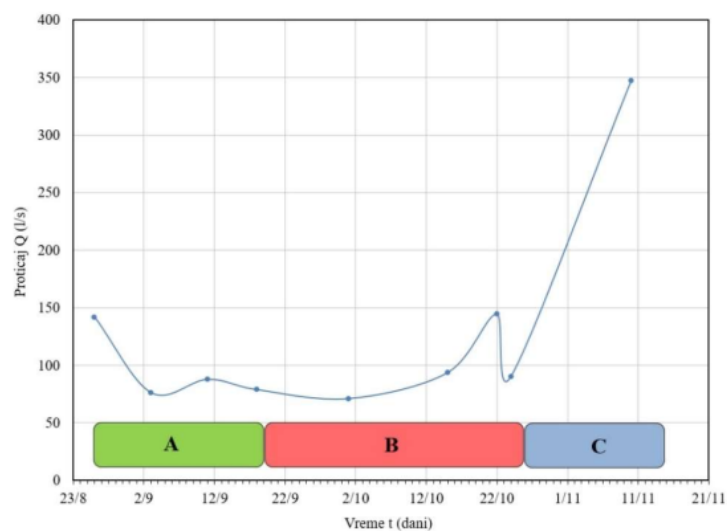
Slika IV.12. Hidrogram Dobrodolske reka na mernom profilu 2
