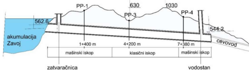
Slika II.2. Podužni profil tunela HE Pirot, sa prikazom tipa iskopa i polažaja pijezometara na trasi tunela [17]
