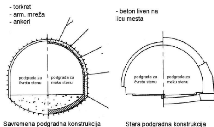
Slika I.15. Uporedni prikaz nove i stare podgradne konstrukcije [88]
