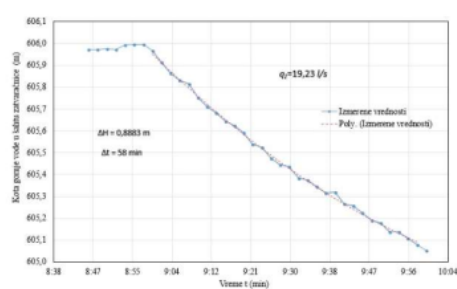
Slika IV.28. I stepenica merenja sumarnih gubitaka u tunelu za t – 38 min i t- 58 min
