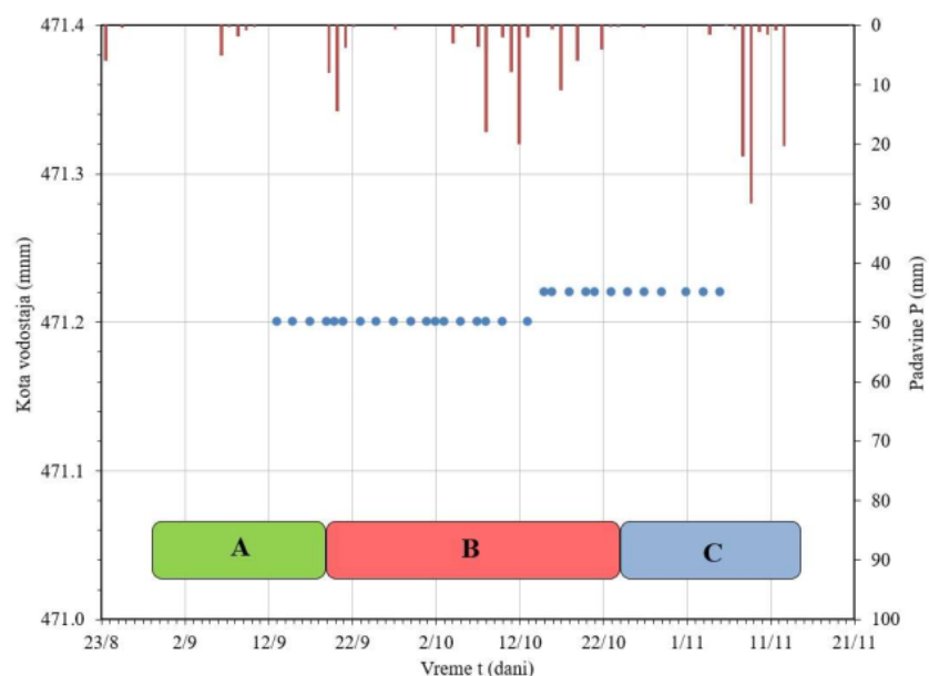
Slika IV.8. Nivogram Dobrodolske reka na vodomernom profilu 1
