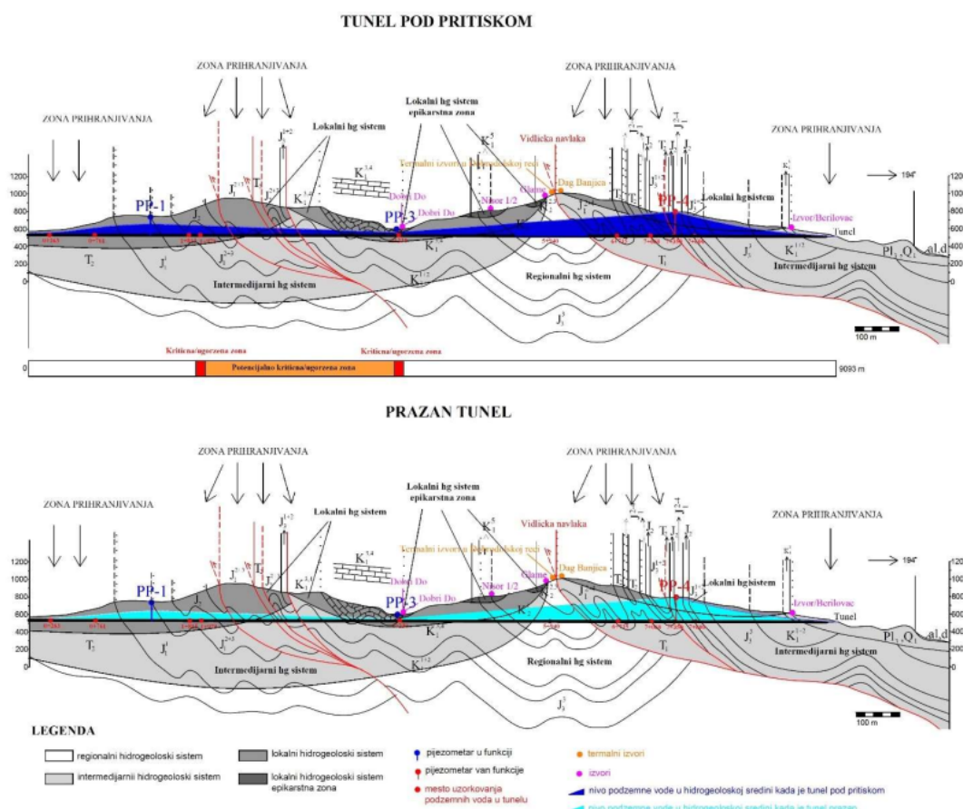
Slika V.3. Konceptualni model uticaja tunela pod pritiskom na kompleksni hidrogeološki sistem
