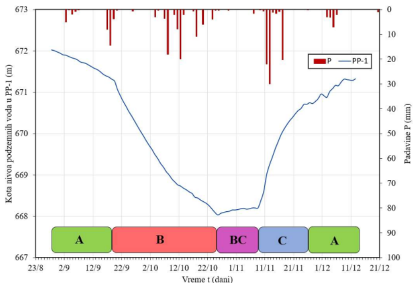
Slika IV.43. Formiranje nove faze - BC kod analize kvantitativnih karakteristika podzemnih voda u pijeziometru PP-1 sa prikazom uticaja padavina na promenu podzemnih voda u PP-1 (interval osmatranja 1 dan) kroz različite režime rada tunela: A, B i C
