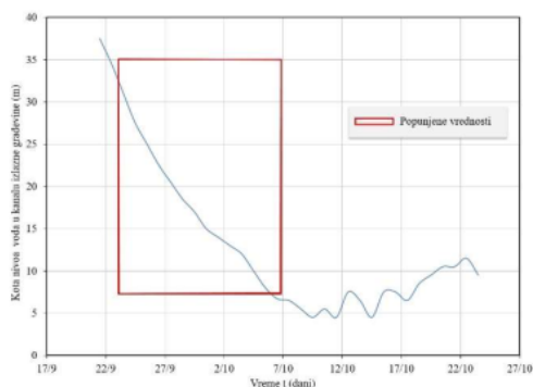
Slika IV.57. Popunjene vrednosti vodostaja na kanalu izlazne građevine
