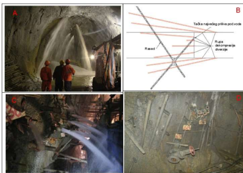
Slika I.19. A – Dotok podzemnih voda pod pritiskom u toku iskopa tunela. B – Diverzija (preusmeravanje) dekomprisijskim injektiranjem radi blokiranja dotoka podzemnih voda. C – Primer koncentrisanih tačaka dotoka podzemnih voda pre i posle (D) tretmana [101].
