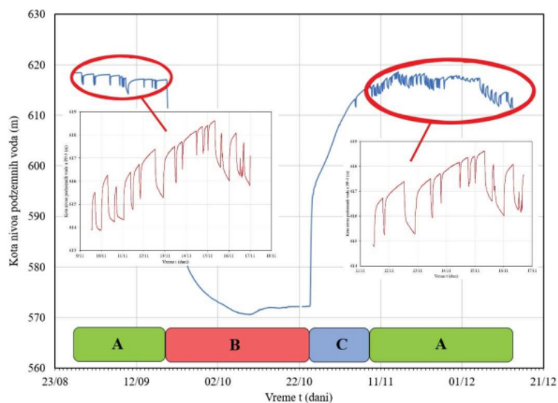
Slika IV.48. Oscilacije nivoa podzemnih voda u pijeometru PP-3 (interval osmatranja na 2 minuta) tokom faze A pod uticajem rada hidrotehničkog tunela [17]
