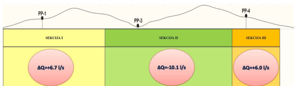
Slika IV.64. Promene vrednosti dotoka kroz Sekcije za I period (21/9/2016 – 7/10/2016)
