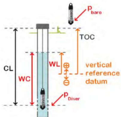
Slika III.2. Postupak barokompenzacije podataka o nivoima podzemnih voda registrovanih dajverima (Diver manual, 2014, Schumberger water services, Eijkelkamp)
