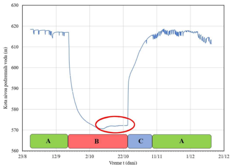
Slika IV.45. Oscilacije nivoa podzemnih voda u pijeziometru PP-3 (interval osmatranja na 2 minuta) kroz različite režime rada tunela: A, B i C, sa posebnim akcentom na fazu B
