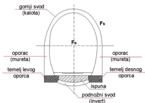
Slika I.8. Elementi poprečnog preseka podzemnog objekta/tunela [87]
