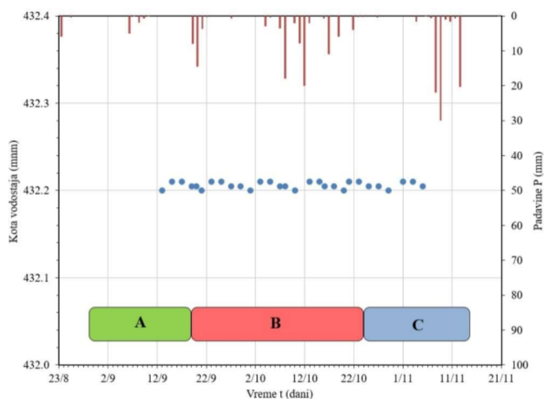
Slika IV.11. Nivoogram Dobrodolske reka na mernom profilu 2
