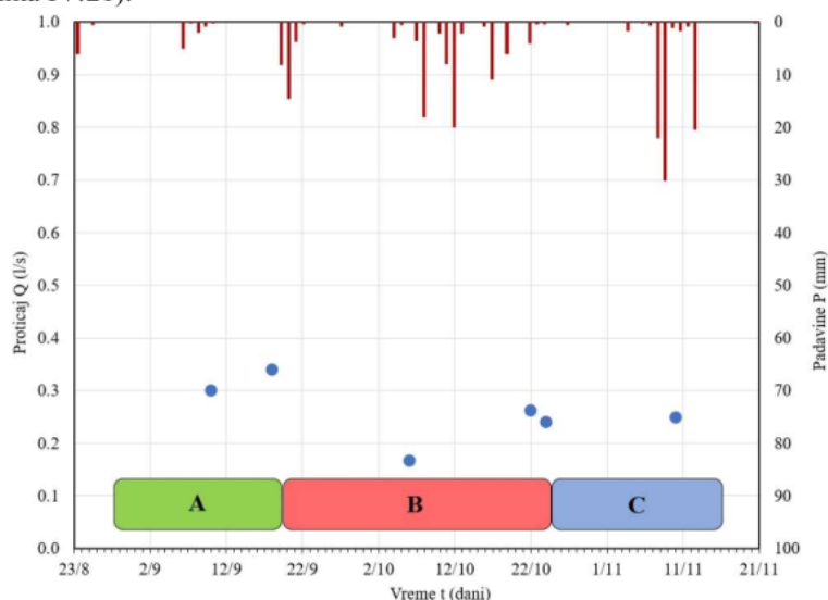
Slika IV.21. Hidrogram izvora Dobri Do u zavisnosti od padavina kroz različite režime rada tunela: A, B i C [104]
