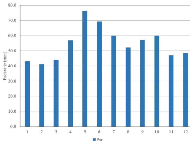
Slika II.5. Unutargodišnja raspodela padavina za period 1990-2016
