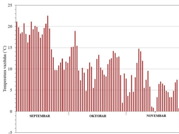
Slika IV.4. Dnevne temperature vazduha za period septembar-novembar 2016. godine
