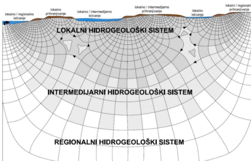
Slika I.3. Hidrogeološki sistemi sa zonama prihranjivanja i isticanja
