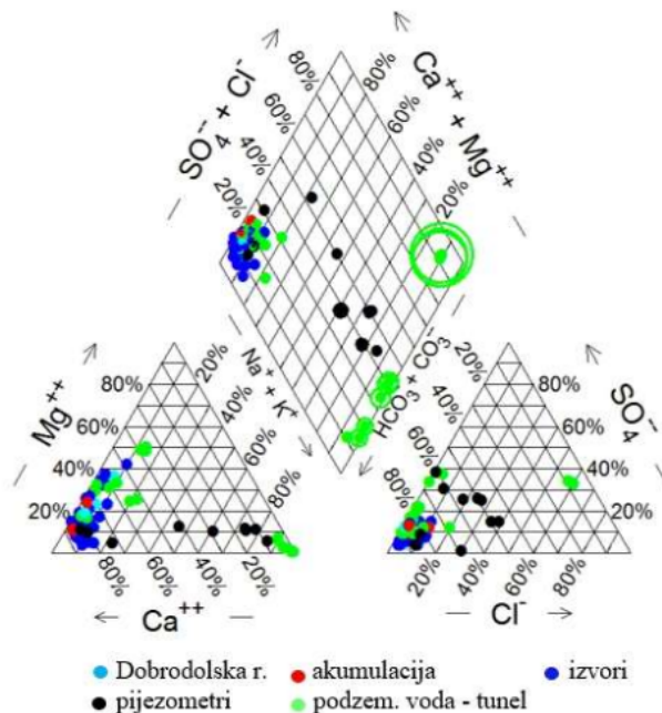
Slika IV.79. Pajperov dijagram hemijskog sastava voda svih uzorkovanih voda (izvori, pijezometri, tunel)
