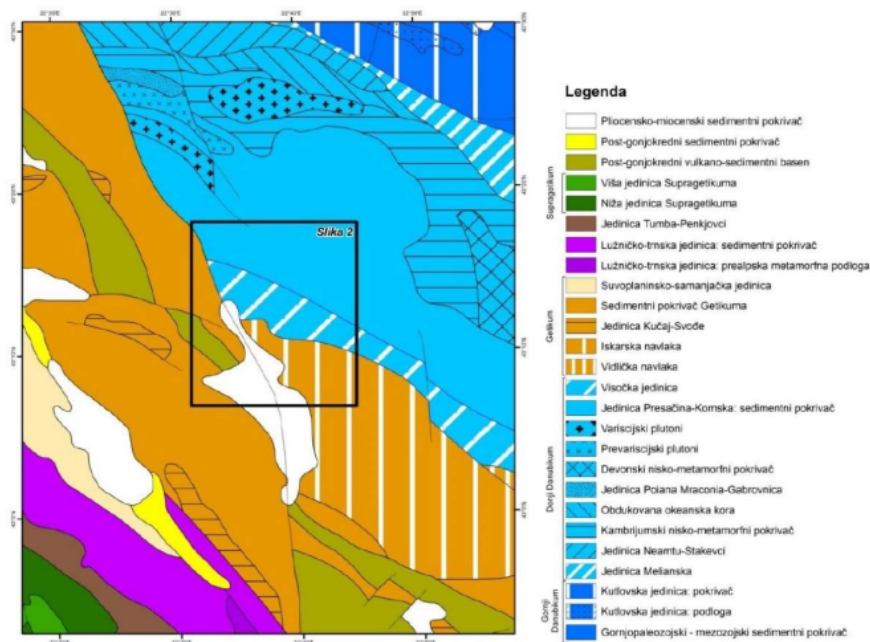
Slika II.7. Geotektonski položaj istraživnog područja [50], [39]
