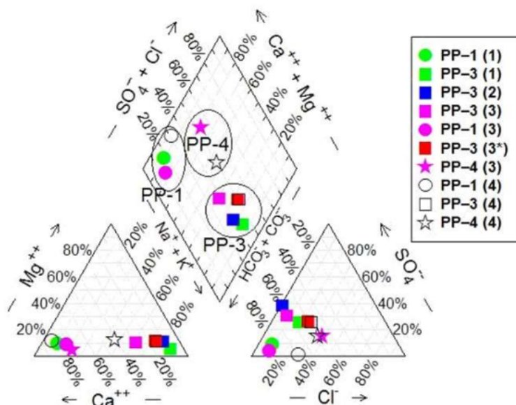
Slika V.3. Pajperov dijagram hemijskog sastava podzemnih voda iz pijeziometara PP-1, PP-3 i PP-4. Legenda: uzorkovanja izvršena (1) – A; (2) – B; (3/3*) – C; (4) – A [40]
