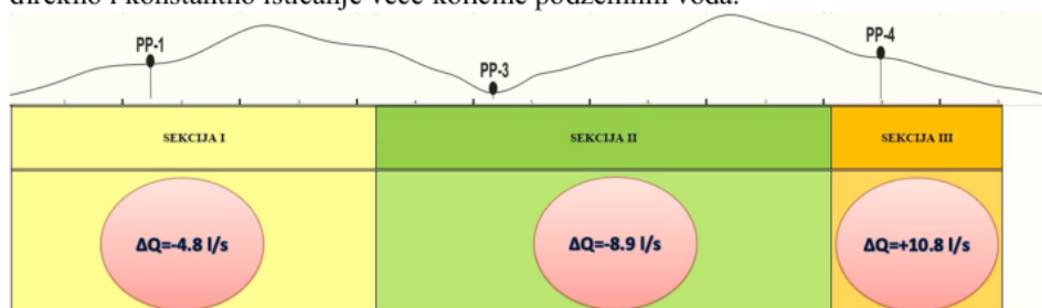
Slika IV.62. Promene vrednosti dotoka kroz Sekcije za ceo period (21/9/2016 – 21/10/2016)
