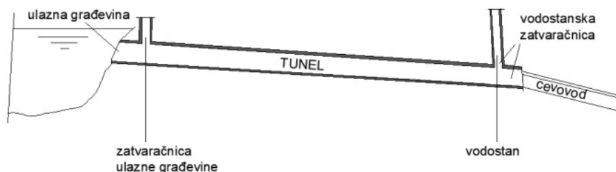
Slika I.18. Šema osnovnih objekata tunela pod pritiskom
