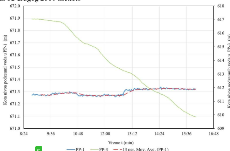
Slika IV.54. Promena nivoa podzemnih voda u piježometrima PP-1 i PP-3 za vreme merenja sumarnih gubitaka
