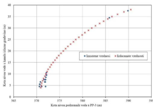
Slika IV.56. Dijagram izmerenih i izračunatih vrednosti vodostaja na kanalu izlazne građevine i piježometru PP-3
