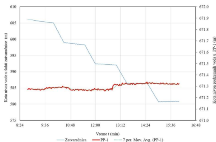
Slika IV.51. Promena nivoa vode u zatvaračnici i pijeozmetru PP-1 za vreme merenja sumarnih gubitaka
