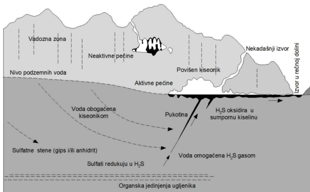
Slika I.6. Stvaranje gasa H_2S u uslovima hipogenog karsta (modifikovano po [47])
