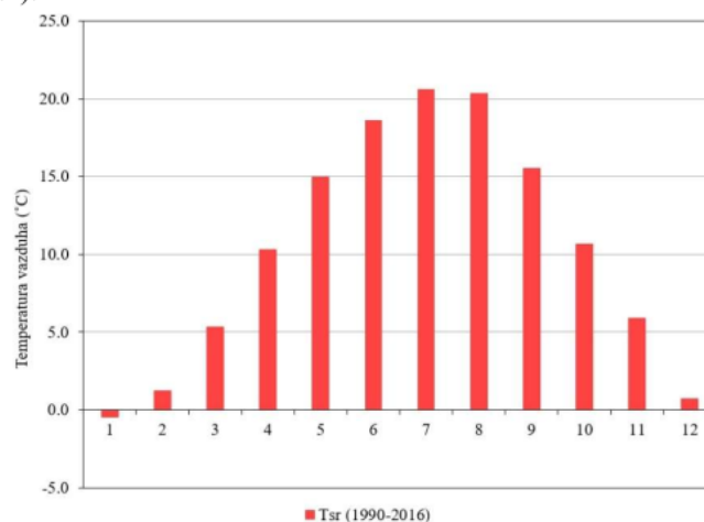
Slika II.4. Unutargodišnja raspodela temperature vazduha za period 1990-2016
