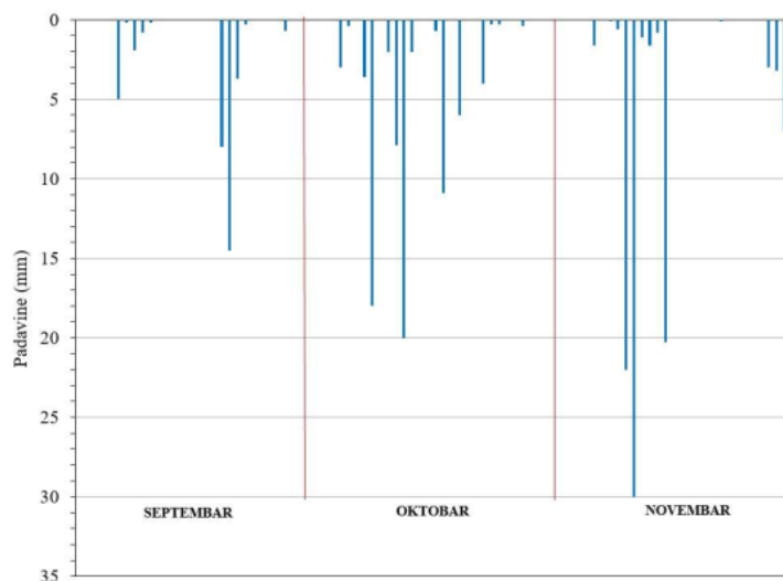
Slika IV.6. Dnevne sume padavina za period septembar-novembar 2016. godine
