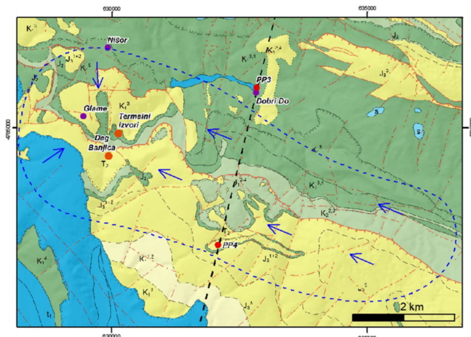
Slika II.9 12. Pretpostavljeno slivno područje termalnog izvora Dag Banjica
