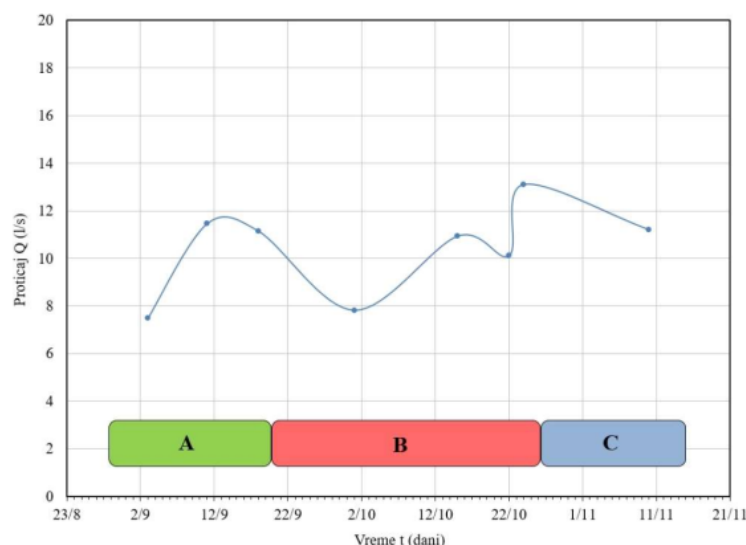
Slika IV.14. Izdašnost termalnog izvora Dag Banjice
