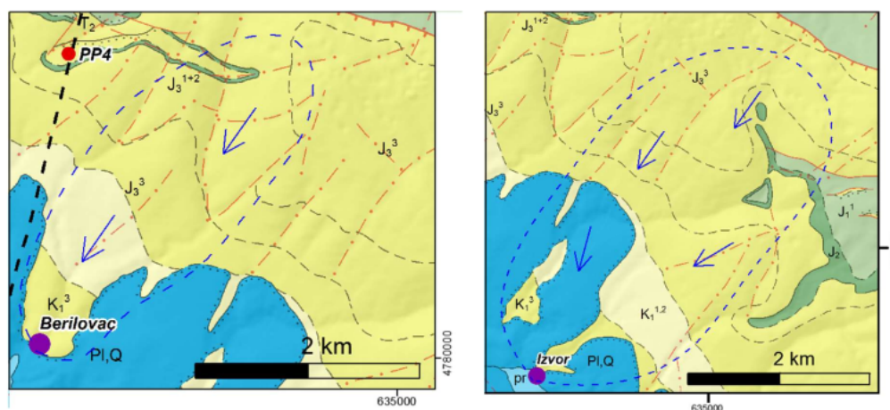
Slika II.8. Pretpostavljeno slivno područje karstnih vrela Berilovac i Izvor
