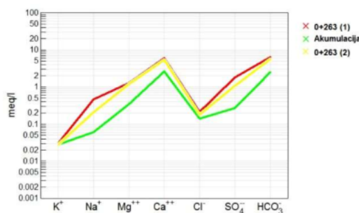
Slika IV.74. Schoeller-ov dijagram voda iz akumulacionog jezera i sa stacionaže 0+263 m. Legenda: 1 - 18/09/2016. ustaljen režim rada tunela; 2 – 22/10/2016. tunel nije u funkciji mesec dana [40]
