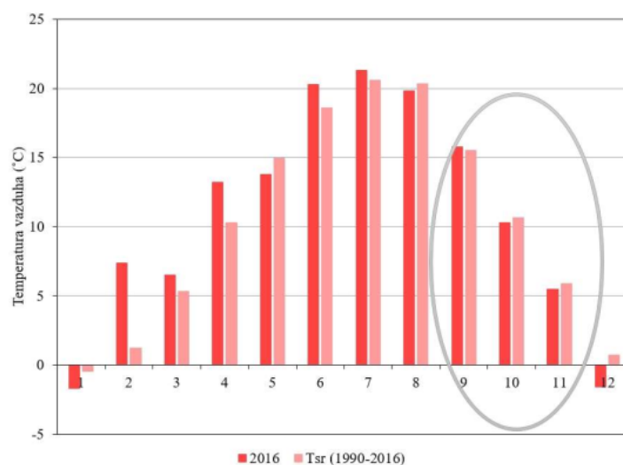
Slika IV.3. Uporedni dijagram unutar godišnje raspodele temperatura vazduha tokom 2016. godine i višegodišnjeg perioda (1990-2016) – met. st. Dimitrovgrad. Krug označava osmatrački period.
