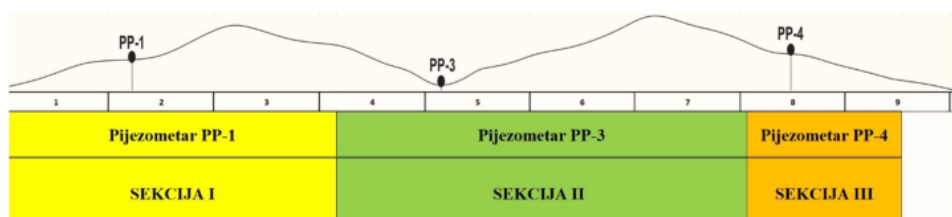
Slika IV.61. Skica profila tunela sa prikazanim sekcijama i odgovarajućim piježometrima
