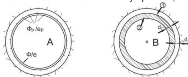
Slika I.13. Armirano betonske obloge: A- Jednoslojna obloga i B-dvoslojna obloga 1-beton, 2-armirani beton ili armirani prskani beton
