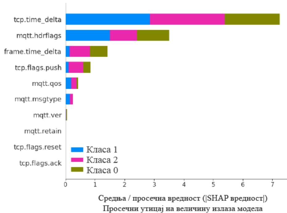
Слика 47 SHAP анализа утицаја карактеристика у бинарној и вишекласној класификацији помоћу XGBoost-a [13]
