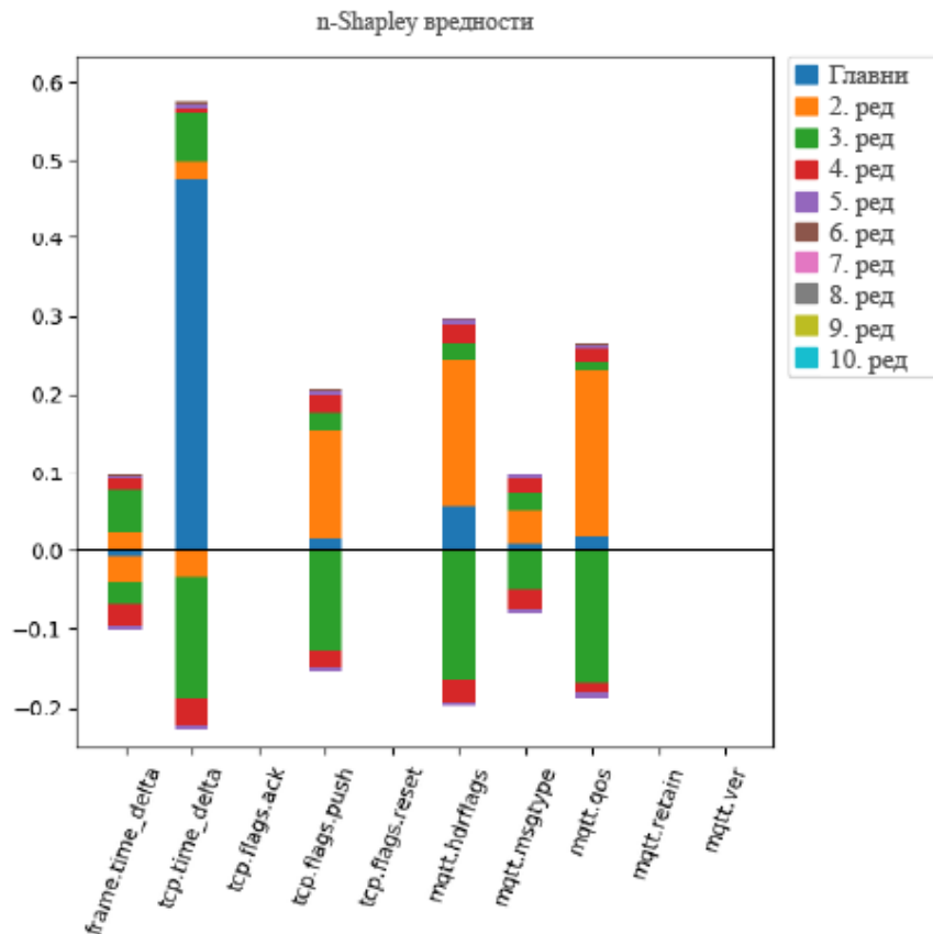
Слика 48 nSHAP анализа 10. реда за бинарну и вишекласну класификацију са приказом интеракција карактеристика [13]
