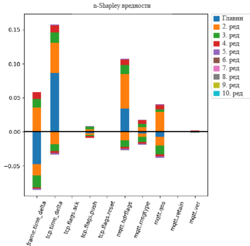
Слика 49 nSHAP анализа 10. реда за бинарну и вишекласну класификацију са приказом интеракција карактеристика [13]
