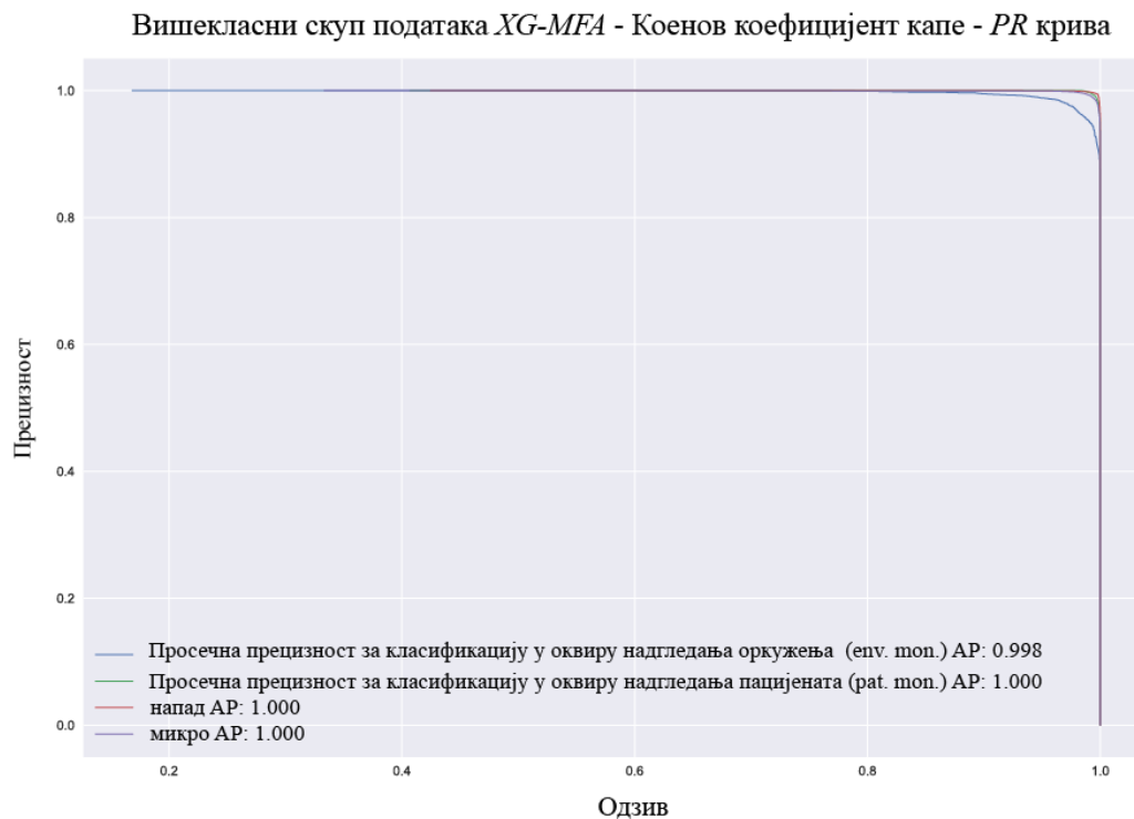
Слика 40 Површина испод криве Precision-Recall , која приказује однос прецизности и одзива за XG-MFA алгоритам, важан за процену модела са неуравнотеженим класама [13]
