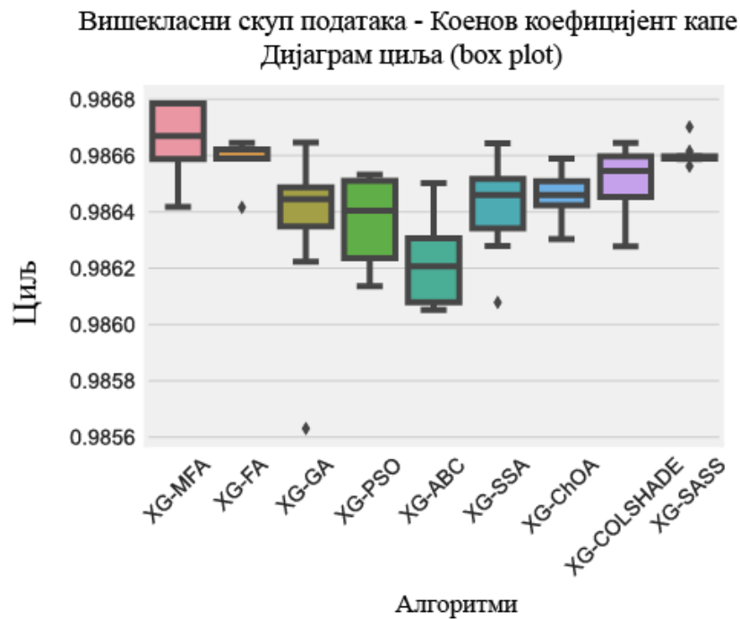
Слика 38 Дијаграм циља за вредности вишекласног скупа података различитих алгоритама, који помоћу Коеновог коефицијента капе [13]
