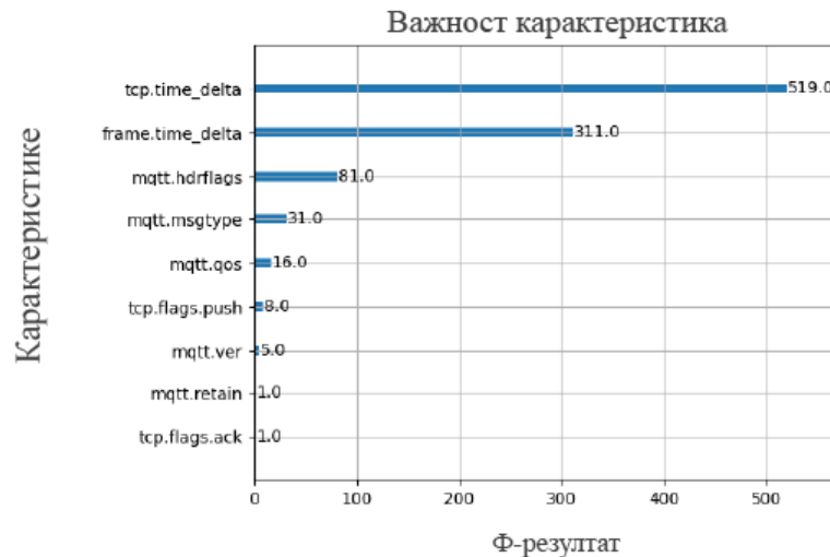
Слика 45 Интерпретација важности карактеристика у бинарној и вишекласној класификацији помоћу XGBoost-a [13]
