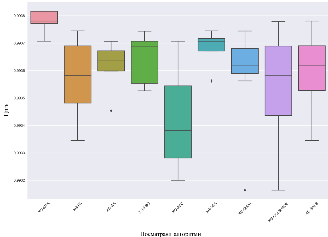
Слика 26 Графичка илустрација дијаграма циља за максималне вредности Коеновог коефицијента капе [13]
