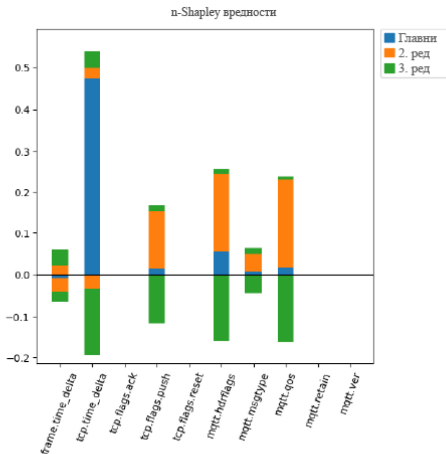
Слика 50 Шапли–Тејлор анализа карактеристика бинарна класификација [13]
