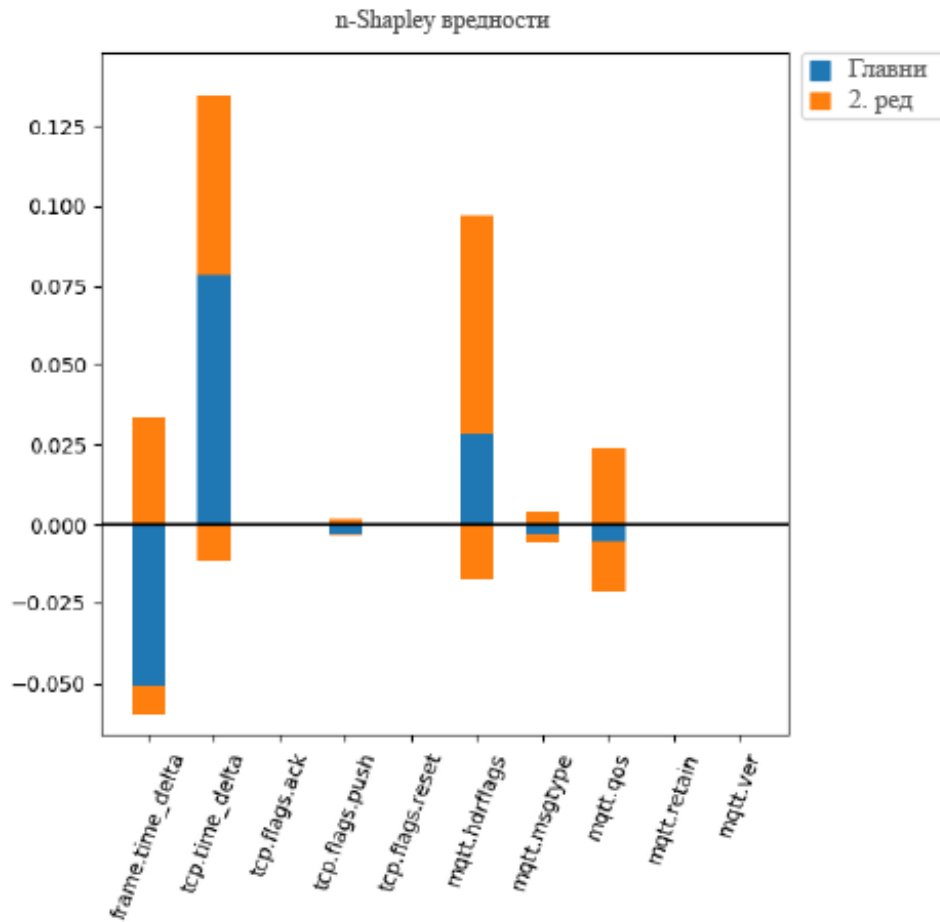
Слика 53 nSHAP анализа другог реда за вишекласну класификацију - вишекласна nSHAP анализа [13]
