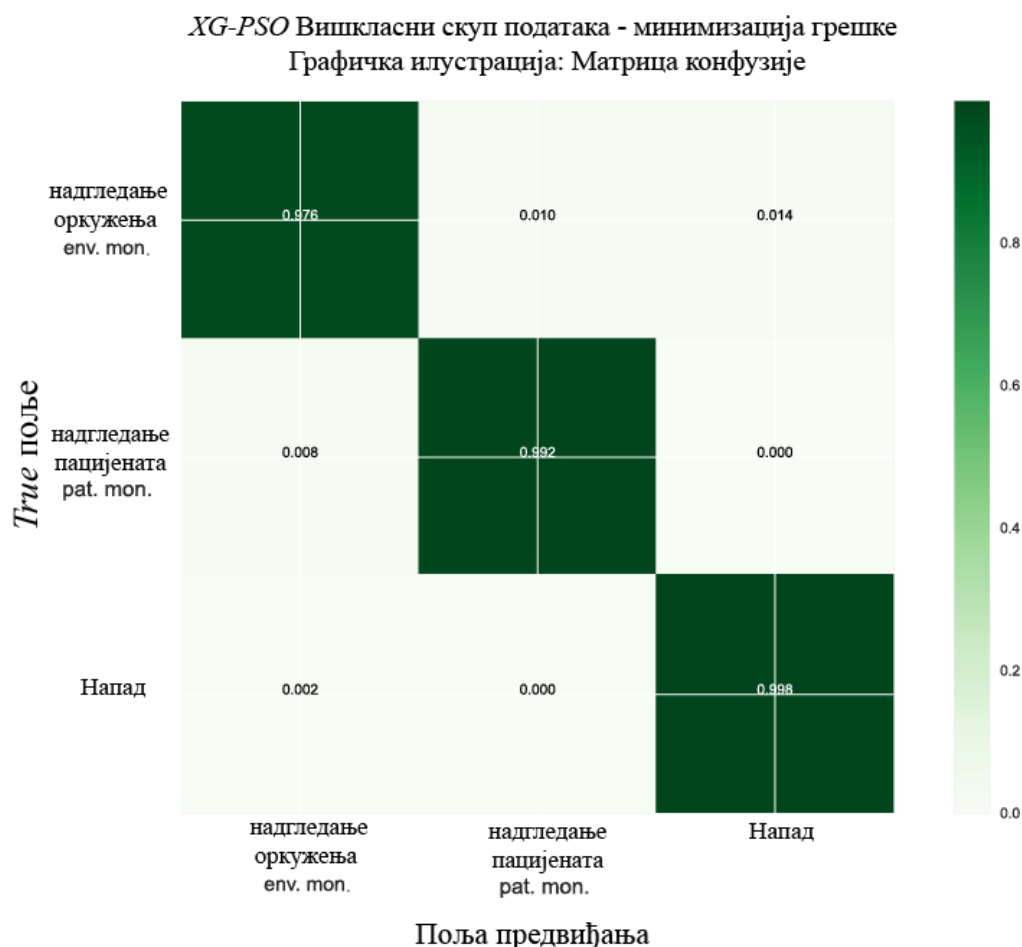
Слика 37 Матрица конфузије за XG-MFA алгоритам, која приказује тачна и нетачна предвиђања за различите класе, помажући тиме идентификације области где модел најчешће греши [13]
