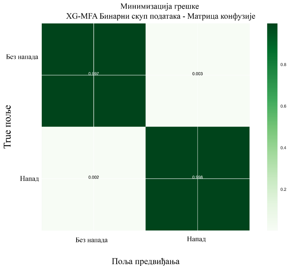
Слика 25 Графичка илустрација бинарног скупа података XG-MFA алгоритма и матрица конфузије [13]
