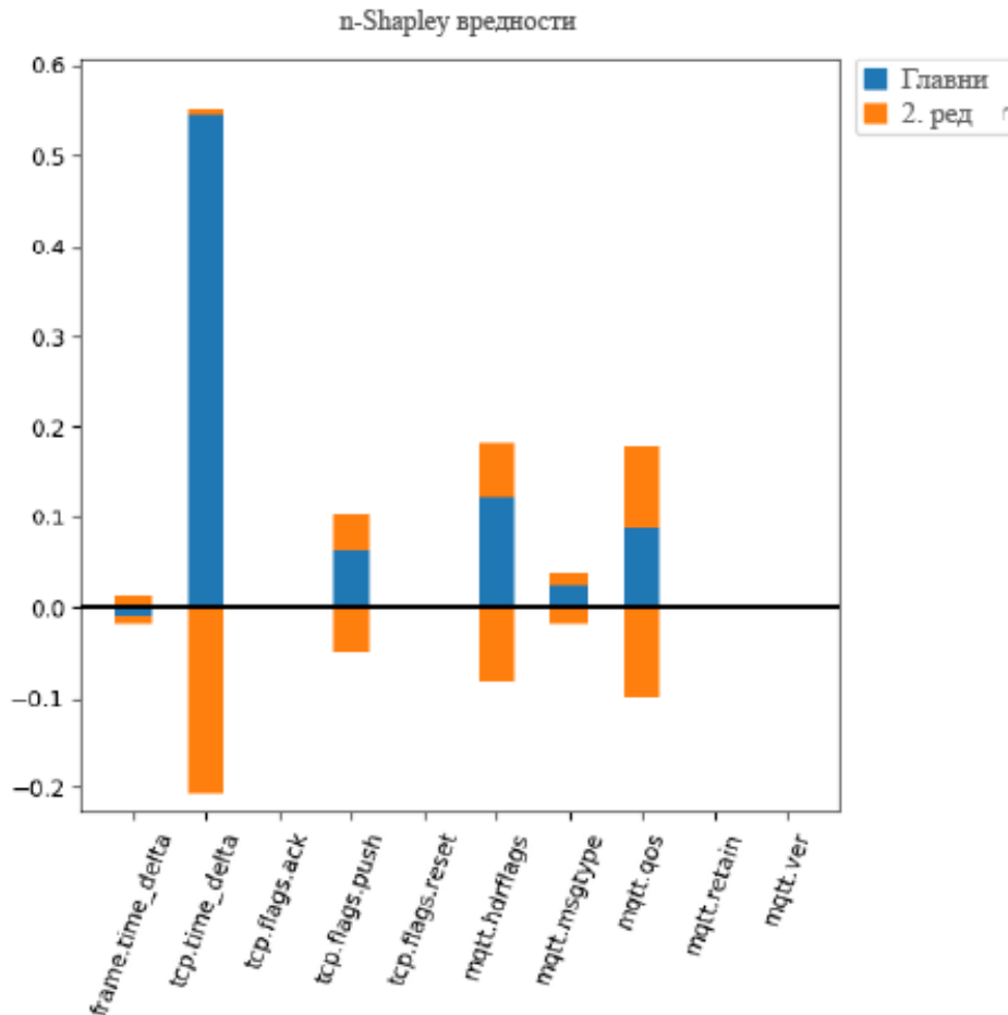
Слика 52 nSHAP анализа другог реда за бинарну и вишекласну класификацију - Бинарна nSHAP анализа [13]
