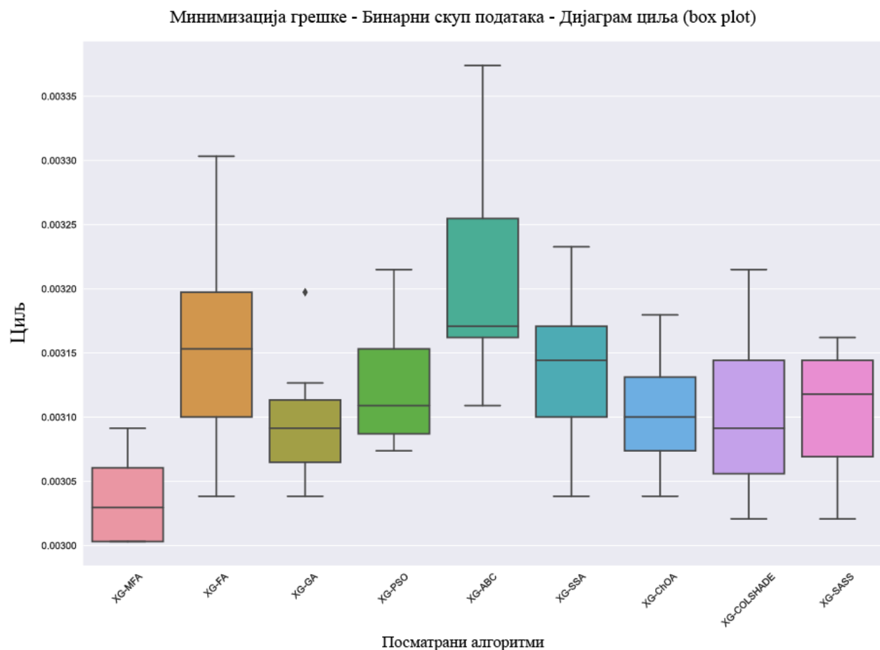
Слика 20 Графикон дијаграма циља за бинарни скуп података [13]
