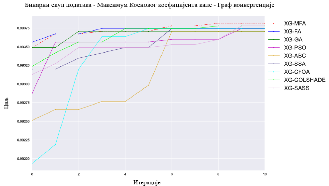
Слика 27 Графикон конвергенције, где се приказују максималне вредности Коеновог коефицијента капе [13]
