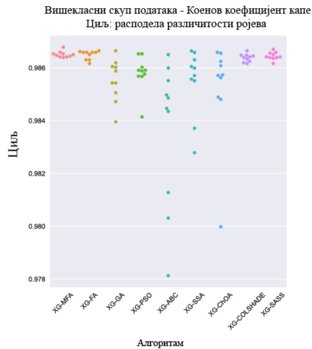
Слика 42 Дијаграм вишекласног скупа података где се помоћу Коеновог коефицијента капе визуализује густину резултата и распон перформанси различитих алгоритама [13]
