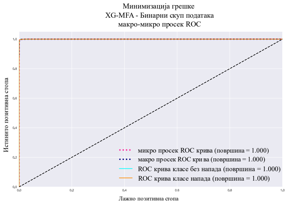
Слика 23 Графикон макро и микро просека ROC криве за бинарни скуп података [13]
