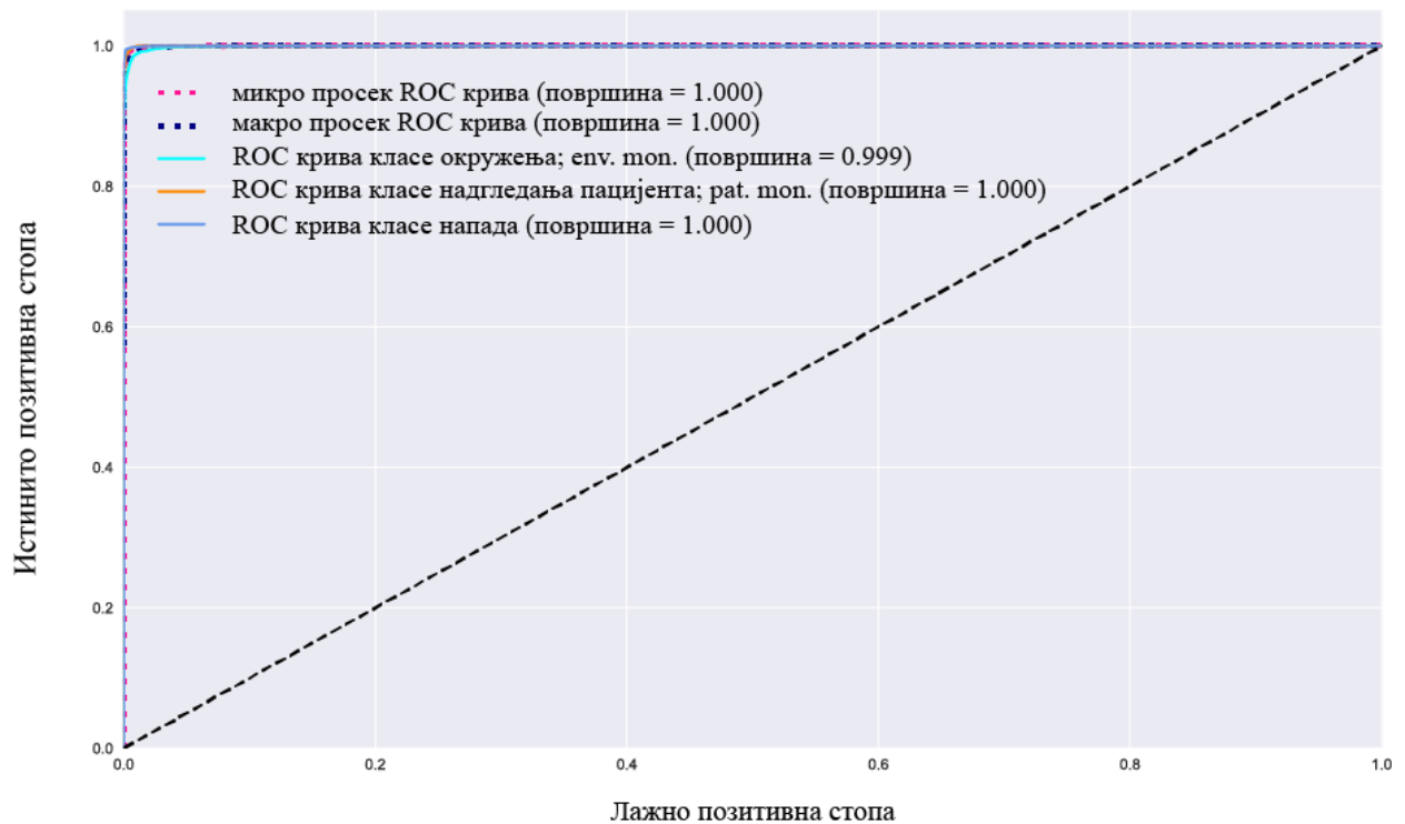
Слика 35 Површина испод криве ROC (енгл. Receiver Operating Characteristic ) са макро и микро просецима за XG-MFA алгоритам, омогућавајући процену перформанси у различитим праговима класификације [13]
