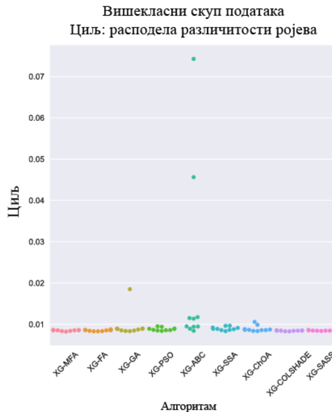
Слика 36 Дијаграм различитости ројева за објективне вредности, који визуализује густину и расподелу резултата међу различитим алгоритмима [13]
