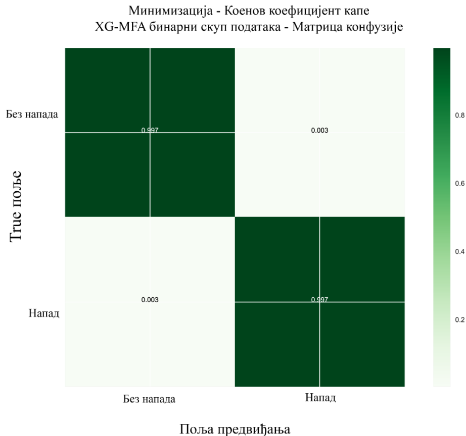
Слика 31 Графичка илустрација матрице конфузије за максималне вредности бинарног скупа података помоћу Коеновог коефицијента капе [13]
