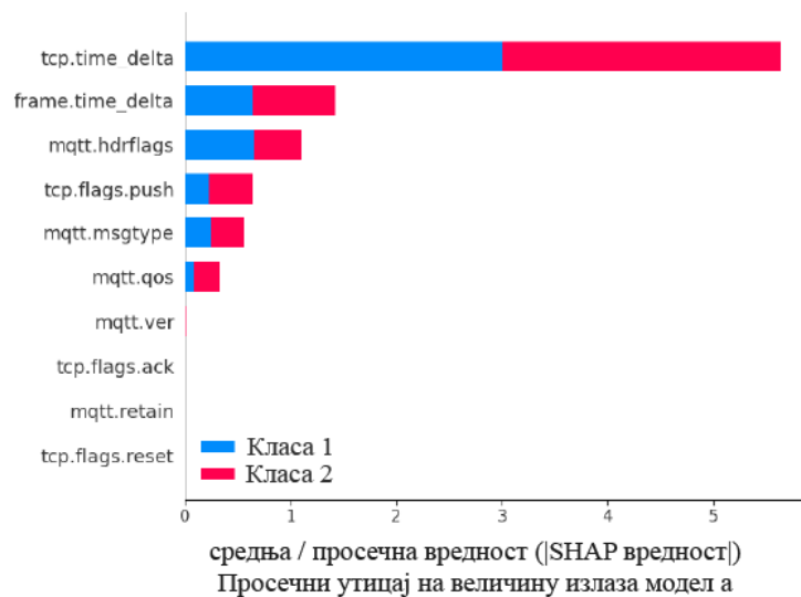
Слика 46 SHAP анализа утицаја карактеристика у бинарној и вишекласној класификацији помоћу XGBoost-a [13]
