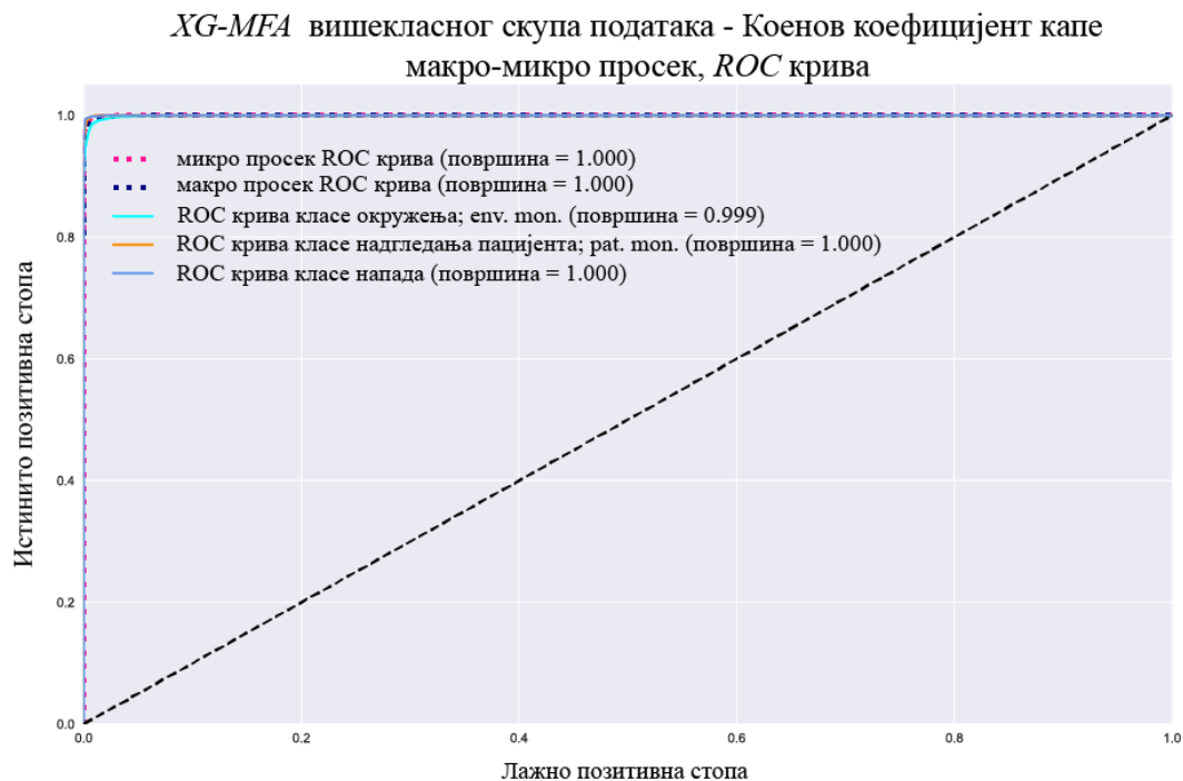
Слика 41 Површина испод криве (енгл. Receiver Operating Characteristic - ROC ), приказујући како алгоритам балансира између истинито позитивних и лажних позитивних предвиђања при различитим праговима [13]
