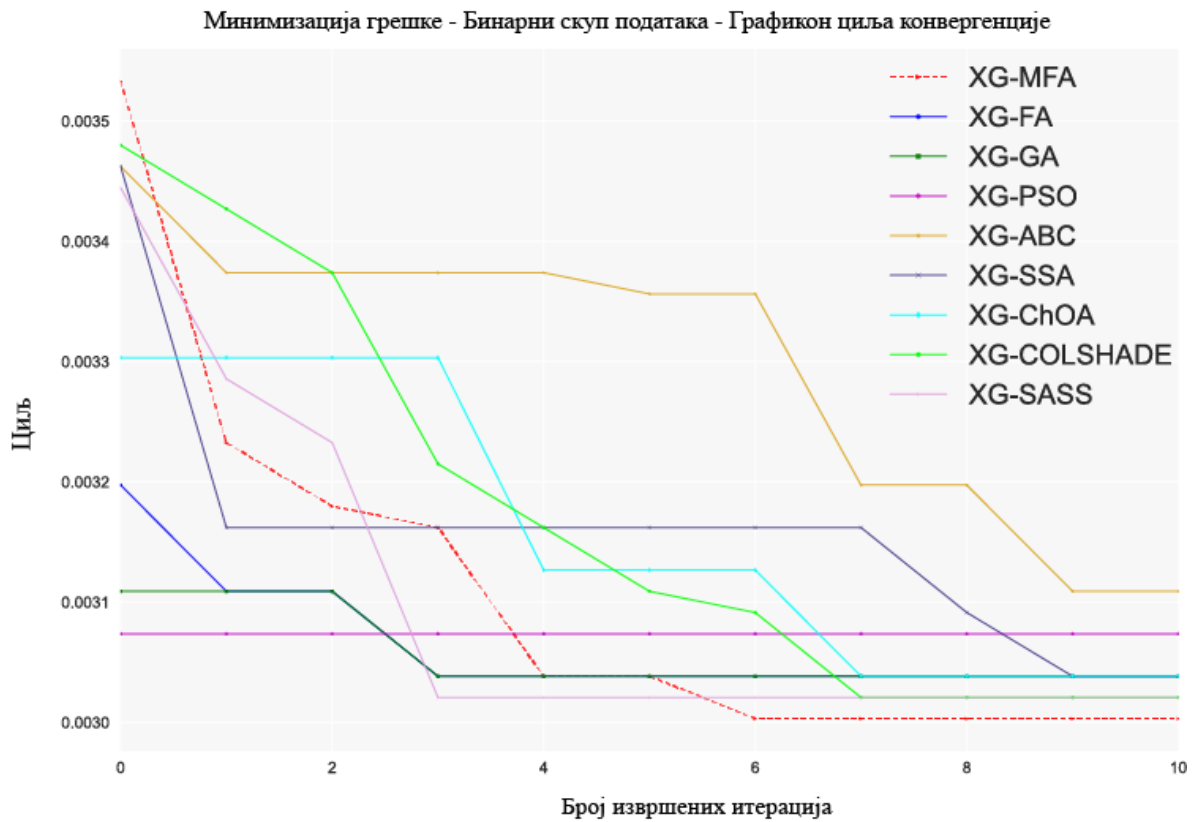
Слика 21 Графикон циља конвергенције за бинарни скуп података [13]
