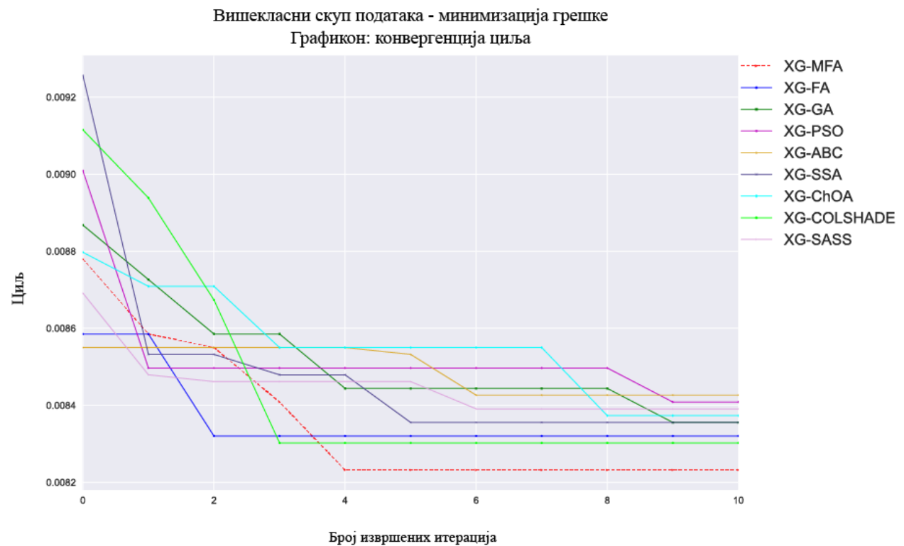
Слика 33 Графикон конвергенције објективне функције током итерација за различите алгоритме, показујући како се перформансе мењају током времена [13]
