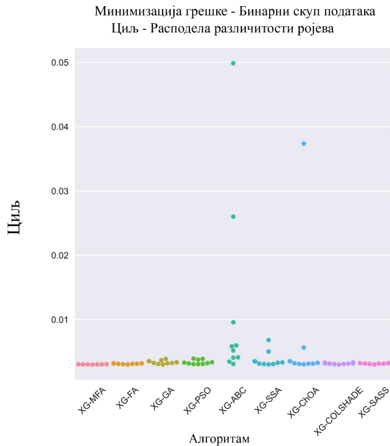
Слика 24 Графичка илустрација расподеле различитости ројева у бинарном скупу података [13]
