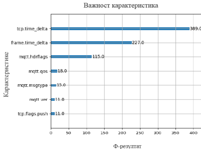
Слика 44 Интерпретација важности карактеристика у бинарној и вишекласној класификацији помоћу XGBoost-a [13]
