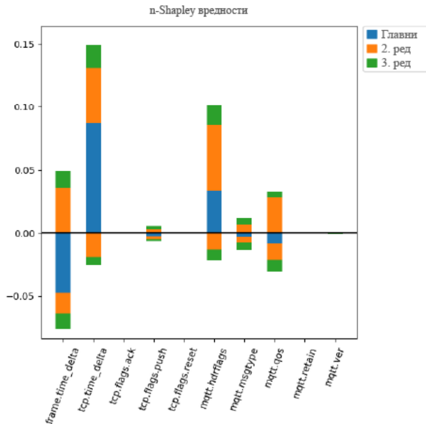
Слика 51 Шапли–Тејлор анализа карактеристика вишекласна класификација [13]
