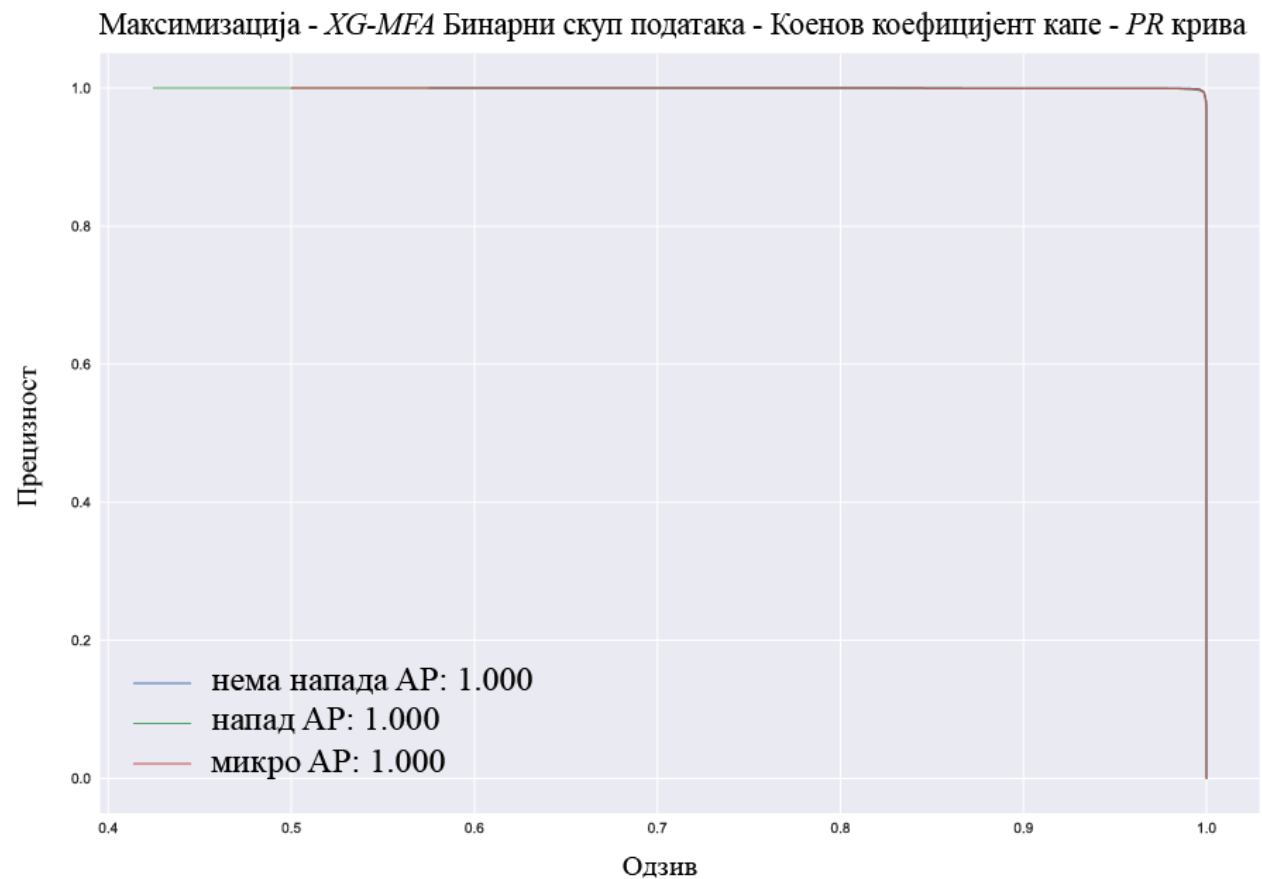
Слика 28 Графичка илустрација PR криве над бинарним скупом података, помоћу максималних вредности Коеновог коефицијента капе [13]
