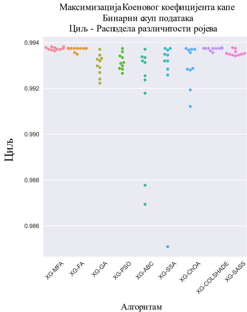
Слика 30 Графичка илустрација расподеле различитости ројева, помоћу максималних вредности Коеновог коефицијента капе [13]
