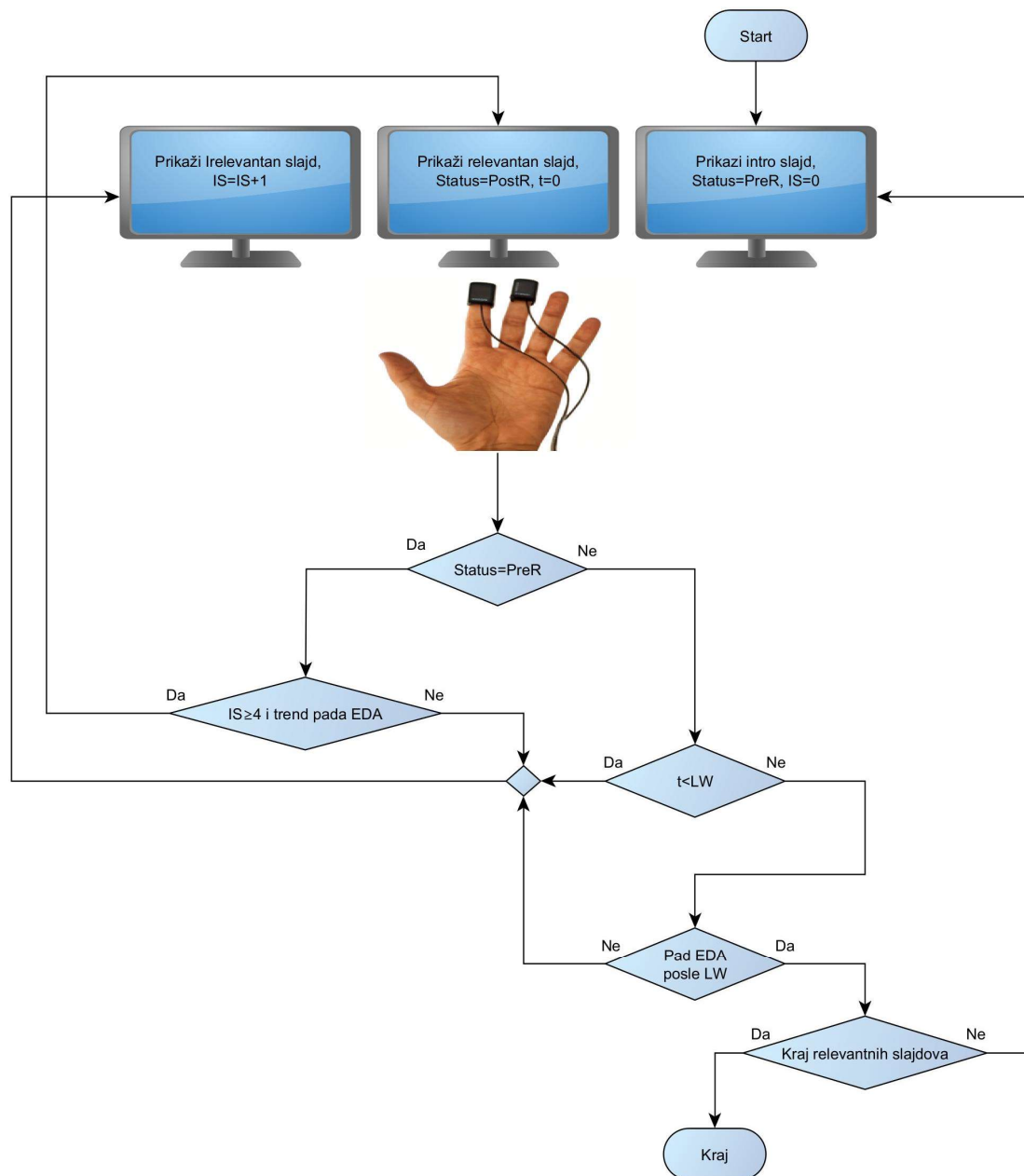
Slika 25. Algoritam za interaktivnu selekciju slajdova
