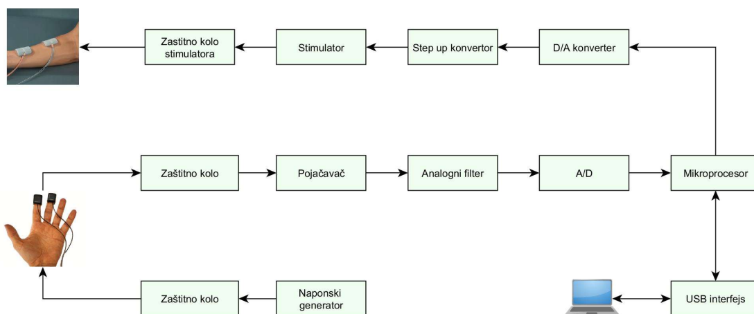
Slika 7. EDA uređaj
