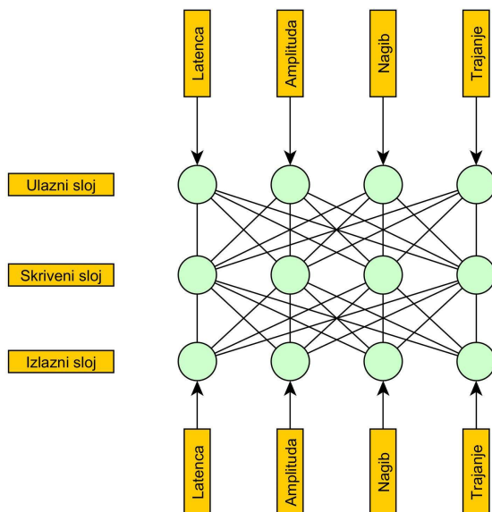
Slika 10. Autoenkoder za korekciju podataka
