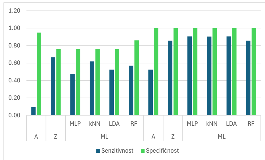
Slika 34. Senzitivnost i spcifičnost sCIT-a i CtTC-a
