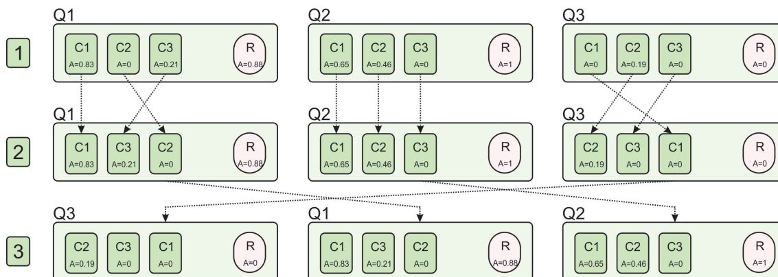
Slika 32. CIT-dataset sorting algoritam za klasifikaciju učesnika
