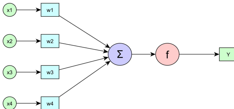
Slika 13. Princip funkcionisanja perceptrona
