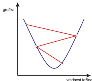
Slika 18. Problem sa padom gradijenta zbog velikog koeficijenta učenja
