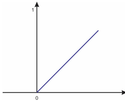
Slika 16. ReLU funkcija
