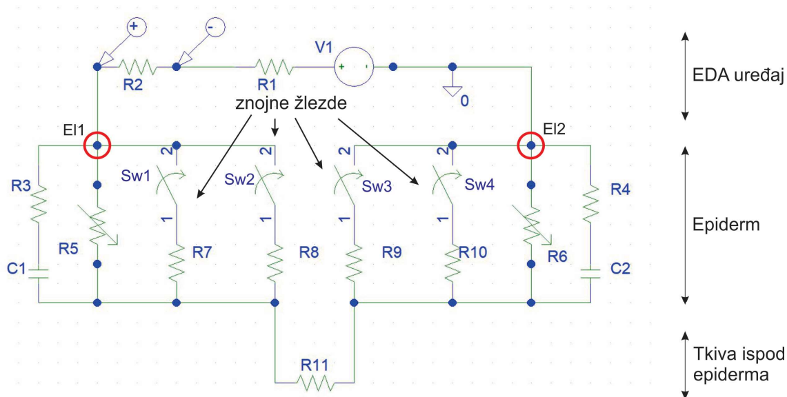
Slika 4. Električni model kože
