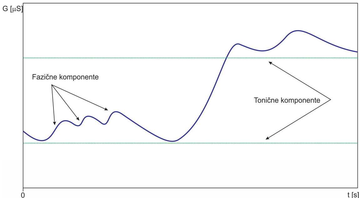
Slika 2. Tonične i fazične komponente EDA
