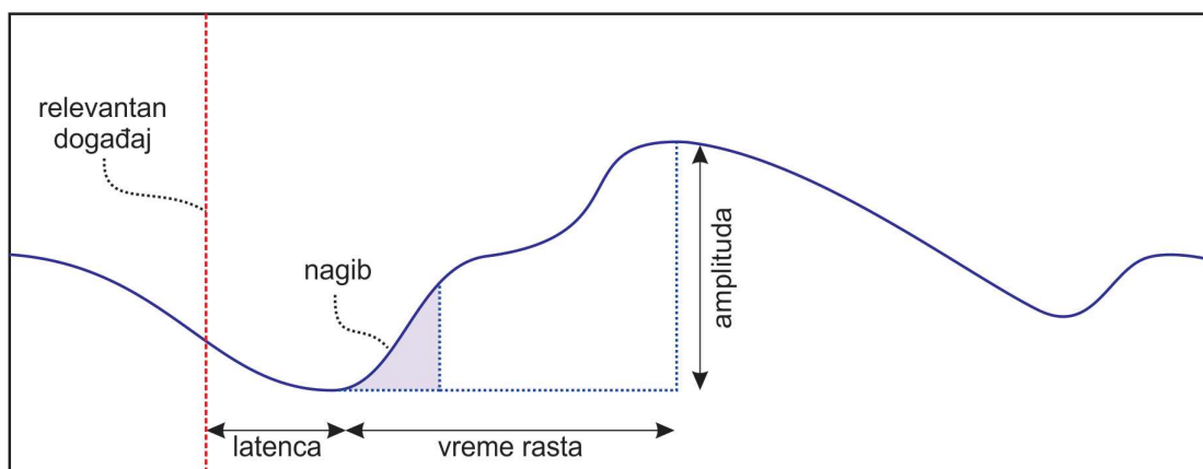
Slika 3. Parametri elektrodermalna reakcije
