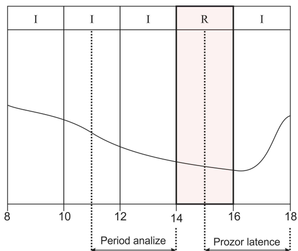
Slika 28. Tipični početak SCR-a kod iCIT-a
