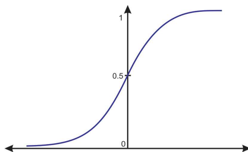
Slika 14. Sigmoidna funkcija
