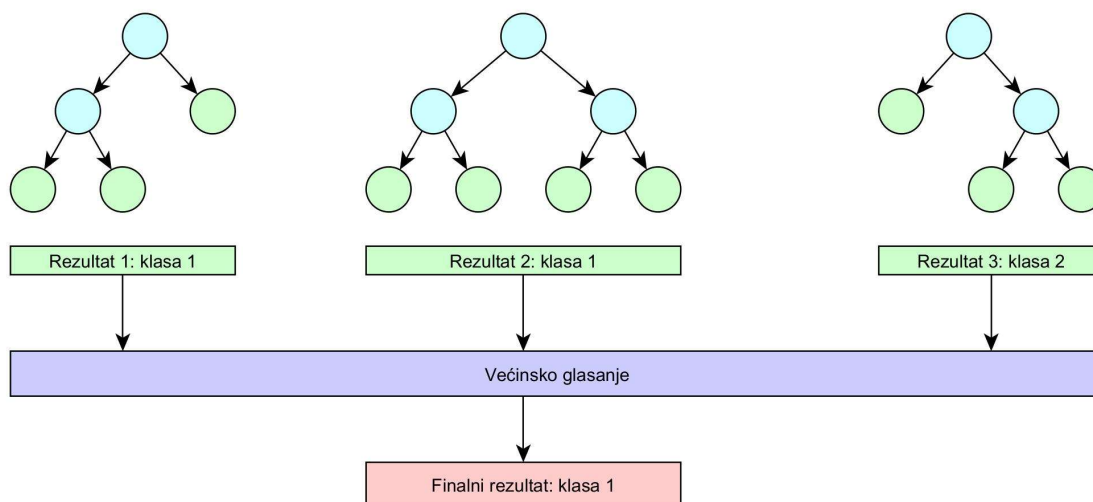
Slika 23. Slučajna šuma
