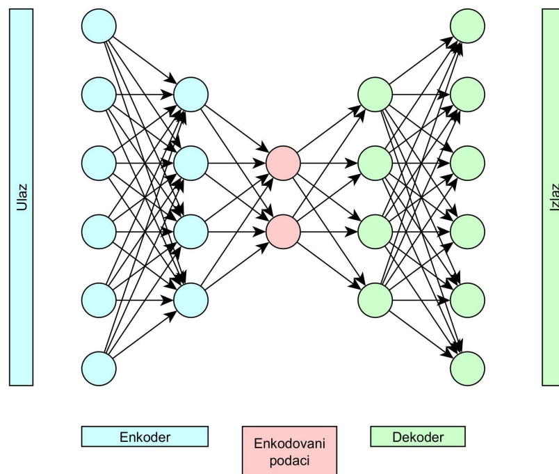
Slika 11. Autoenkoder za smanjenje dimenzionalnosti
