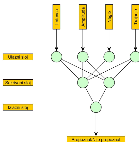
Slika 12. MLP Klasifikacija slajda na osnovu EDR parametara
