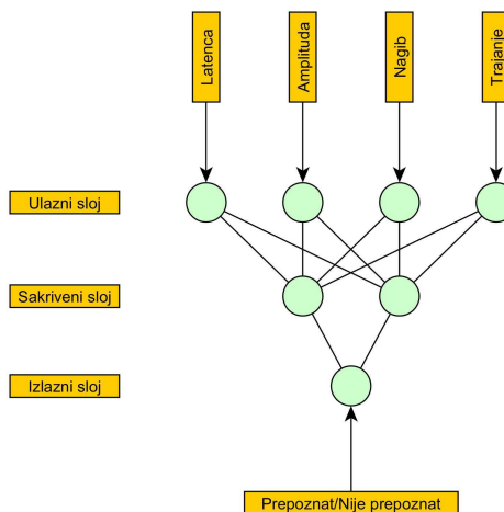
Slika 9. Supervizovano učenje MLP-a
