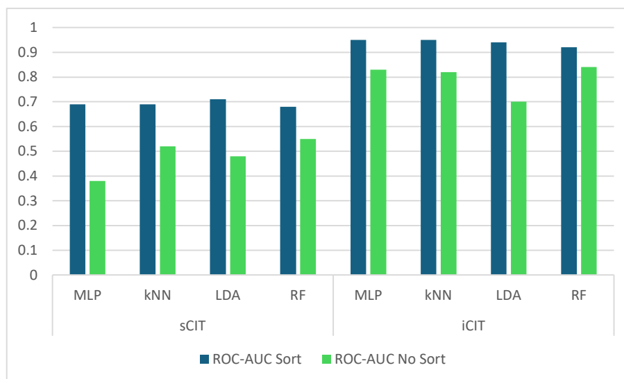
Slika 35. ROC-AUC i CIT-dataset sorting algoritam
