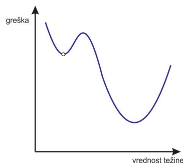
Slika 19. Problemi pada gradijenta sa lokalnim minimumima
