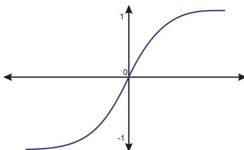
Slika 15. Tangens hiperbolički
