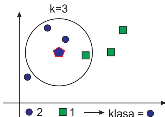
Slika 20. kNN klasifikacija
