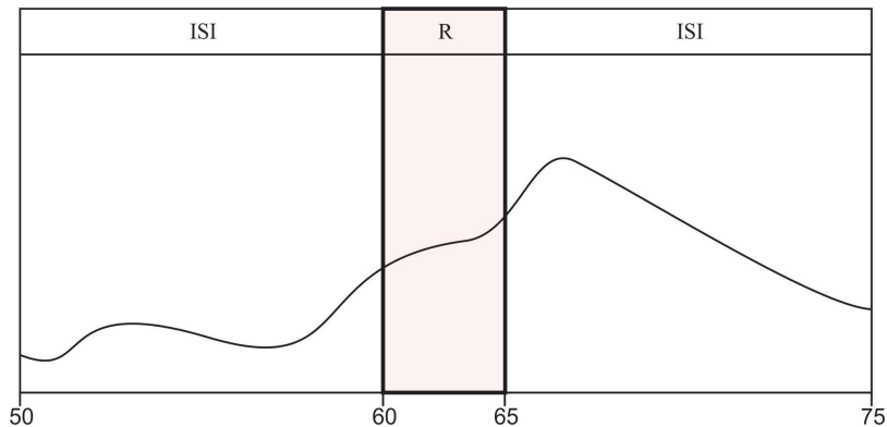
Slika 27. Prikaz relevantnog slajda tokom rastuće ivice SCR-a
