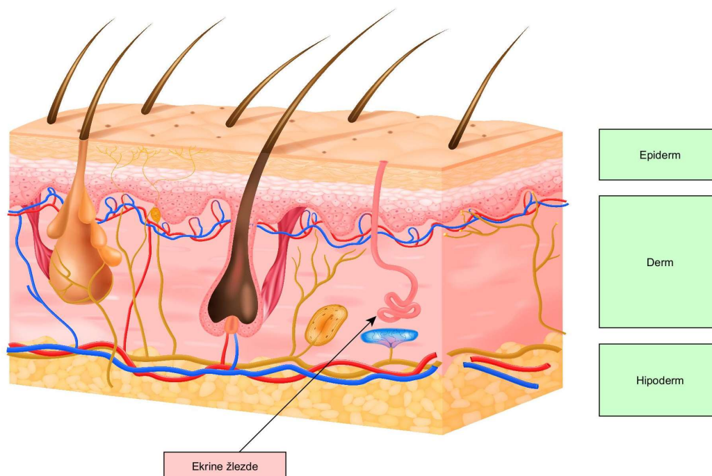
Slika 1. Anatomija kože [84]
