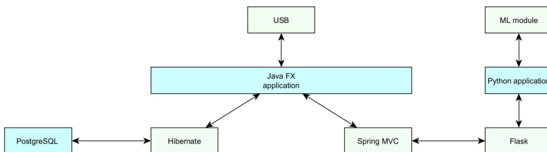
Slika 8. PC softver za kontrolu iCIT uređaja
