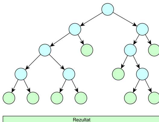
Slika 22. Jedno drvo odlučivanja
