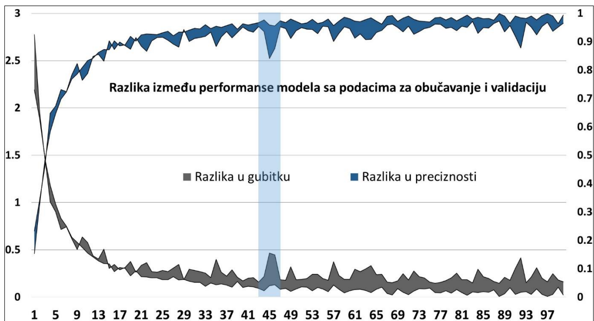
Slika 53. Razlike u funkcijama gubitka i preciznosti modela zasnovanog na dvodimenzionalnom skupu podataka
