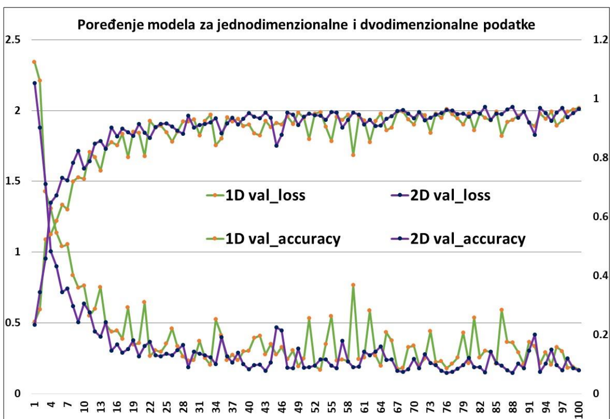
Slika 52. Poređenje tačnosti i gubitaka modela za 1-D i 2-D podatke
