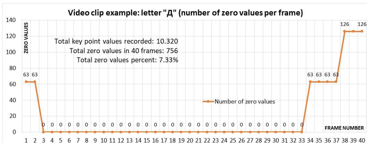
Slika 16. Broj ključnih tačaka koji nisu prepoznati (Radaković M., et al., 2024)
