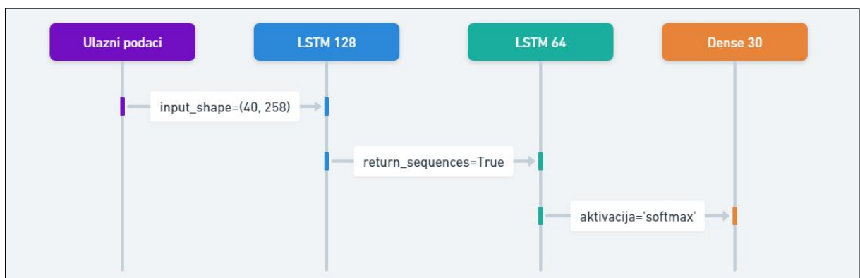
Slika 35. Grafički prikaz modela neuronske mreže
