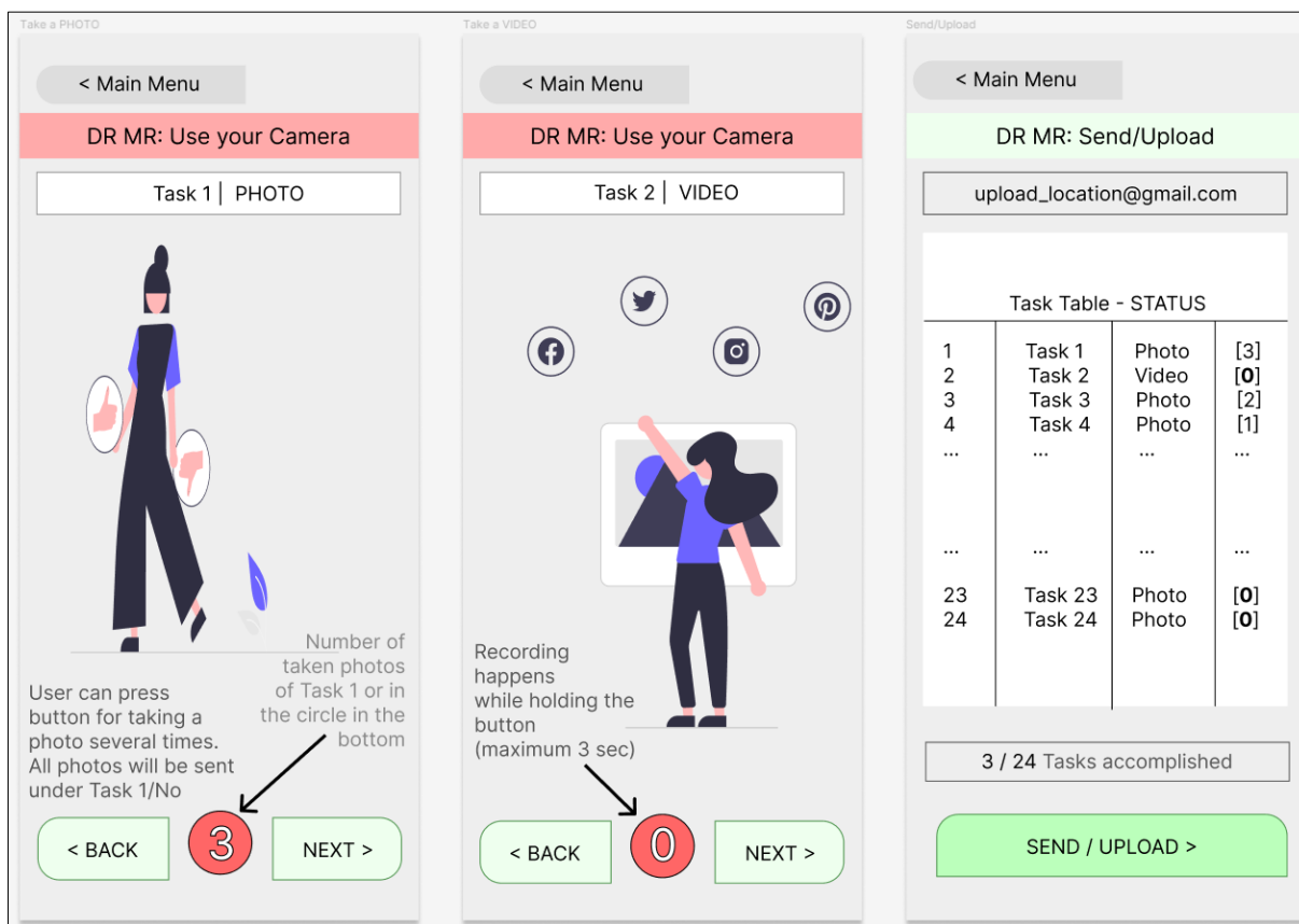
Slika 6. Dizajn funkcionalnog dela Android aplikacije DR MR
