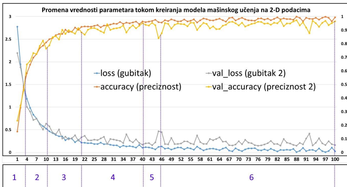
Slika 48. Promena vrednosti parametara tokom kreiranja 2-D modela mašinskog učenja
