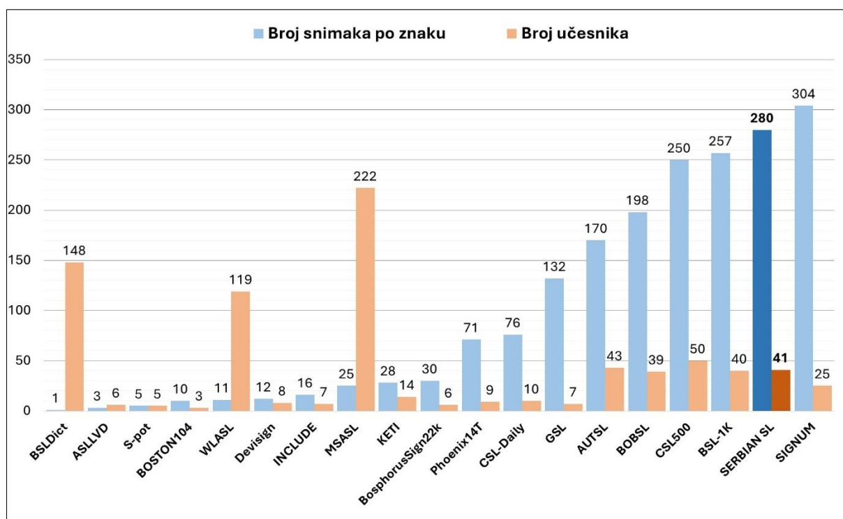
Slika 27. Poređenje kreirane baze podataka SZJ sa drugim bazama
