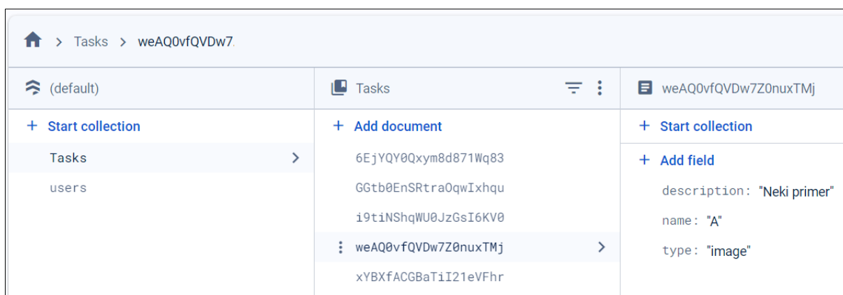
Slika 5. Firebase pregled postavljenih zadataka
