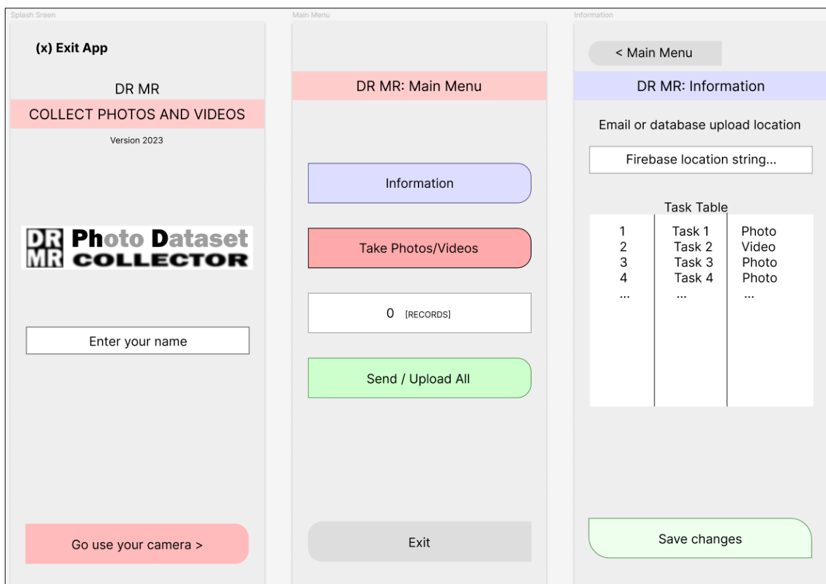
Slika 4. Dizajn Android mobilne aplikacije DR MR
