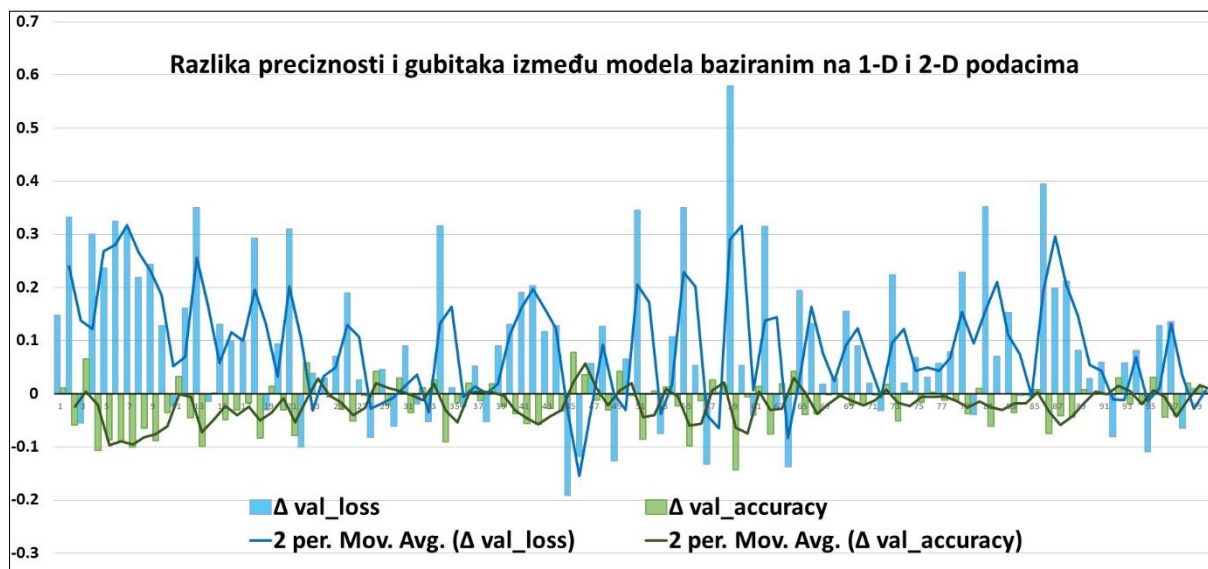
Slika 51. Poređenje preciznosti i grešaka između modela zasnovanih na jednodimenzionalnim i dvodimenzionalnim podacima
