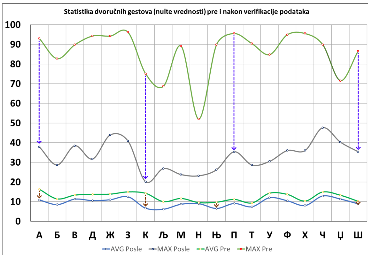
Slika 24. Pre i nakon čišćenja za dvoručne gestove
