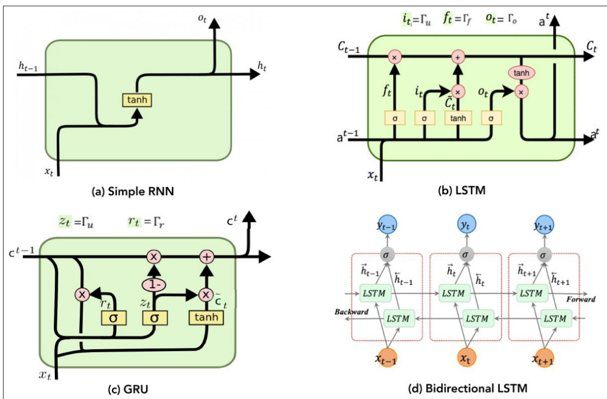
Slika 36. Struktura modela: Simple RNN, LSTM, GRU, Bi-LSTM (Apaydin et al., 2020)
