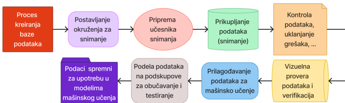
Slika 12. Algoritam kreiranja baze podataka (Radaković M., et al., 2024)
