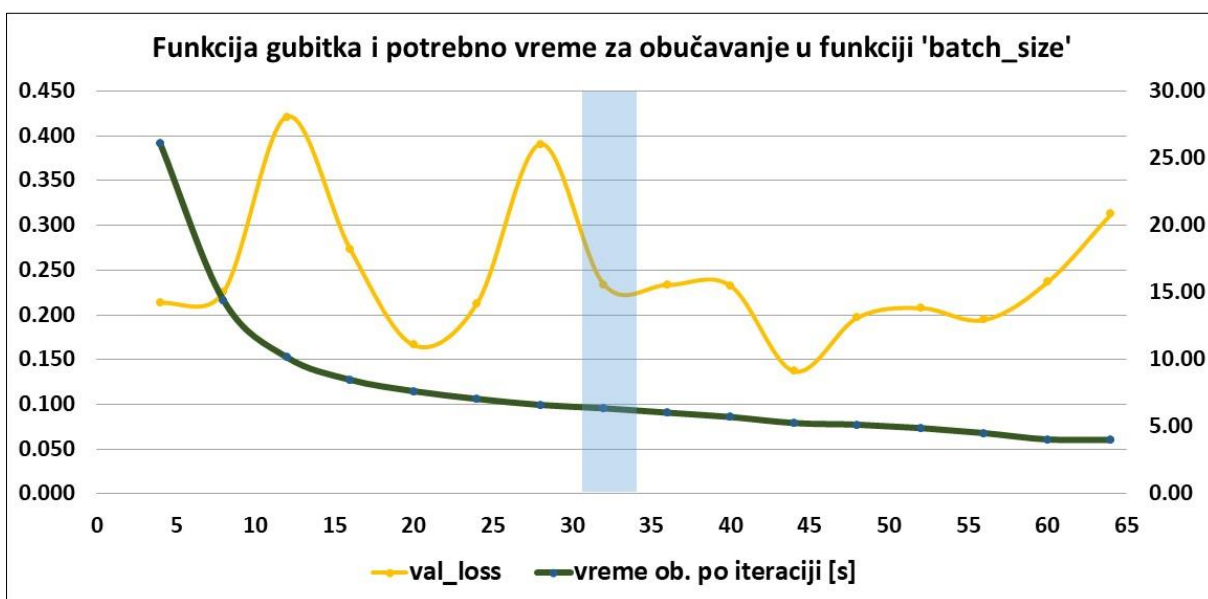
Slika 55. Gubitak modela u funkciji batch_size parametra
