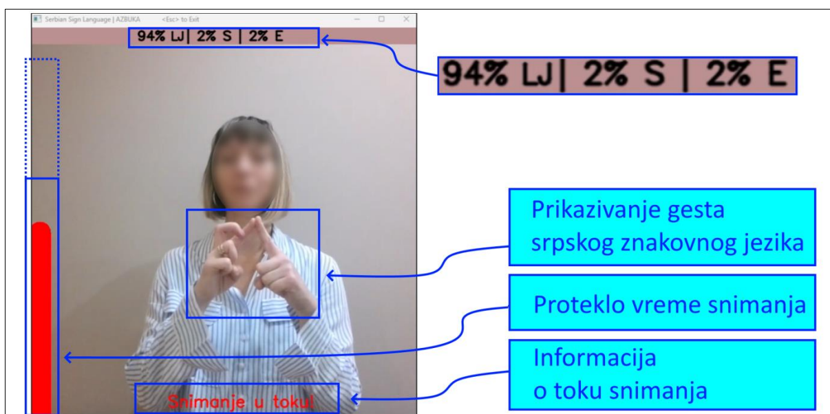
Slika 58. Korisnički interfejs programa za prepoznavanje gestova srpskog znakovnog jezika
