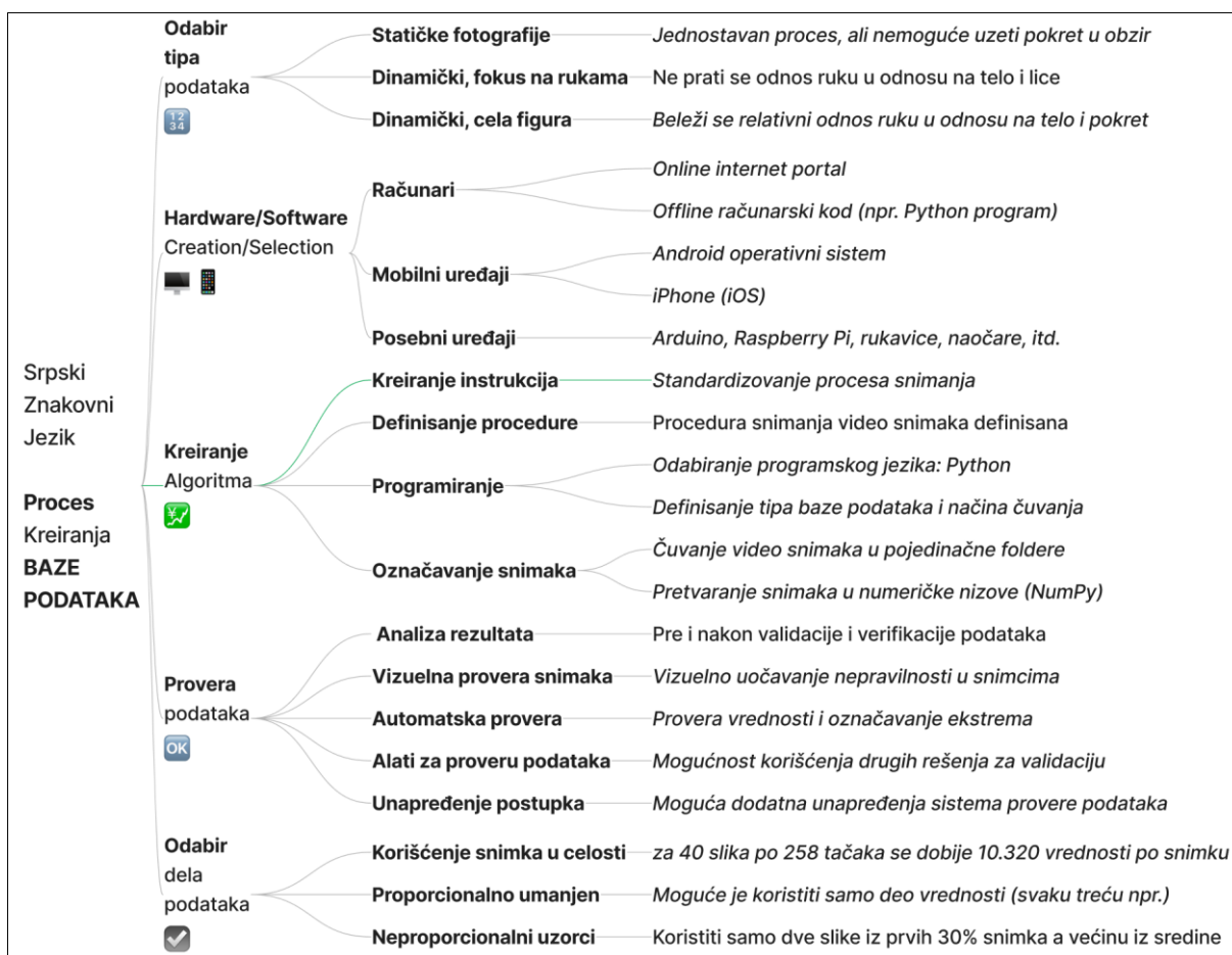
Slika 2. Koncept kreiranja baze podataka srpskog znakovnog jezika
