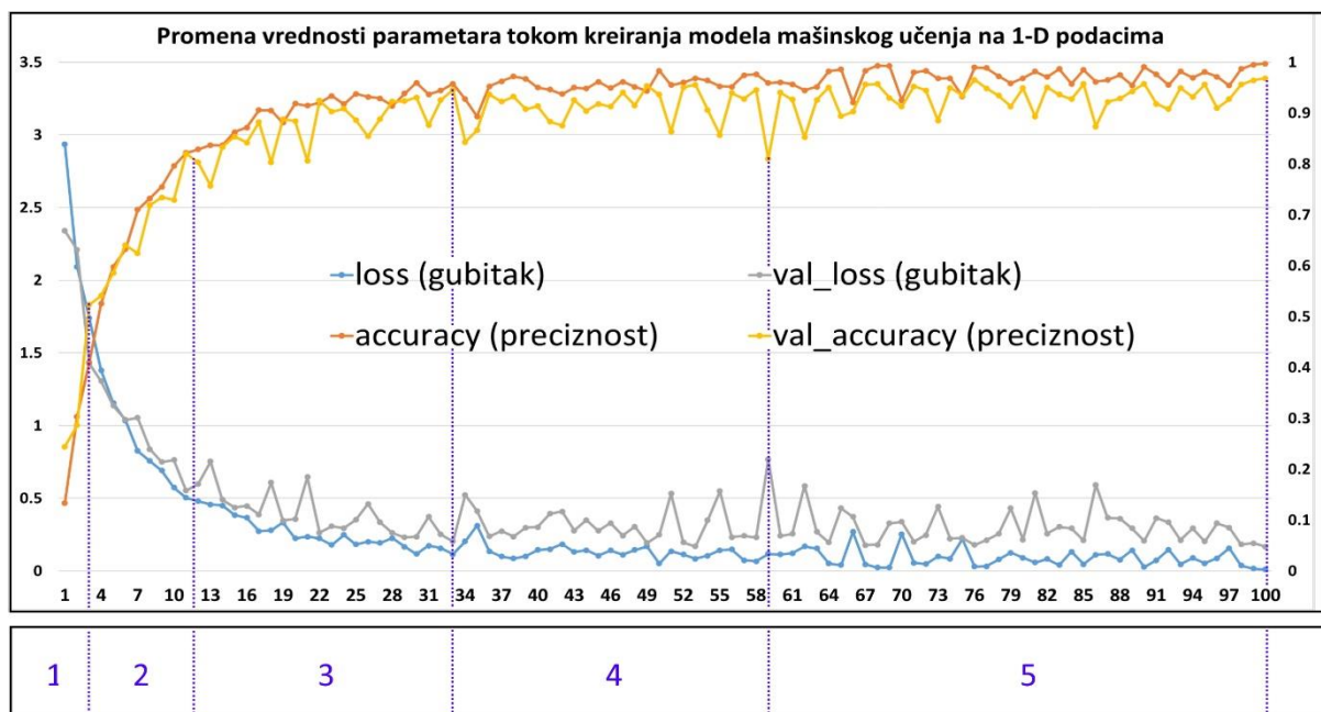
Slika 46. Promena vrednosti parametara tokom kreiranja 1-D modela mašinskog učenja
