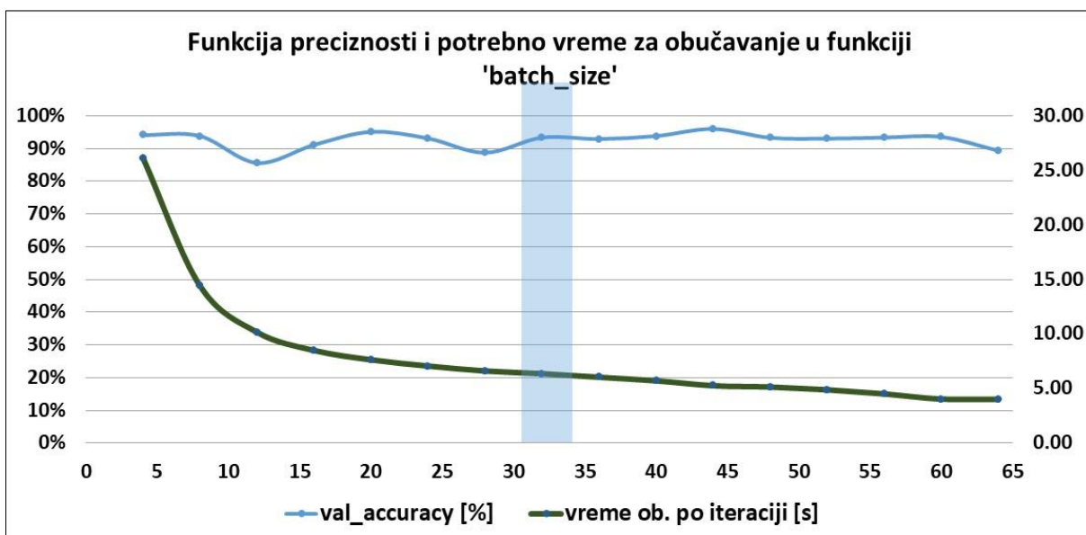
Slika 54. Preciznost modela u funkciji batch_size parametra
