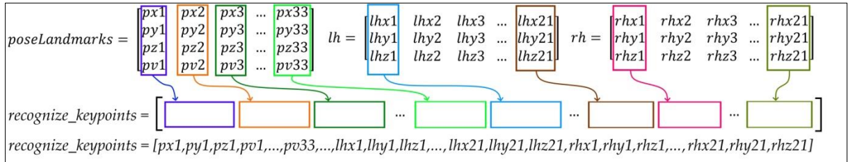
Slika 17. Prikaz transformacije podataka iz matrica u jednodimenzionalni niz
