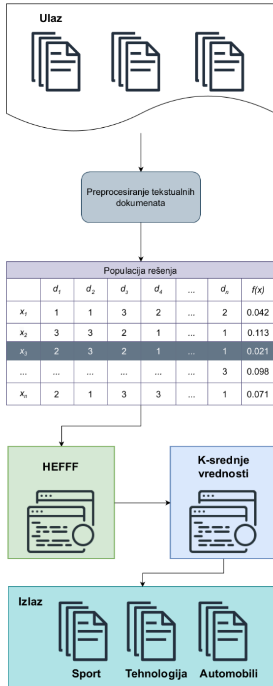
Slika 20: Dijagram toka klasterovanja tekstualnih dokumenata
