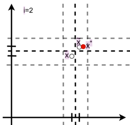
Slika 10: Primer OBL-a u dvodimenzijonalnom prostoru ( i = 2 )
