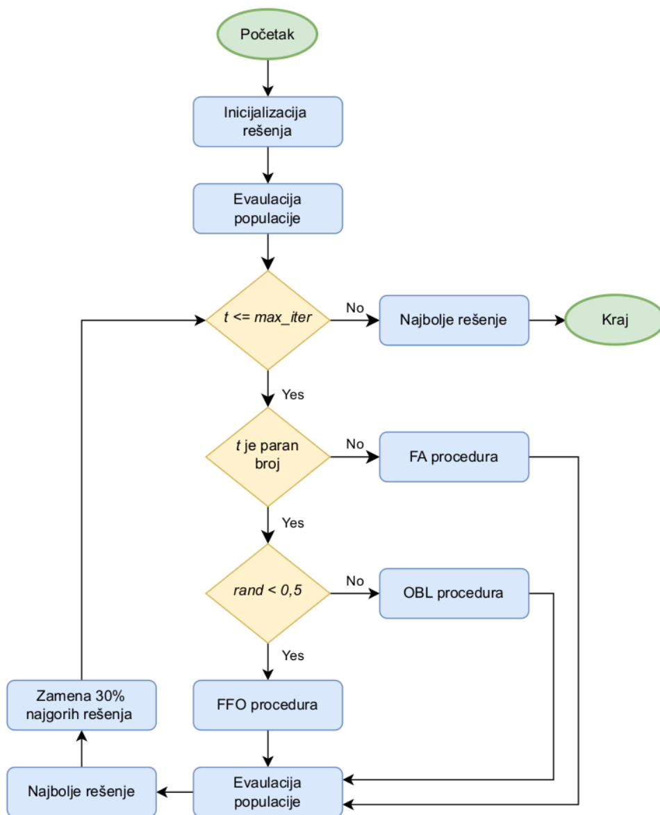
Slika 17: Dijagram toka predloženog HEFFF algoritma
