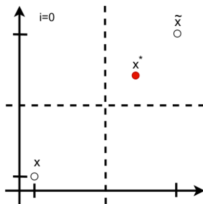
Slika 8: Primer OBL-a u dvodimenzijonalnom prostoru ( i = 0 )
