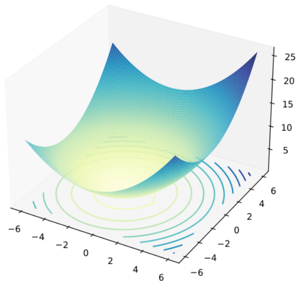
Slika 31: 3D grafikon dvodimenzionalne Happy Cat funkcije
