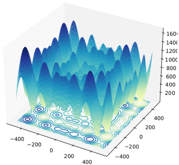
Slika 27: 3D grafikon dvodimenzionalne Schwefel funkcije
