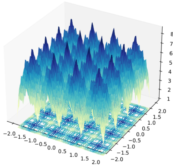
Slika 25: 3D grafikon dvodimenzionalne Weierstrass funkcije
