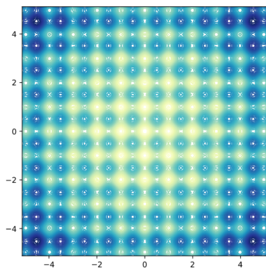
Slika 22: Kontur grafikon dvodimenzionalne Rastrigin funkcije
