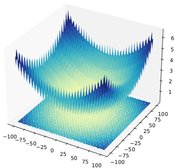
Slika 23: 3D grafikon dvodimenzionalne Griewank funkcije
