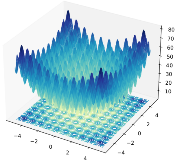
Slika 21: 3D grafikon dvodimenzionalne Rastrigin funkcije
