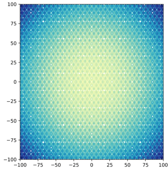
Slika 24: Kontur grafikon dvodimenzionalne Griewank funkcije
