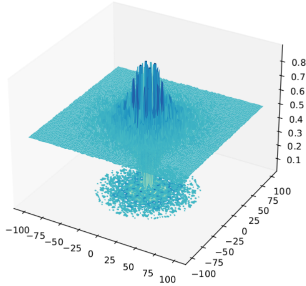
Slika 29: 3D grafikon dvodimenzionalne Schaffer funkcije
