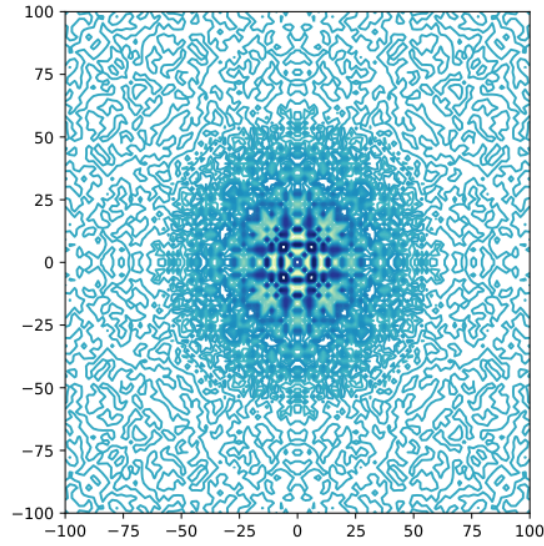
Slika 30: Kontur grafikon dvodimenzionalne Schaffer funkcije
