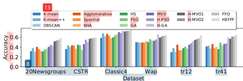
Slika 37: Uporedni prikaz rezultata tačnosti HEFFF metode i ostalih komparabilnih metoda
