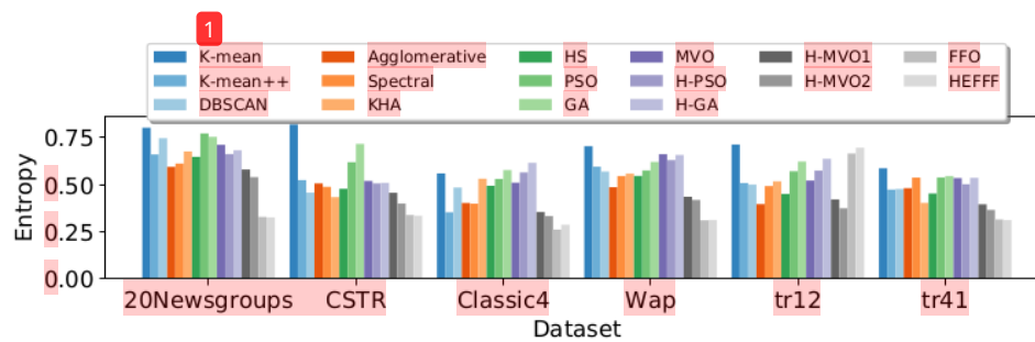
Slika 42: Uporedni prikaz rezultata entropije HEFFF metode i ostalih komparabilnih metoda
