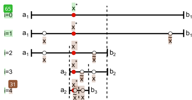
Slika 7: Primer OBL-a u jednodimenzijonalnom prostoru
