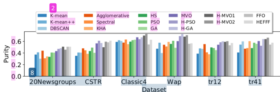
Slika 41: Uporedni prikaz rezultata čistoće HEFFF metode i ostalih komparabilnih metoda
