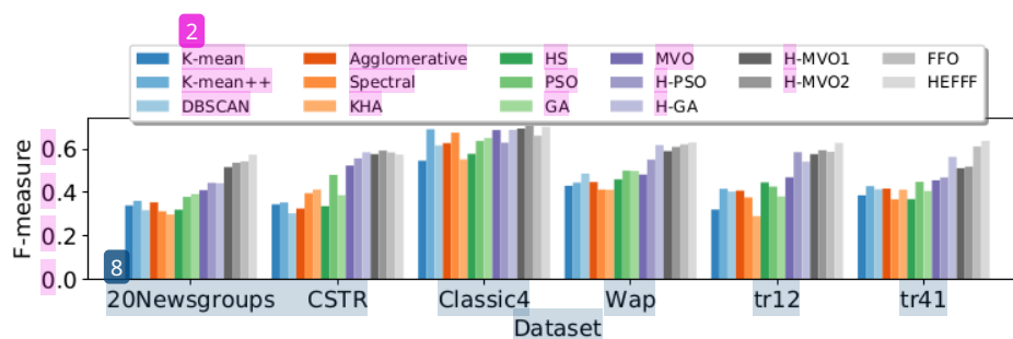
Slika 40: Uporedni prikaz rezultata F-mere HEFFF metode i ostalih komparabilnih metoda
