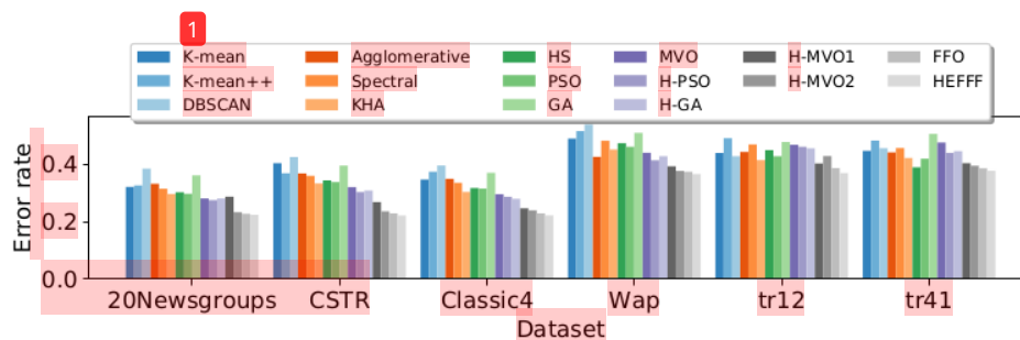
Slika 36: Uporedni prikaz rezultata stope greške HEFFF metode i ostalih komparabilnih metoda
