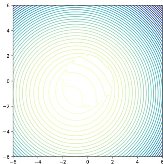
Slika 32: Kontur grafikon dvodimenzionalne Happy Cat funkcije
