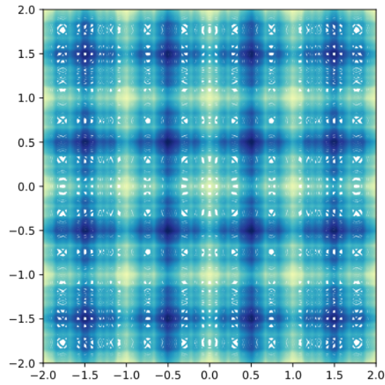
Slika 26: Kontur grafikon dvodimenzionalne Weierstrass funkcije
