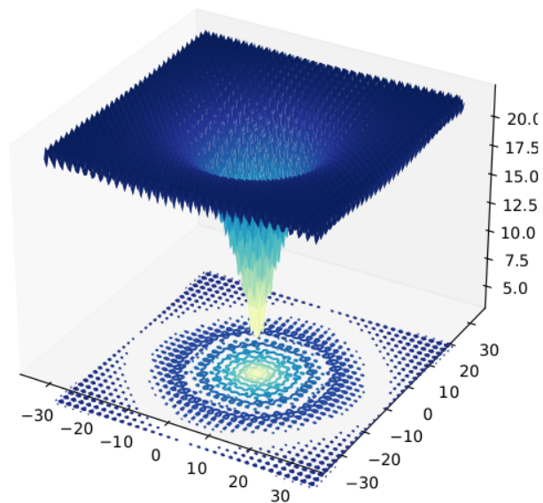
Slika 33: 3D grafikon dvodimenzionalne Ackley funkcije
