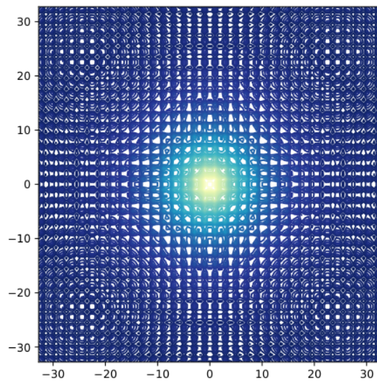
Slika 34: Kontur grafikon dvodimenzionalne Ackley funkcije
