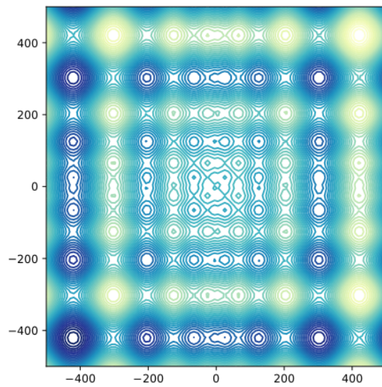
Slika 28: Kontur grafikon dvodimenzionalne Schwefel funkcije
