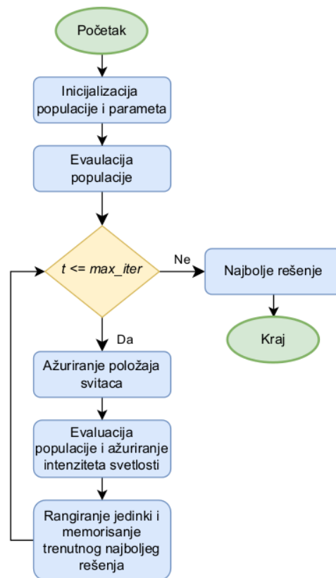
Slika 6: Dijagram toka algoritma svica
