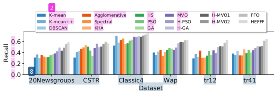
Slika 39: Uporedni prikaz rezultata odziva HEFFF metode i ostalih komparabilnih metoda
