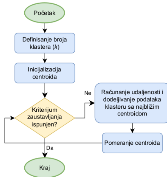
Slika 16: Dijagram toka algoritma K-srednjih vrednosti
