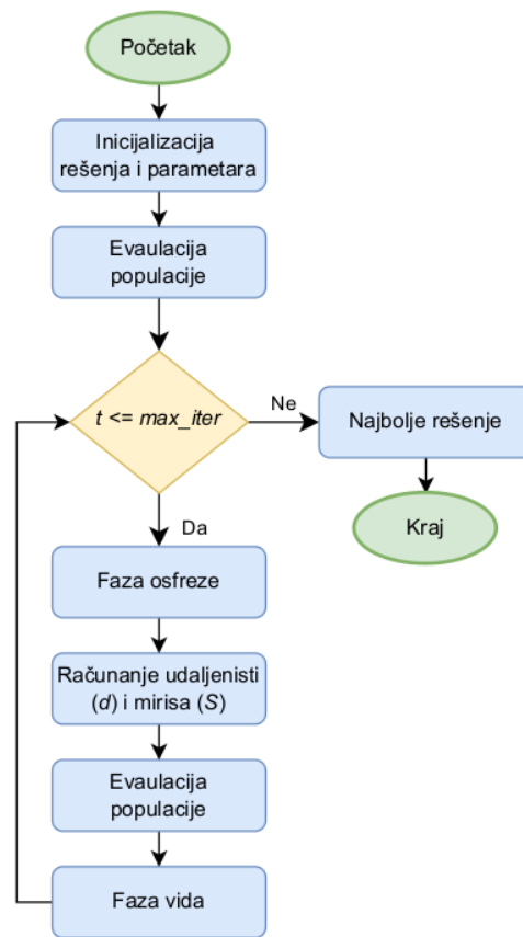
Slika 5: Dijagram toka originalnog algoritma voćne mušice
