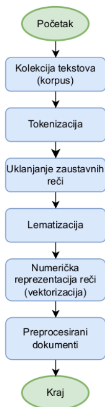
Slika 18: Dijagram toka procesa obrade ulaznih tekstualnih podataka
