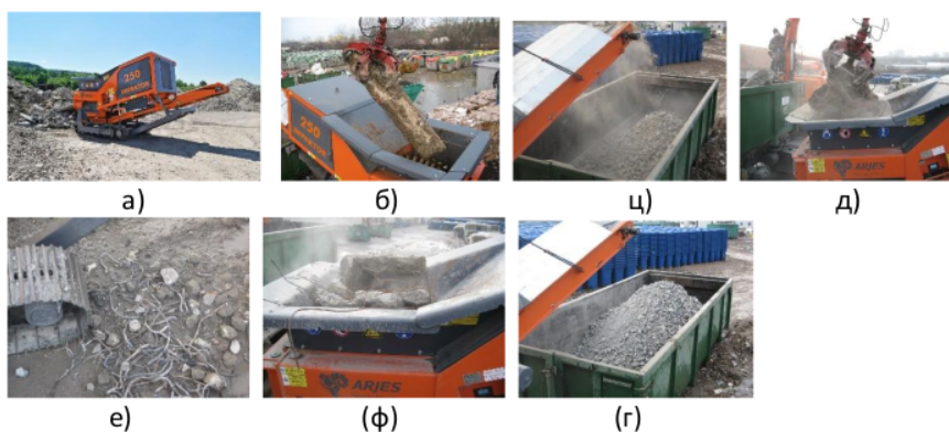
Слика 12- Процес дробљења
