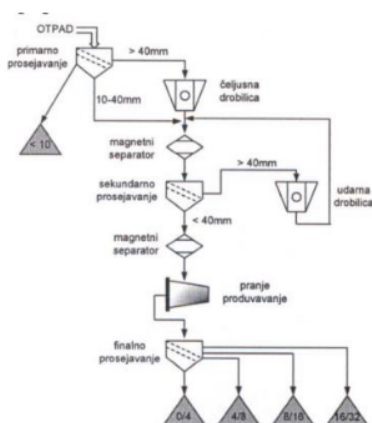
Слика 3 -Шематски приказ процеса ресиклаже грађевинског отпада
