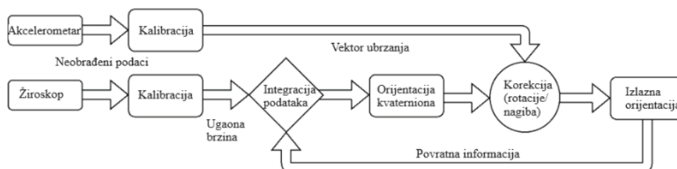
Slika 17. Pojednostavljeno prikazivanje filtera. Orijentacija je prvobitno određena integracijom ugaone brzine dobijne od žiroskopa nakon kalibracije. Orijentacija se zatim koriguje (rotacija i nagib) sa vektorom ubrzanja [79].
