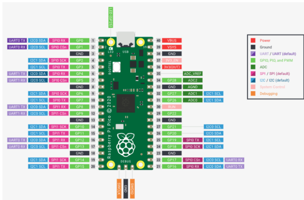
Slika 24. Pinout dijagram Raspberry Pi Pico RP2040
