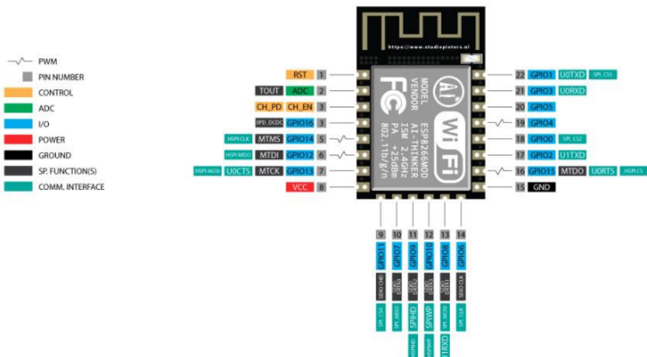
Slika 32. Pinout dijagram za ESP8266 Wi-Fi modul
