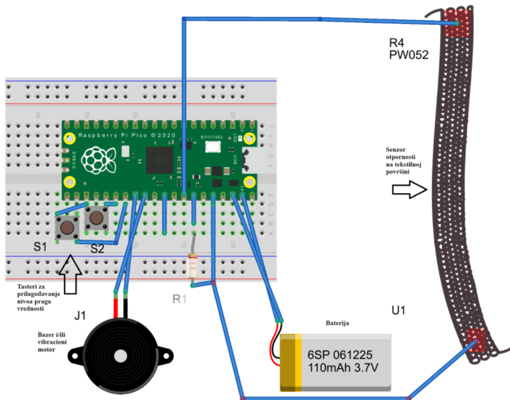
Slika 25. Grafički prikaz povezanih komponenti sa mikrokontolerom
