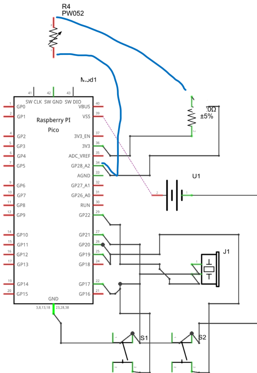
Slika 26. Šematski prikaz povezivanja komponenti
