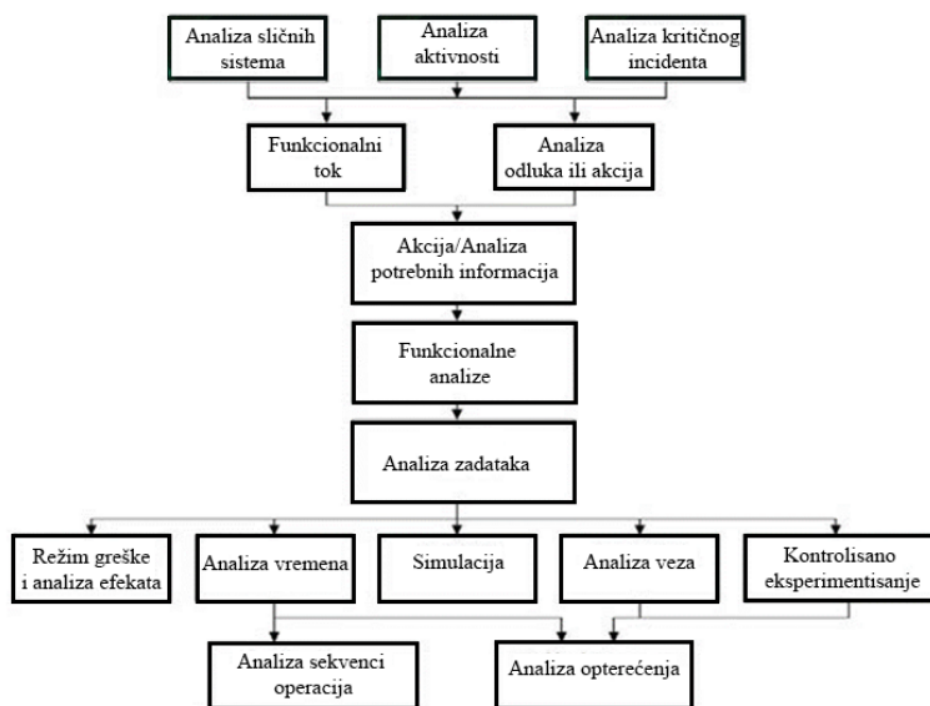
Slika 14. Chapanisov dijagram toka analize razvoja odeće specijalne namene
