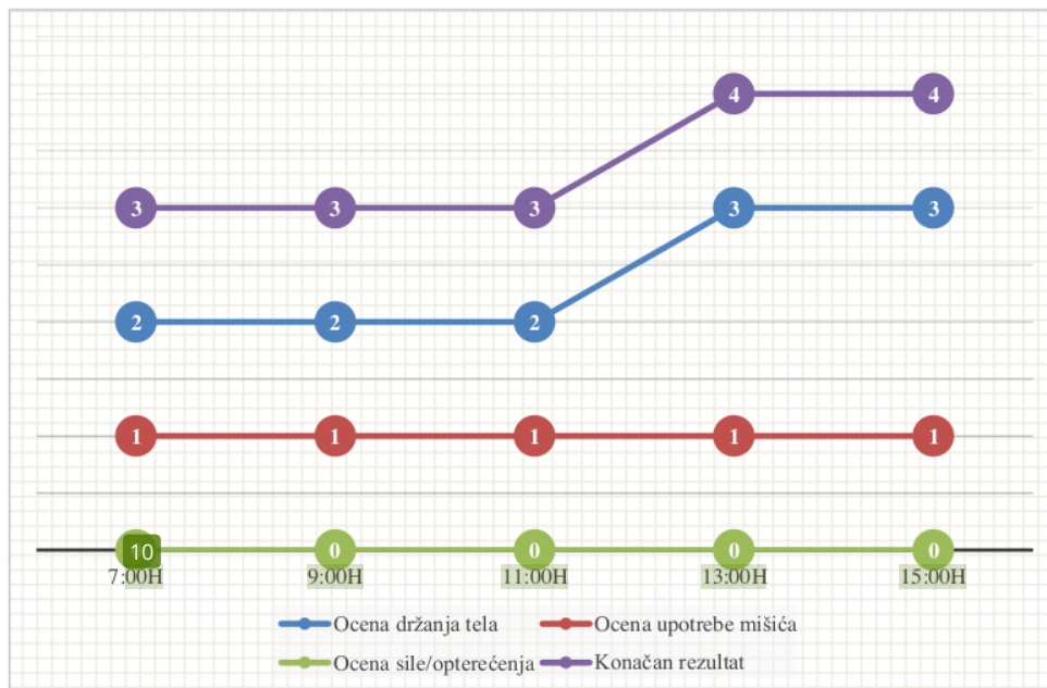
Slika 37. Grafikon pokazuje poboljšanja u smanjenju rizika ergonomije
