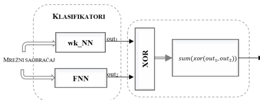
Slika 17. XOR detektor
