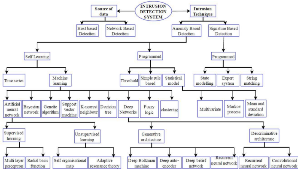
Slika 3. Klasifikacija IDS-a
