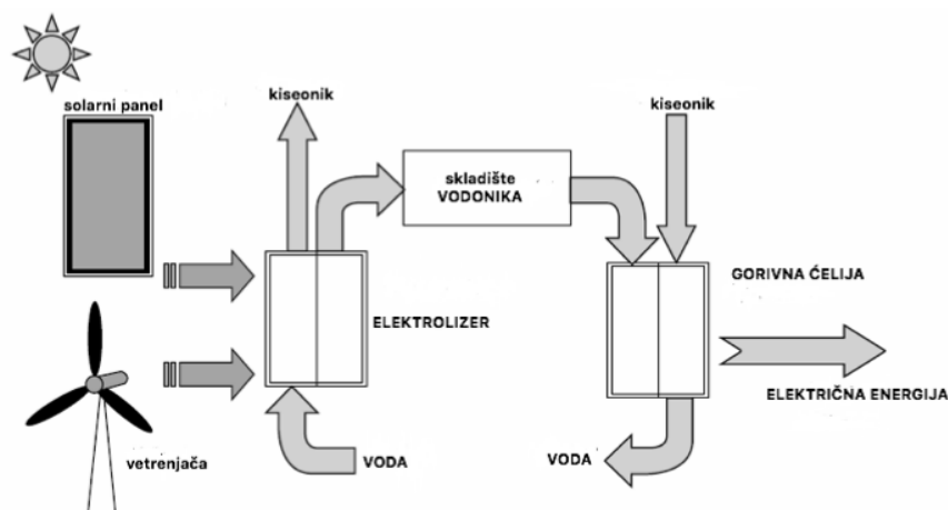
Slika 2.8. OIE u sprezi sa elektrolizerom i gorivnim ćelijama proizvode zelenu električnu energiju (preuzeto i modificirano iz [57])
