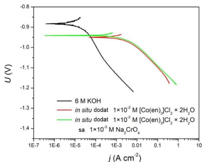
Slika 5.6. Tafelova polarizaciona kriva za reakciju izdvajanja vodonika u 6M KOH i polarizacione krive nakon in situ dodatog Co-Cr aktivatora u različitim odnosima pri temperaturi od 333K [54]
