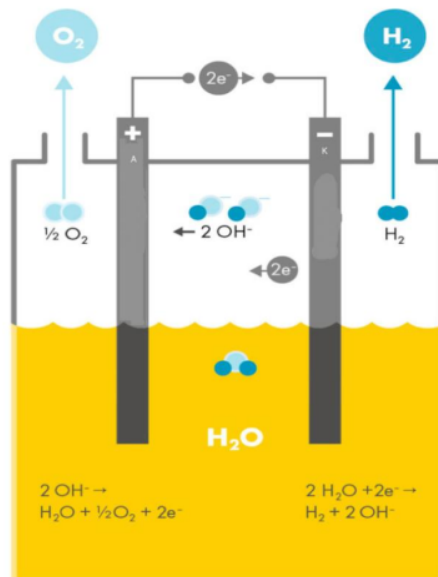
Slika 2.2. Princip procesa elektrolize (preuzeto i modificirano iz [39])
