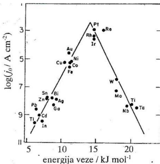
8 Slika 2.4. Gustina struje u funkciji energije veze vodonik-metal na različitim metalima (vulkanska kriva) [45][48]
