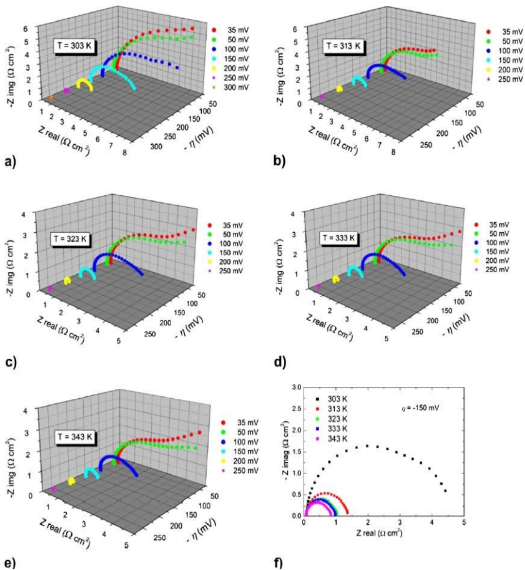
Slika 5.8. 3D spektri impedanse snimljeni na različitim temperaturama predstavljeni Niquist-ovim dijagramima (a-e) i uporedni prikaz Nyquist-ovih dijagrama na nadnaponu od -150 mV (f) [54]
