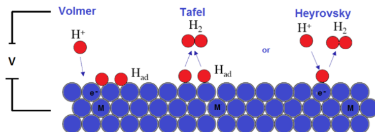
Slika 2.5. Stupnjevi u procesu izdvajanja vodonika (preuzeto iz [54])
