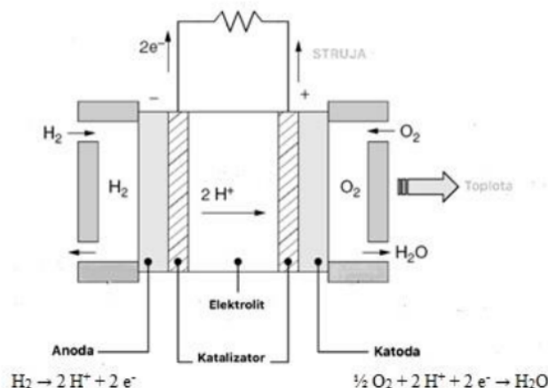
Slika 2.6. Šematski prikaz konfiguracije gorivne ćelije sa membranom propusnom za protone (PEM) (preuzeto i modifikovano iz [56])
