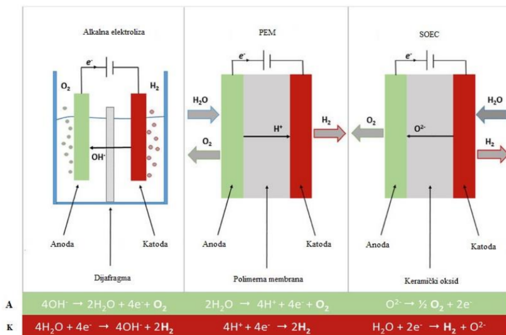
Slika 2.3. Šematski prikaz tri elektrolitičke tehnologije za dobijanje "zelenog" vodonika (preuzeto i modifikovano iz [46])
