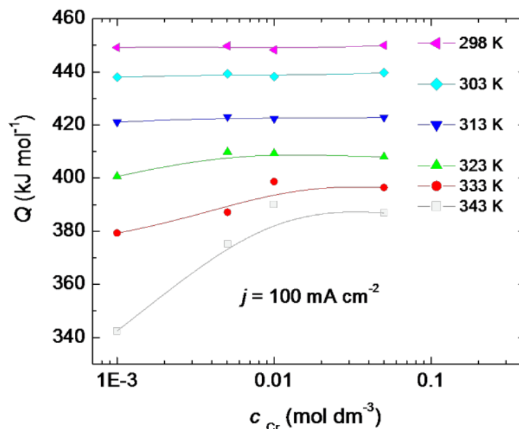
Slika 5.2. Potrošnja energije alkalnog elektrolizera u funkciji koncentracije in situ dodatih j.a. na različitim temperaturama pri konstantnoj gustini struje od 100mAcm -2 [116]
