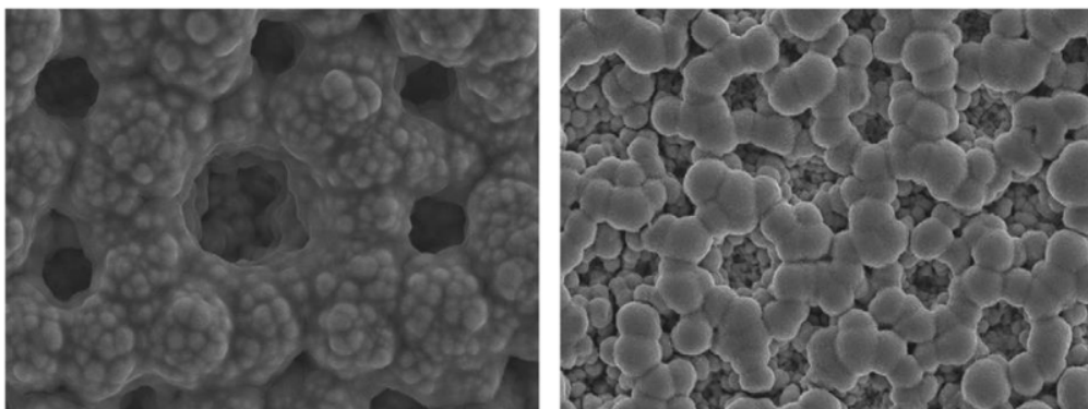
Slika 5.5. Fotografije dobijene SEM tehnikom, na kojima se vidi površina niklene katode nakon elektrolitičkog in situ procesa (Levo: 0.01M Co kompleks, desno: 0.01M Co kompleks +0.001M Cr so) na uveličanju od 2000 puta [116]
