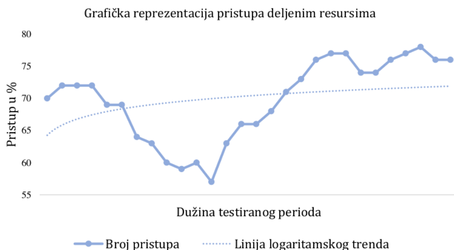
Ilustracija 15 - Grafička reprezentacija pristupa deljenim resursima
