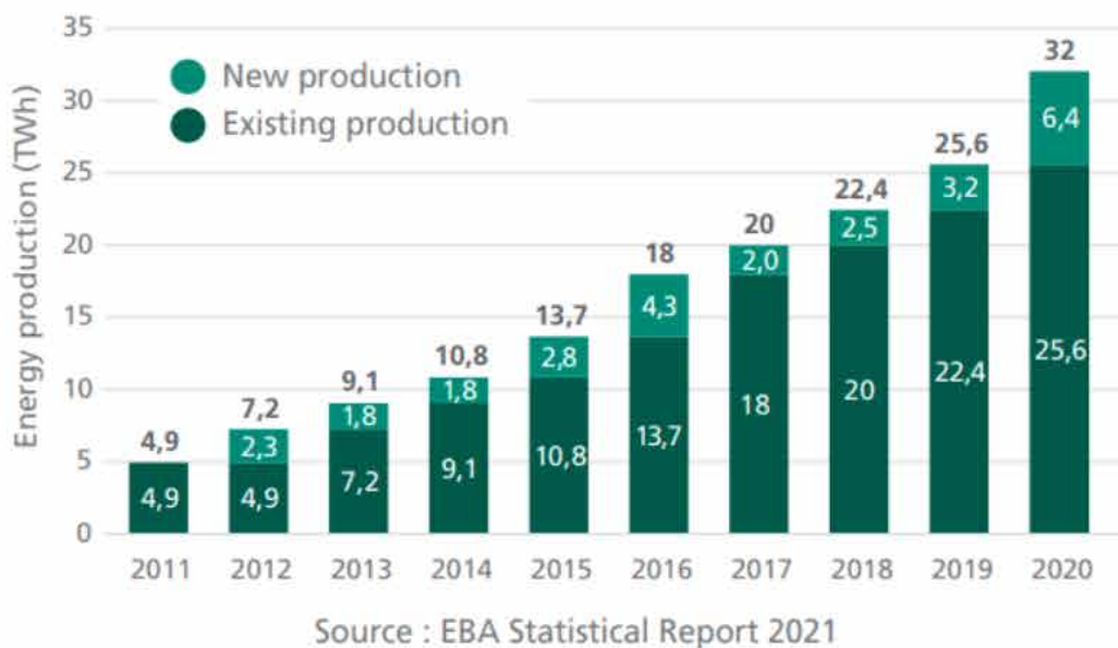
Slika 2, Produkcija biometana u GIE (67 članova u 27 država Evrope) (Izvor: GIE_EBA_BIO_2021_A0_FULL_3D_253_online.pdf)
