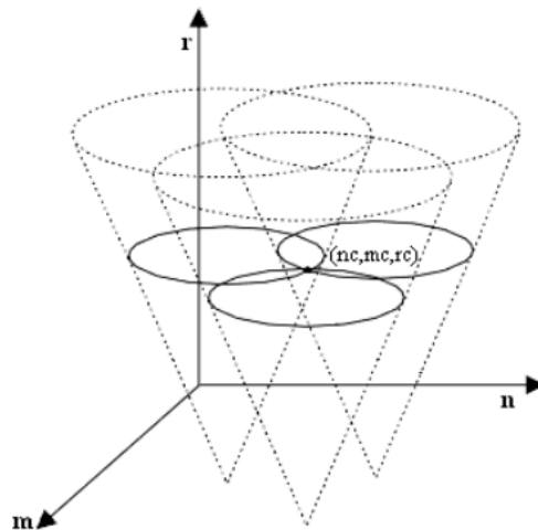
Slika 4-9 Hafova transformacija kružnica
