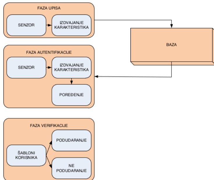
Slika 4-12: Biometrijski sistemi- faze
