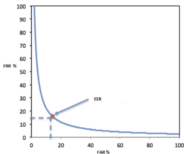
Slika 4-13 Primer ROC krive [8]
