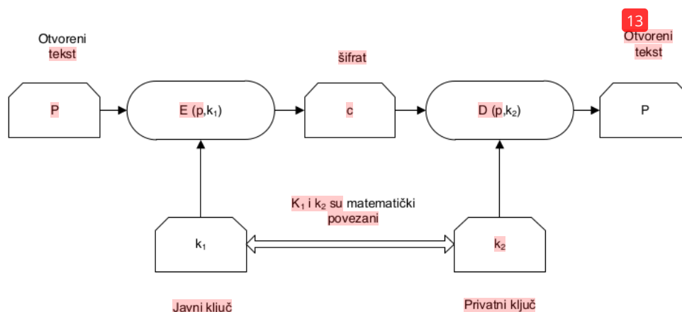
Slika 3-9 Algoritam sa javnim ključem
