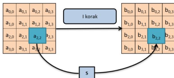
Slika 3-5 I korak - zamena bajtova
