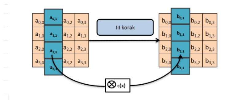
Slika 3-7 III korak - Mešanje podataka po kolonama
