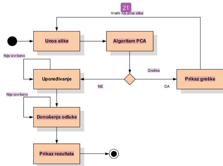
Slika 4-4: Dijagram aktivnosti
