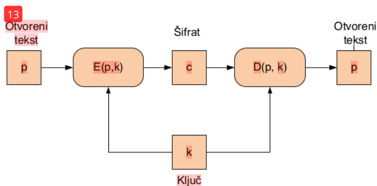
Slika 3-2 Simetrični algoritmi
