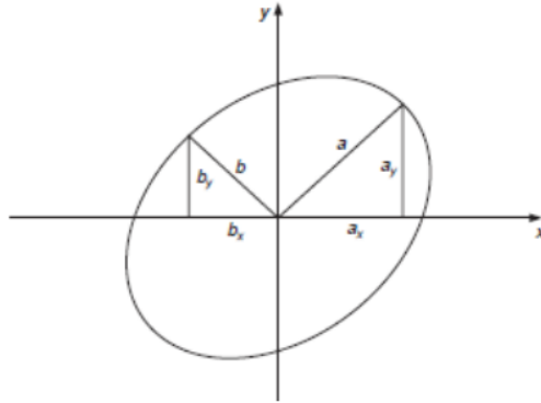
Slika 4-10 Hafova transformacija elipsa
