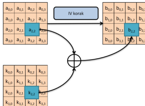
Slika 3-8 AES IV korak - dodavanje podključa
