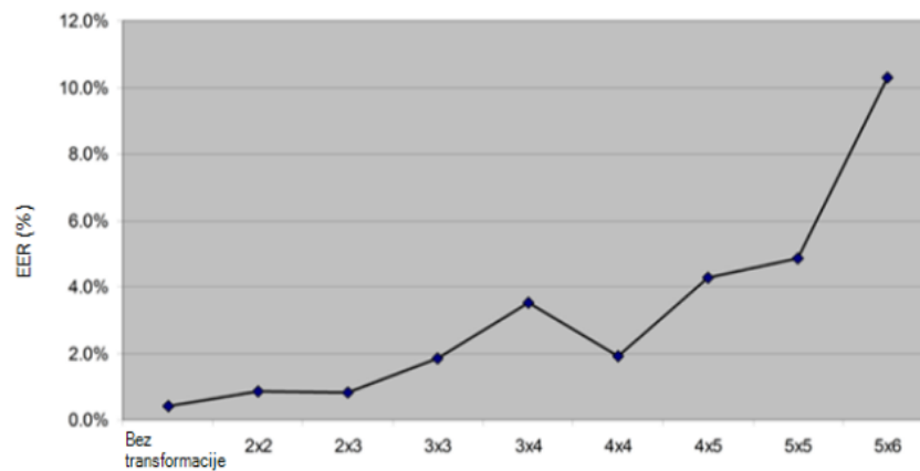
Slika 5-5 Određivanje optimalnog broja ćelija u neinvertibilnoj transformaciji
