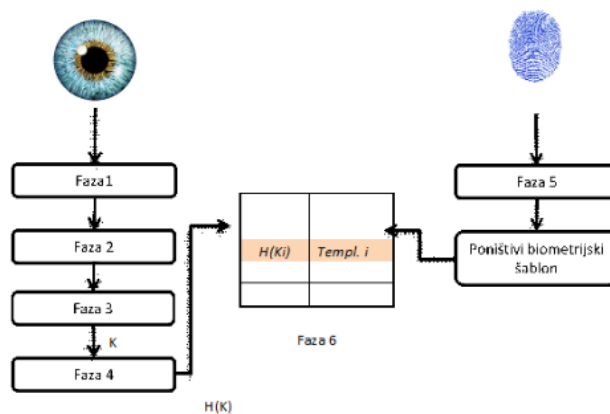
Slika 5-1 Predloženo rešenje – faza upisa
