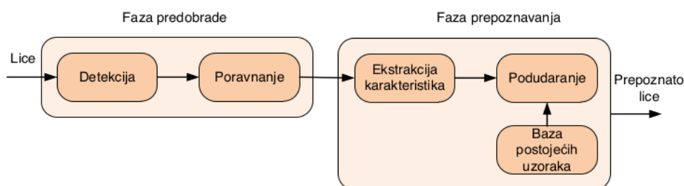
Slika 4-3: Prepoznavanje lica opisano kroz faze
