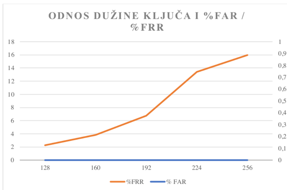
Slika 5-8 Grafički prikaz % FAR i % FRR
