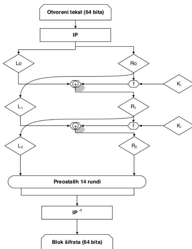
Slika 3-3 DES algoritam [36]
