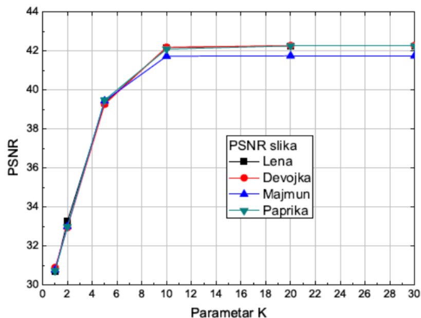
Slika br. 35 PSNR iz prenesenih slika Lena, Devojka, Majmun i Paprika kroz Rajsov FSO turbulentni kanal
