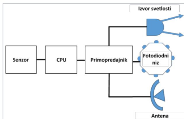
Slika br. 9 Blok dijagram RF/FSO bežičnog senzorskog čvora u BNTSM
