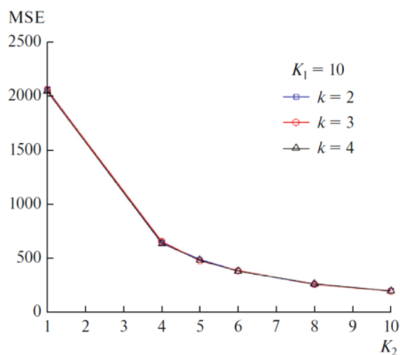
Slika br. 47 Kvalitativno merenje MSE za prenetu sliku Lena preko boresighta/dvostruke Rajsove turbulentncije za različite vrednosti parametra veličine bloka k .
