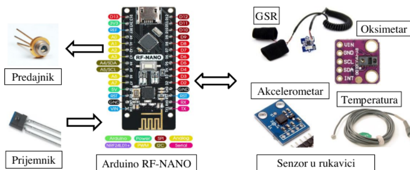
Slika br. 26 Senzorski čvor br.3 u rukavici
