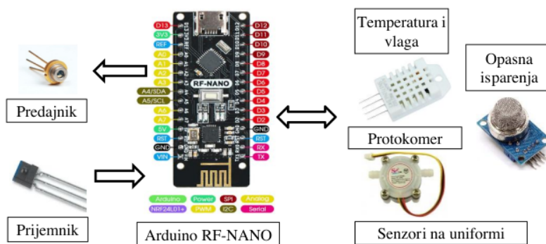
Slika br. 27 Senzorski čvor br. 4 na uniformi
