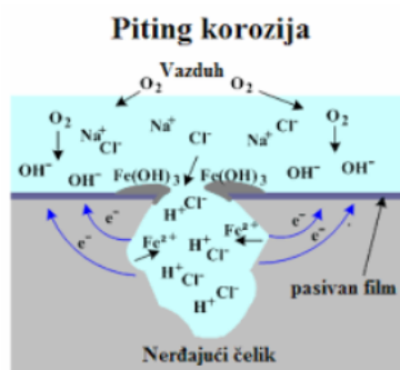
Slika 2. Primer piting korozije čelika [7]
