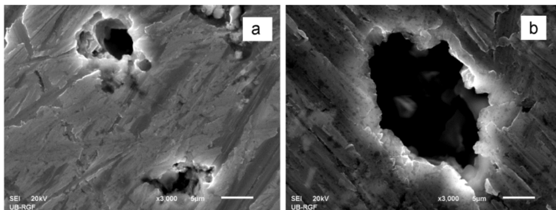
Slika 13. Izgled pitova nastalih tokom ispitivanja korozije kod legure aluminijuma a) prirodno starene (NA) i b) veštački starene (AA) [67]
