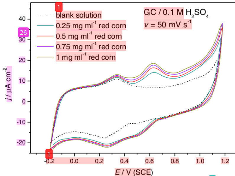
Slika 8. CV voltamogrami za različite koncentracije pigmenta crvenog kukuruza na GC elektrodi u 0.1 M H 2 SO 4 ; pri brzini promene polarizacionog potencijala sa vremenom od v = 50 \text{ mV s}^{-1} [61]
