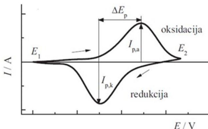
Slika 3. Zavisnost struje od potencijala (ciklični voltamogram) [2]
