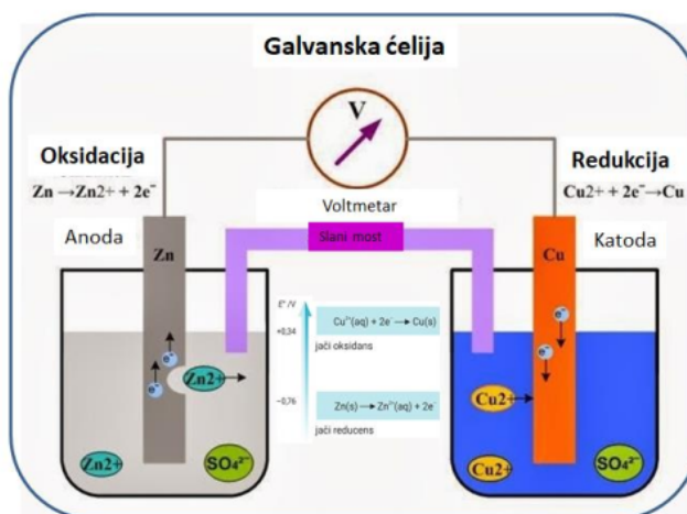
Slika 1. Primer elektrohemijske korozije dva metala
