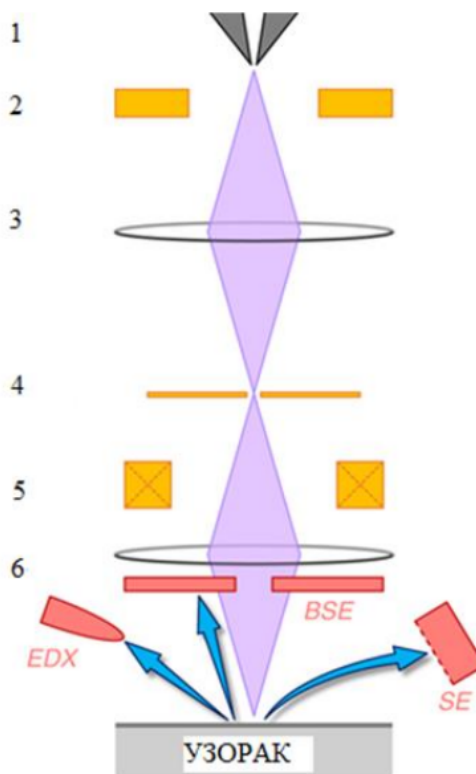
Slika 5. Delovi skenirajućeg elektronskog mikroskopa
