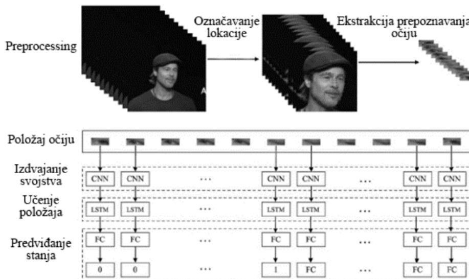
Slika 12 - Pregled LRCN metode [12]
