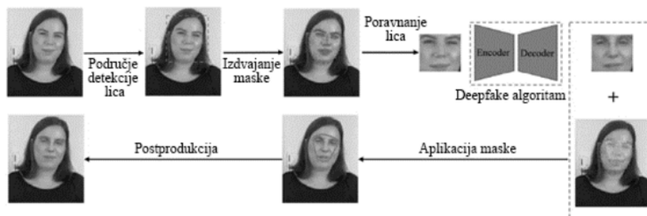
Slika 3 - Proces generisanja video kadrova zamene lica [12]
