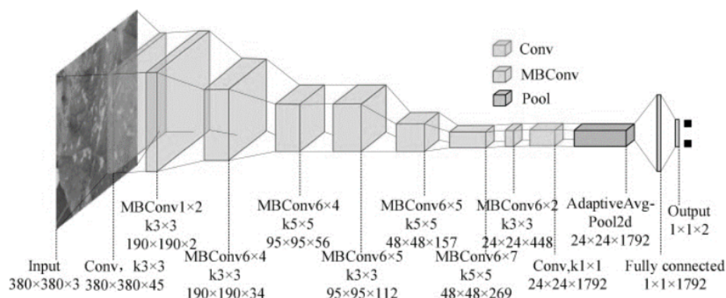
Slika 24 – Mrežna struktura EfficientNet-B4
