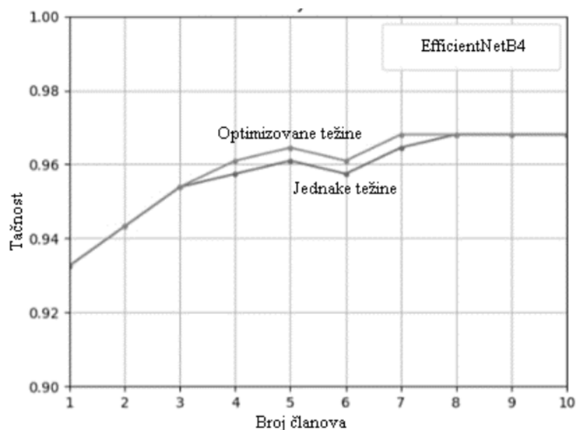
Grafikon 5 - Prikaz rezultata za EfficientNetB4
