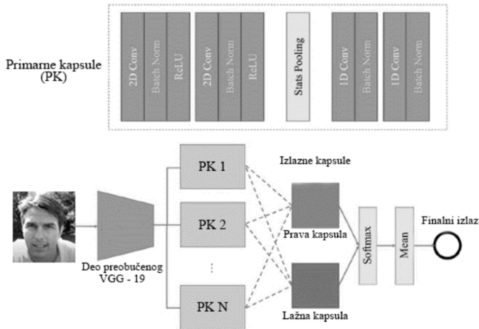
Slika 8 – Prikaz šeme kapsule [27]
