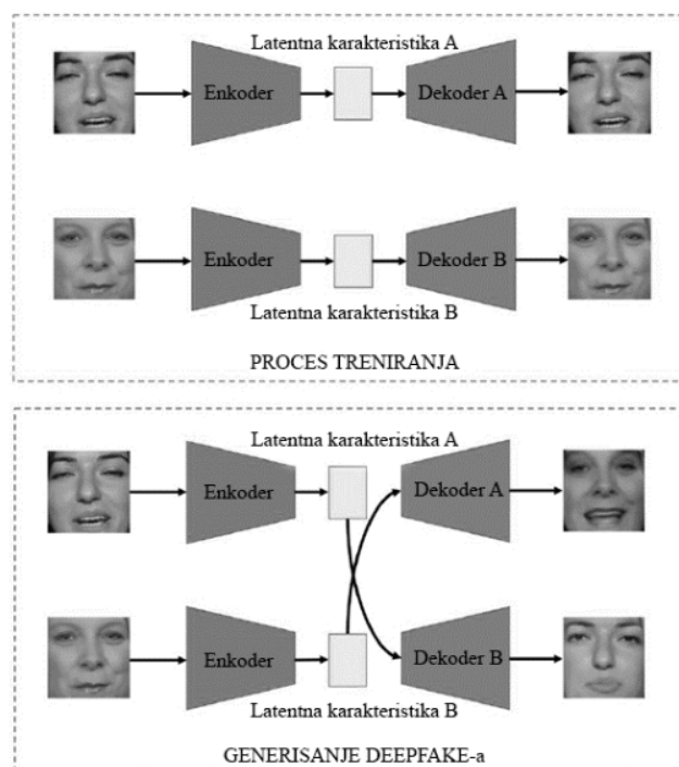
Slika 4 - Autoenkoderi koji se koriste za zamenu lica [12]
