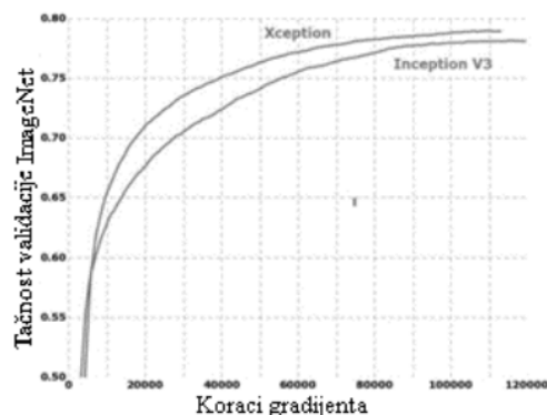
Grafikon 1 – Performanse obuke na skupu podataka ImageNet
