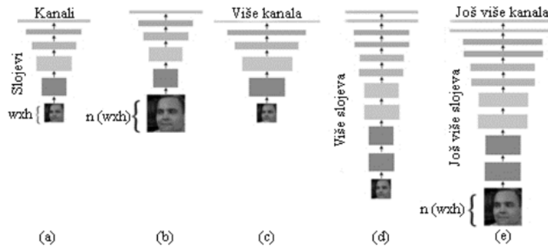
Slika 25 – Poređenje skaliranja modela
