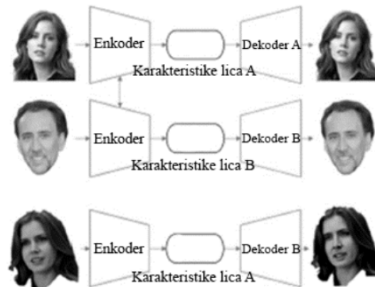
Slika 2 – Dve mreže koje dele isti koder
