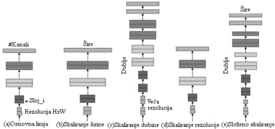
Slika 23 – Skaliranje svih dimenzija u konstantnom odnosu [103]
