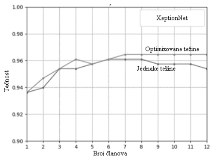
Grafikon 4 - Prikaz rezultata za XceptionNet
