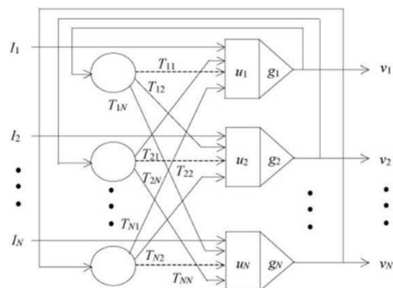
Slika 19 – Struktura Hopfildove neuralne mreže [75]
