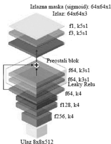
Slika 7 – Tehnika dekodiranja alata za zamenu lica [27]
