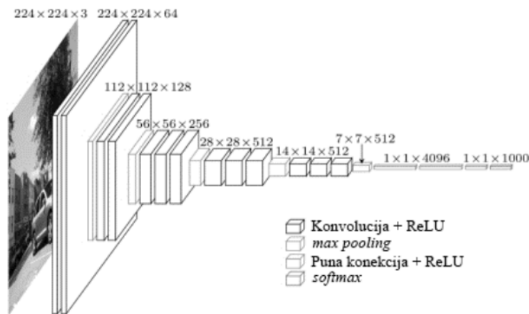
Slika 20 – VGG arhitektura neuronske mreže [82]
