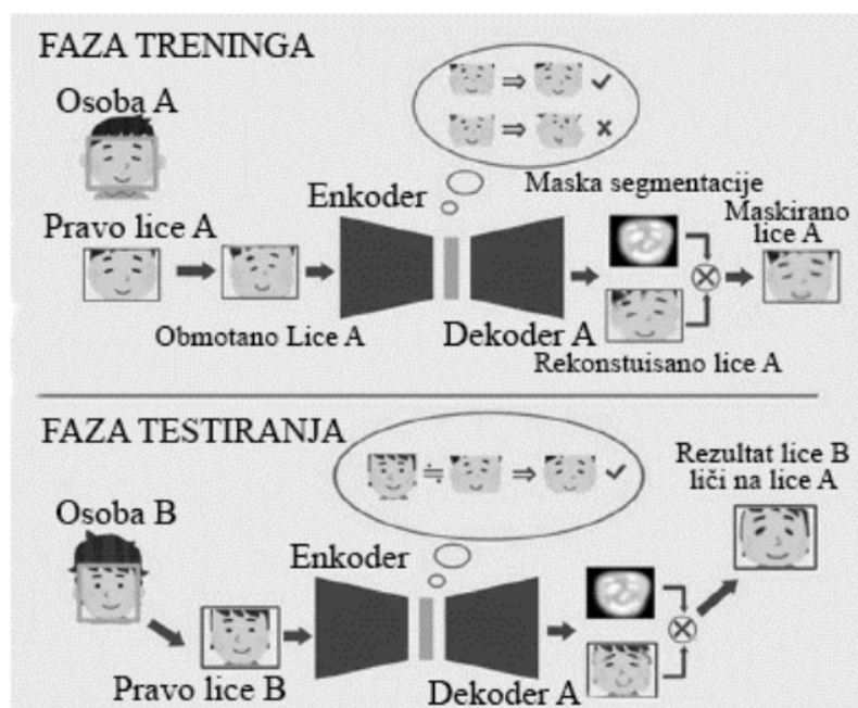
Slika 5 - Prikaz GAN metode [12]
