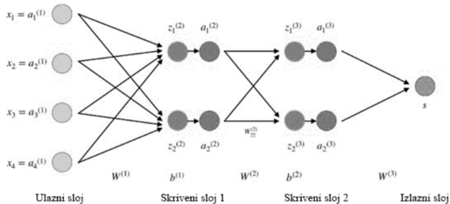
Slika 16 - Jednostavna četvoroslojna ilustracija neuronske mreže
