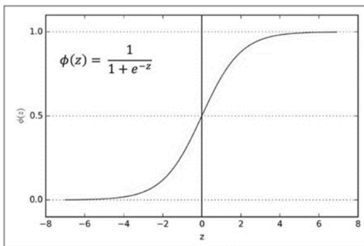
Slika 15 - Sigmoidna kriva
