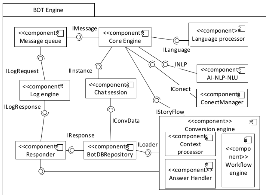
Slika 24. Dijagram komponenti BOT engine-a
