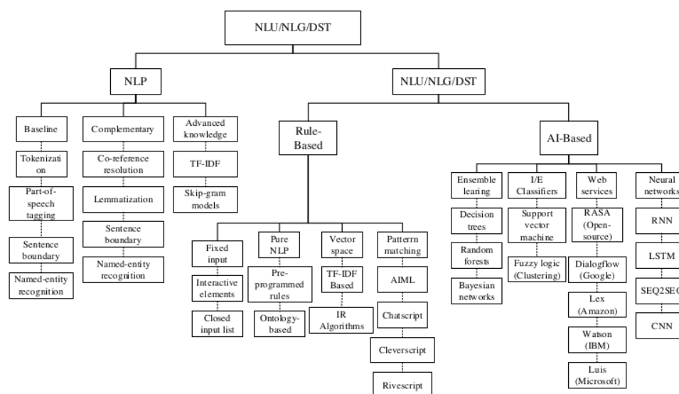
Slika 6. Metode, tehnike i tehnologije razvoja četbota
