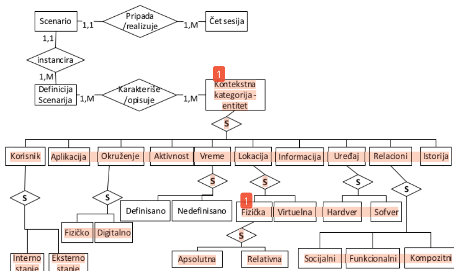
Slika 25. Referentne kontekstne kategorije
