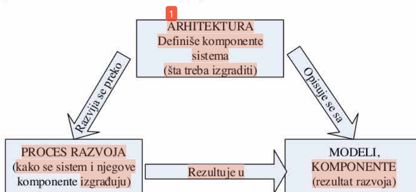
Slika 18. Metodološki principi
