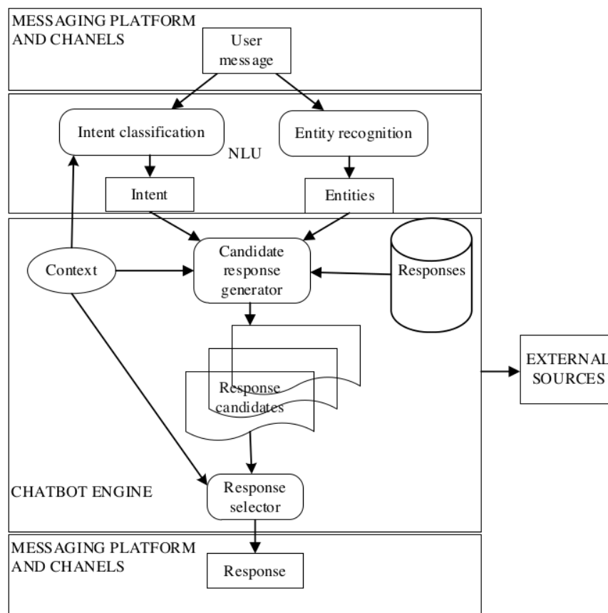
Slika 19. Opšta referentna arhitektura
