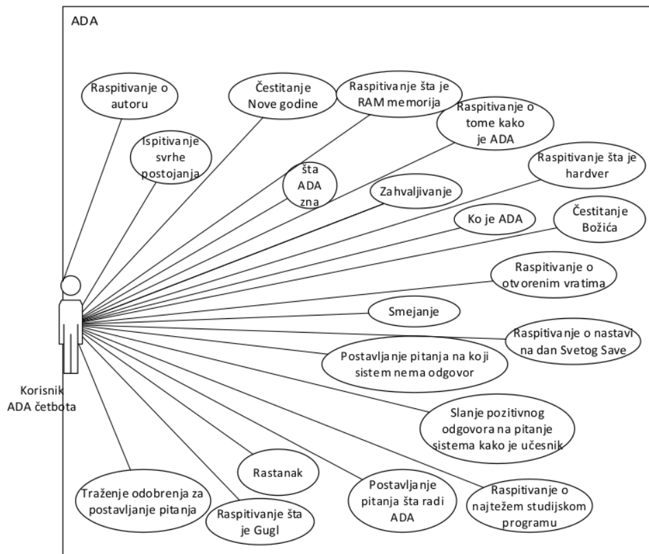
Slika 37. Dijagram slučajeva korišćenja za pružanje opštih informacija
