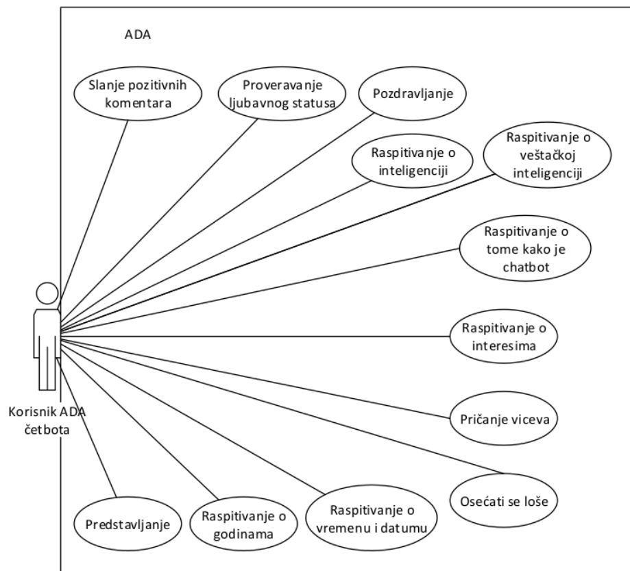
Slika 38. Dijagram slučajeva korišćenja za zabavne scenarije
