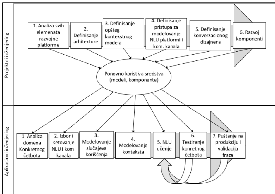
Slika 22. Dualni životni ciklus razvoja adaptivne platforme
