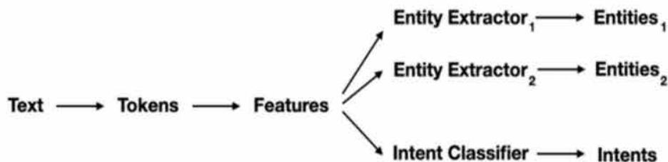
Slika 14. Ekstrakcija entiteta u NLU planu izvršavanja
