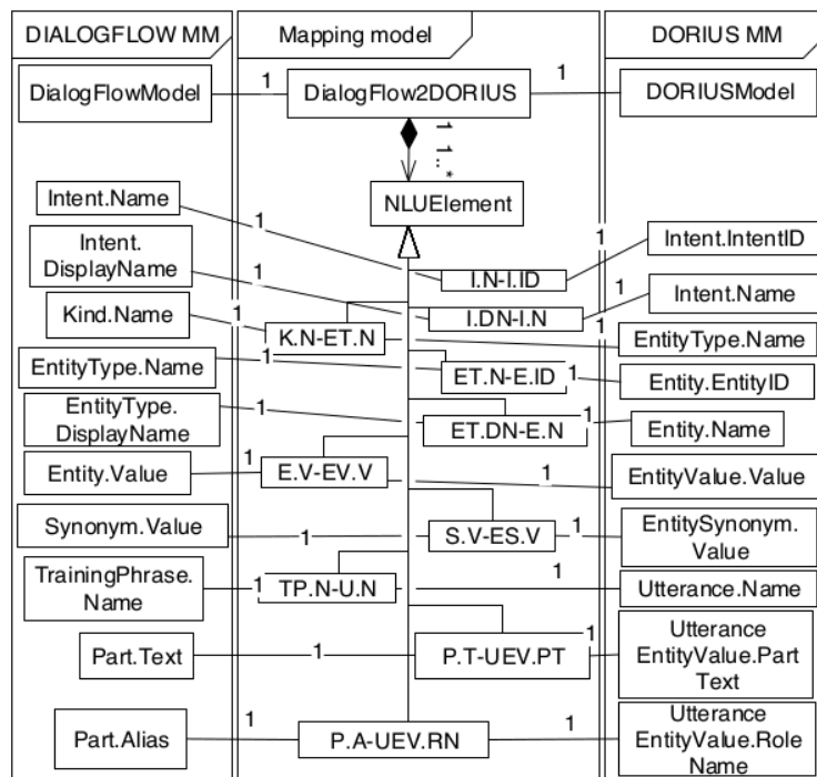
Slika 31. Model preslikavanja Dialogflow2DORIUS
