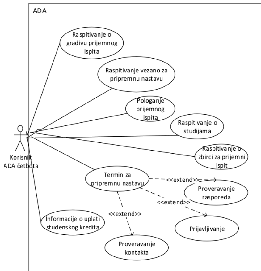
Slika 42. Dijagram slučajeva korišćenja za pripremnu nastavu i polaganje ispita
