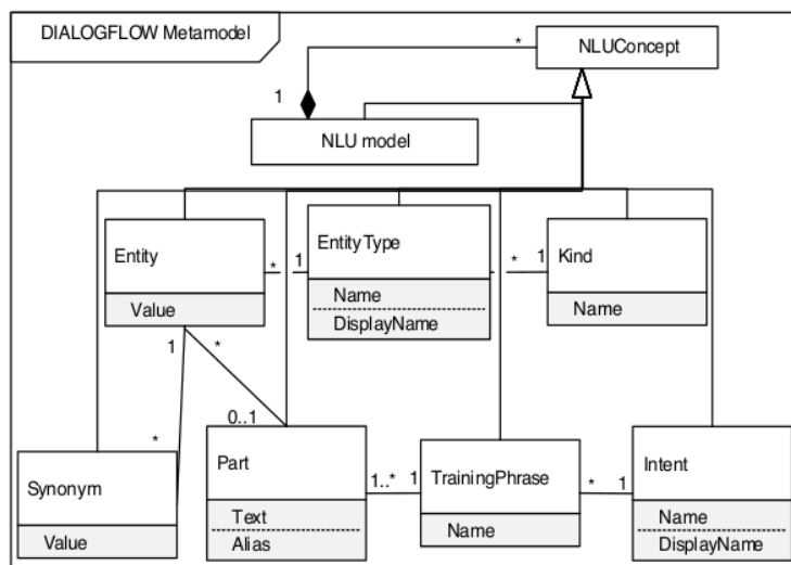
Slika 30. Dialogflow metamodel
