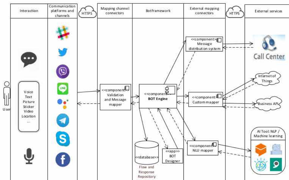
Slika 23. Logička arhitektura
