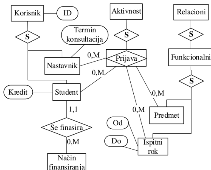
Slika 54. Primer kontekstnog modela
