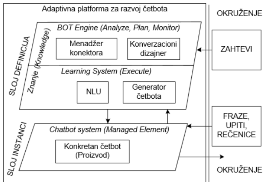
Slika 20. Referentna arhitektura adaptivne platforme za razvoja čebota
