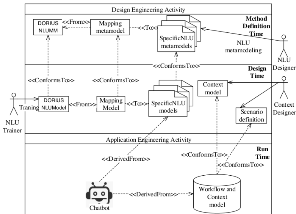
1 Slika 27. Arhitektura modela
