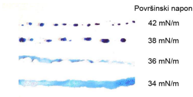
Slika 46: Primer testiranja površinskog napona folije sa različitim tečnostima
