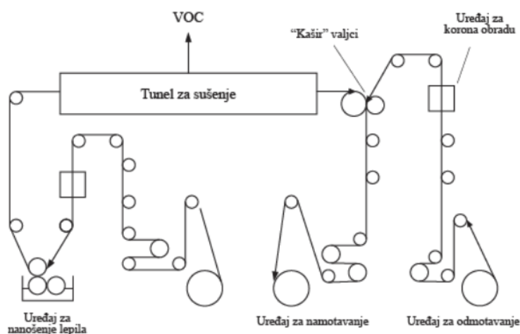
Slika 5: Postupak suvog kaširanja lepilom sa rastvaračem (Balaban, 2013)
