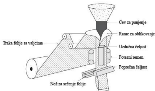
Slika 13. Vertikalna mašina za oblikovanje i pakovanje
