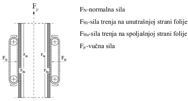
Slika 21: Kretanje folije pomoću vučnog remena (Hertlein, 1998)
