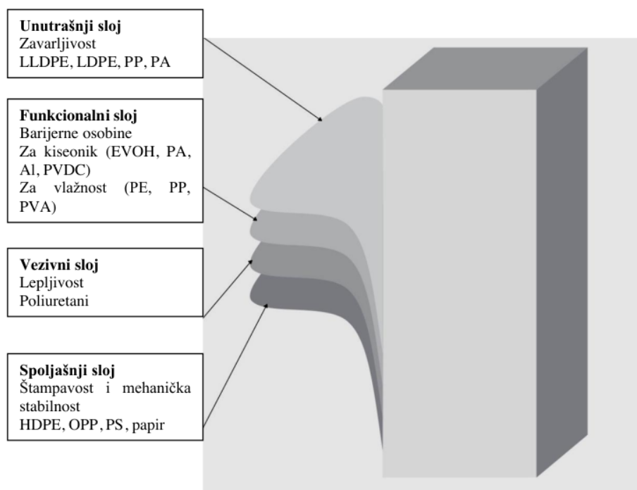
Slika 3: Različiti slojevi višeslojne ambalaže (Anukiruthika i dr., 2020)
