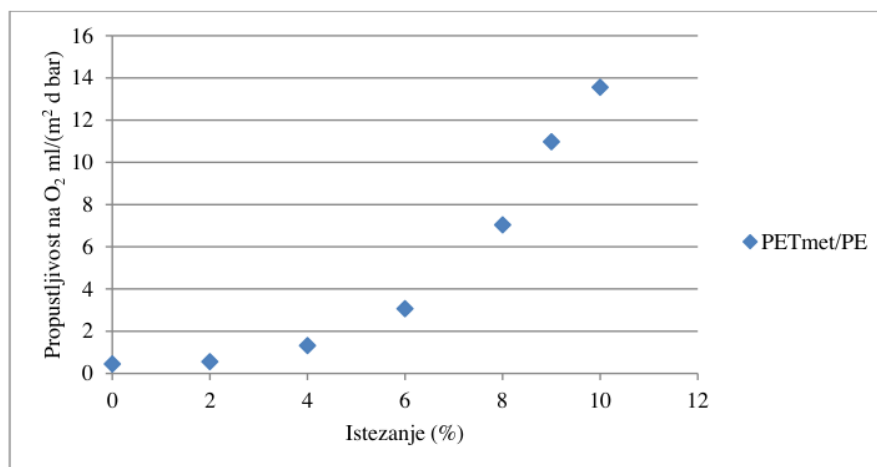
Slika 44: Uticaj istezanja na propustljivost kod PETmet/PE folije
