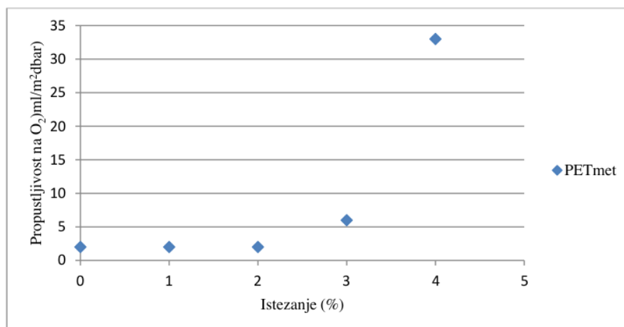
Slika 43: Uticaj istezanja na propustljivost kod PETmet folije
