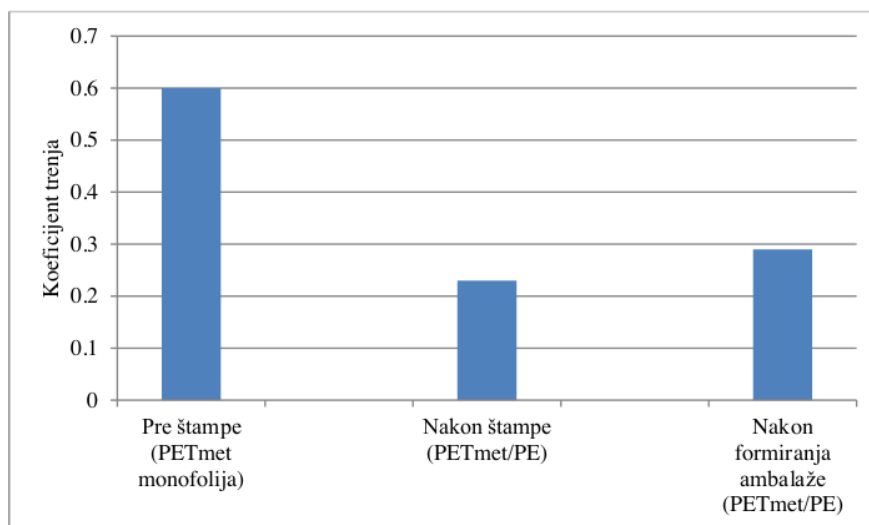
Slika 39: Koefficijenti trenja PETmet folije (pre) i nakon štampe i formiranja ambalaže (PETmet/PE)
