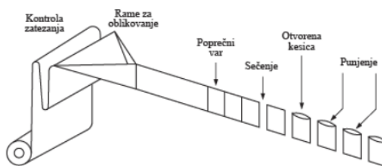
Slika 14: Horizontalna mašina za pakovanje
