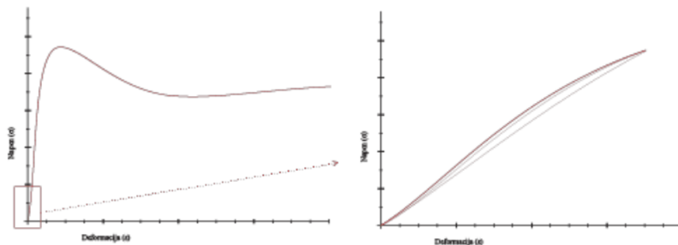
Slika 20: Određivanje modula sekante
