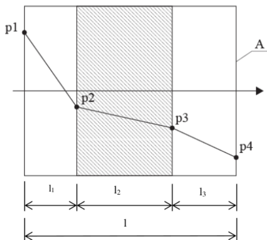
Slika 23: Prolaz gasa kroz višeslojnu foliju i razlika pritisaka kroz troslojnu višeslojnu foliju
