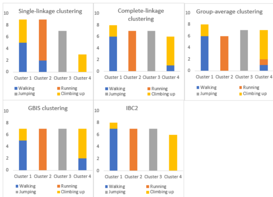
Slika 3: Komparativni rezultati klasterovanja, kada je broj klastera unapred dat, koristeći RealWorld bazu podataka
