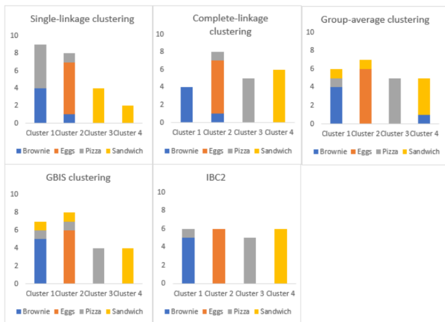
Slika 2: Komparativni rezultati klasterovanja, kada je broj klastera unapred dat, koristeći CMU-MMAC bazu podataka
