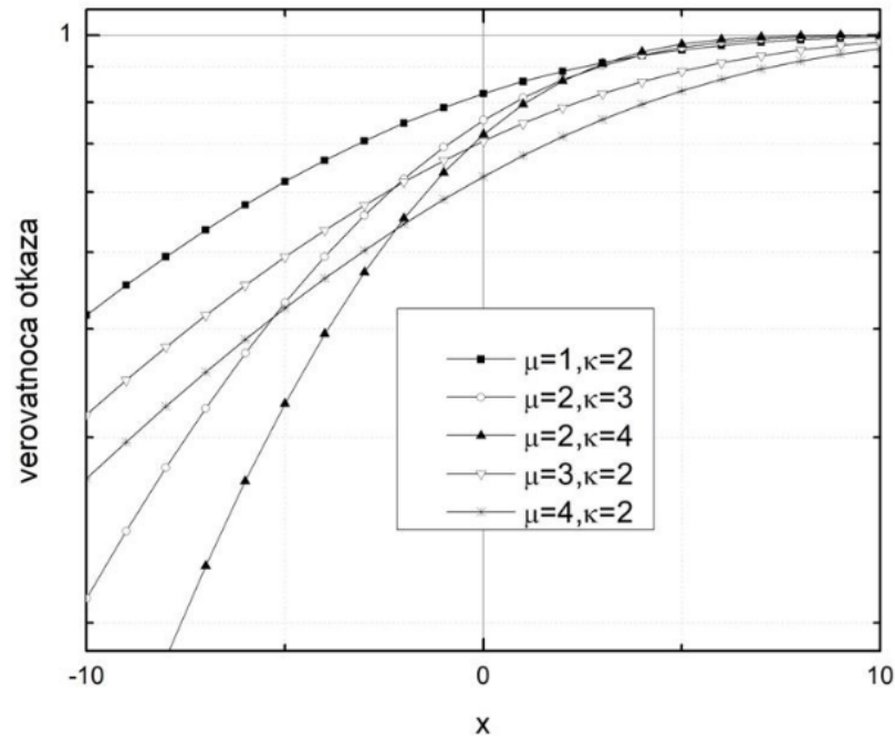
Slika 3.3. Verovatnoća otkaza bežičnog digitalnog telekomunikacionog sistema
