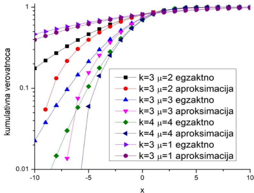
Slika 3.11. Kumulativna verovatnoća signala u zavisnosti od anvelope signala
