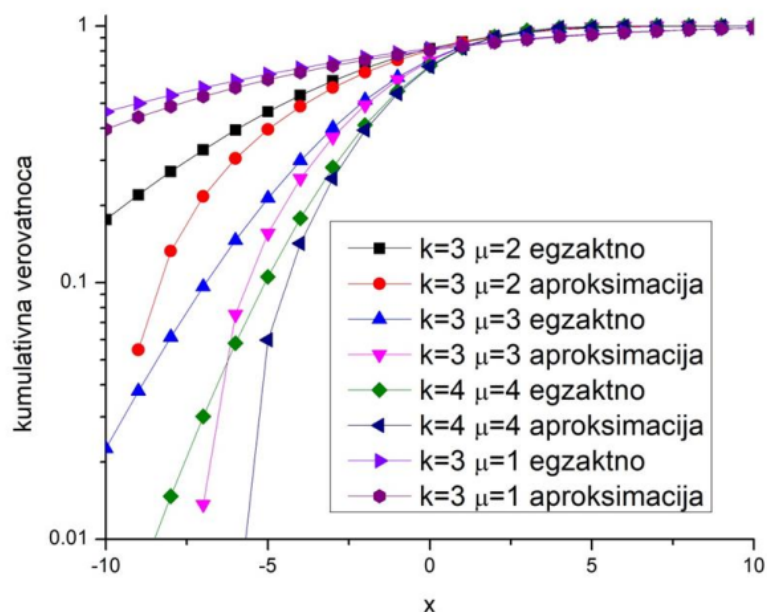
Slika 3.5. Kumulativna verovatnoća (k-μ) slučajnog procesa
