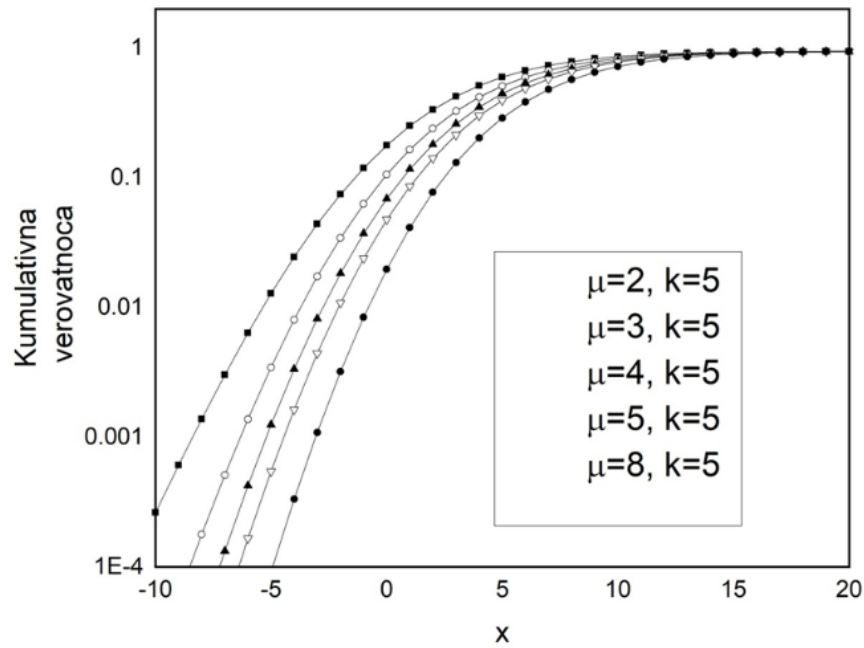
Slika 3.4. Kumulativna verovatnoća (k-μ) slučajnog procesa u zavisnosti od anvelope signala
