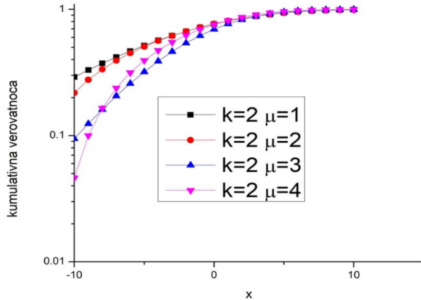
Slika 3.1. Kumulativna verovatnoća signala ( k - \mu ) nasumične varijable
