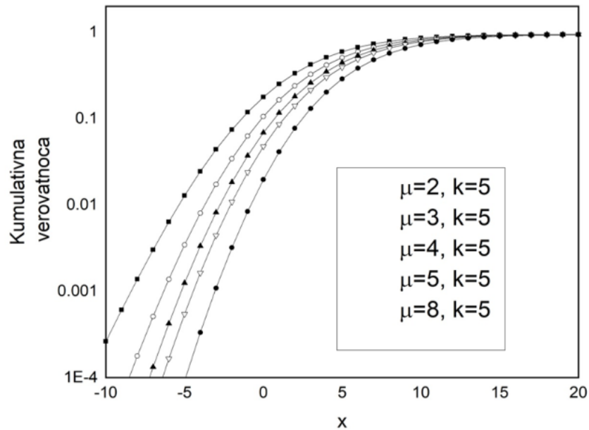
Slika 3.7. Kumulativna verovatnoća (k-μ) slučajne promenljive
