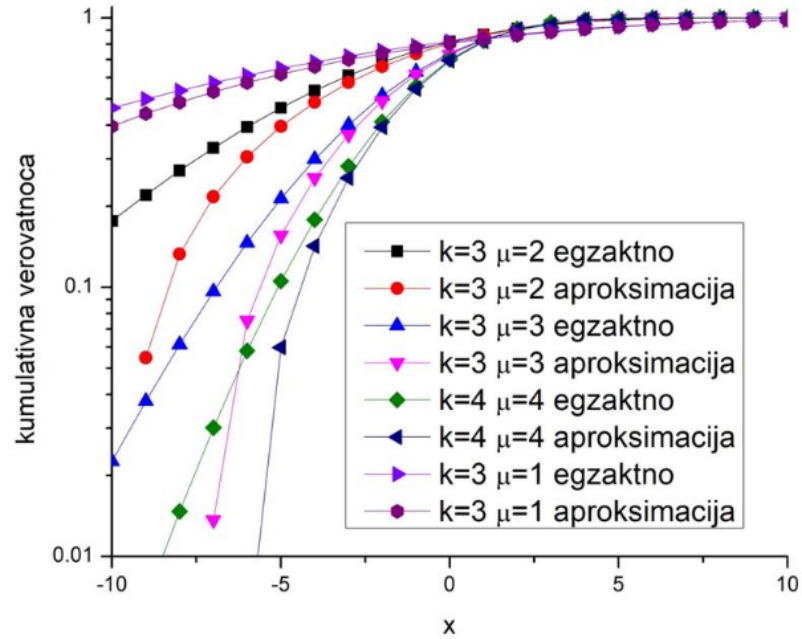
Slika 3.2. Kumulativna verovatnoća u zavisnosti od anvelope signala x
