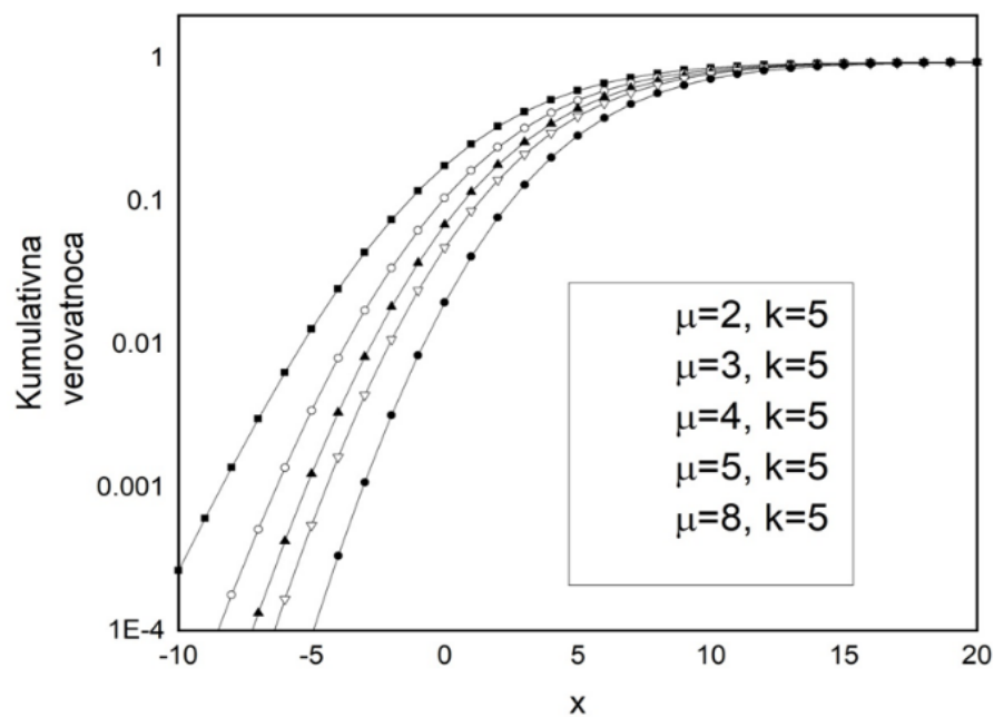
Slika 3.9. Kumulativna verovatnoća signala u zavisnosti od anvelope signala
