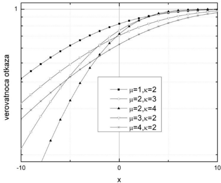
Slika 3.6. Verovatnoća otkaza bežičnog digitalnog telekomunikacionog sistema u prisustvu (k-\mu) fedinga
