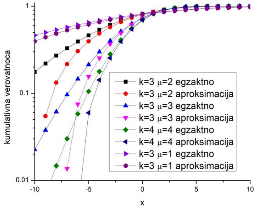
Slika 3.8. Kumulativna verovatnoća bežičnog digitalnog telekomunikacionog sistema
