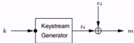
Slika 2.7: Proces dešifrovanje u aditivnim sekvencijalnim kriptografskim algoritmima, [15]
