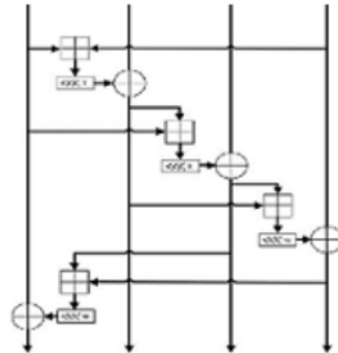
Slika 2.11: Deo transformacije u kriptografskom algoritmu Salsa 20
