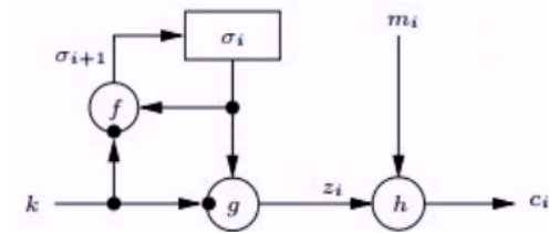
Slika 2.4: Proces šifrovanja eksterno sinhronizovanim sekvencijalnim kriptografskim algoritmom, [15]
