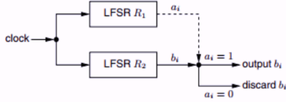
Slika 2.15: Grafički prikaz generatora neuniformne decimacije, [15]
