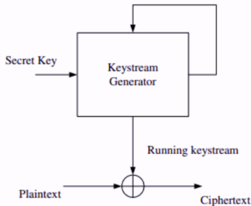
Slika 2.3: Grafički prikaz aditivnog sekvencijalnog kriptografskog algoritma
