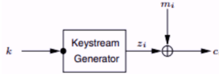
Slika 2.6: Proces šifrovanje u aditivnim sekvencijalnim kriptografskim algoritmima, [15]
