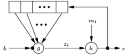
Slika 2.8: Proces šifrovanja samosinhronišućih kriptografskih algoritama, [15]
