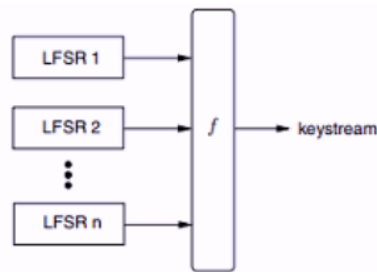
Slika 2.12: Kombinacioni sekvencijalni kriptografski generator, [15]
