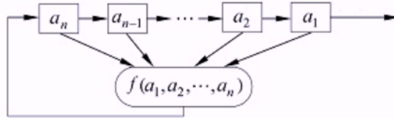
Slika 2.10: Pomerački registar sa povratnom spregom, [15]
