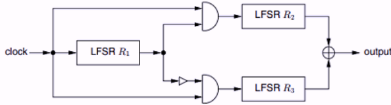
Slika 2.14: Grafički prikaz generatora alternirajućeg takta, [15]
