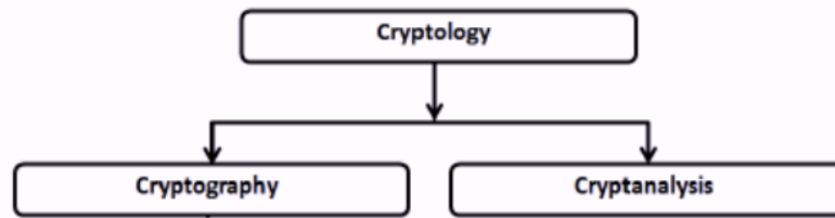
Slika 2.1: Taksonomija kriptologije
