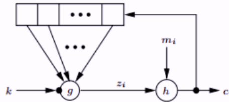
Slika 2.9: Proces dešifrovanja u samosinhronizujućim sekvencijalnim kriptografskim algoritmima, [15]
