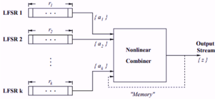
Slika 2.13: Nelinearni kombajner generator sa memorijom
