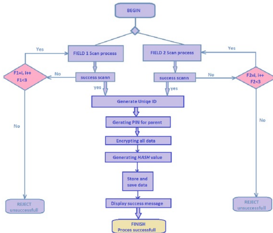
Slika 10 - ALGORITAM ZA AKVIZICIJU PODATAKA
