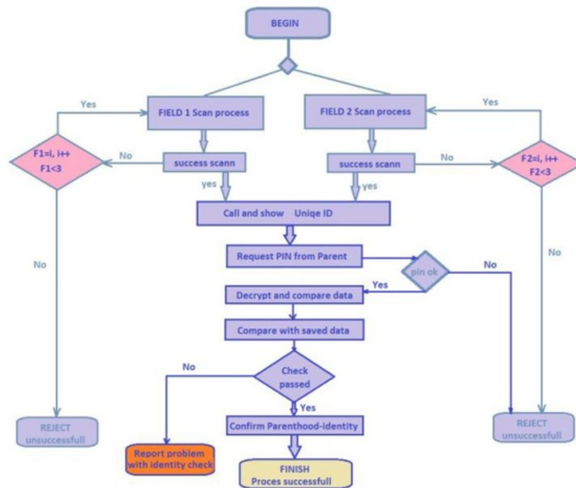
Slika 11 - ALGORITAM ZA VERIFIKACIJU PODATAKA
