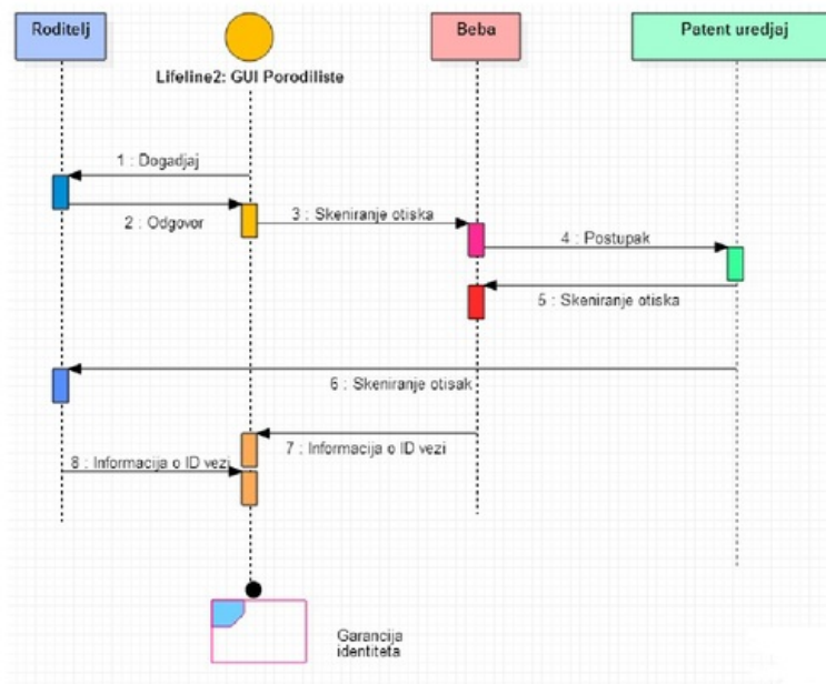
Slika 13 - Dijagram sekvenci
