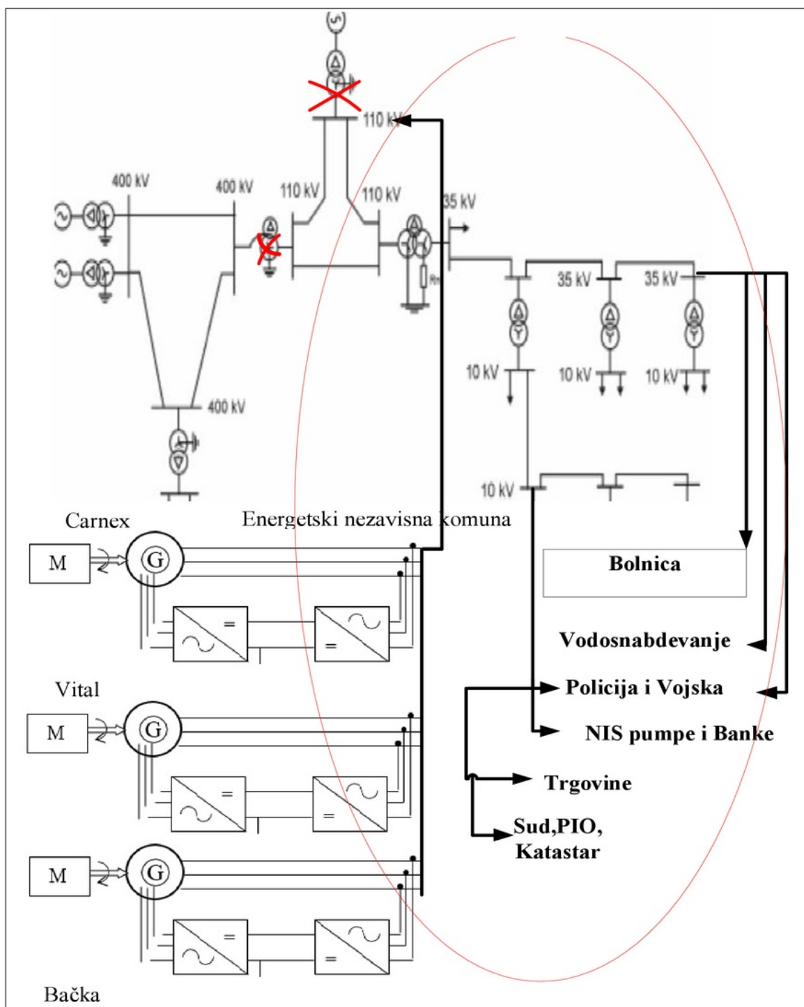
Slika 16/2 Šemtski prikaz stvaranja energetske nezavisne komune u Vrbasu izvor [72]
