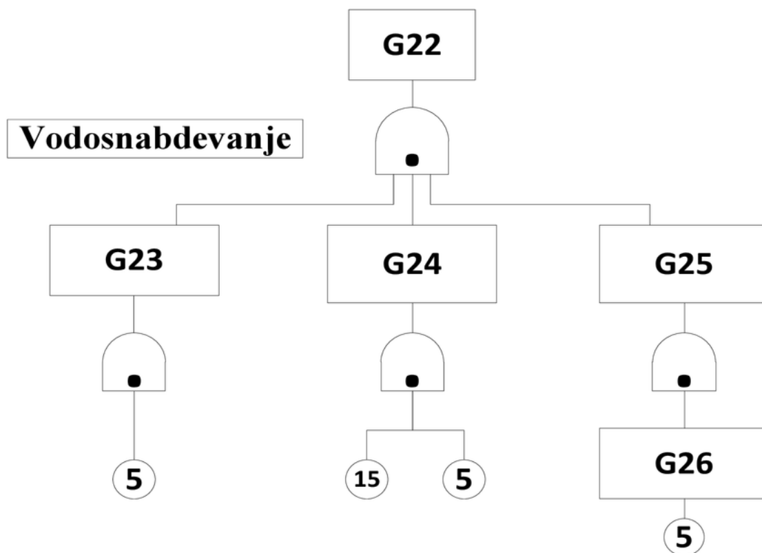
Dijagram 7 Prikaz stabla neispravnosti kolaspa vodosnabdevanja
