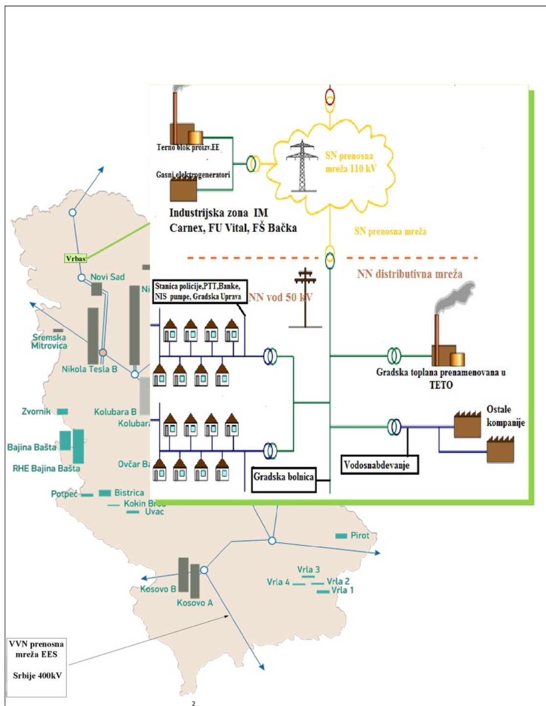
Slika 15/1 Šematski prikaz stvaranja energetski nezavisne komune u Vrbasu izvor [72]
