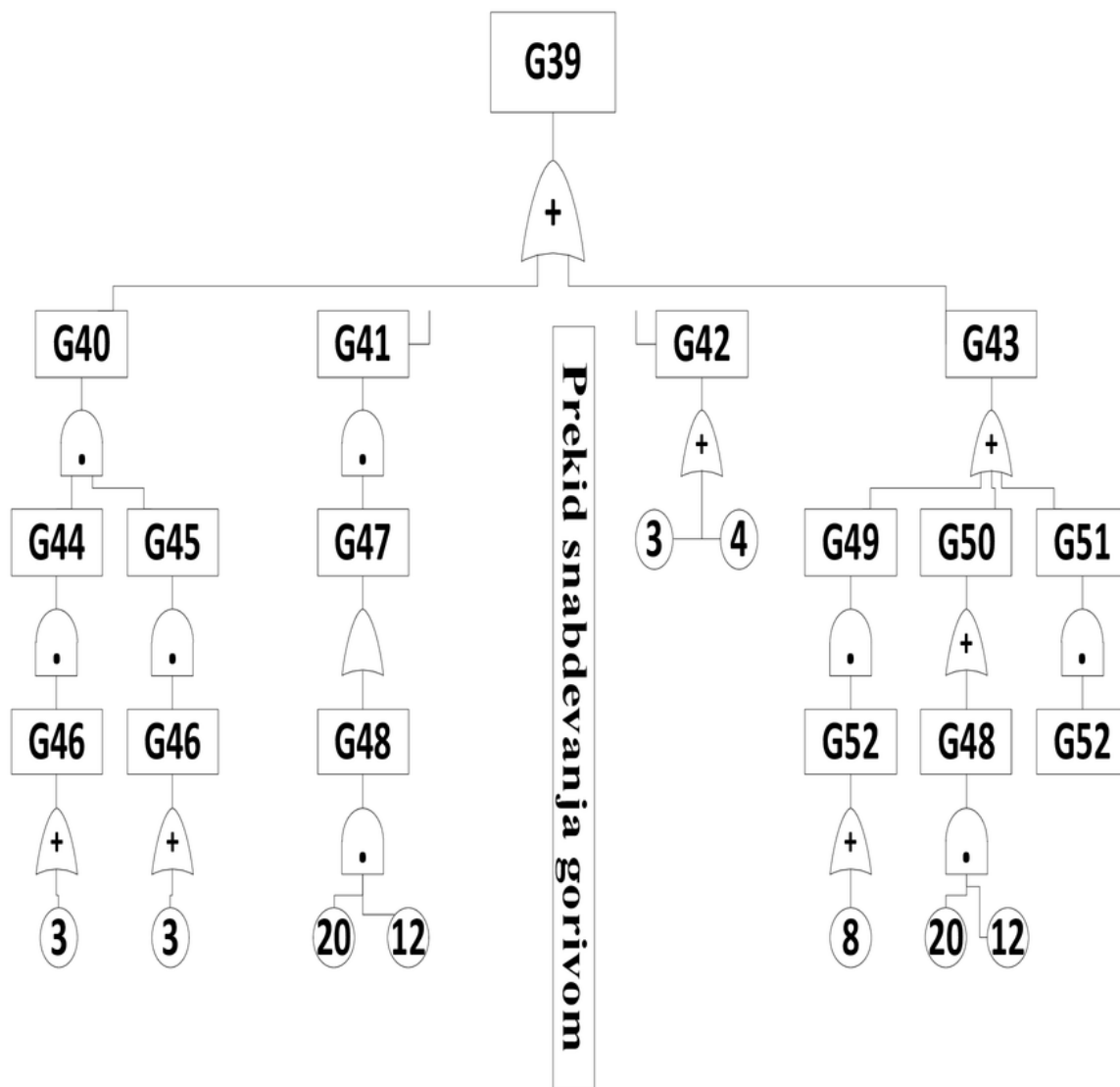
Dijagram 9 Šema otkaza koji dovode do kolapsa snabdevanja gorivom
