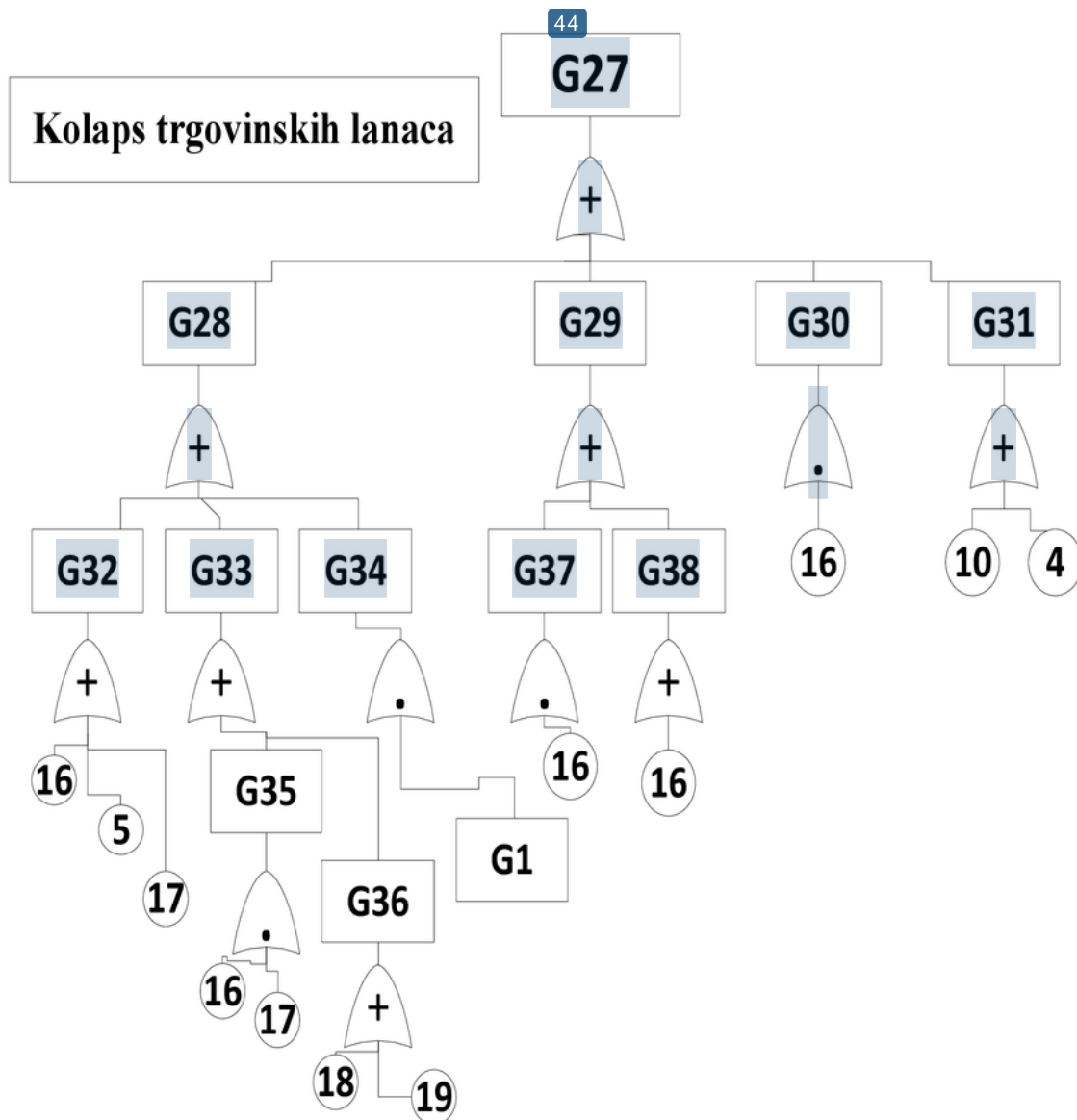
Dijagram 8 Šema otkaza koji dovode do kolapsa kompanija koje se bave snabdevanjem hranom
