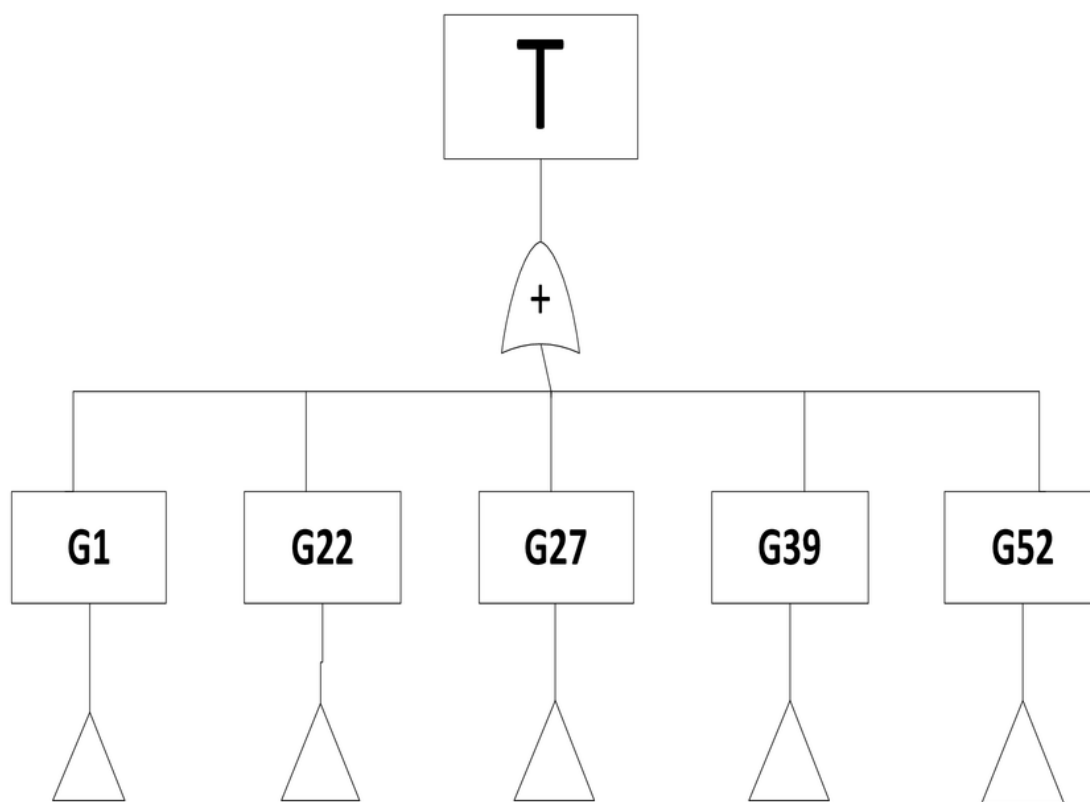
Dijagram 4 Stablo neispravnosti gde je vršni događaj T kolaps EESa i Telekomunikacija
