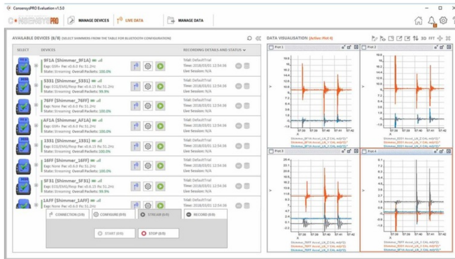
Slika 24. Aplikacija „ConsensysPRO“
