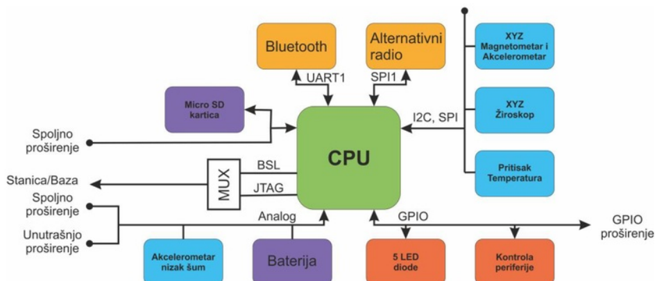
Slika 23. Struktura Shimmer uređaja
