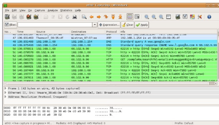
Slika 14. Prikaz uočenih paketa [27]
