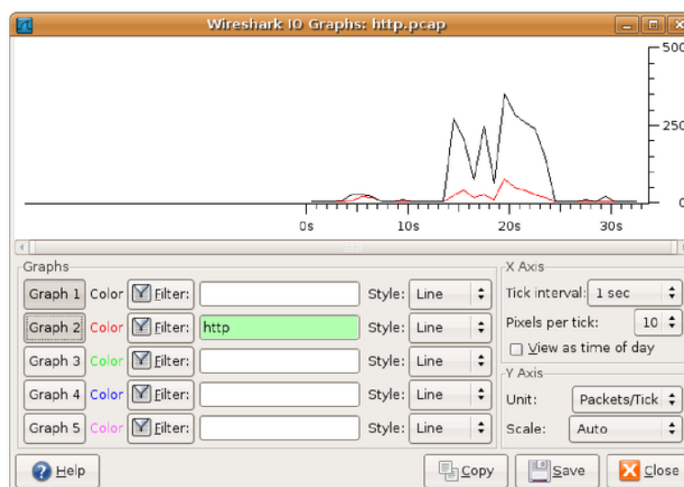
Slika 15. Grafički prikaz sumiranog prometa [27]
