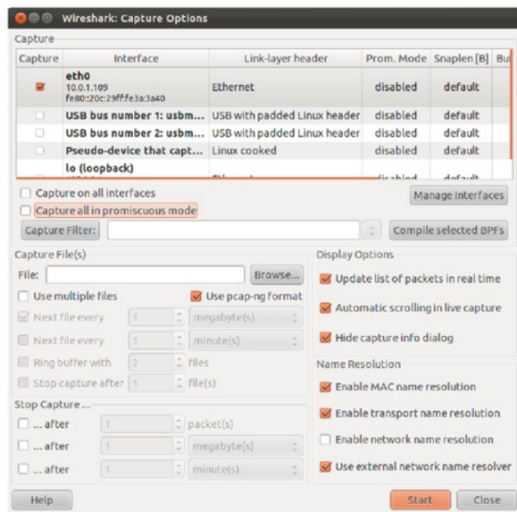
Slika 13. Prikaz mogućnosti uočenja [27]
