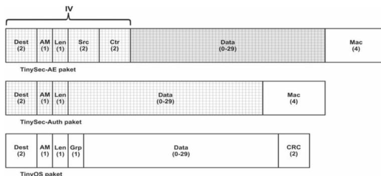
Slika 12. Formati poruka
