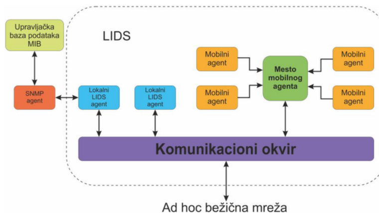
Slika 11. LIDS arhitektura
