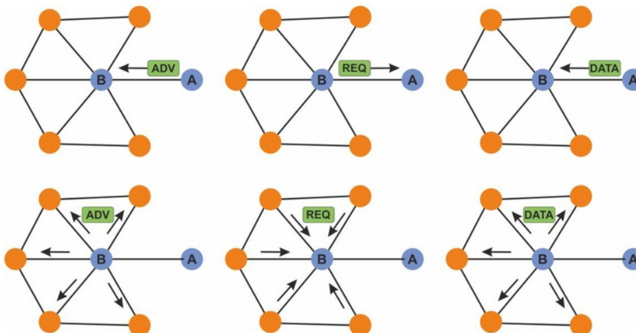
Slika 8. SPIN protokol
