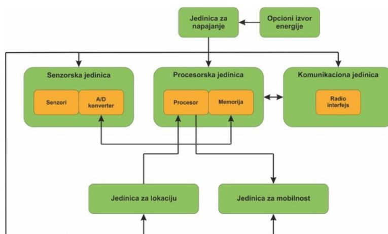
Slika 5. Struktura senzorskog čvora
