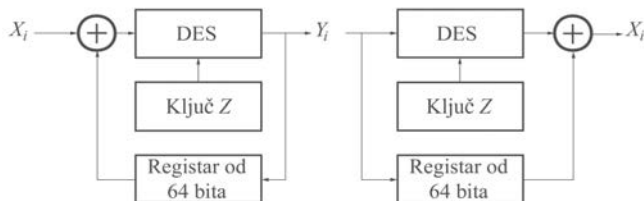
Slika 5.3.5. Način rada blok-šifre u kome se ulančavaju blokovi šifrata
