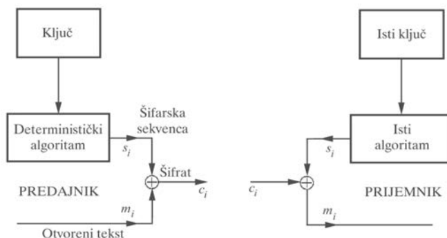
Slika 5.3.1. Principna šema sekvencijalnog šifarskog sistema
