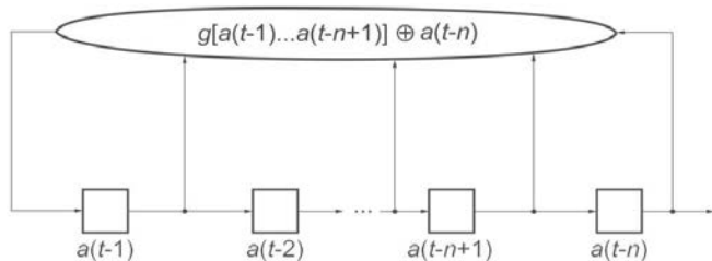
Slika 5.3.2. Pomerački registar sa povratnom spregom
