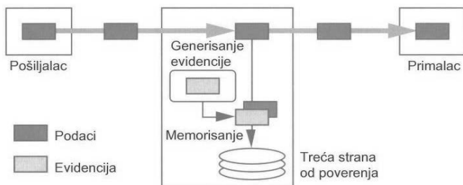
Slika 10.6.4. Neporecivost porekla sa trećom stranom od poverenja na komunikacionom putu – evidencija se skladišti
