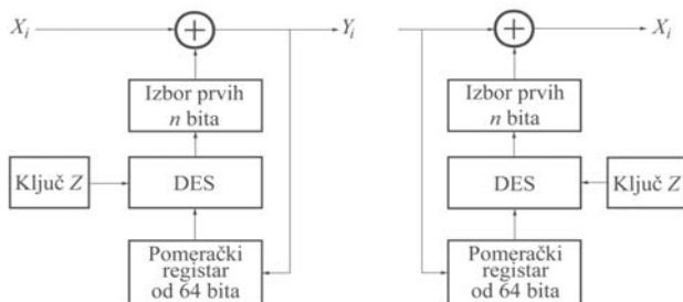
Slika 5.3.6. Način rada blok-šifre sa šifratom u povratnoj sprezi
