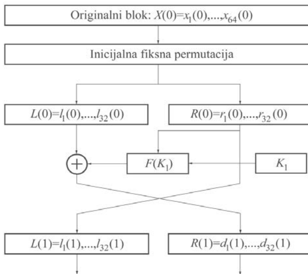
Slika 5.3.3. Inicijalna transformacija i prva runda DES-a
