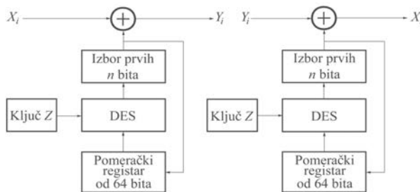
Slika 5.3.7. Način rada blok-šifre sa izlaznim nizom u povratnoj sprezi.
