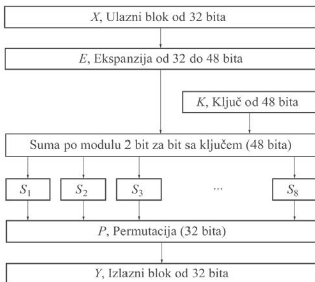
Slika 5.3.4. Struktura funkcije F u DES-u
