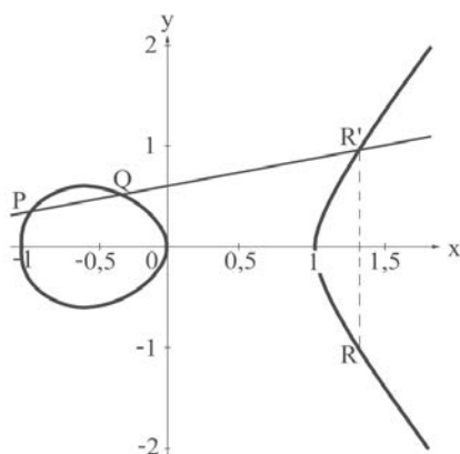
Slika 5.3.8. Eliptička kriva
