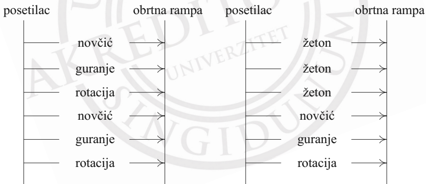
Slika 3.4 Model obrtna rampe predstavljen tragovima događaja
