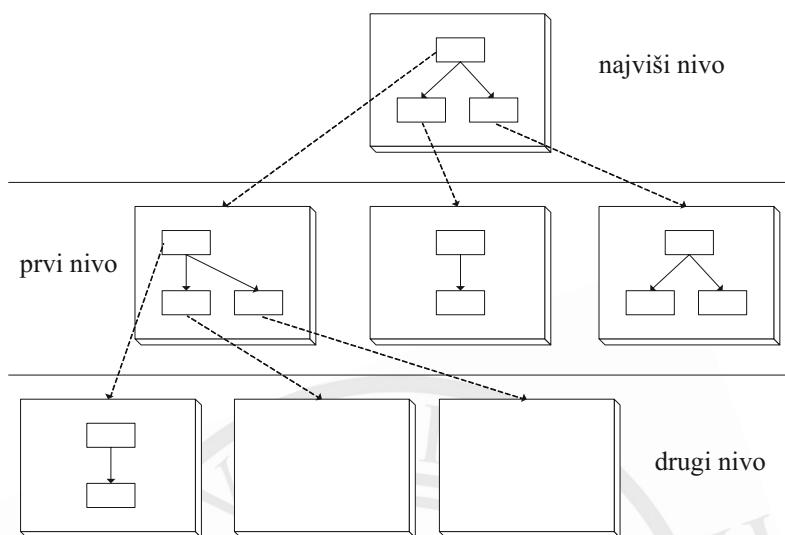
Slika 4.2 Nivoi modularnosti
