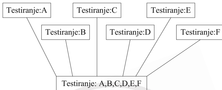
Slika 7.6 Testiranje po principu „velikog praska“
