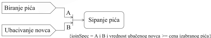
Slika 5.16 Primer specifikacije spajanja
