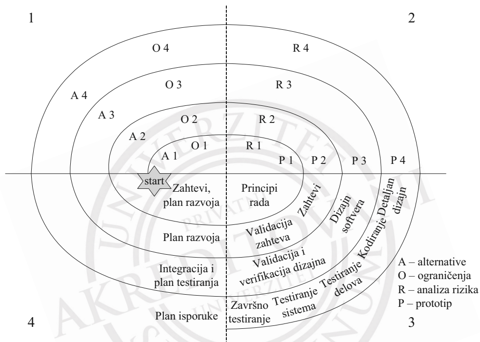
Slika 2.8 Spiralni model
