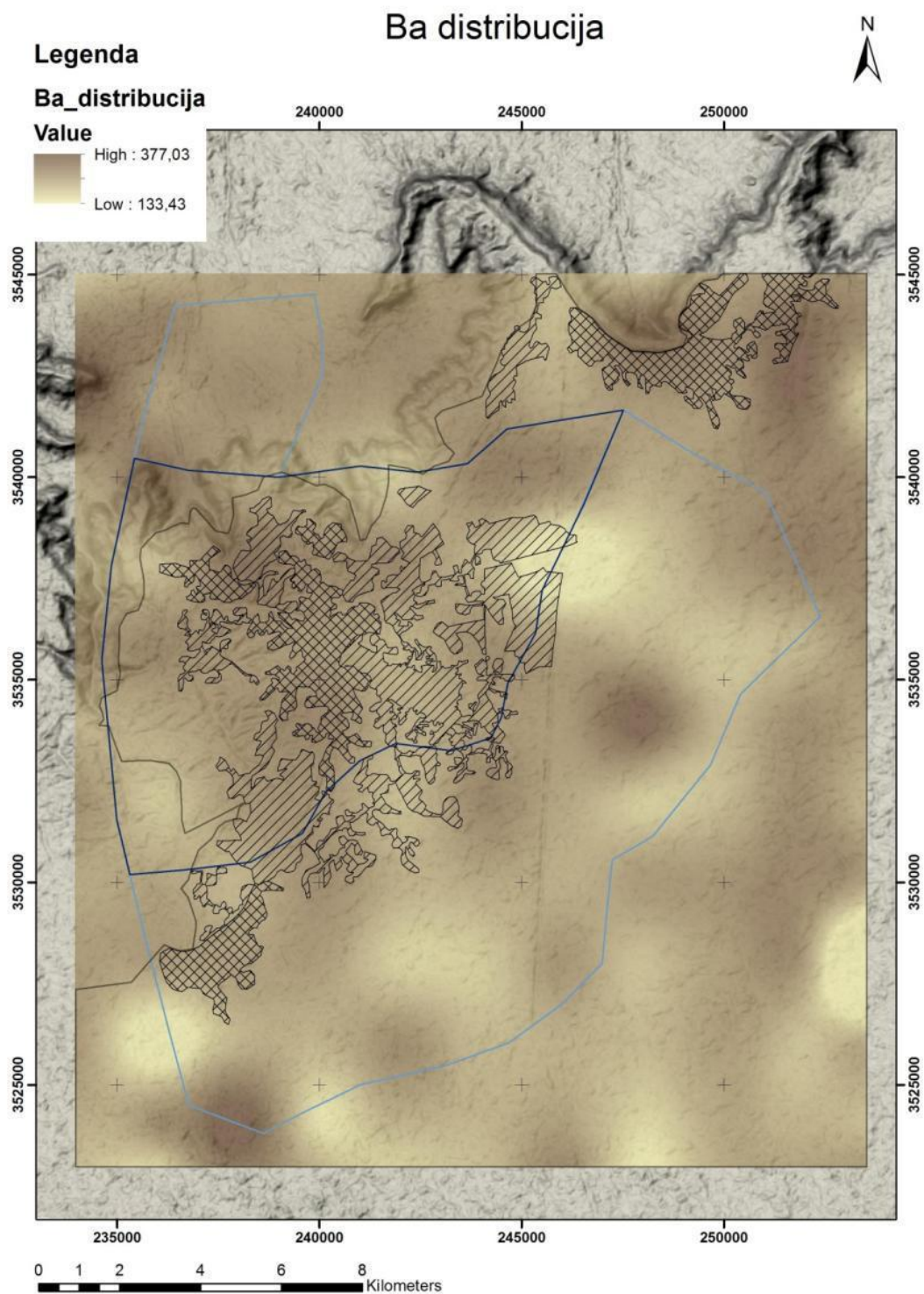
Slika 8.26: Interpolacija distribucija Ba srazmerno izmerenim sadržajima
