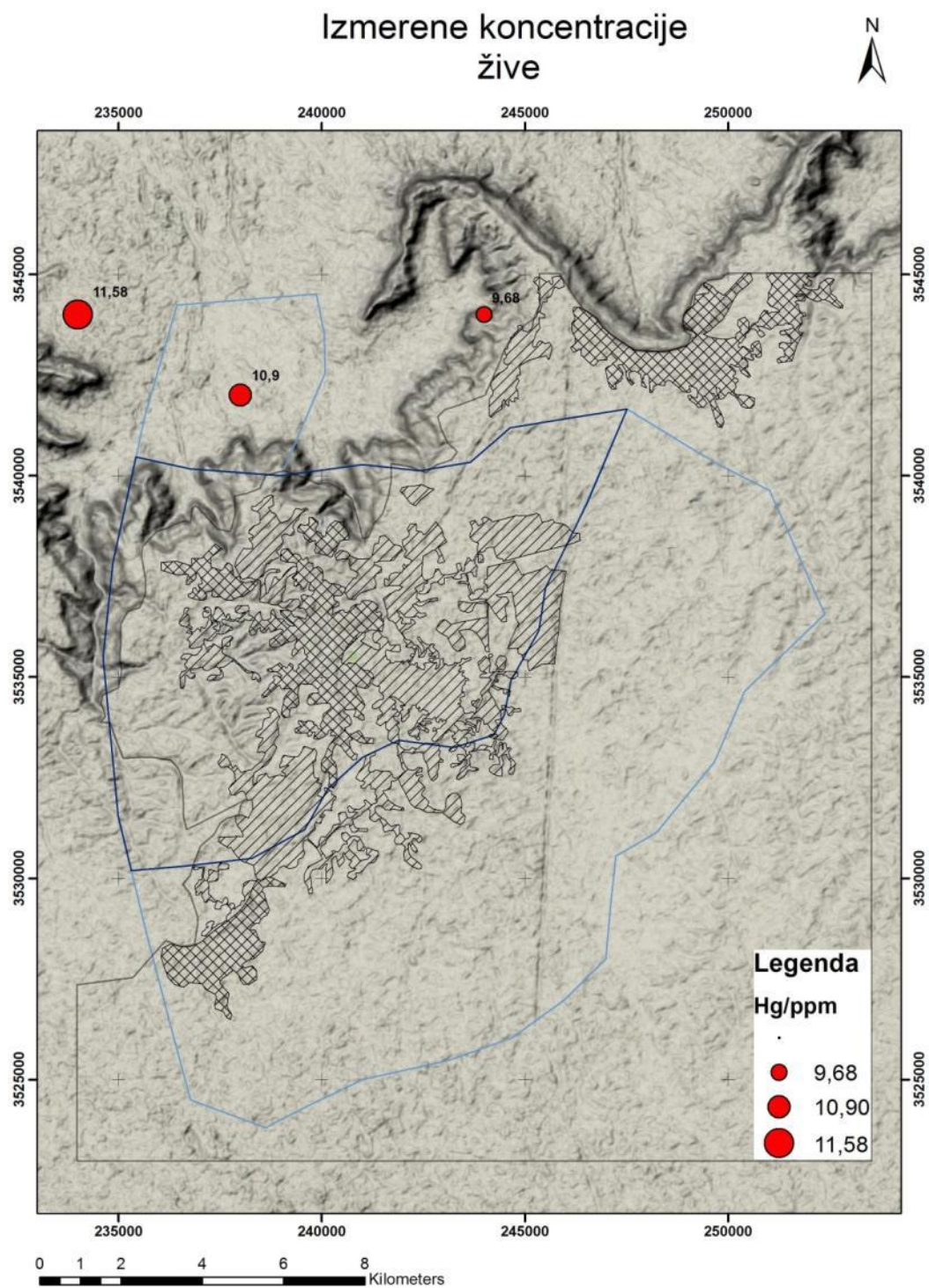
Slika 8.23: Tačkasta distribucija Hg srazmerno izmerenim sadržajima
