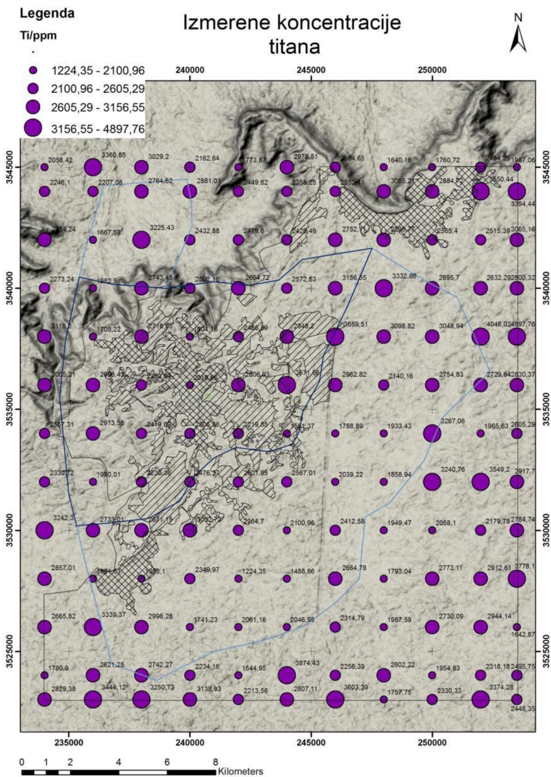
Slika 8.7: Tačkasta distribucija Ti srazmerno izmerenim sadržajima
