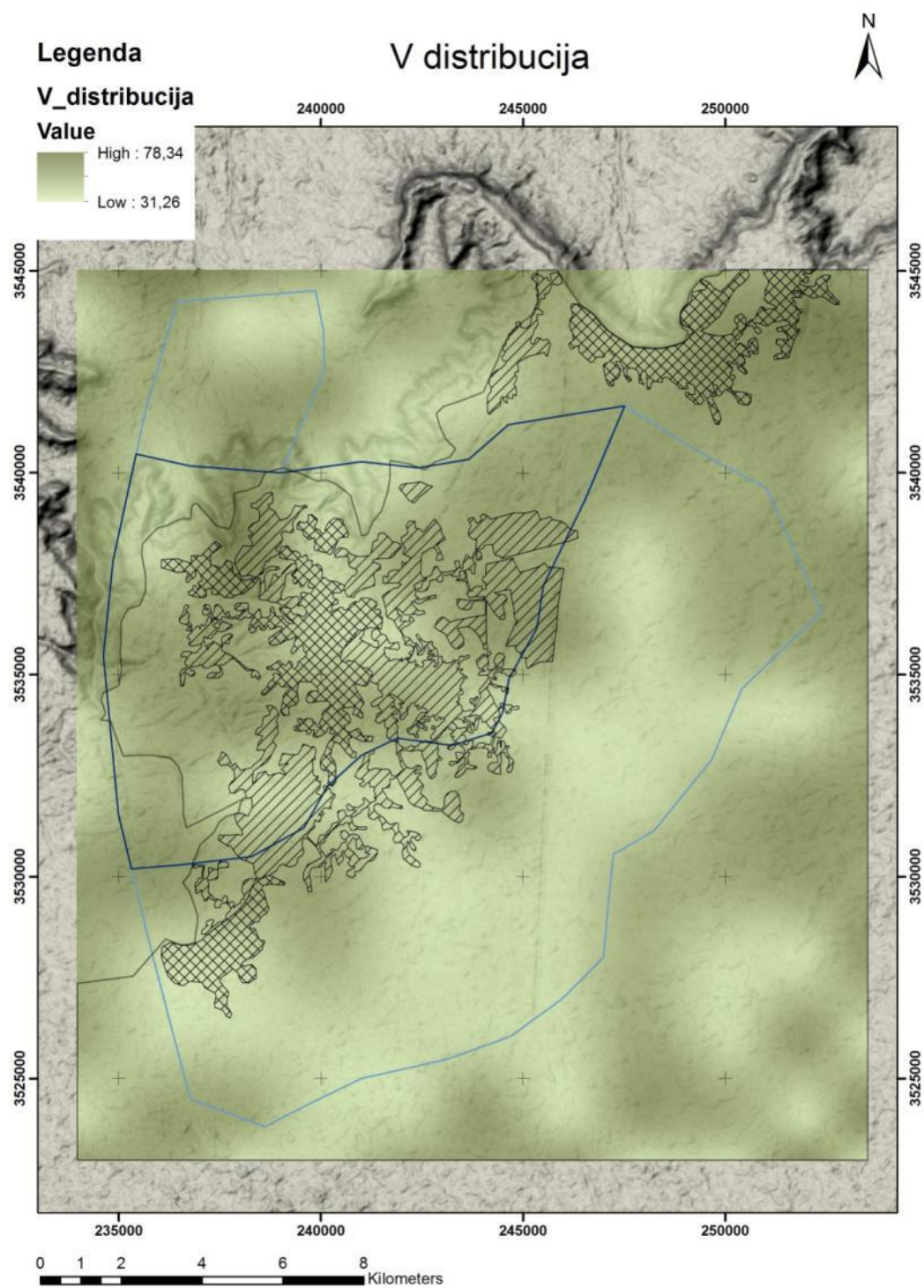
Slika 8.6: Interpolacija distribucija V srazmerno izmerenim sadržajima
