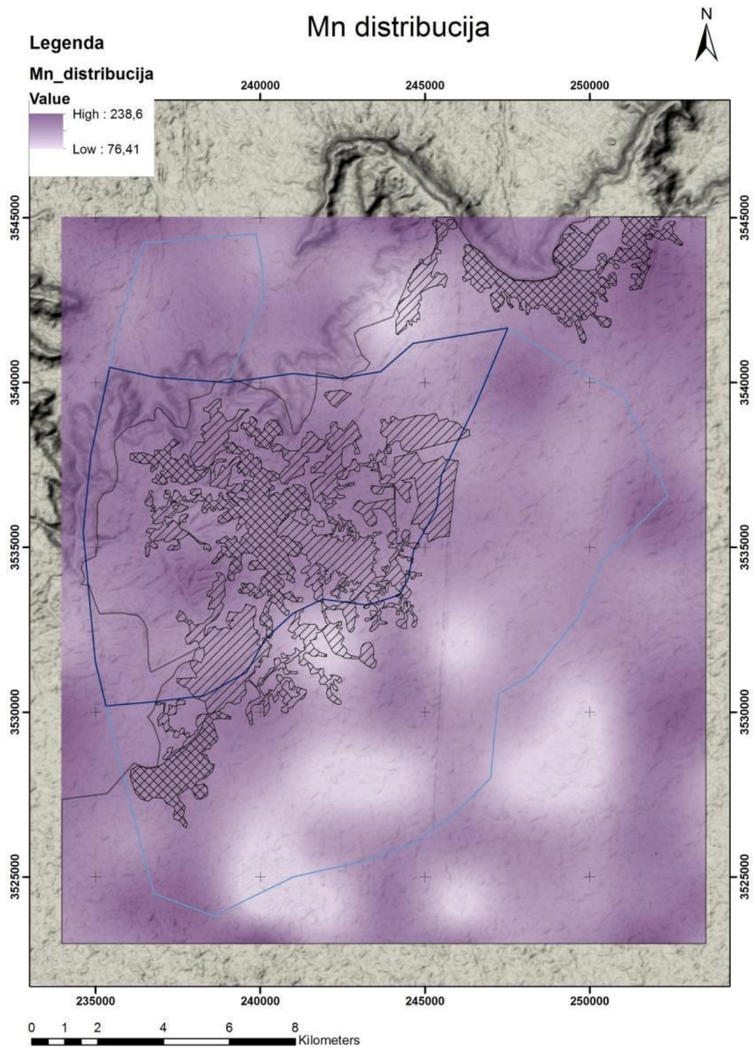
Slika 8.16: Interpolacija distribucija Mn srazmerno izmerenim sadržajima
