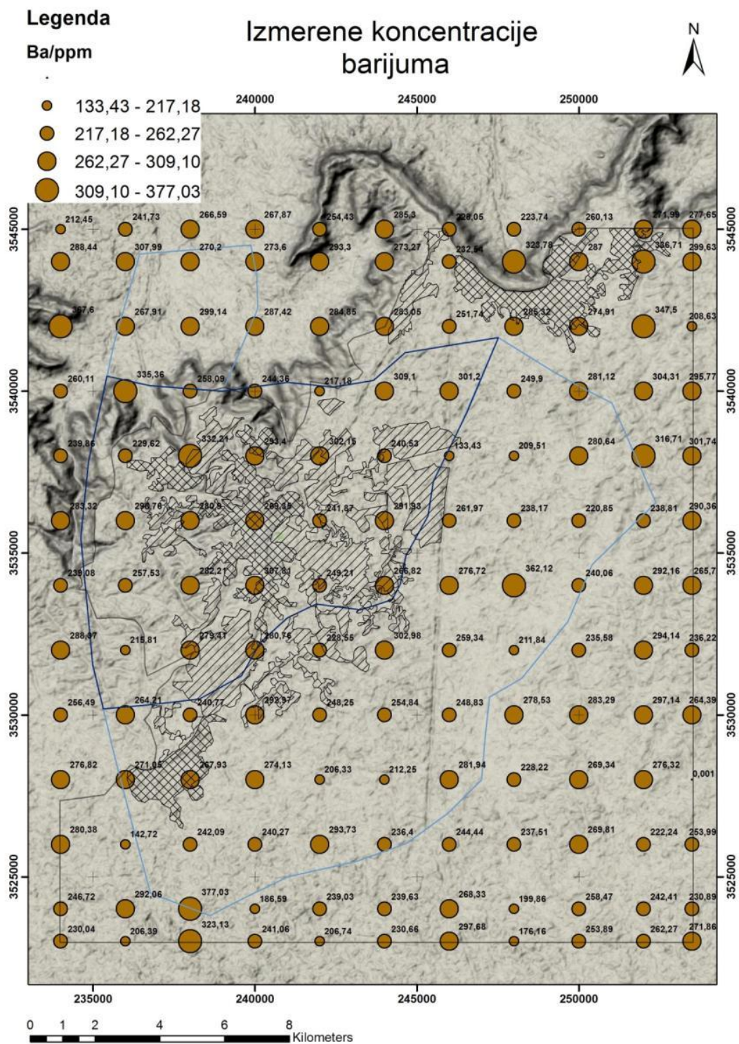
Slika 8.25: Tačkasta distribucija Ba srazmerno izmerenim sadržajima
