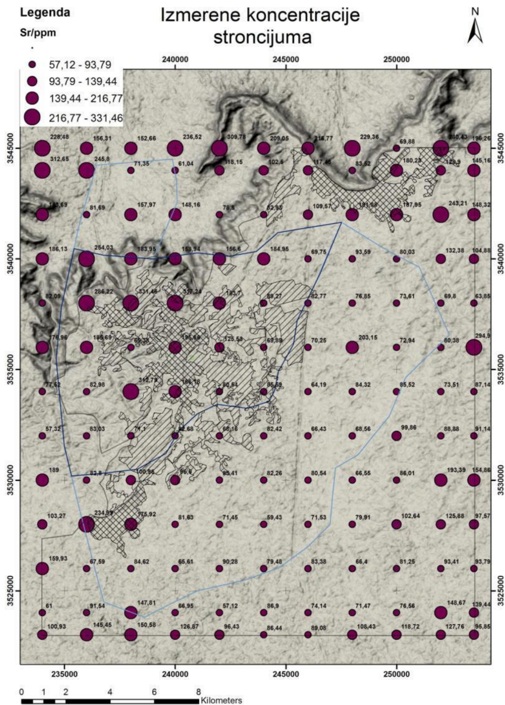
Slika 8.29: Tačkasta distribucija Sr srazmerno izmerenim sadržajima
