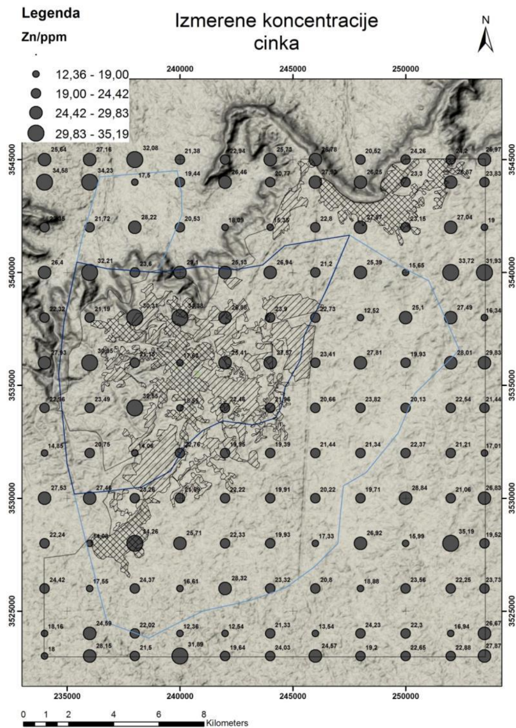
Slika 8.13: Tačkasta distribucija Zn srazmerno izmerenim sadržajima
