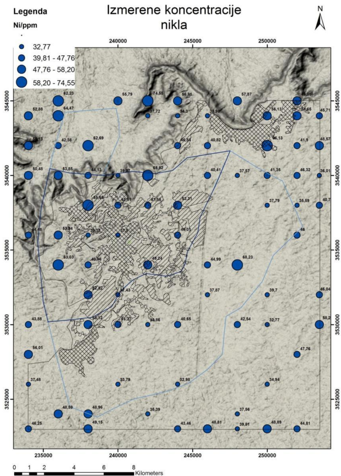
Slika 8.3: Tačkasta distribucija Ni srazmerno izmerenim sadržajima
