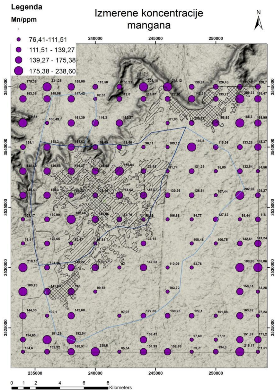
Slika 8.15: Tačkasta distribucija Mn srazmerno izmerenim sadržajima
