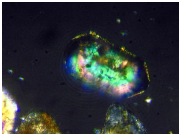
Slika 4.24: Mikroskopski snimak uzorka Zn136 - cirkon
