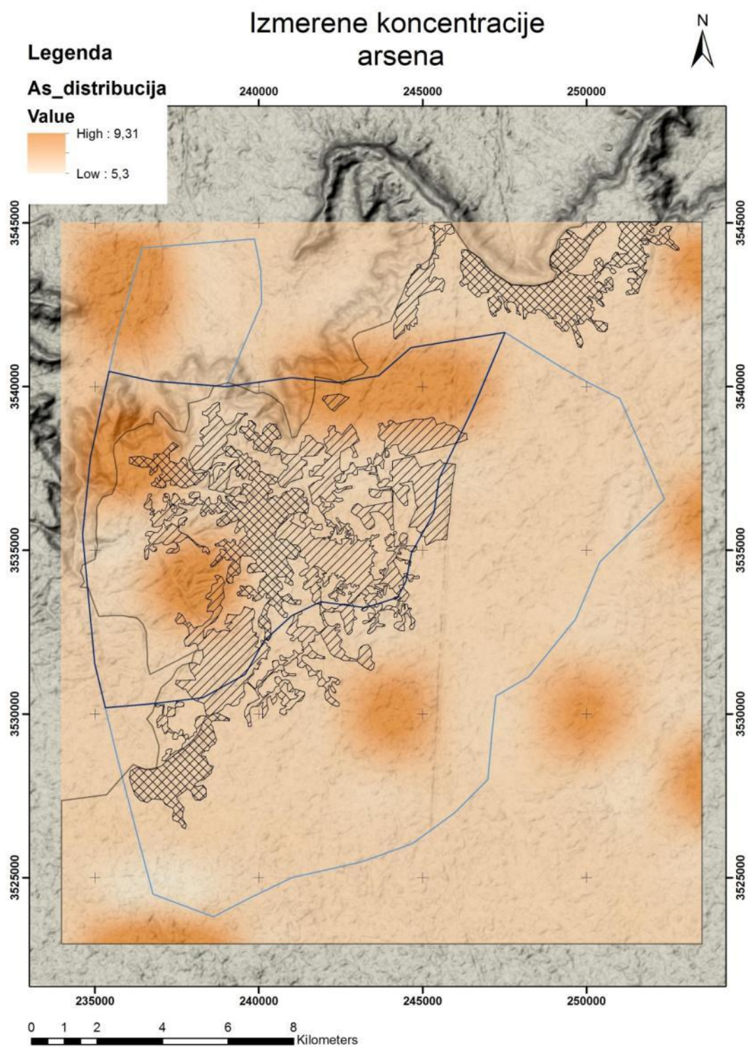
Slika 8.22: Interpolacija distribucija As srazmerno izmerenim sadržajima
