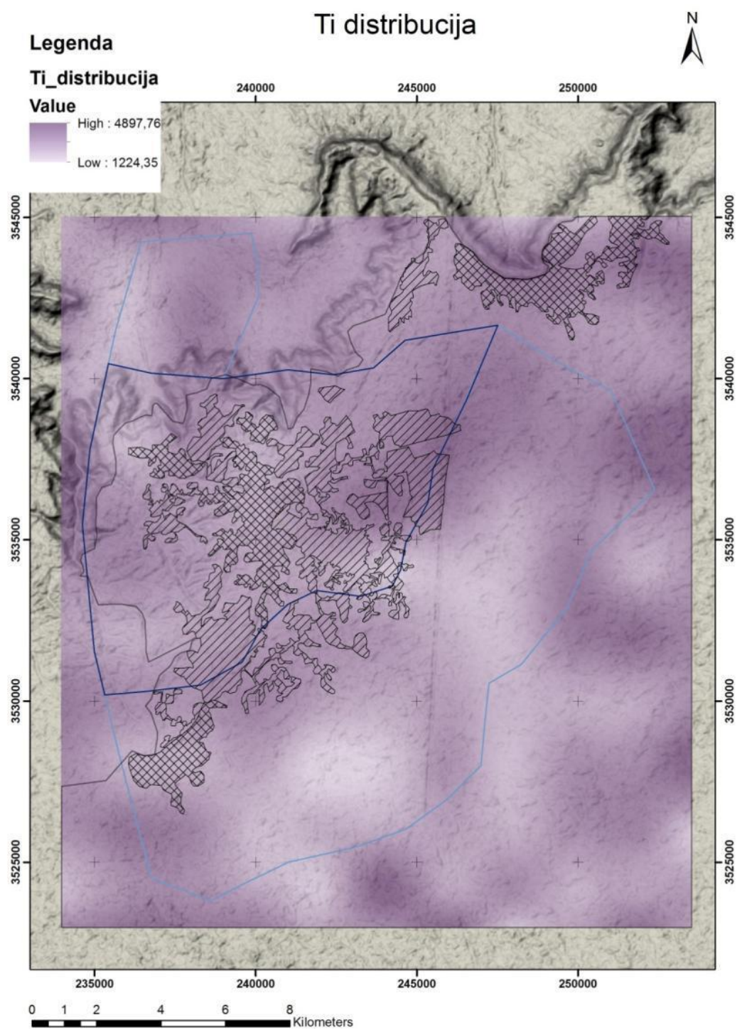
Slika 8.8: Interpolacija distribucija Ti srazmerno izmerenim sadržajima
