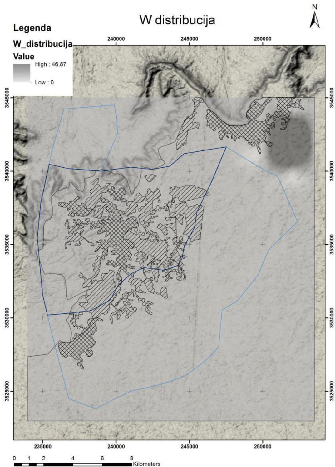
Slika 8.38: Interpolacija distribucija W srazmerno izmerenim sadržajima
