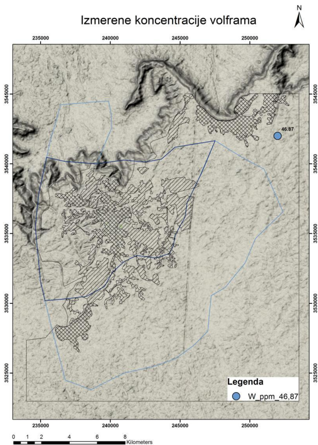
Slika 8.37: Tačkasta distribucija W srazmerno izmerenim sadržajima
