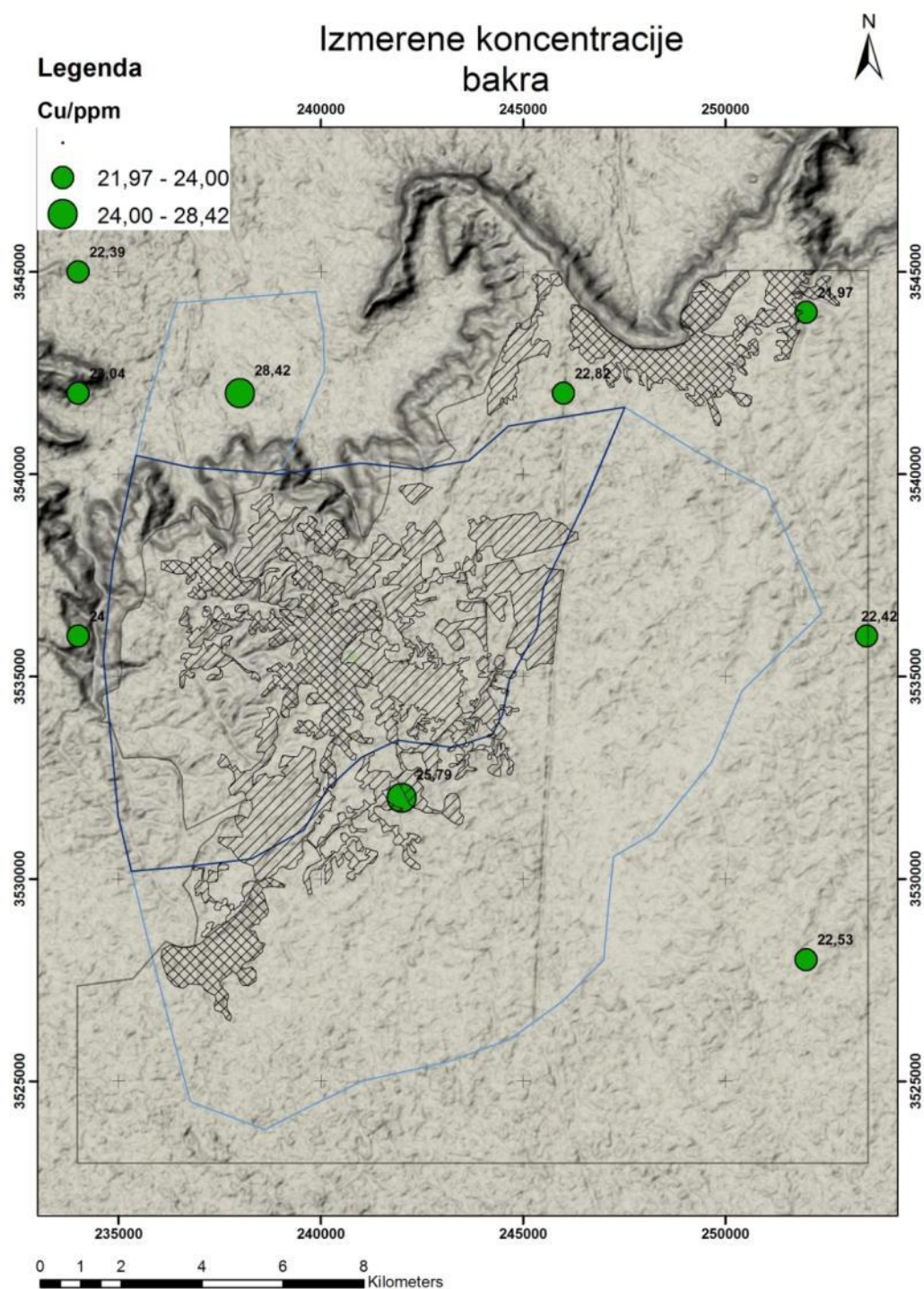
Slika 8.9: Tačkasta distribucija Cu srazmerno izmerenim sadržajima
