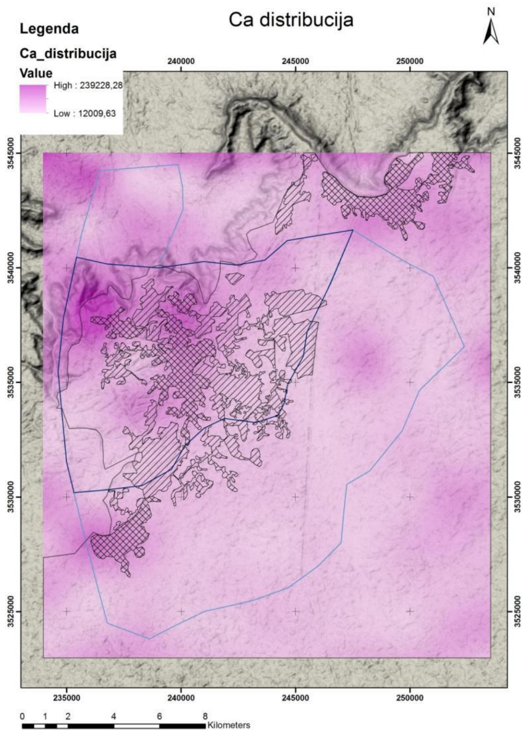
Slika 8.28: Interpolacija distribucija Ca srazmerno izmerenim sadržajima
