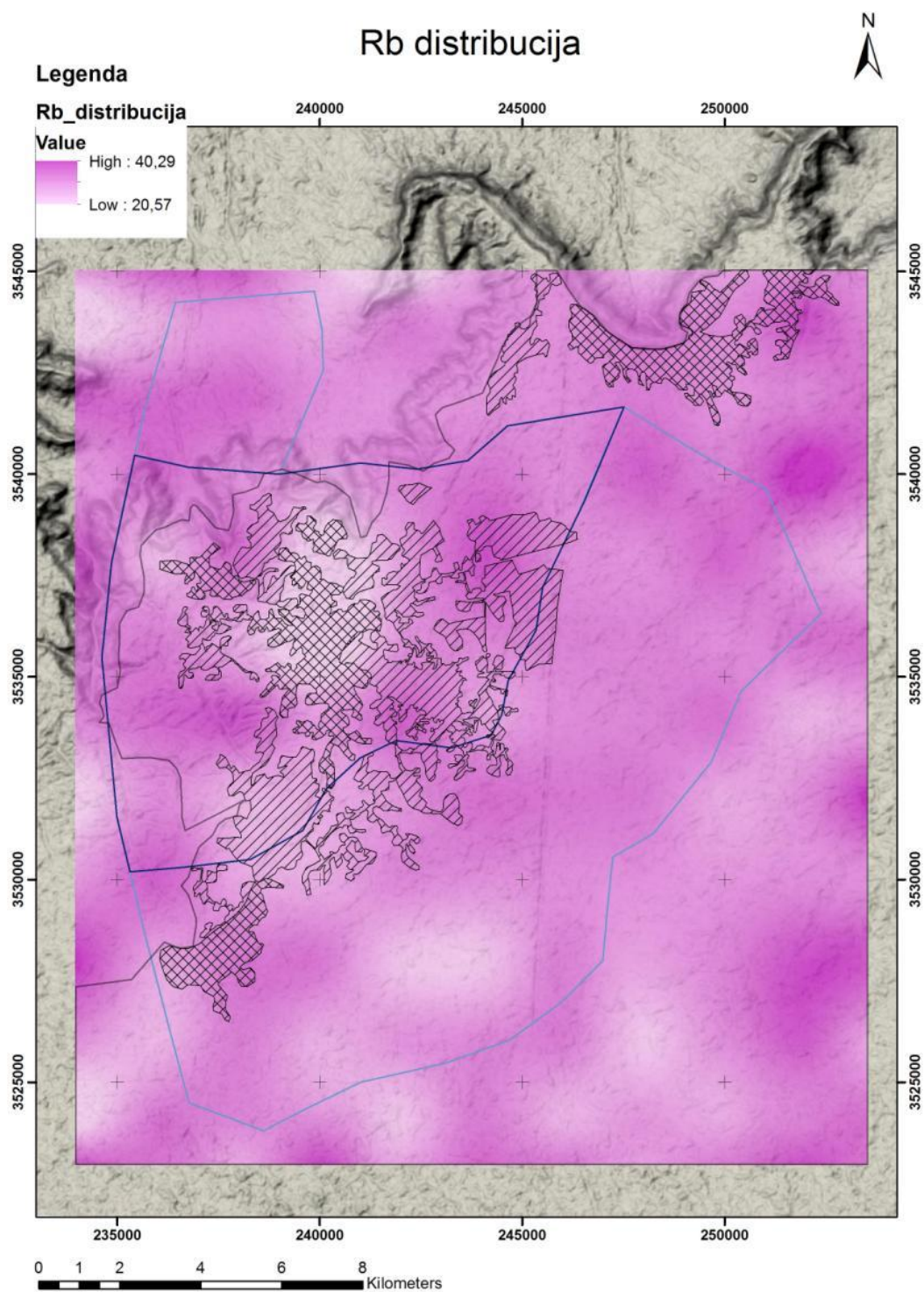
Slika 8.34: Interpolacija distribucija Rb srazmerno izmerenim sadržajima
