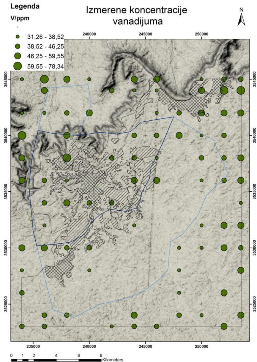
Slika 8.5: Tačkasta distribucija V srazmerno izmerenim sadržajima
