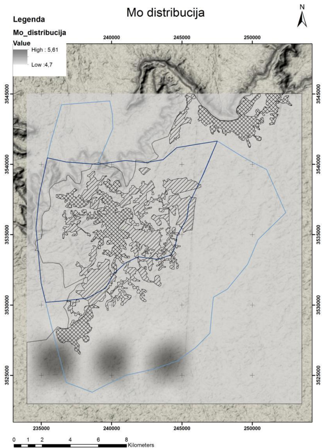
Slika 8.36: Interpolacija distribucija Mo srazmerno izmerenim sadržajima
