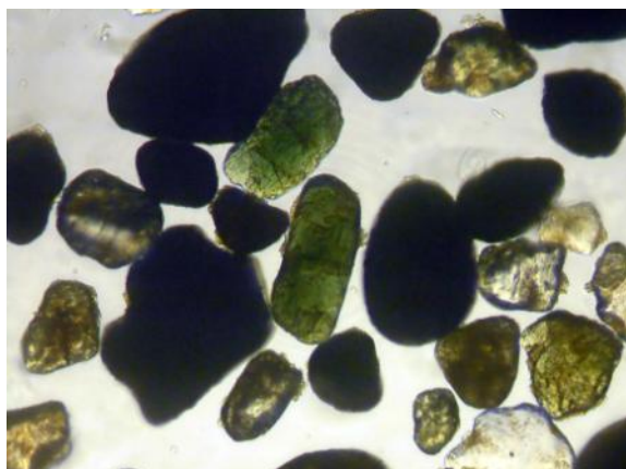
Slika 4.12: Mikroskopski snimak uzorka Zn059, teške frakcije
