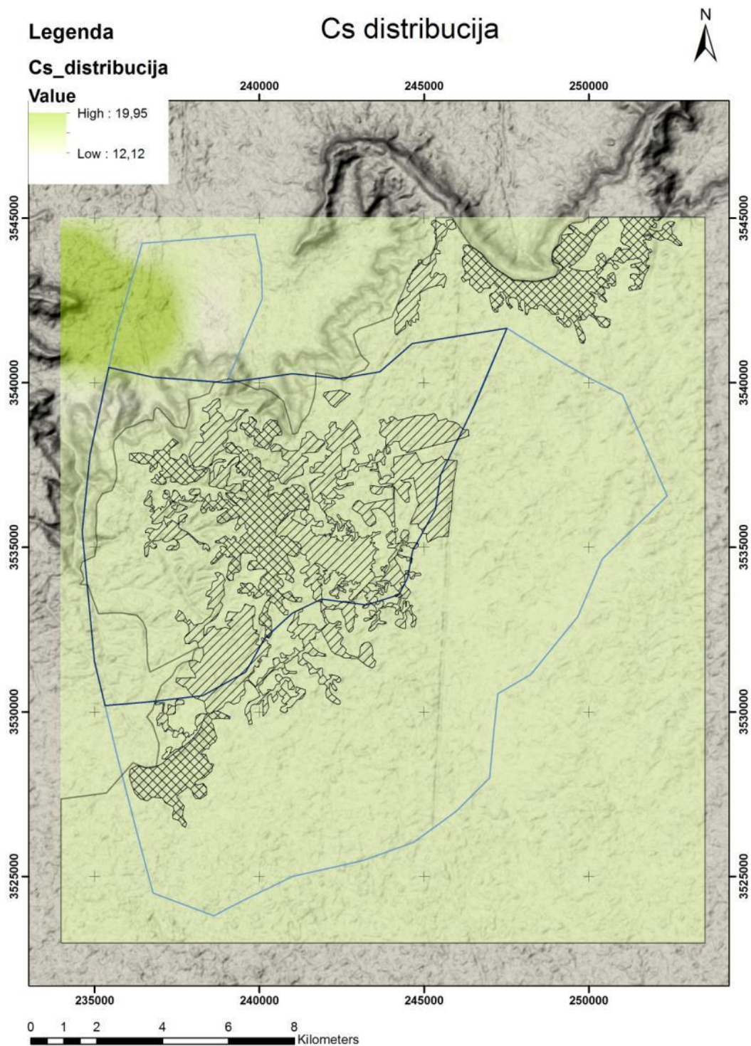
Slika 8.32: Interpolacija distribucija Cs srazmerno izmerenim sadržajima
