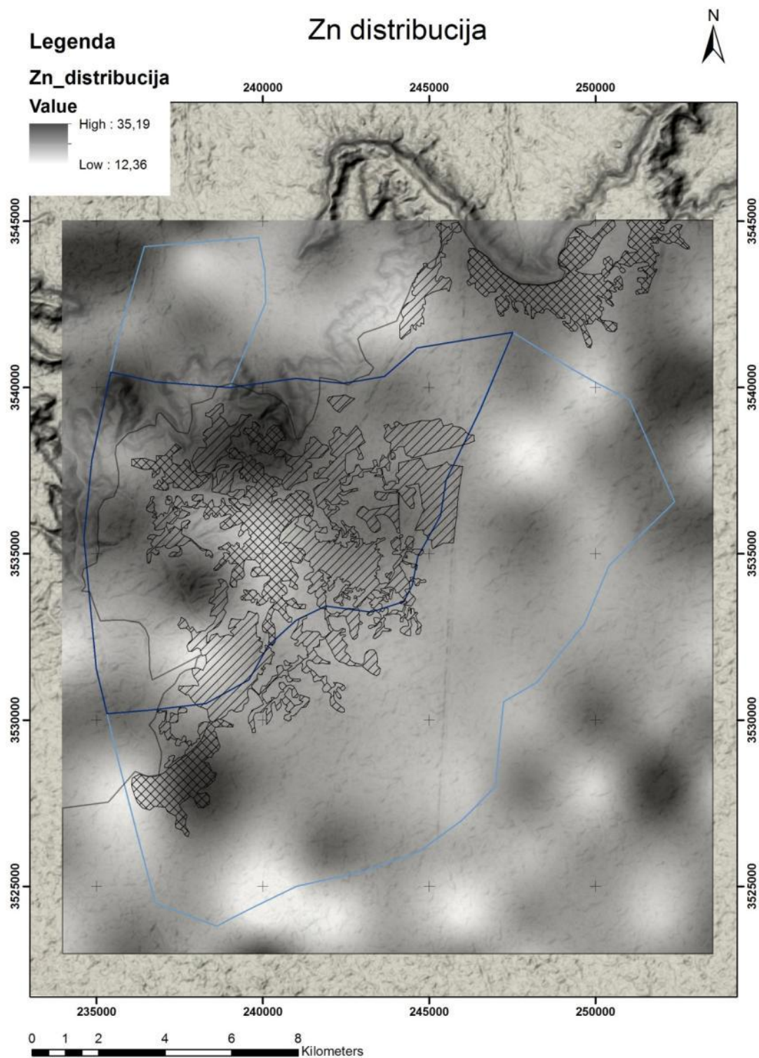
Slika 8.14: Interpolacija distribucija Zn srazmerno izmerenim sadržajima
