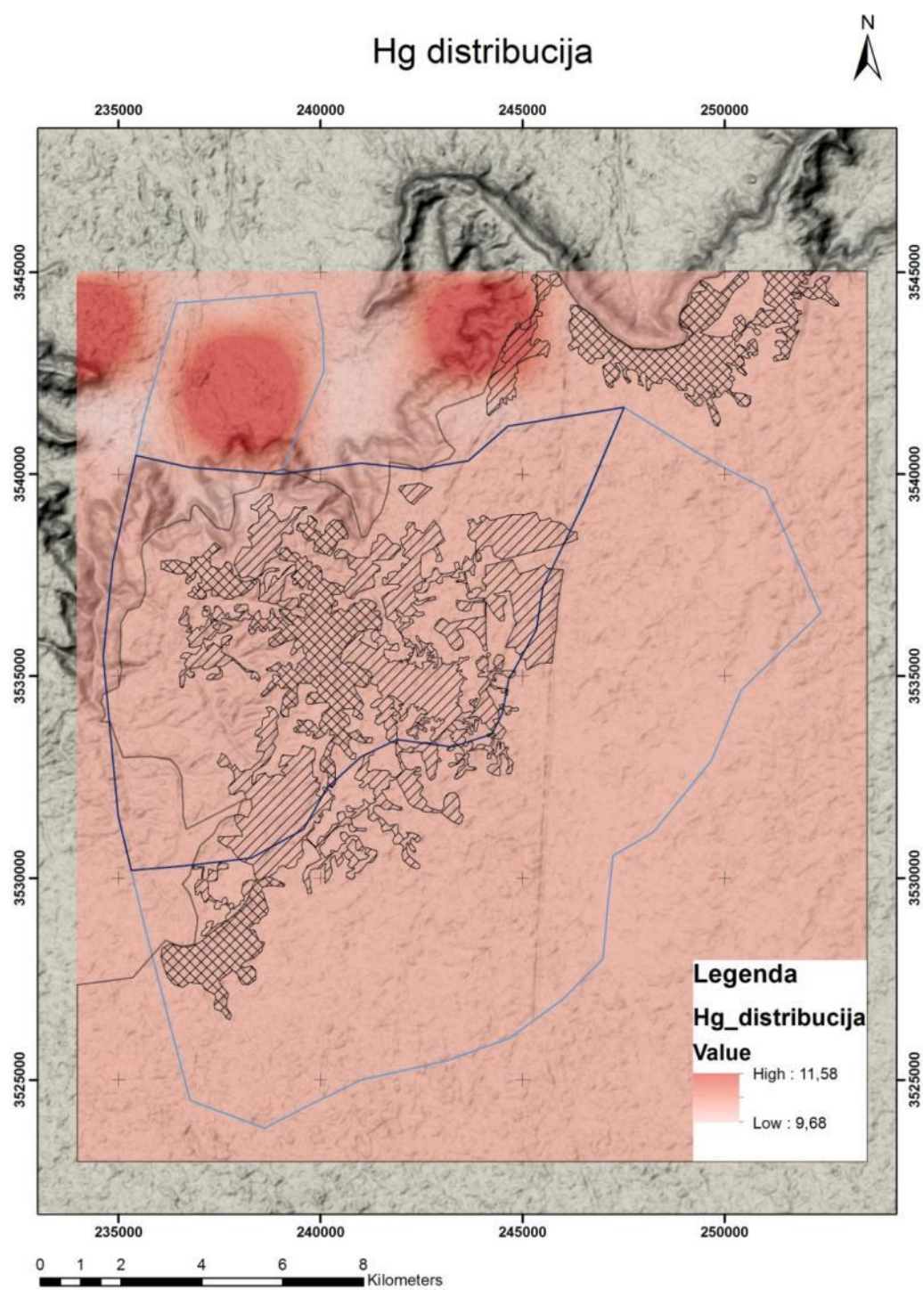
Slika 8.24: Interpolacija distribucija Hg srazmerno izmerenim sadržajima
