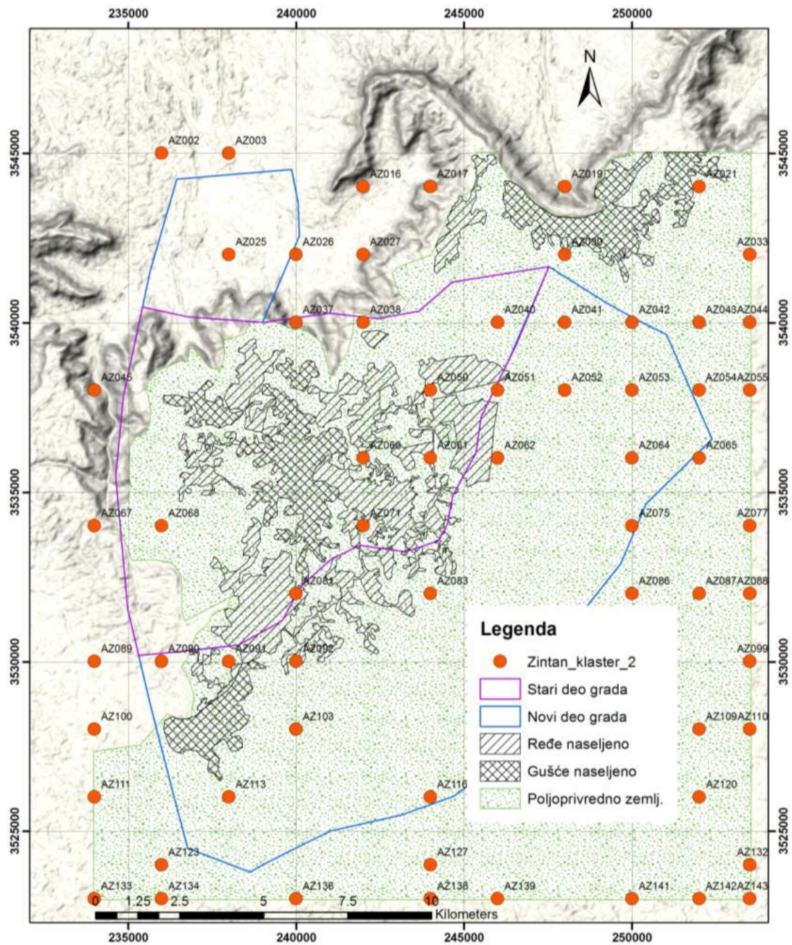
Slika 10.5: Prostorna distribucija uzoraka iz Klastera 2
