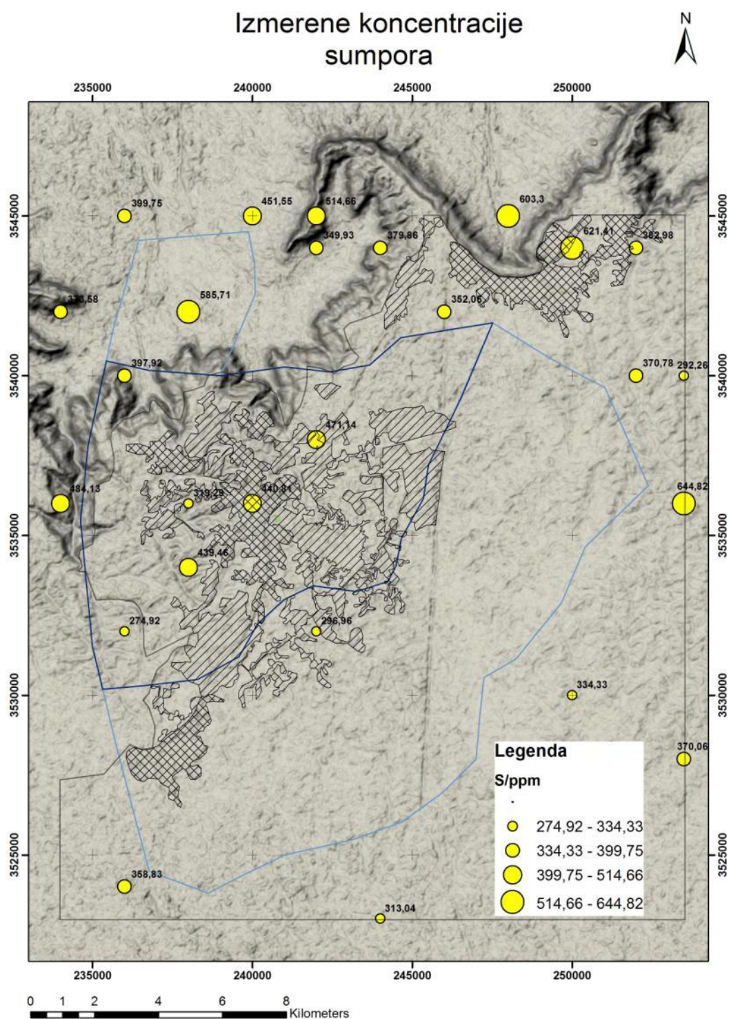
Slika 8.19: Tačkasta distribucija S srazmerno izmerenim sadržajima
