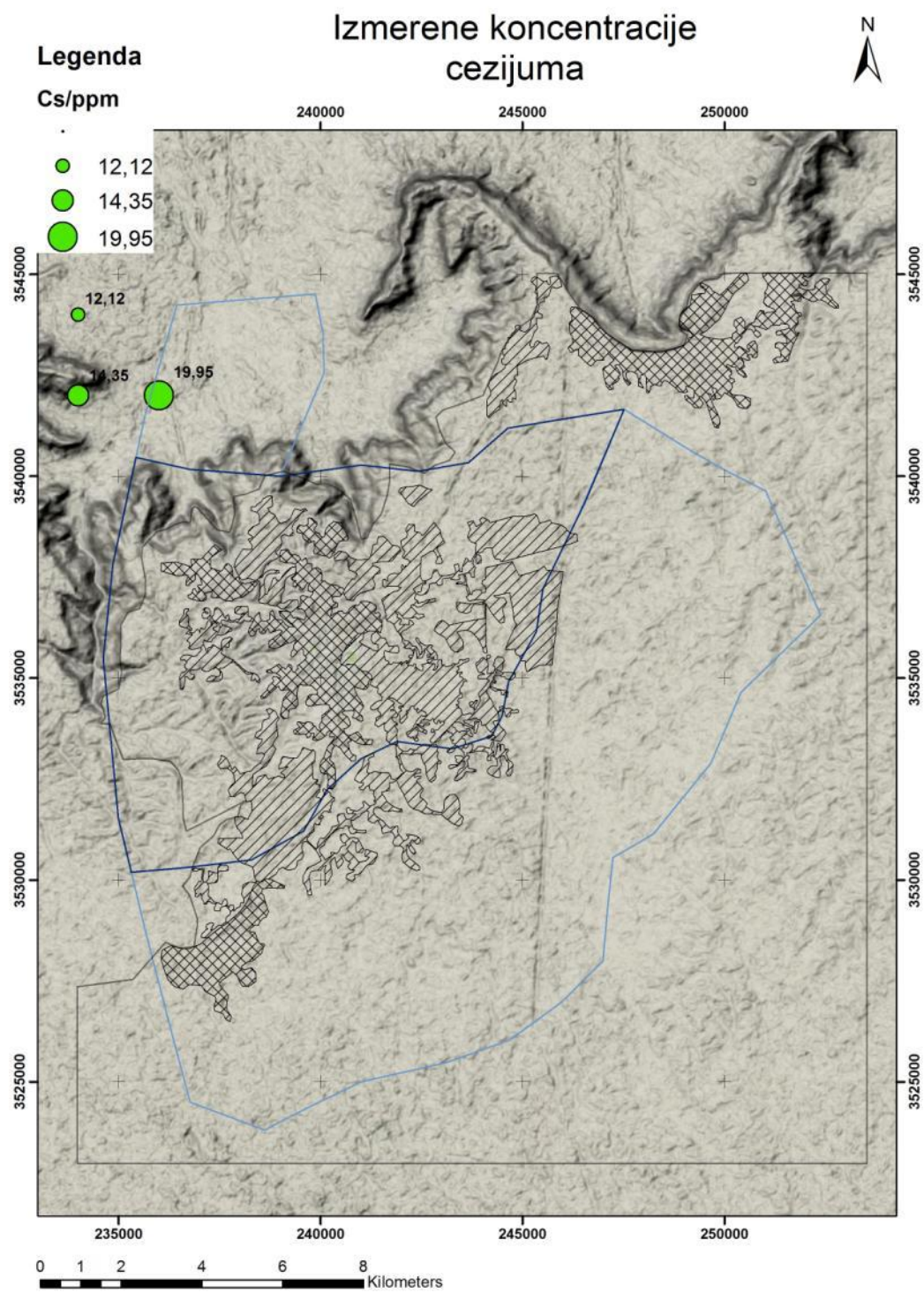
Slika 8.31: Tačkasta distribucija Cs srazmerno izmerenim sadržajima
