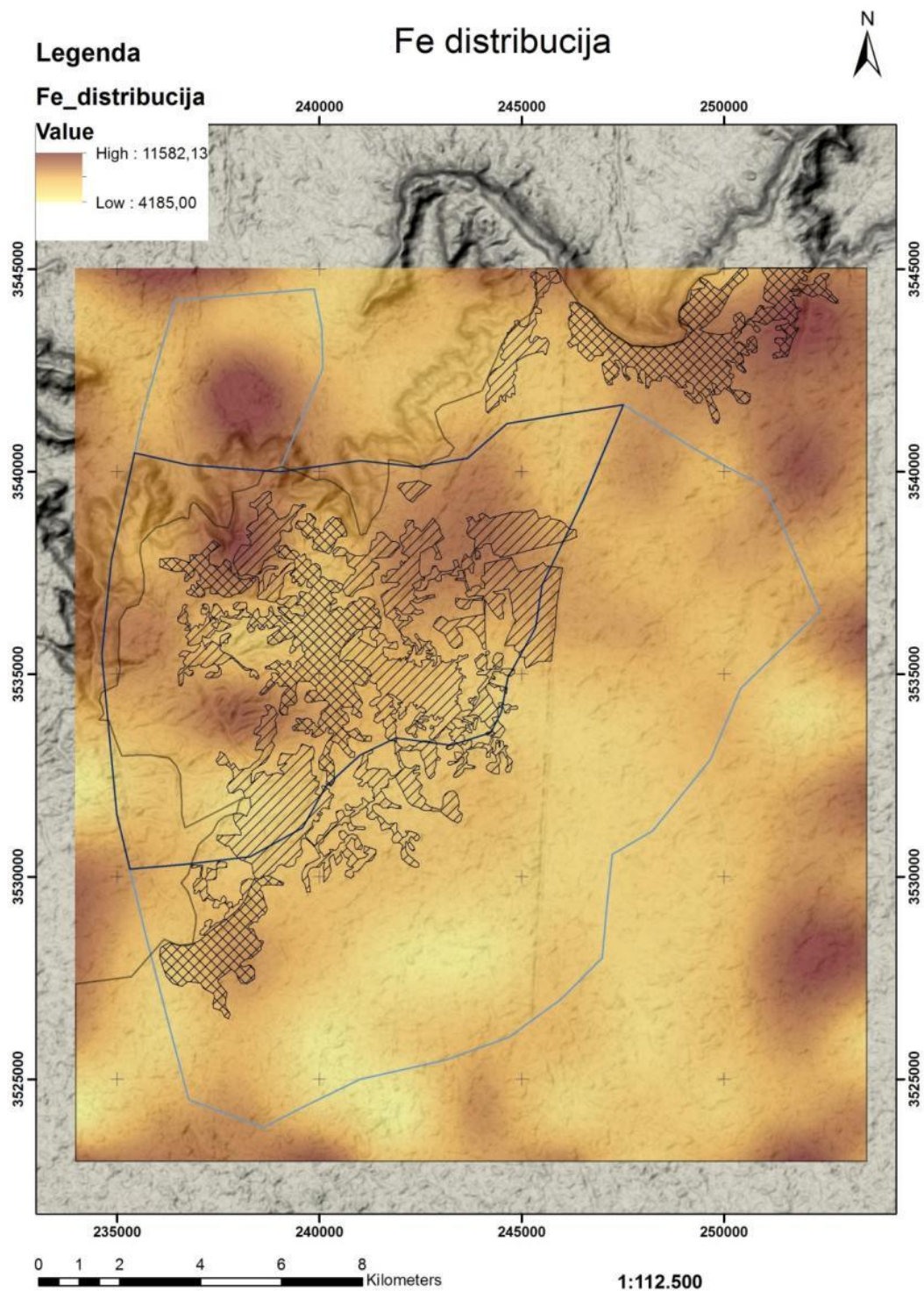
Slika 8.18: Interpolacija distribucija Fe srazmerno izmerenim sadržajima
