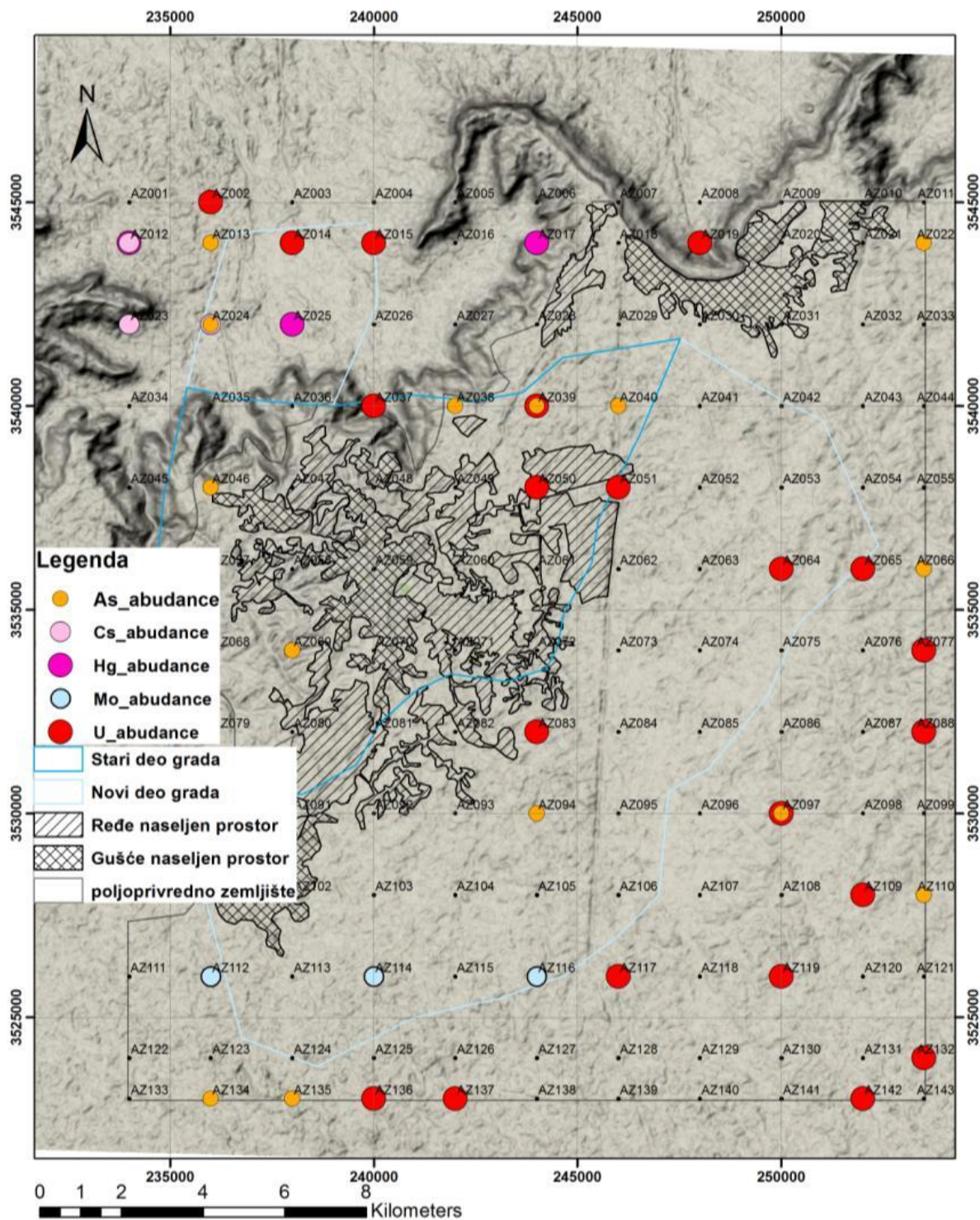
Slika 11.1: Distribucija polutanata povišenih koncentracija na prosoru Zintana
