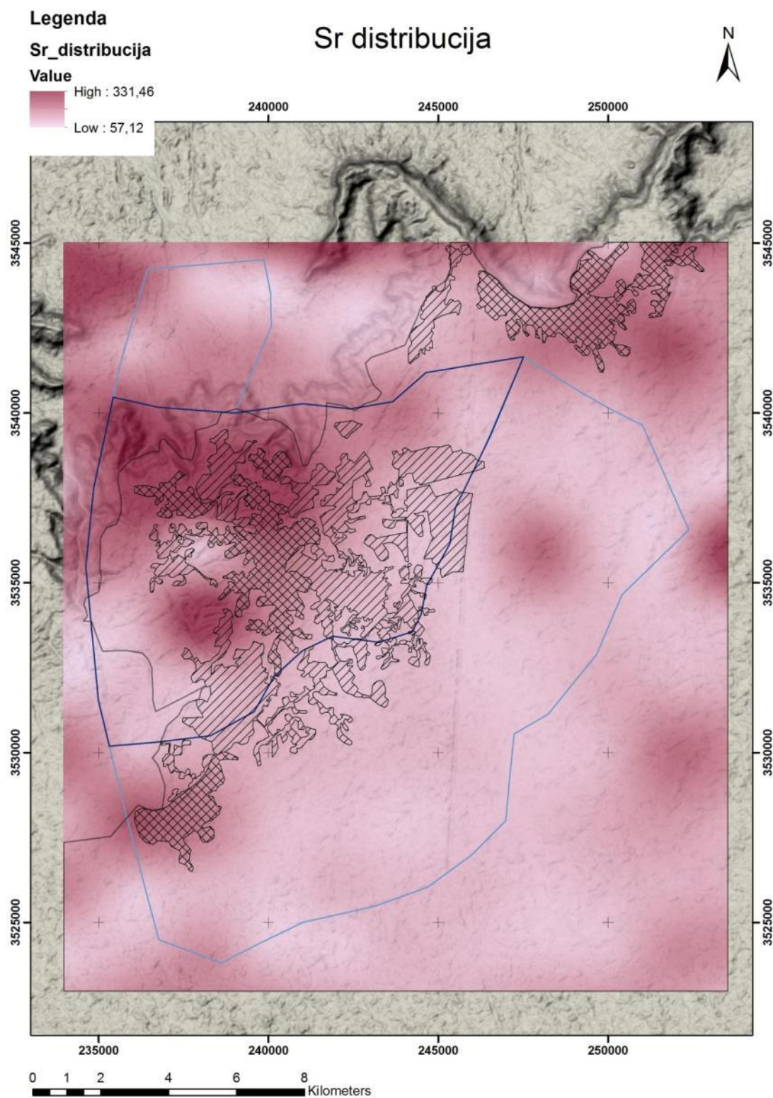
Slika 8.30: Interpolacija distribucija Sr srazmerno izmerenim sadržajima
