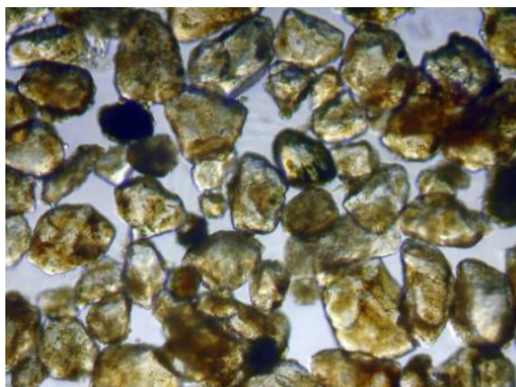
Slika 4.18: Mikroskopski snimak uzorka Zn109, lake frakcije
