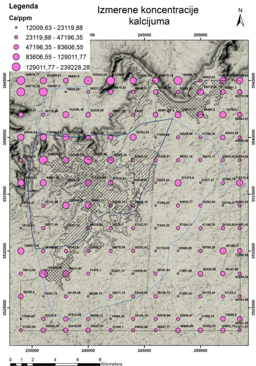
Slika 8.27: Tačkasta distribucija Ca srazmerno izmerenim sadržajima
