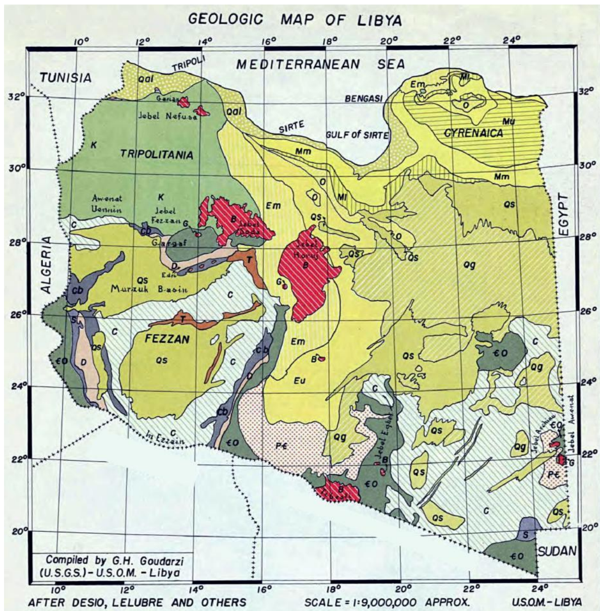
Slika 4.1: Šematska geološka karta Libije (Goudrazi, 1959)
