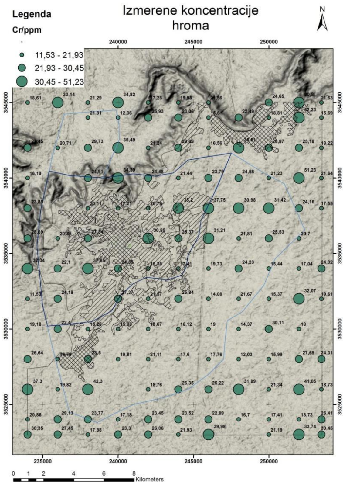
Slika 8.1: Tačkasta distribucija Cr srazmerno izmerenim sadržajima
