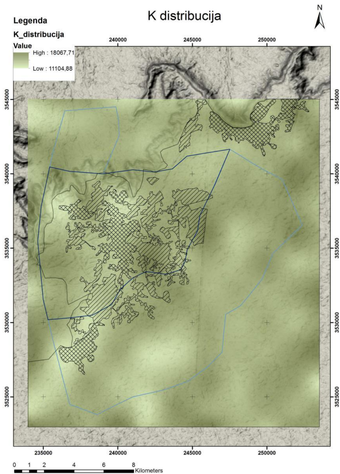
Slika 8.40: Interpolacija distribucija K srazmerno izmerenim sadržajima
