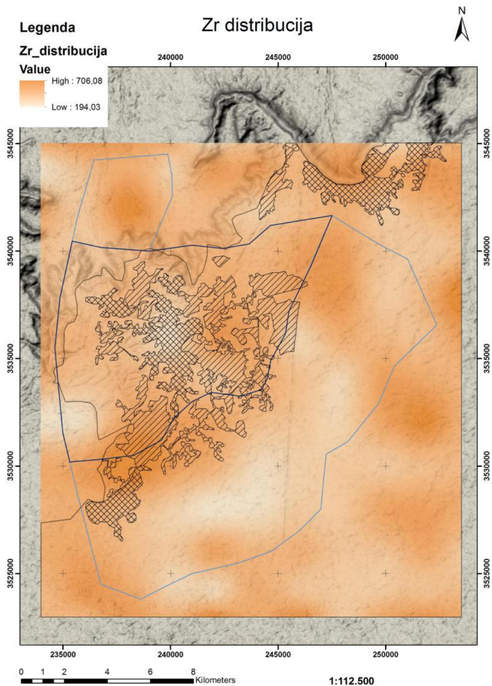
Slika 8.46: Interpolacija distribucija Zr srazmerno izmerenim sadržajima
