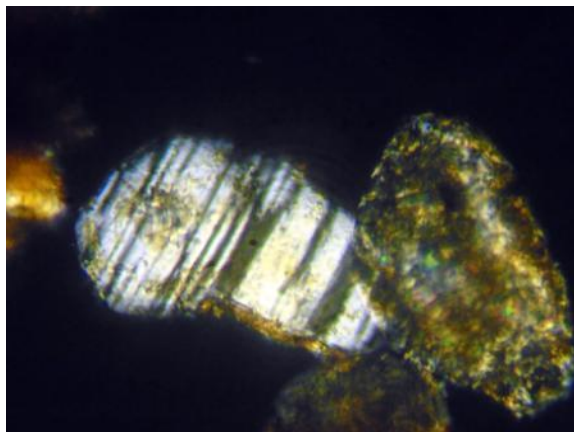
Slika 4.20: Mikroskopski snimak uzorka Zn120
