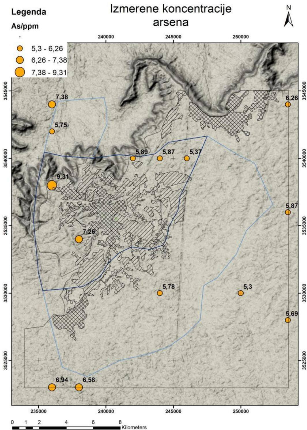
Slika 8.21: Tačkasta distribucija As srazmerno izmerenim sadržajima
