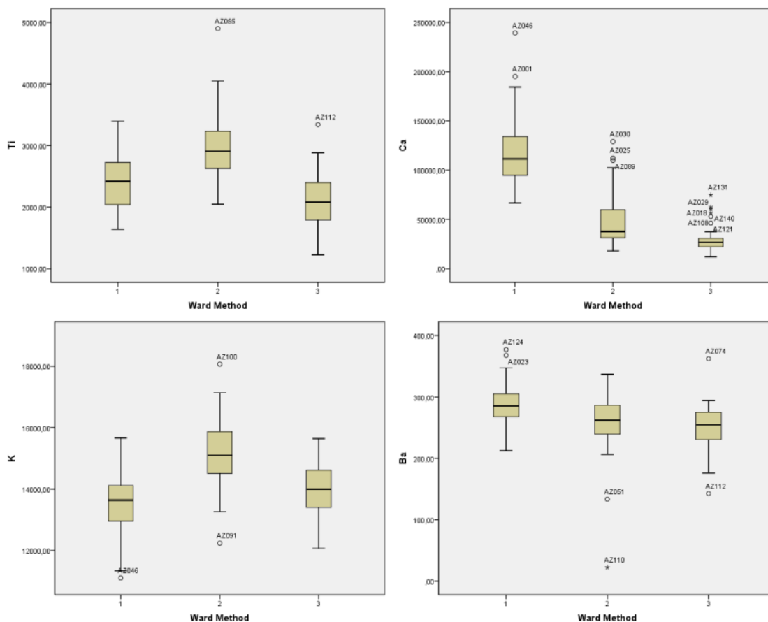
Slika 10.3: Boks-plot dijagrami analiziranih hemijskih elemenata (tj. varijabli), po grupama (koncentracije izražene u ppm; elementi dijagrama: minimum, donji kvartil (najnižih 25 % vrednosti), medijana, gornji kvartil (najviših 25 % vrednosti), maksimum i ekstremne vrednosti (outliers 6 ).
