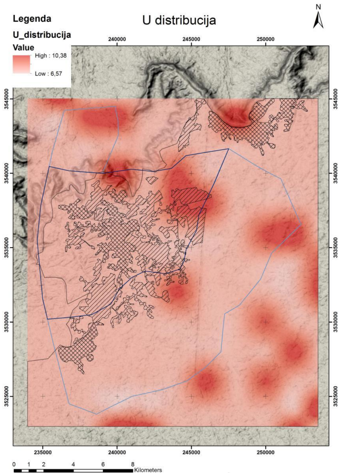
Slika 8.42: Interpolacija distribucija U srazmerno izmerenim sadržajima
