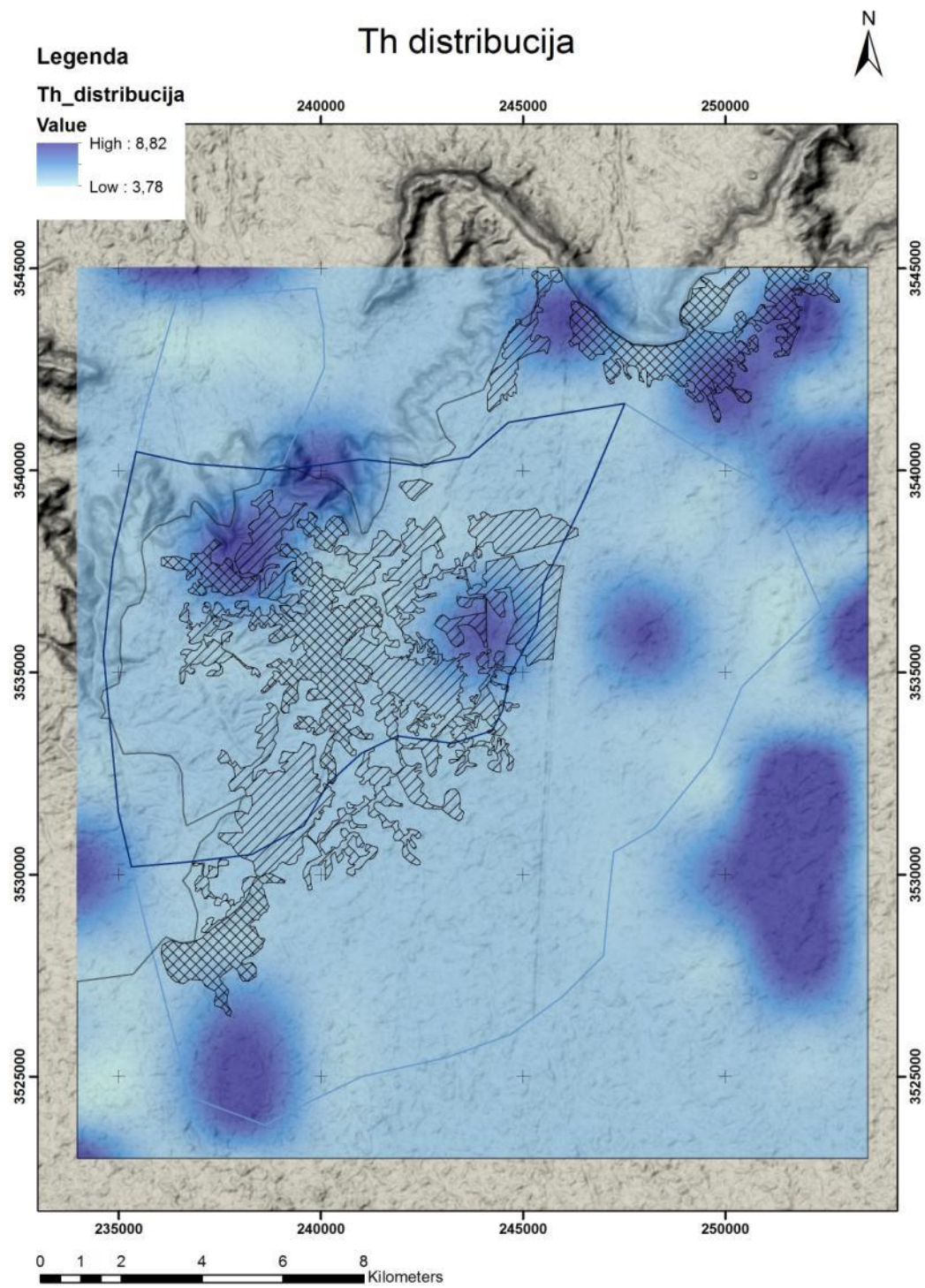
Slika 8.44: Interpolacija distribucija Th srazmerno izmerenim sadržajima
