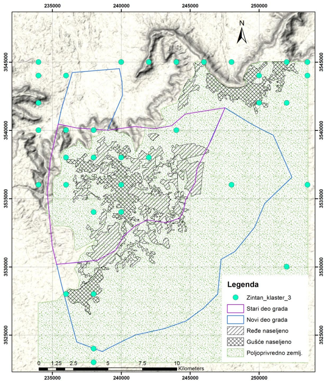
Slika 10.6: Prostorna distribucija uzoraka iz Klastera 3
