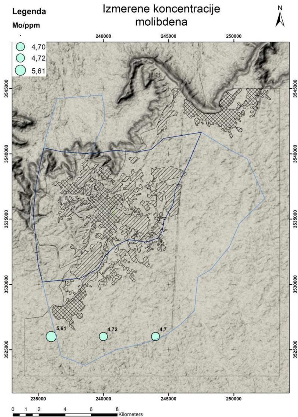
Slika 8.35: Tačkasta distribucija Mo srazmerno izmerenim sadržajima
