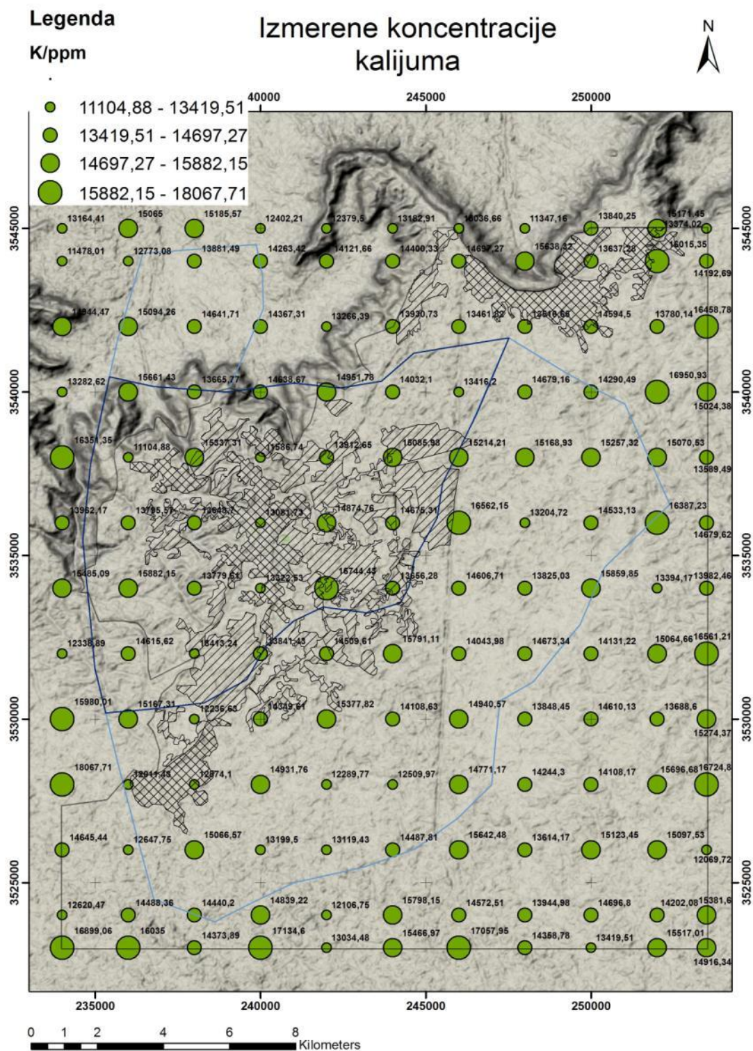
Slika 8.39: Tačkasta distribucija V srazmerno izmerenim sadržajima
