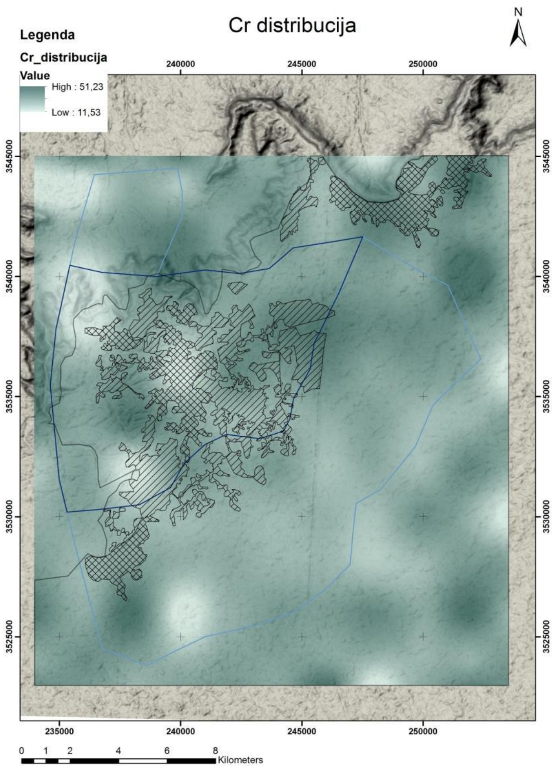
Slika 8.2: Interpolacija distribucija Cr srazmerno izmerenim sadržajima
