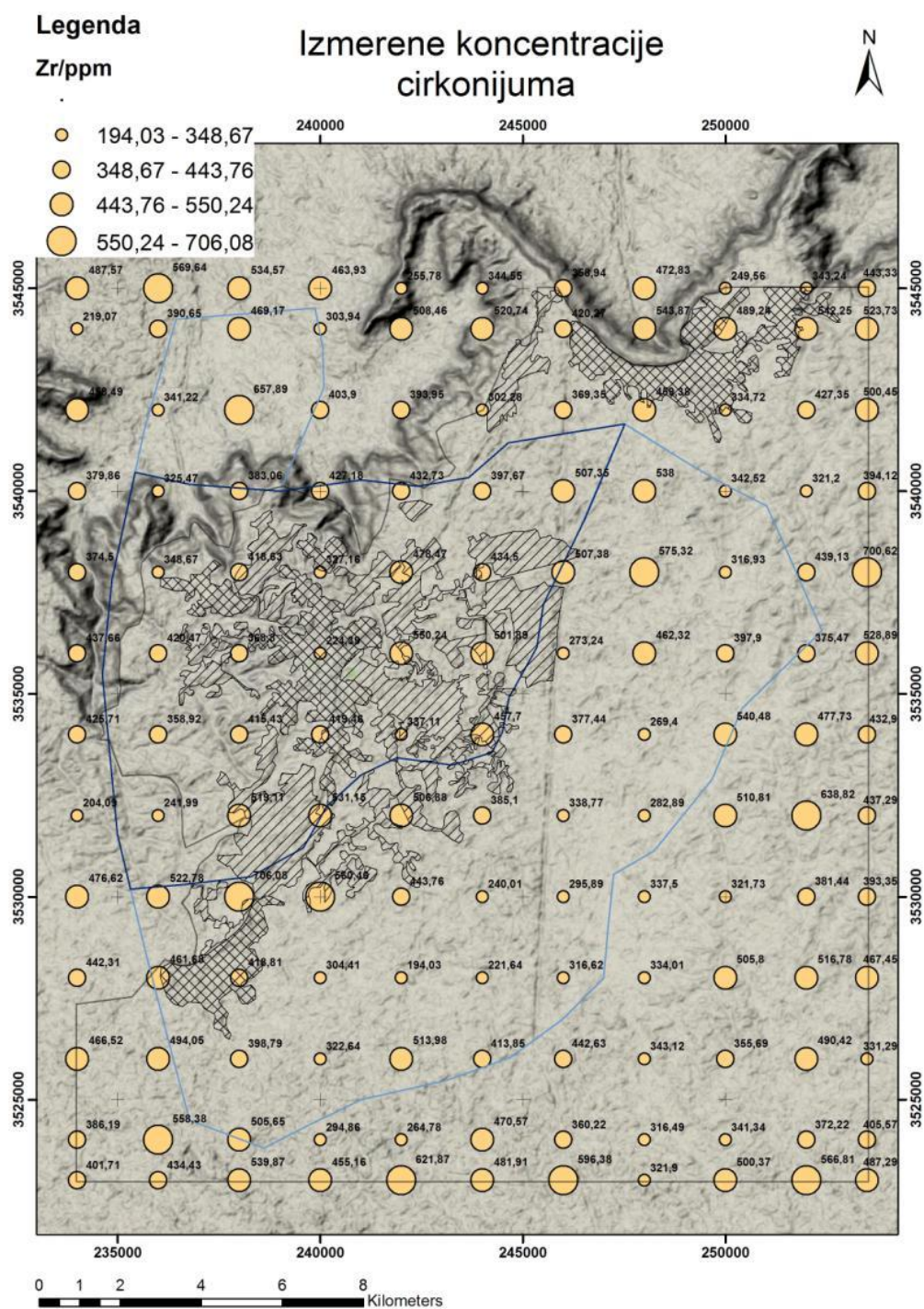
Slika 8.45: Tačkasta distribucija Zr srazmerno izmerenim sadržajima
