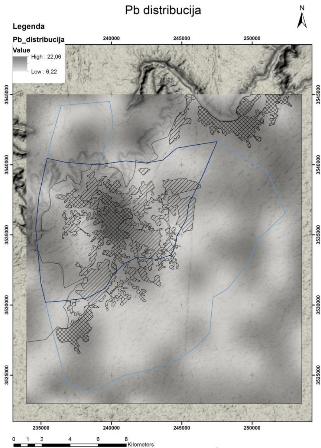
Slika 8.12: Interpolacija distribucija Pb srazmerno izmerenim sadržajima
