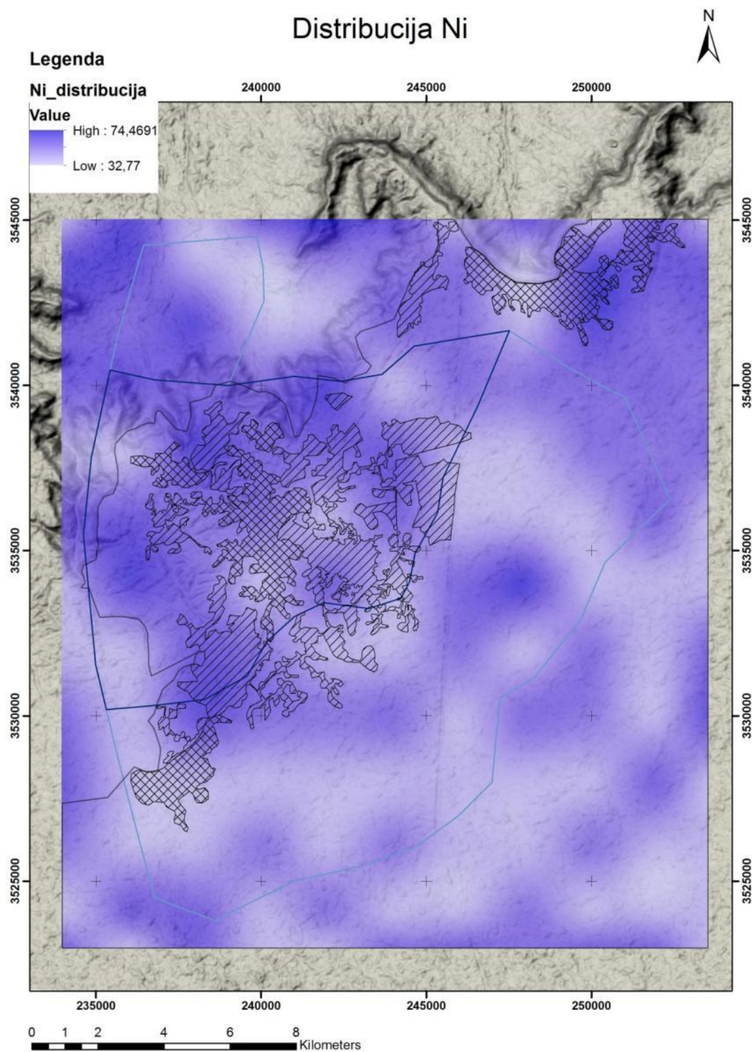
Slika 8.4: Interpolacija distribucija Ni srazmerno izmerenim sadržajima
