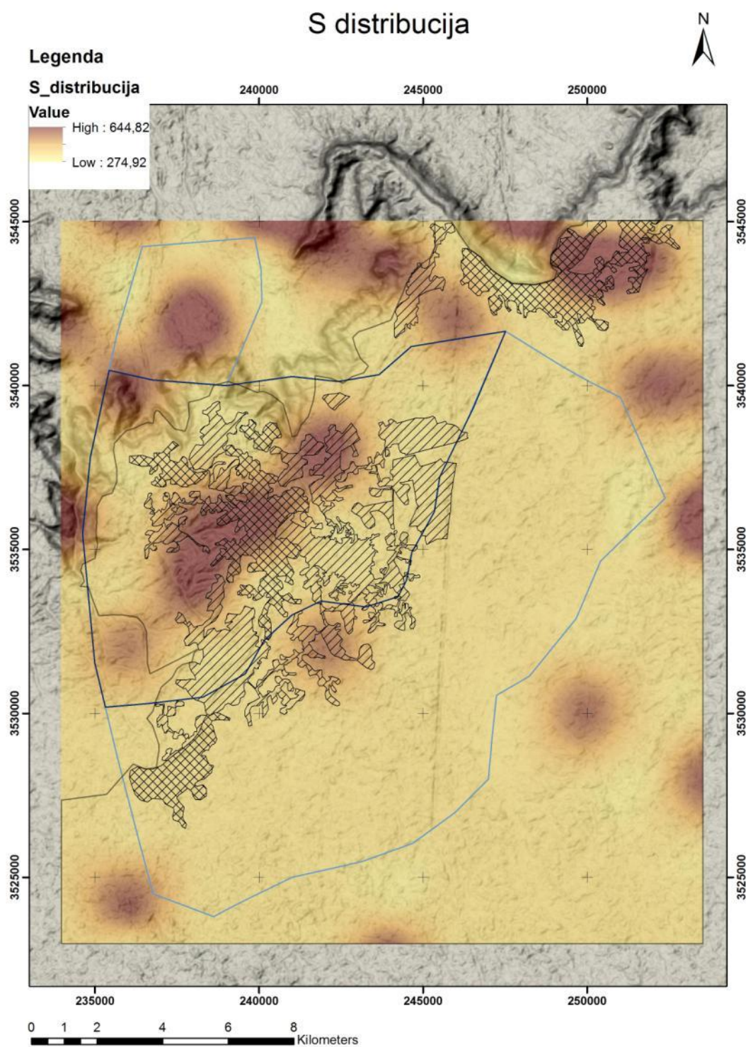
Slika 8.20: Interpolacija distribucija S srazmerno izmerenim sadržajima
