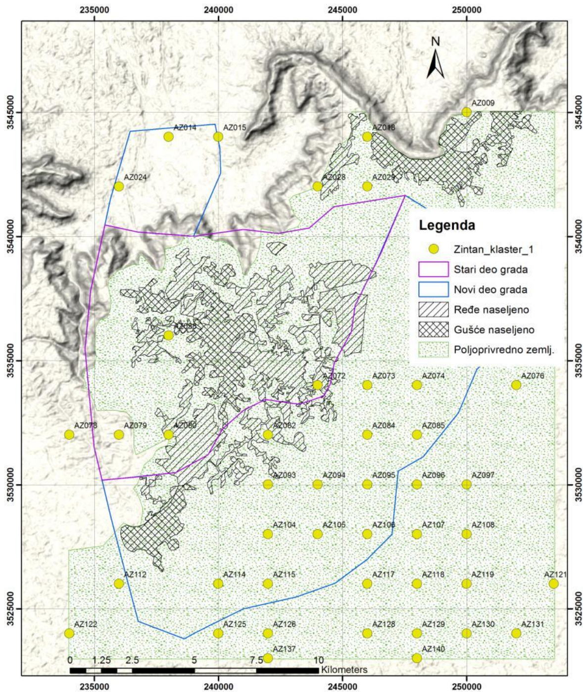
Slika 10.4: Prostorna distribucija uzoraka iz Klastera 1
