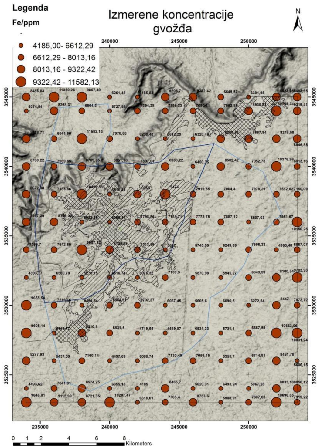
Slika 8.17: Tačkasta distribucija Fe srazmerno izmerenim sadržajima
