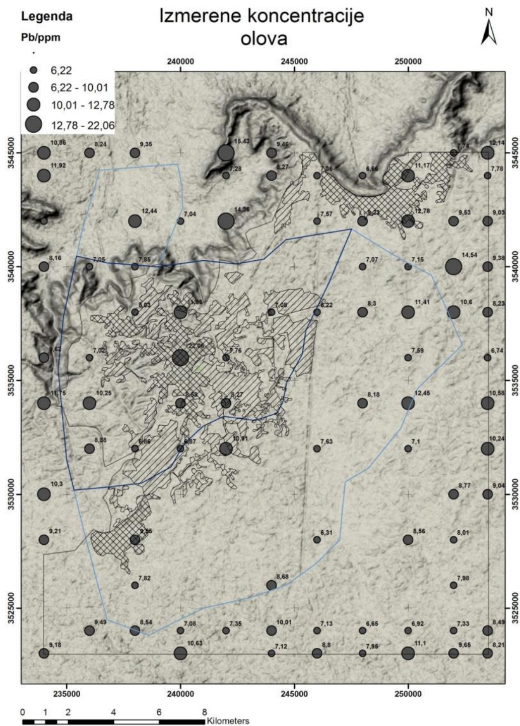
Slika 8.11: Tačkasta distribucija Pb srazmerno izmerenim sadržajima
