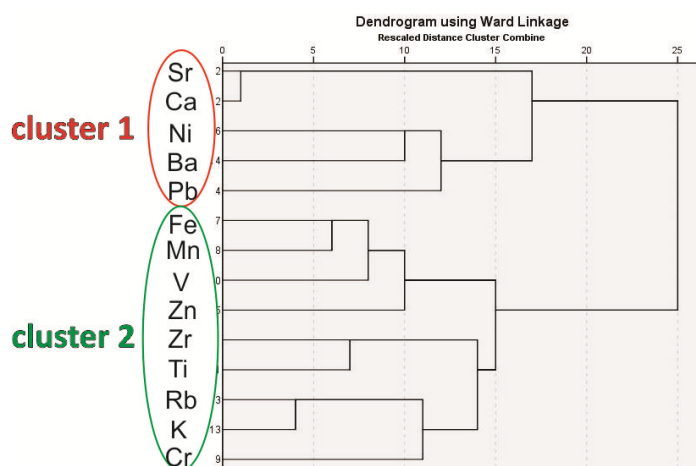
Slika 10.1: Dendrogram 14 analiziranih elemenata, dobijen R-mod klaster analizom (mera sličnosti: euklidsko rastojanje, način povezivanja: Vordov metod).
