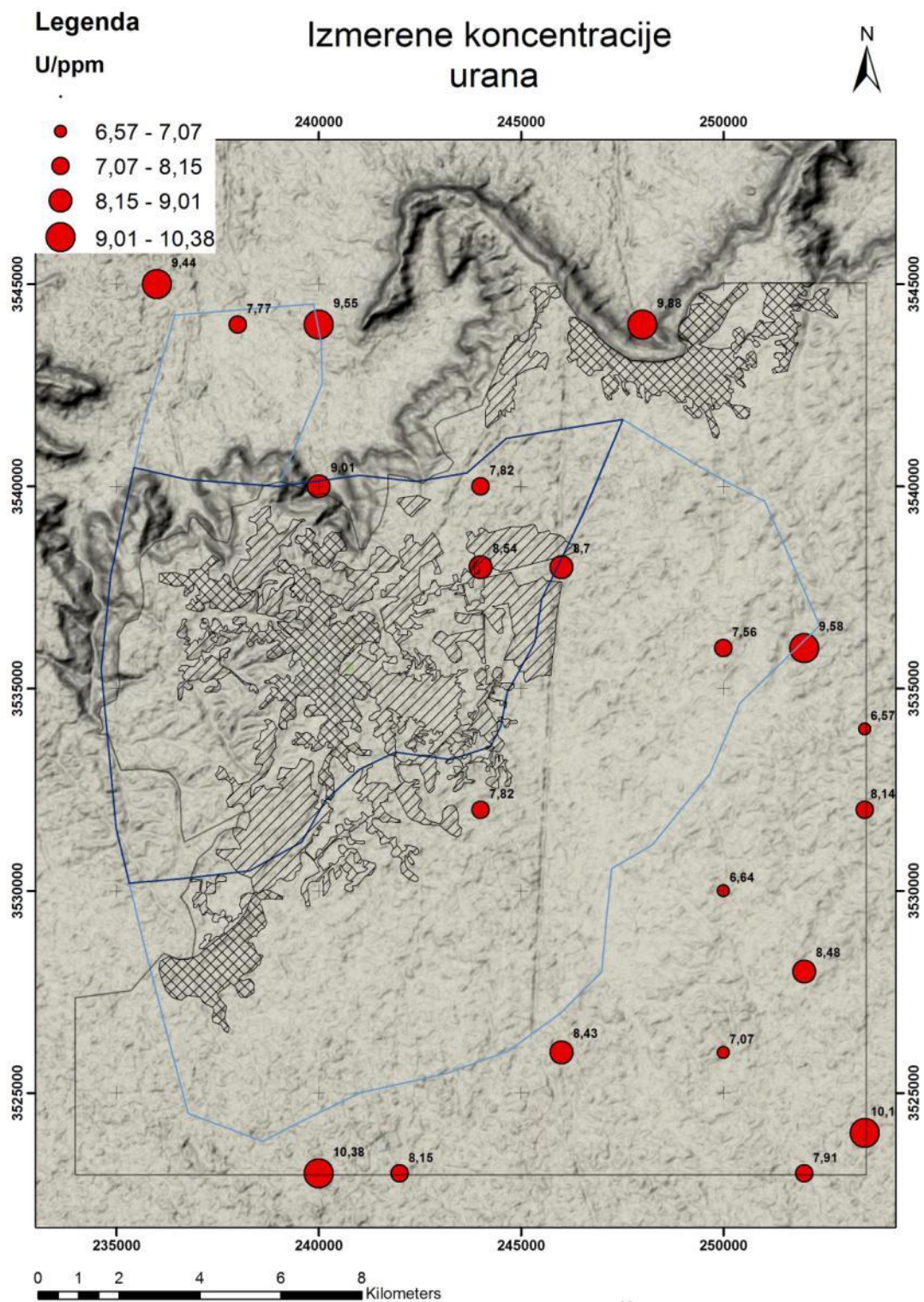
Slika 8.41: Tačkasta distribucija U srazmerno izmerenim sadržajima
