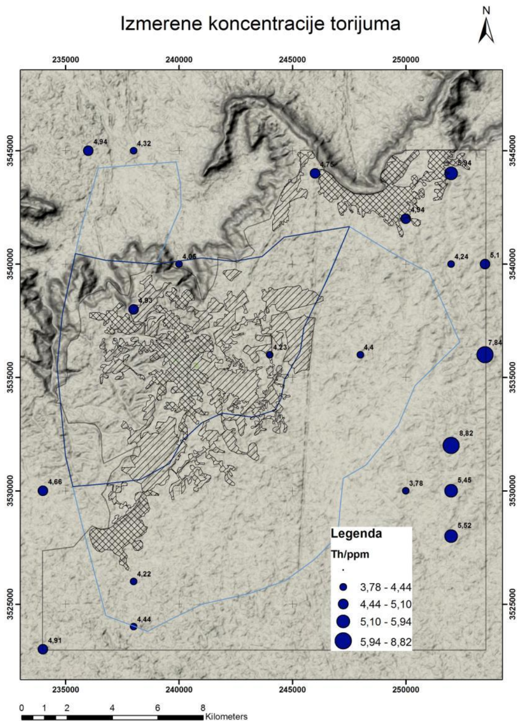
Slika 8.43: Tačkasta distribucija Th srazmerno izmerenim sadržajima
