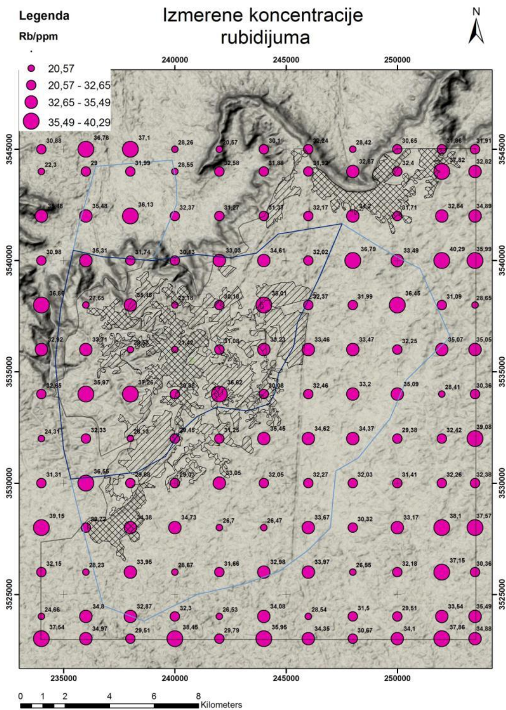
Slika 8.33: Tačkasta distribucija Rb srazmerno izmerenim sadržajima
