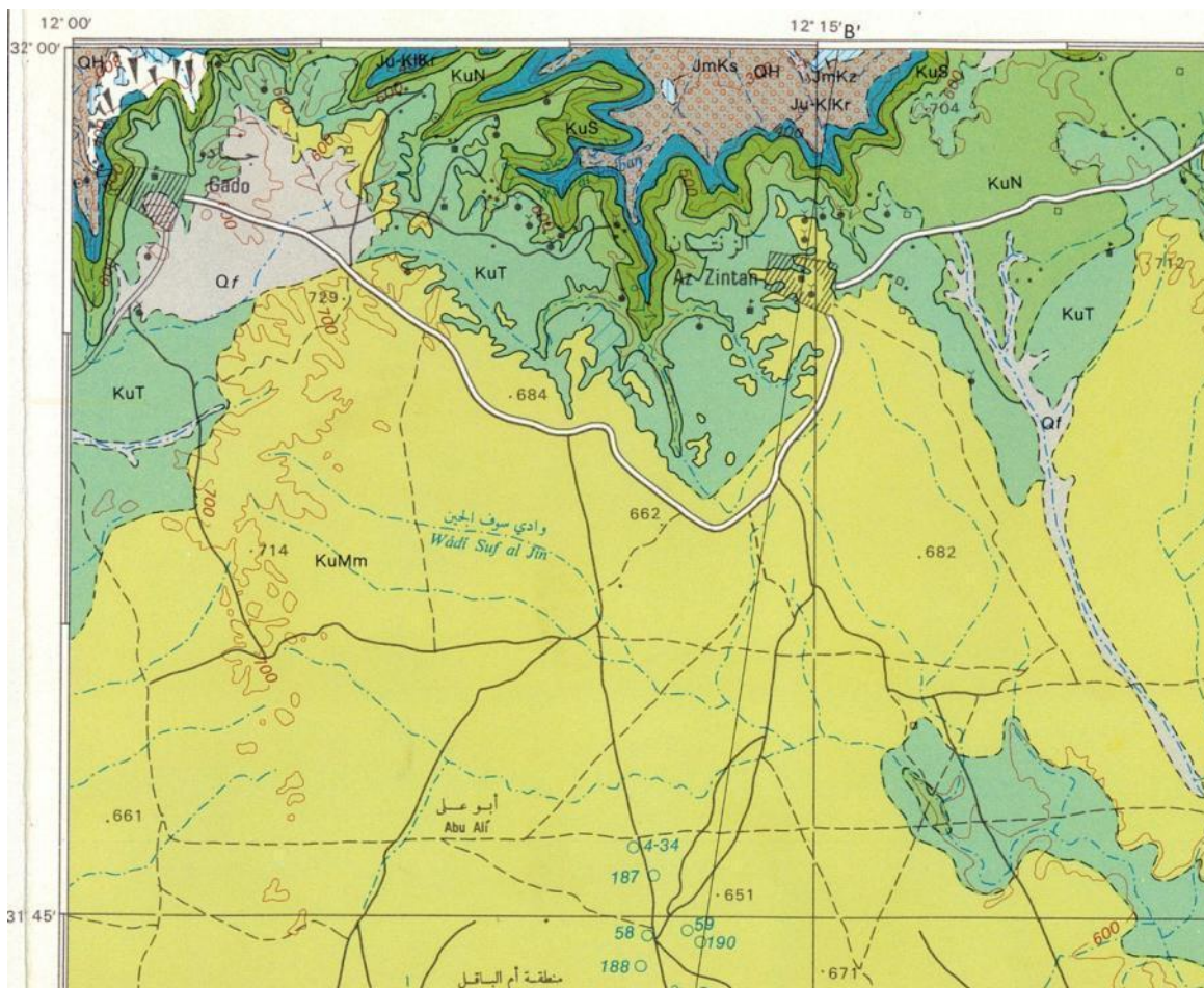
Slika 4.2: Geolška karta 1:250000 grada Zintana, list Mizdah, (Antonović 1977)
