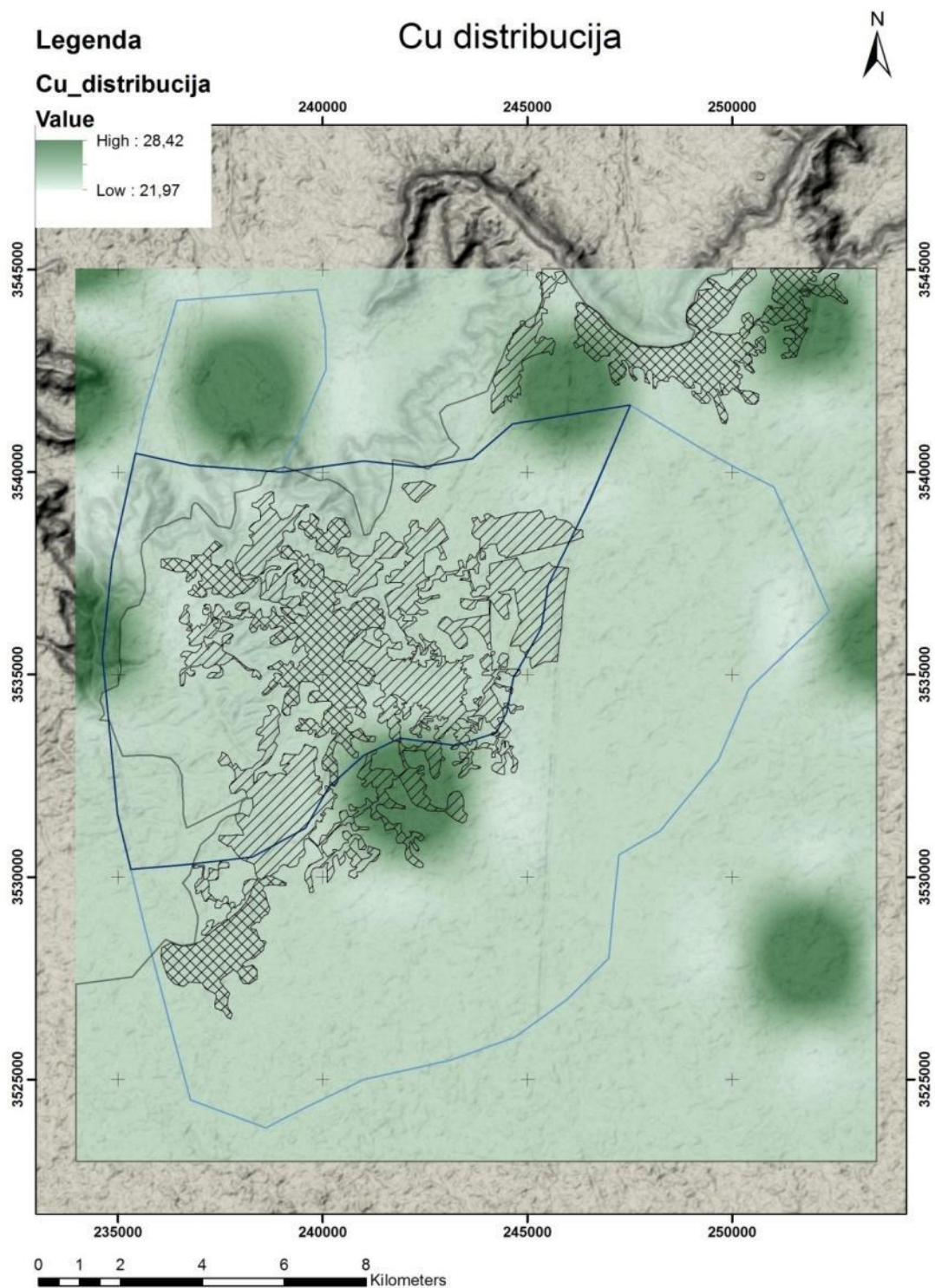
Slika 8.10: Interpolacija distribucija Cu srazmerno izmerenim sadržajima
