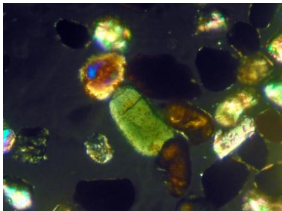
Slika 4.16: Mikroskopski snimak uzorka Zn082, teške frakcije
