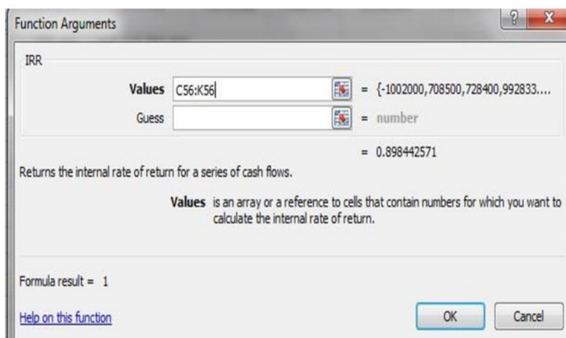
Slika 3-2 Računanje ISP u Excel-u
