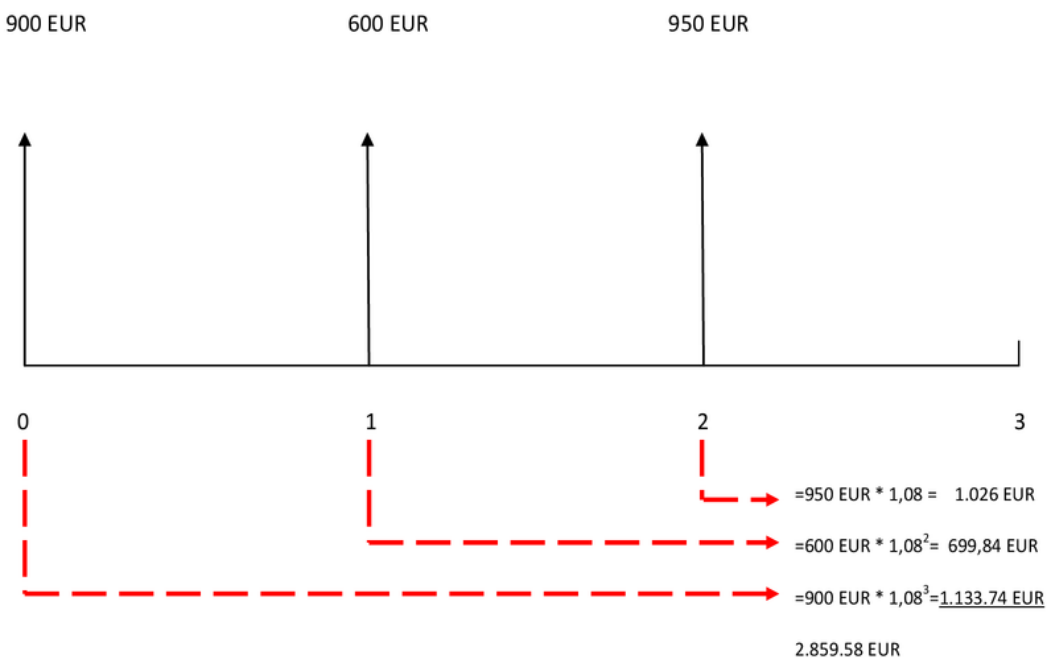
Slika 2-2 Buduća vrednost višestrukih novčanih tokova
