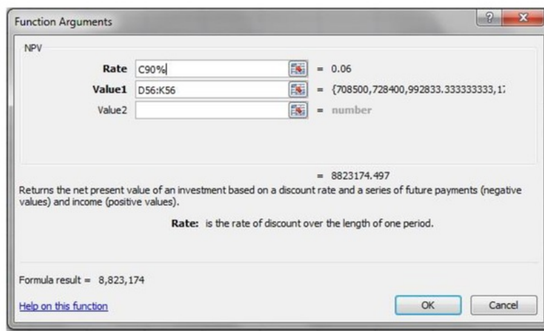
Slika 3-1 Računanje NSV-a u Excel-u
