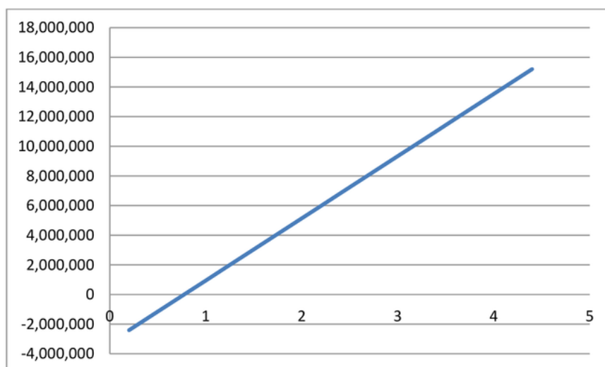
Grafikon 3-2 Analiza senzitivnosti na primeru cene i NSV-a u EUR (X osa-cena, Y osa- NSV)
