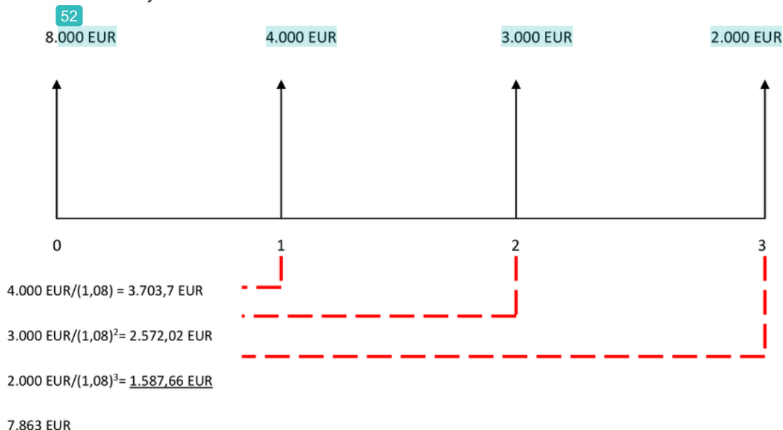
Slika 2-3 Sadašnja vrednost niza novčanih tokova
