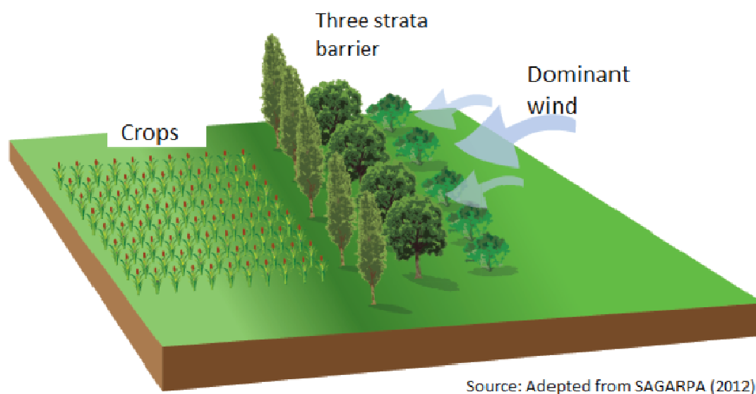
Slika 17. Delovanje vetrozaštitnog pojasa
