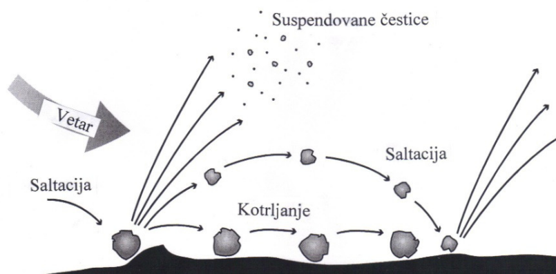
Slika 4. Elementi kretanja zemljišnih čestica pod uticajem vetra
