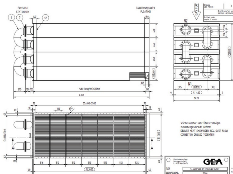
Slika 20 – Razmenjivač toplote dimnih gasova
