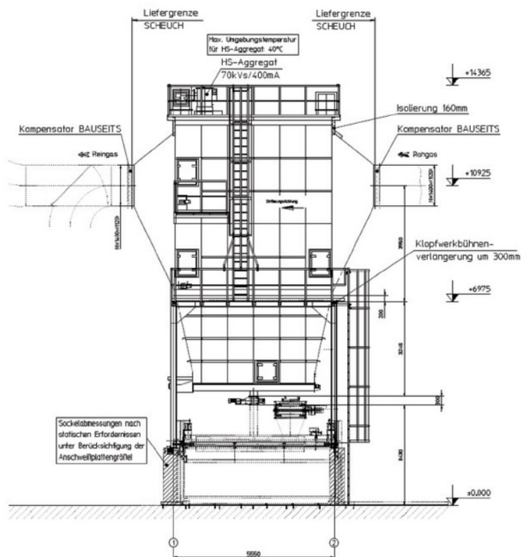
Slika 19 – Elektro filter
