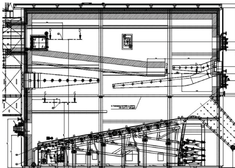
Slika 17 – Ložište
