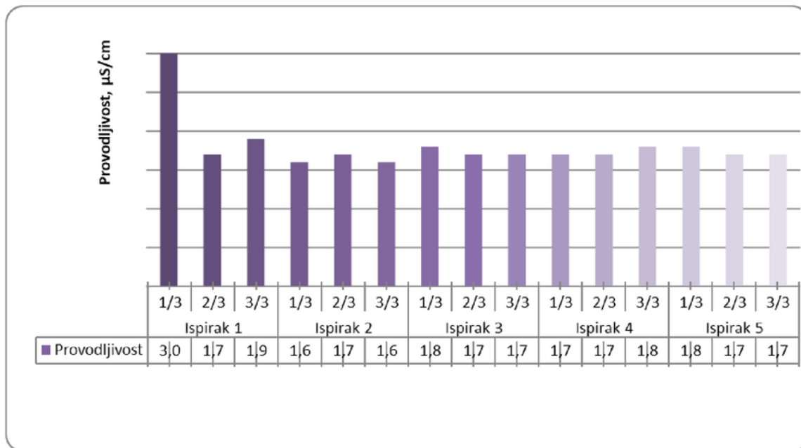
Grafik 5. Grafički prikaz rezultata ispitivanja provodljivosti hemijskih ispiraka HI1-HI5 tokom drugog ispitivanja
