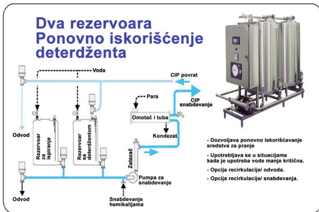
Slika 15: Sistem za automatsko čišćenje sa dva tanka
