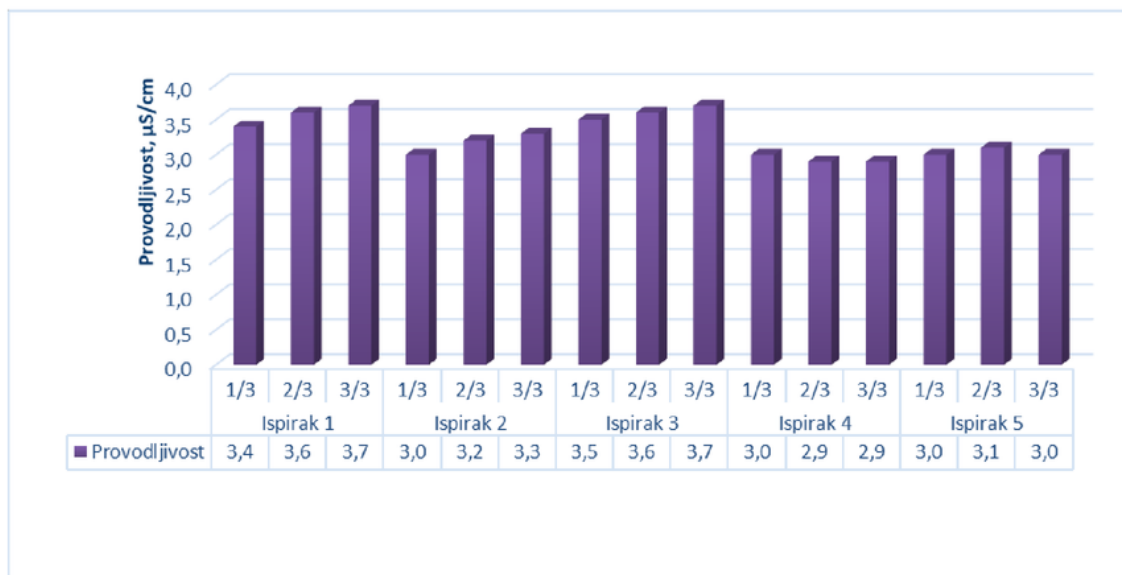
Grafik 2. Grafički prikaz rezultata ispitivanja provodljivosti hemijskih ispirka HI1-HI5 tokom prvog ispitivanja
