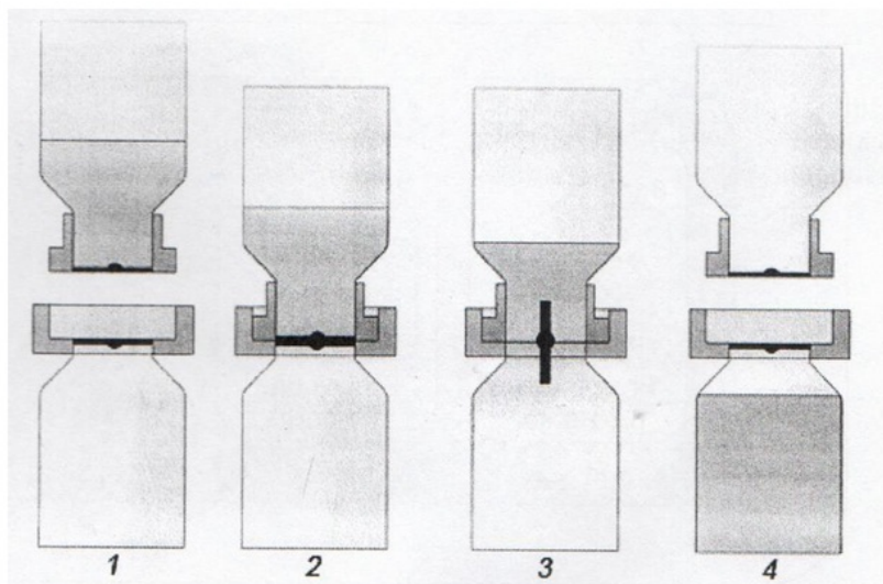
Slika 6. prikaz operacije zatvorenog procesa
