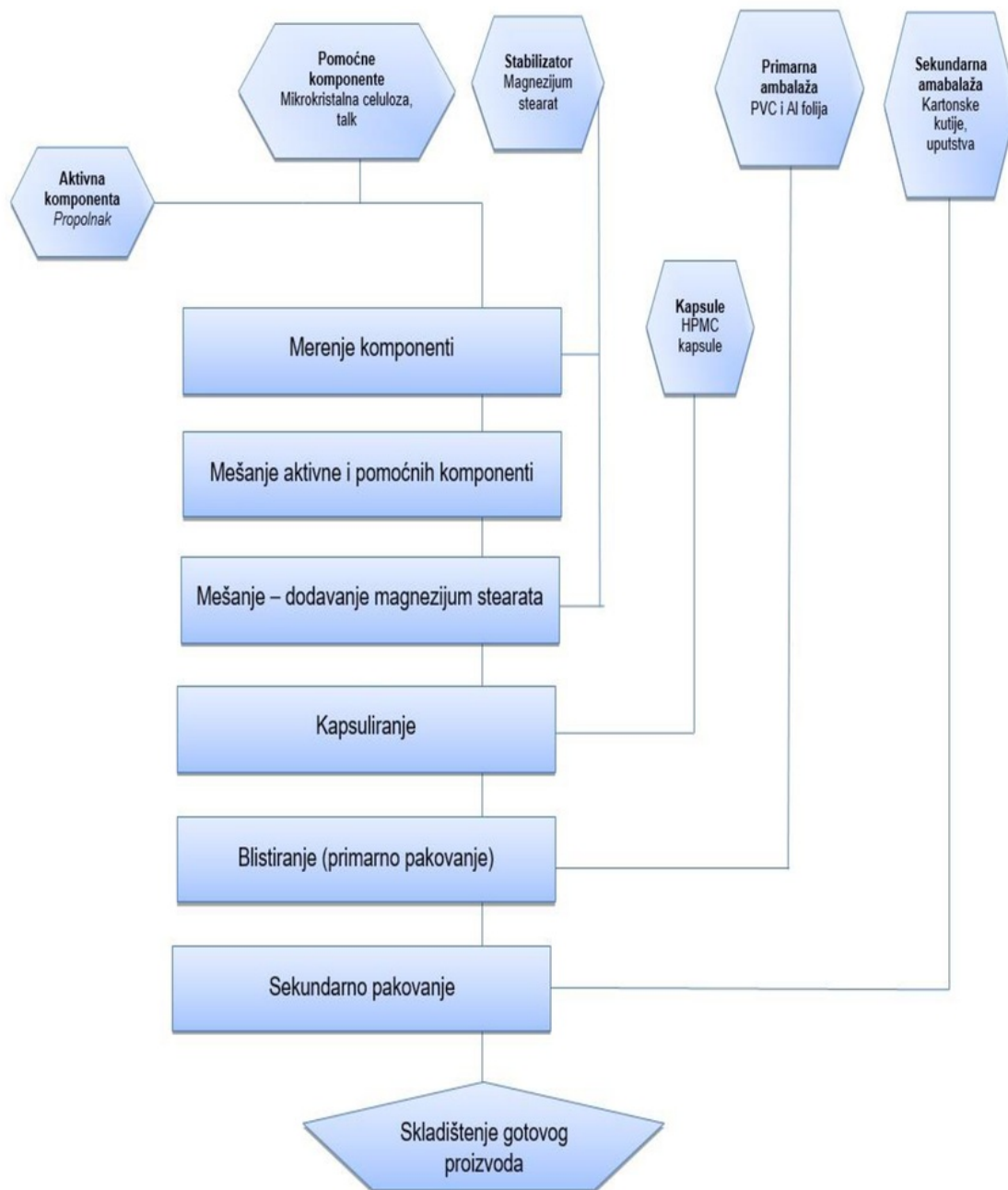
Slika 40: Dijagram toka procesa proizvodnje Propomucil kapsula
