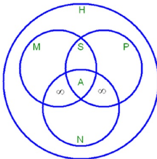
Slika 7. Vrste homomorfizama
