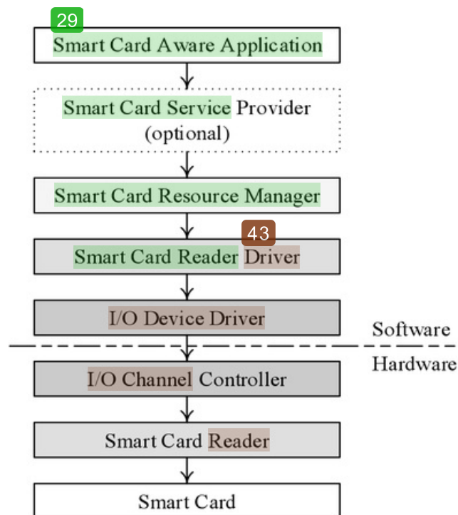
Slika 12. PC/SC arhitektura
