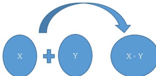
Slika 8. Homomorfizam nad šifarskim sistemom
