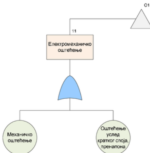
Слика 9.7 Дијаграм електромеханичког оштећења
