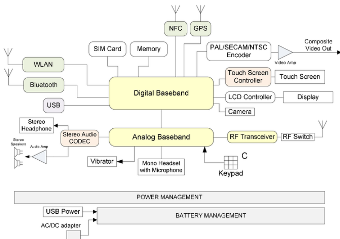
Слика 9.1 Општа блок шема паметног телефона
