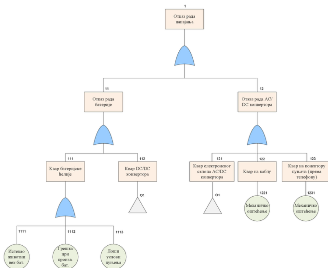
Слика 9.6 Стабло отказа рада напајања мобилног телефона
