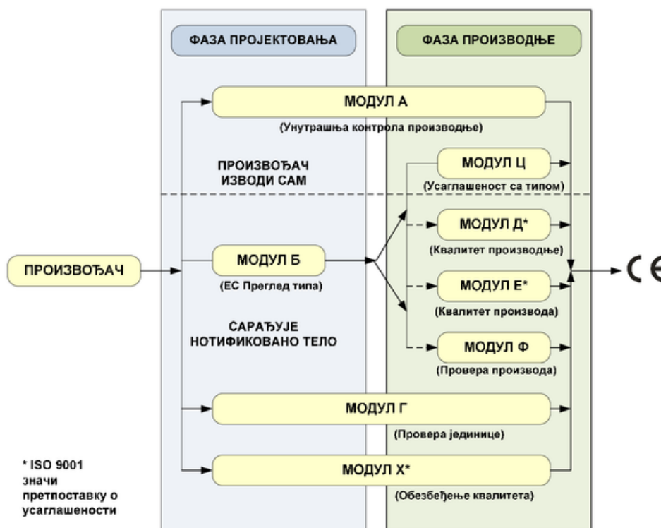
Слика 2.4 Дијаграм поступка за оцењивање усаглашености
