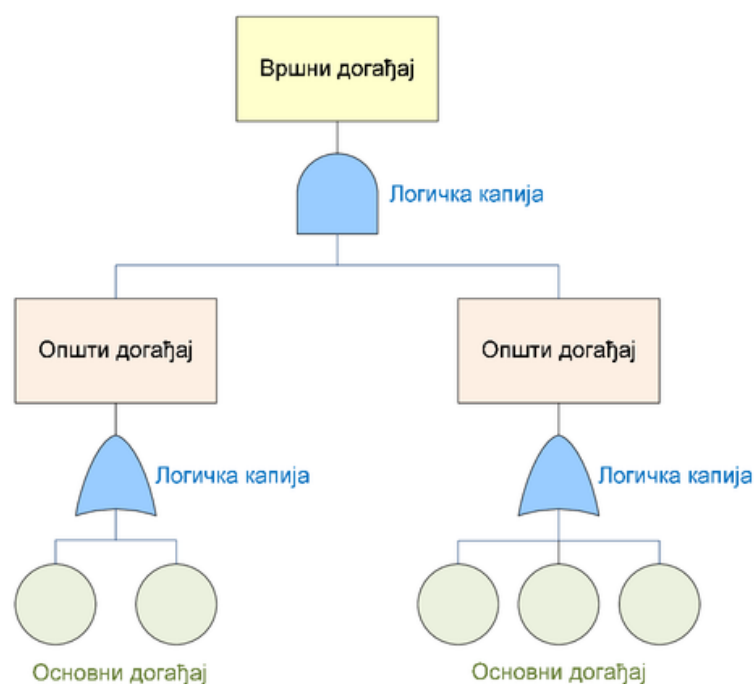
Слика 5.1 Пример графичке презентације стабла отказа
