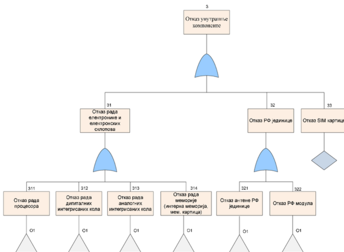
Слика 9.9 Стабло отказа унутрашњих компоненти мобилног телефона
