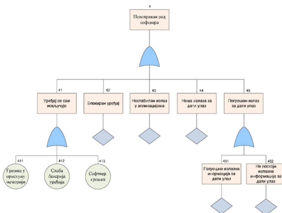
Слика 9.10 Стабло отказа софтвера мобилног телефона
