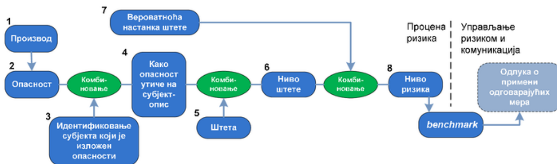
Слика 4.2. Радна верзија процедуре за оцену ризика производа који не испуњавају основне захтеве Директиве о РИТТ опреми
