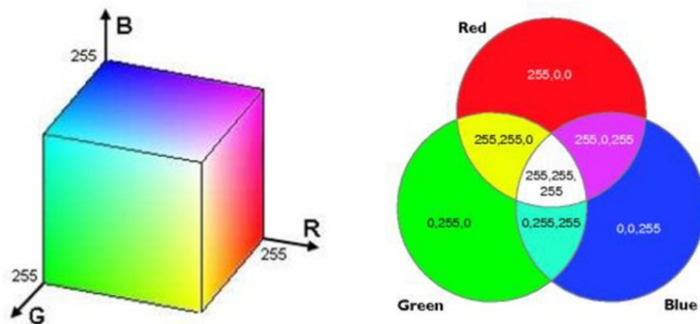
Slika 41. Koordinatni prikaz RGB modela
