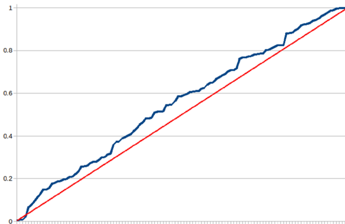
Slika 34. Grafik slučajne raspodele audio uzorka 1
