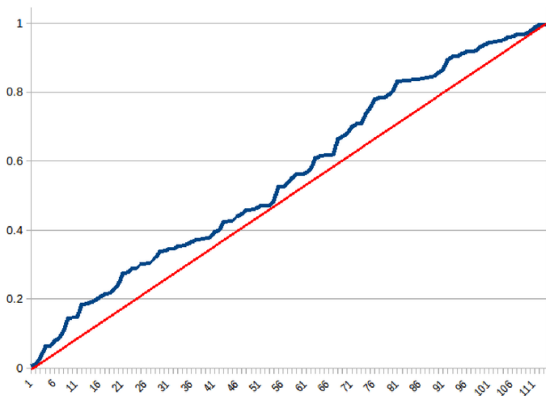
Slika 49. Grafik slučajne raspodele video uzorka 5
