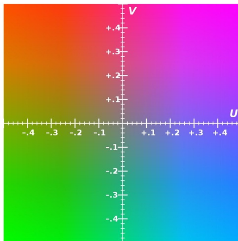
Slika 42. Koordinatni prikaz YUV modela
