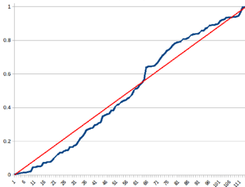
Slika 46. Grafik slučajne raspodele video uzorka 2
