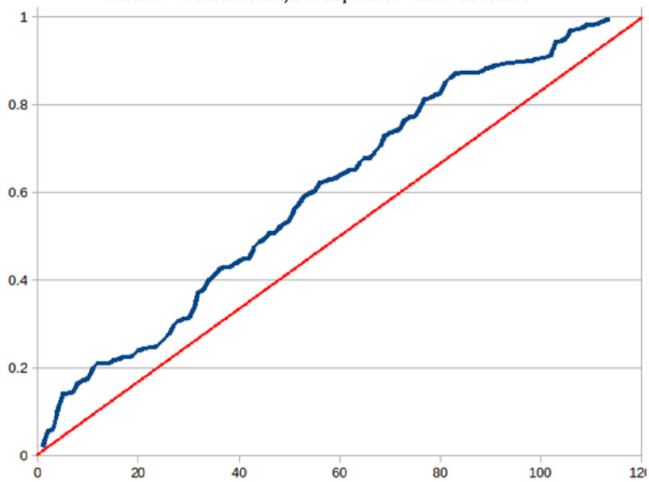
Slika 48. Grafik slučajne raspodele video uzorka 4
