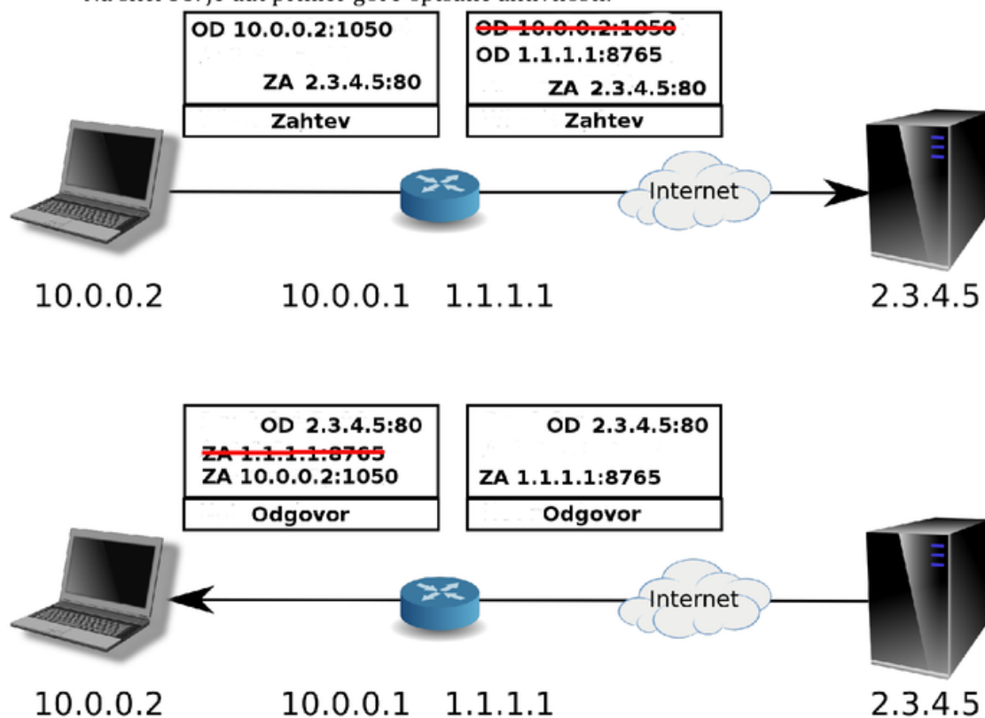
Slika 55. UDP Punch hole proces
