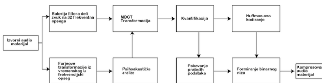
Slika 33. Blok šema kompresije .mp3 audio formata
