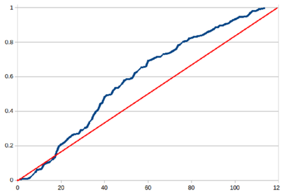
Slika 47. Grafik slučajne raspodele video uzorka 3
