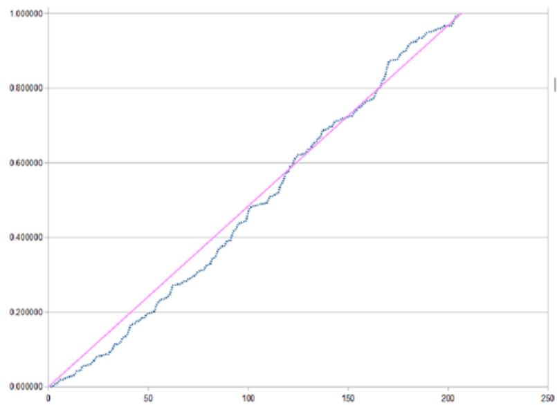
Slika 24. Grafik primera idealne slučajne raspodele
