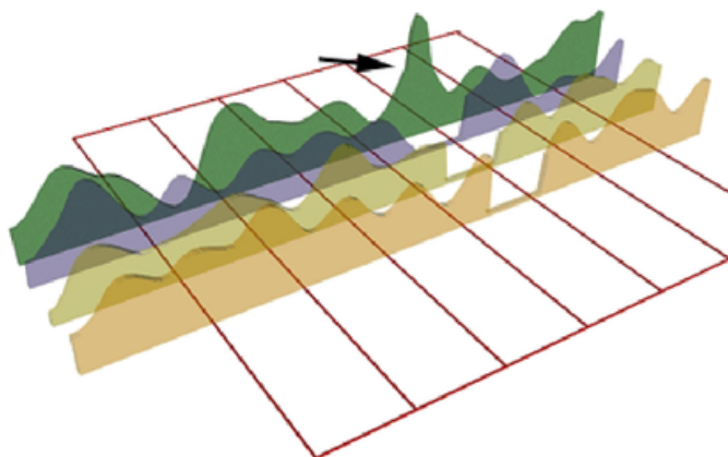
Slika 32. 3D akustički model polifonog zvučnog signala
