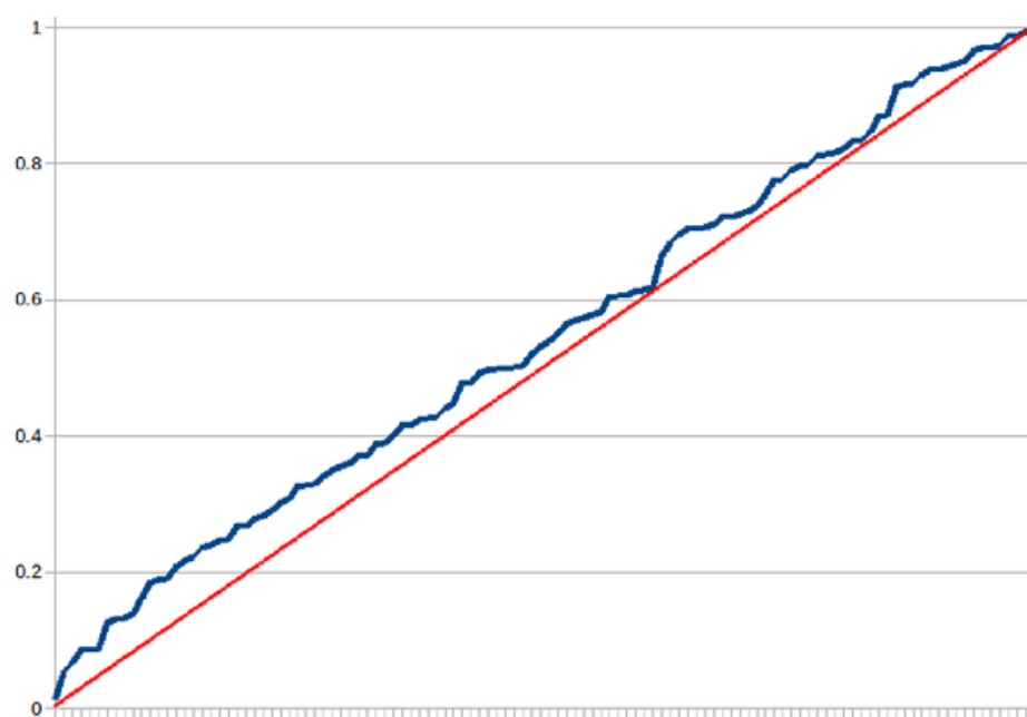
Slika 45. Grafik slučajne raspodele video uzorka 1
