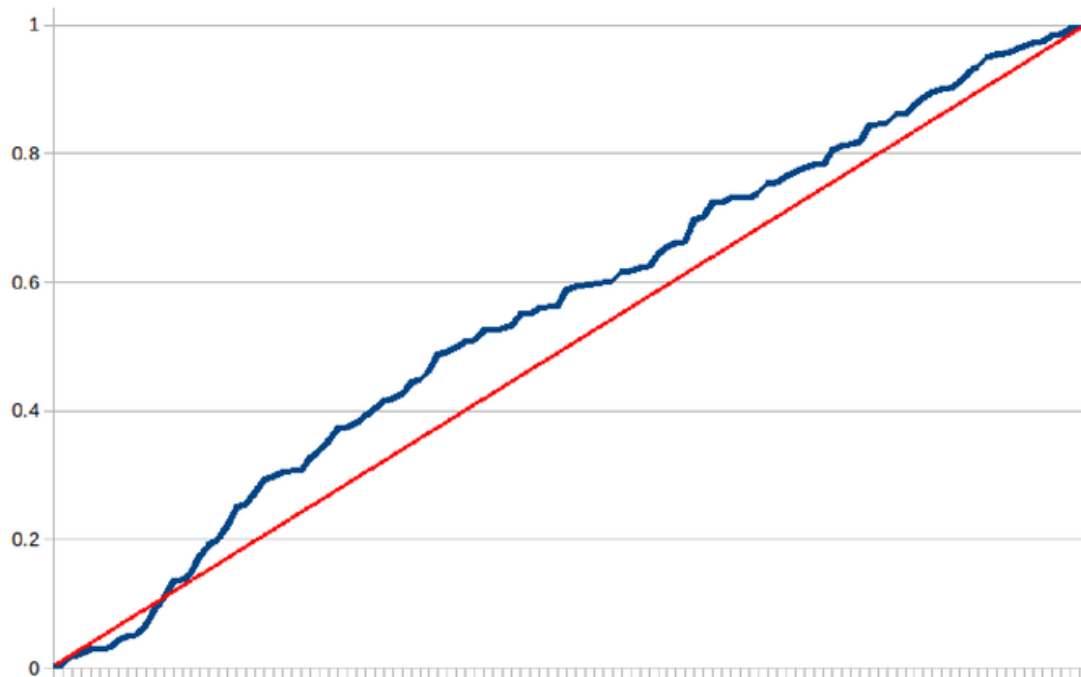
Slika 35. Grafik slučajne raspodele audio uzorka 2
