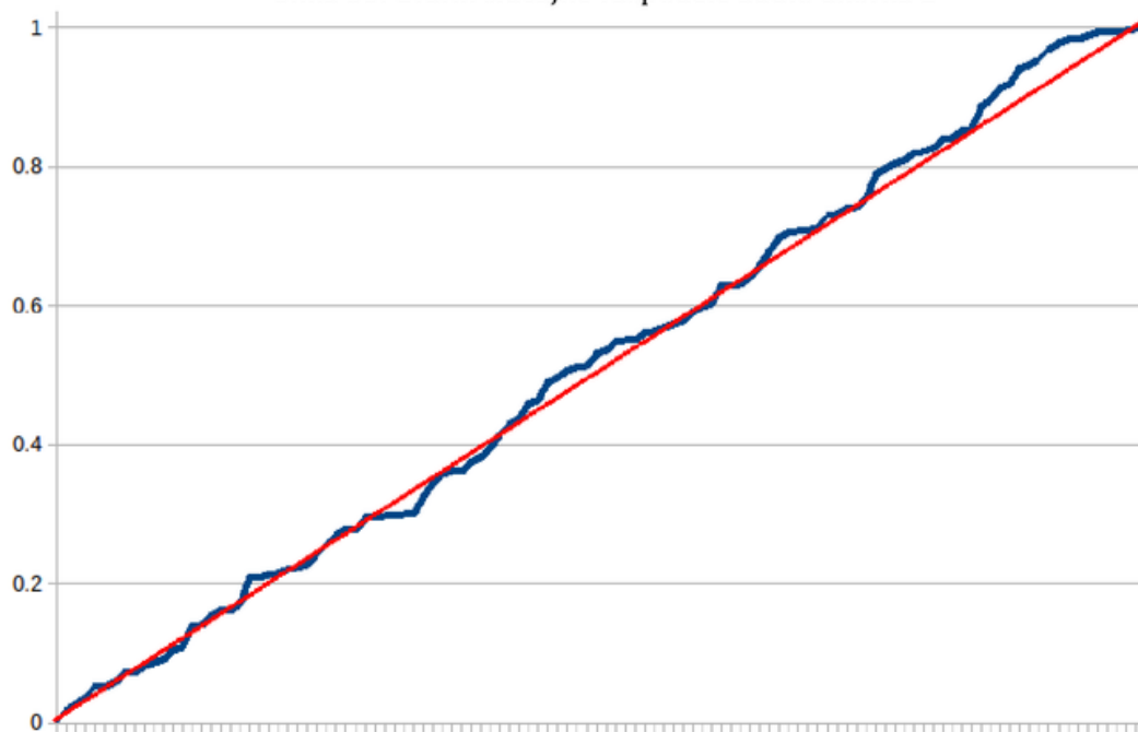
Slika 36. Grafik slučajne raspodele audio uzorka 3
