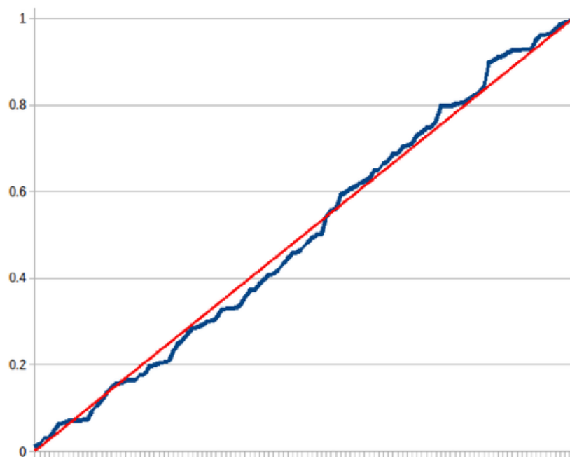
Slika 31. Grafik slučajne raspodele uzorka slike u .PNG formatu (b&w)
