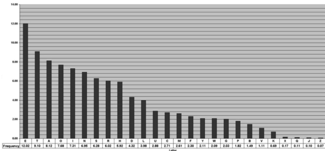
Slika 23. Statistika učestalosti pojedinih slova u abecedi
