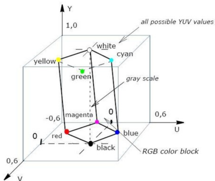
Slika 40. Vektorski YUV model boja
