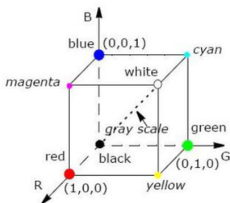
Slika 39. Vektorski RGB model boja
