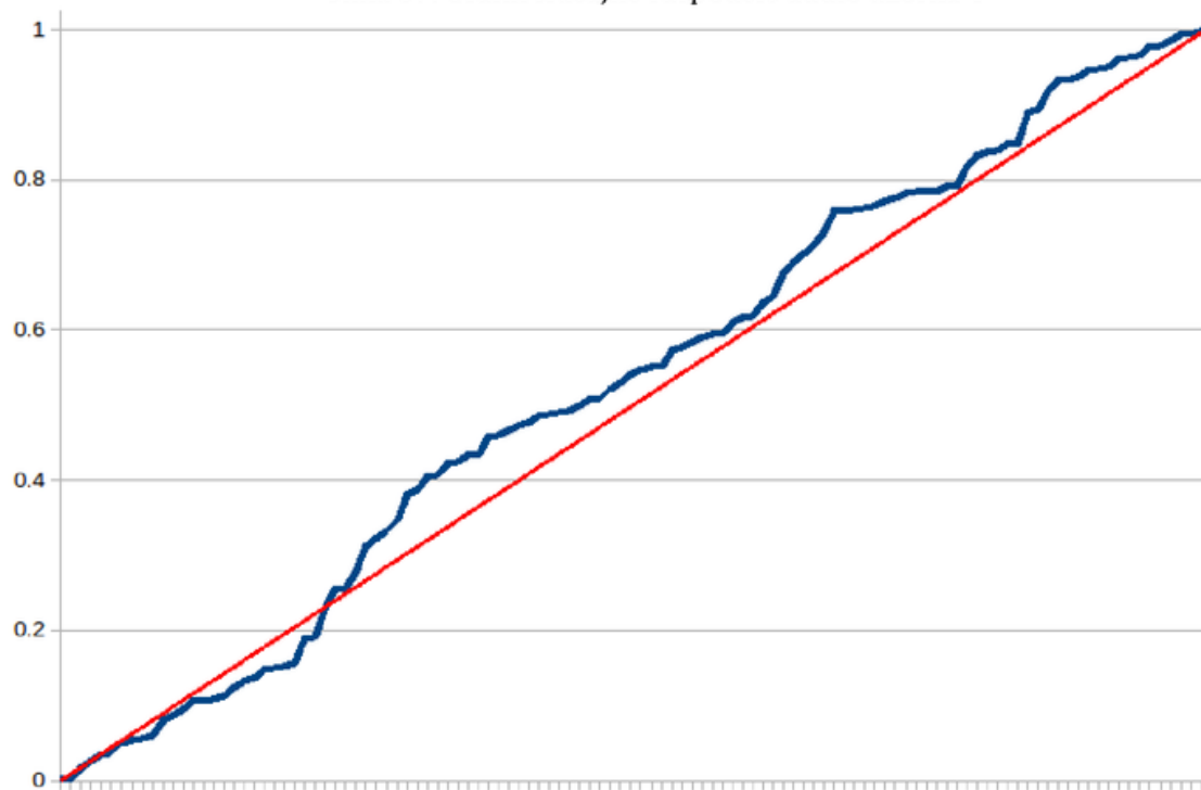
Slika 38. Grafik slučajne raspodele audio uzorka 5
