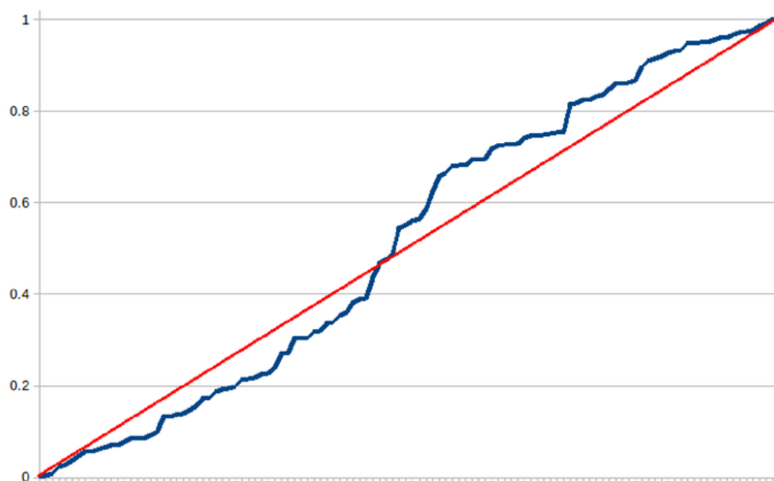
Slika 37. Grafik slučajne raspodele audio uzorka 4
