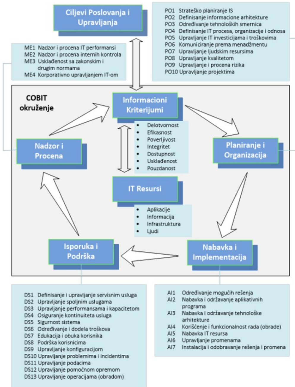
Slika 12- Cobit okvir 49
