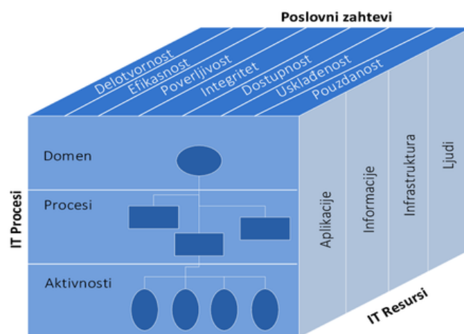
Slika 16- COBIT kocka
