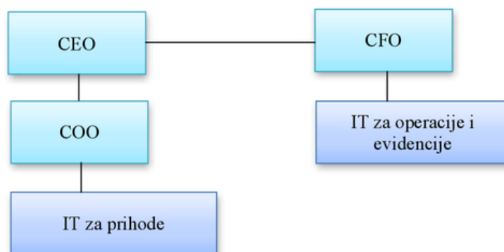
Slika 3 -Struktura izveštavanja
