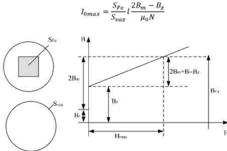
Слика 5.2.1.2. Попречни пресек гвозденог језгра и карактеристика магнетног
