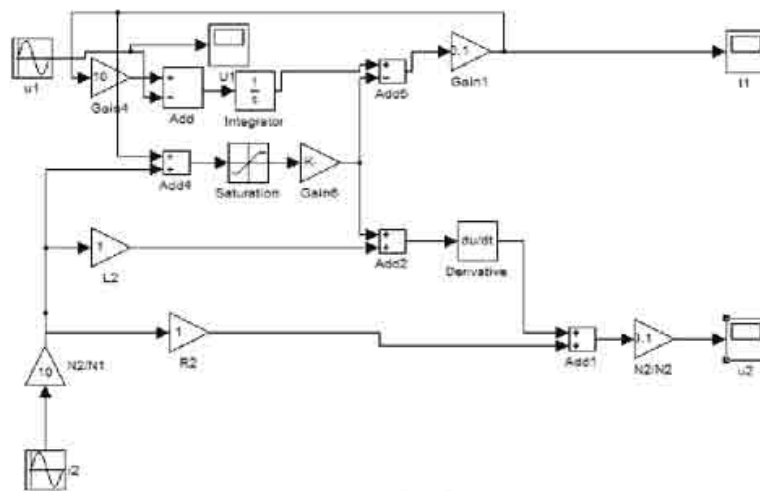
Слика 5.1.2.11 Засићен трансформатор
