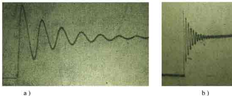
Слика 1.1.1. Развијене "слободне" компоненте напона (L. Fallou, Bulletin 1 ), а) напонског трансформатора 110/10kV, у четвртини периоде, б) енергетског трансформатора 4000kVA, 70 kV у половини периоде.
