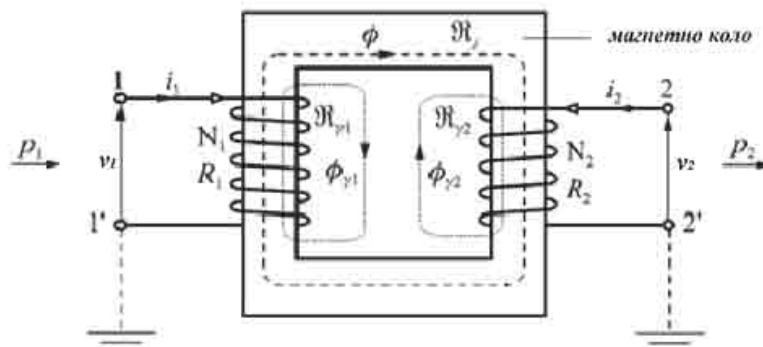
Слика 5.1.2. Једнофазни трансформатор
