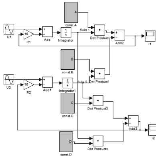
Слика 5.1.1.3. Поједностављена шема једнофазног трансформатора
