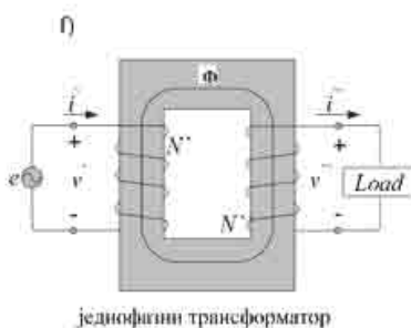
једнофазни трансформатор
