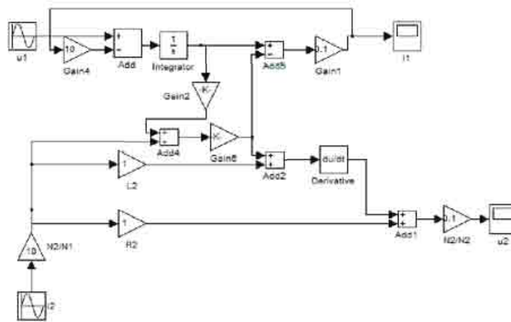
Слика 5.1.2.1 Модел једнофазног трансформатора са оптерећењем и линеарном карактеристиком магнетичног
