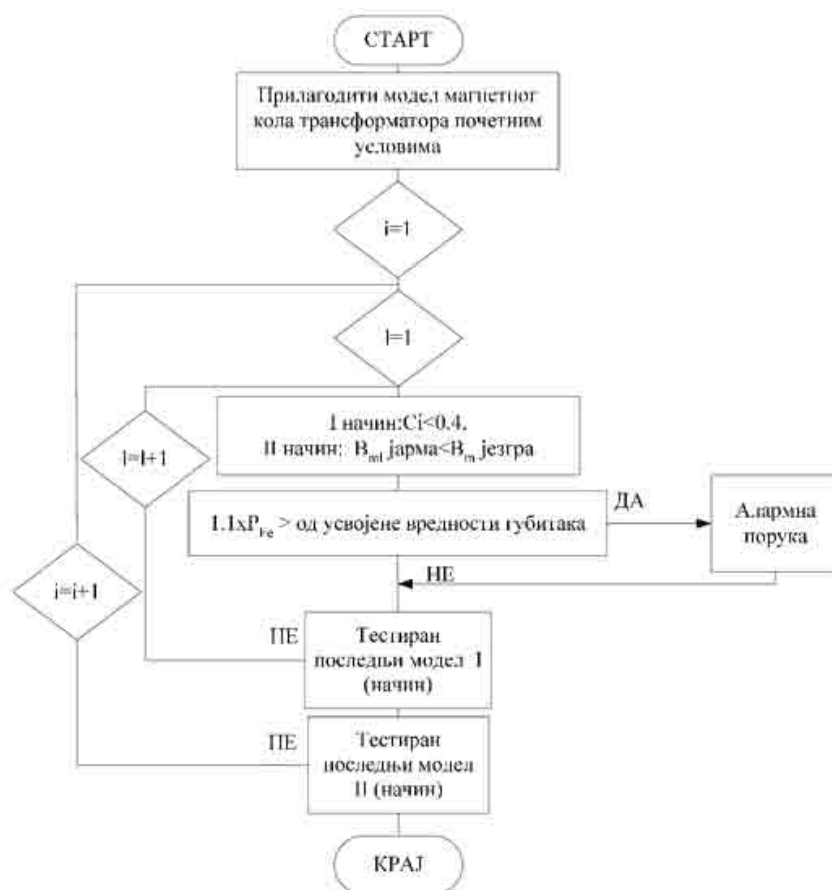
Слика 5.3.1.2. Граф дијаграм за прорачун магнетног кола
