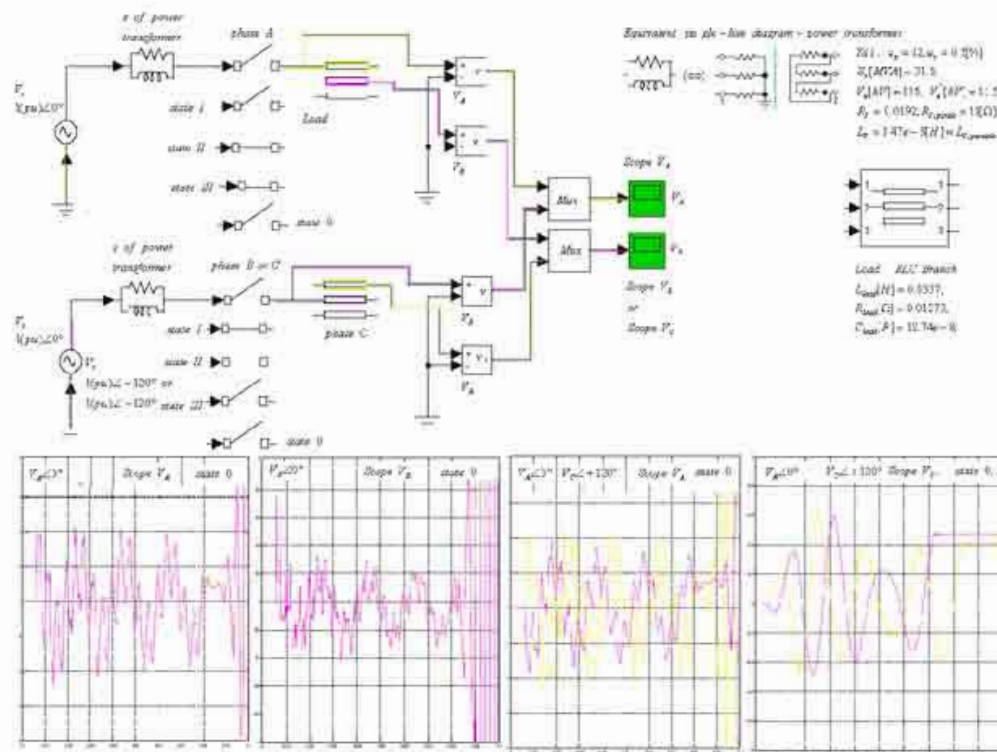
Слика 4.4.1. а)Основна шема за симулацију транзијентних пренапона у MATLABУ, б)дијаграми 0 теста
