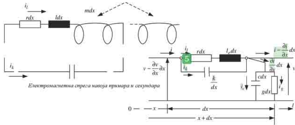
а) Параметри једног навоја намотаја примара енергетског трансформатора
