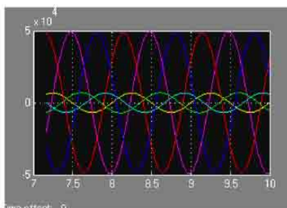
Слика.3.5.3. Графичка демонстрација струје примара и секундара неоптерећеног енергетског трансформатора Y\delta-11 , који је алгоритмом описан у моделу
