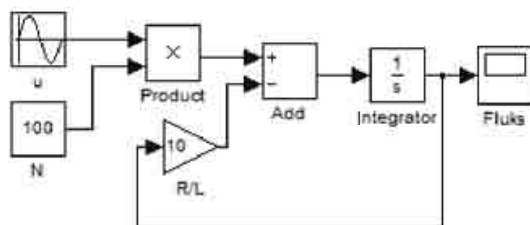
Слика..5.1.2.3. Симулација флукса
