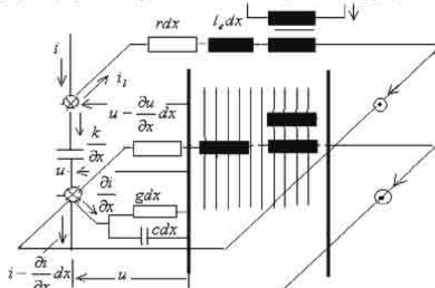
Слика 2.1.4.2.. Електромагнетни параметри једног навојка
