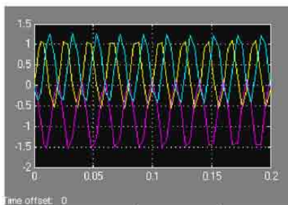
Слика.3.5.5. Графичка демонстрација магнетног флукса неоптерећеног енергетског трансформатора Y\delta-11 , који је алгоритмом описан у моделу.
