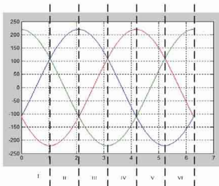
Слика 5.1.6.Магнетни флуке који тече у стубу трофазног трансформатора
