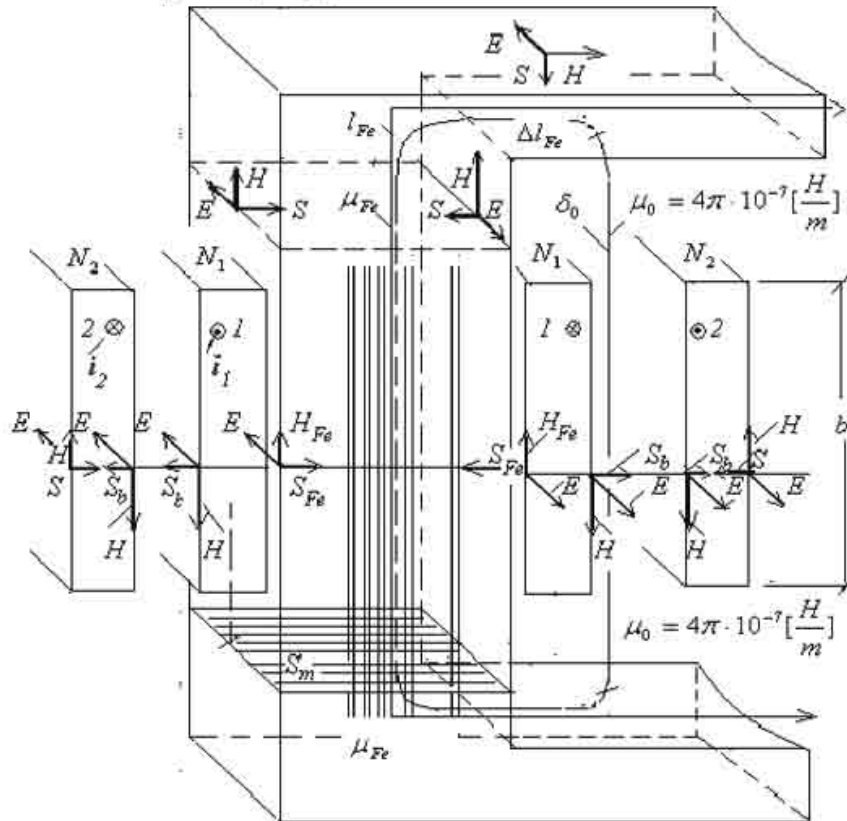
b) Prenos snage iz primara u sekundar kroz magnetno kolo
