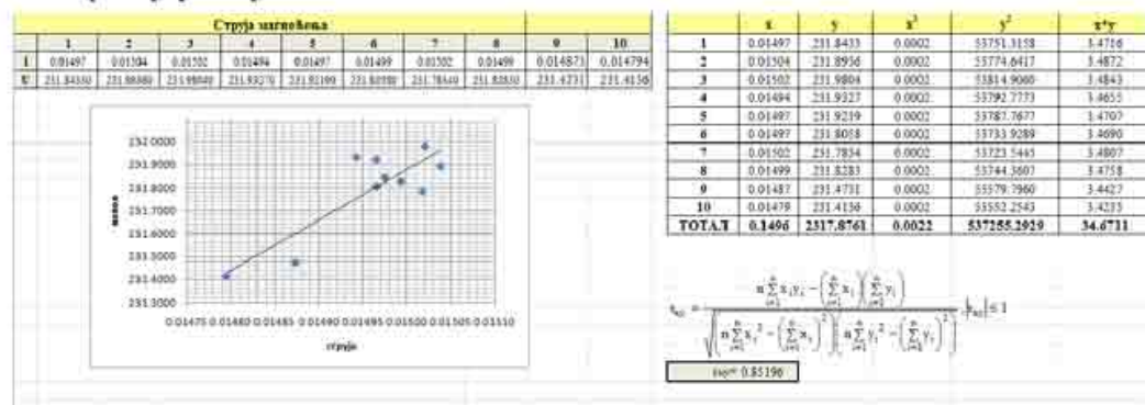
Слика 5.2.2.7. Коефицијент корелације, јака корелација
