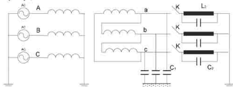
Слика 4.3.1. Енергетски трансформатор са трофазним прекидачем према реактору
