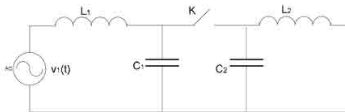
Слика 4.2.1. Једнополни приказ ситуације прекида у колу
