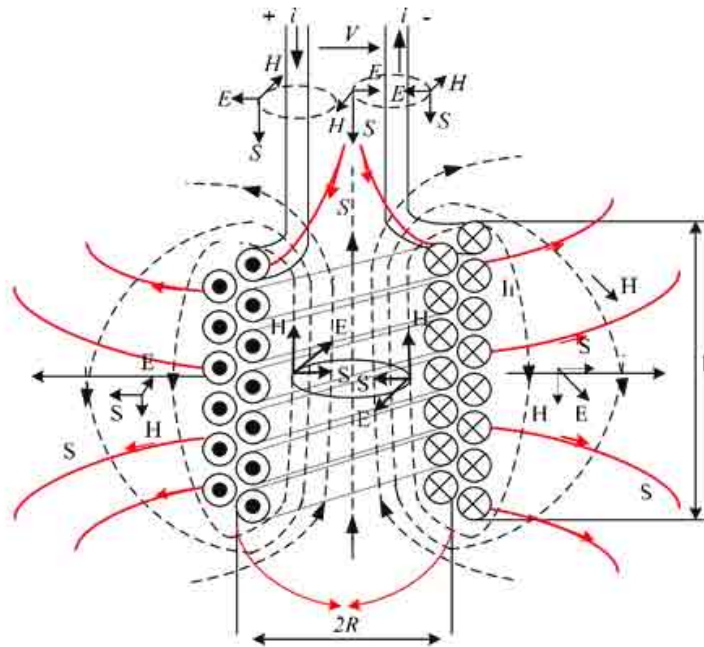
Слика 2.1.4.1.a. Расподела флукса снаге (Пинтингов вектор) у цилиндричном намотају
