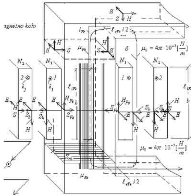
Слика 2.1.3.1. Димензије магнетног кола трансформатора и висине намотаја примара и секундара
