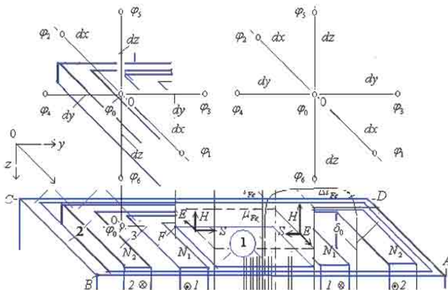
Слика 1. 3. 1. 6. Потенцијал у тачки 0, \Phi_0 изражен је помоћу потенцијала у тачкама 1,2,3,4,5,6: \Phi_1, \Phi_2, \Phi_3, \Phi_4, \Phi_5, \Phi_6 у чворовима мреже на одстојањима dz, dy, dx у Картезијанском координатном систему (Rene Descarte 2 )
