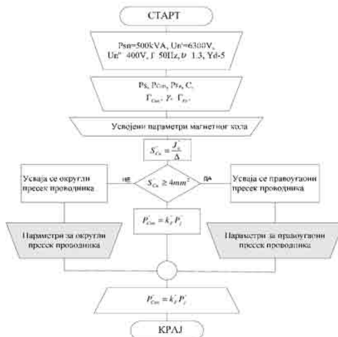
Слика 5.4.1.1. Итеративни поступак прорачуна намотаја ниског напона
