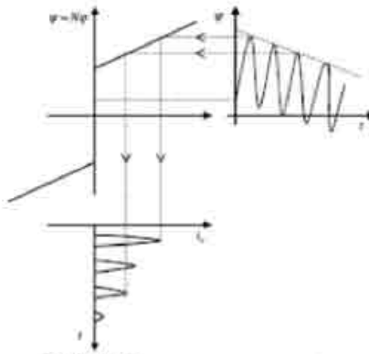
Слика 5.1.2.10. Временски ток струје укључења
