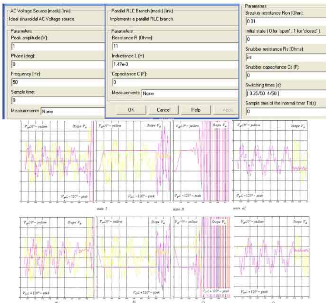
Слика 4.4.2. Дијаграми транзијентних пренапона на изводима трансформатора за различита динамичка стања – укључења и искључења фаза A, B, C.
