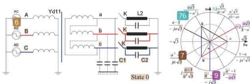
Слика 4.3.1. Енергетски трансформатор са трофазним прекидачем према реактору
