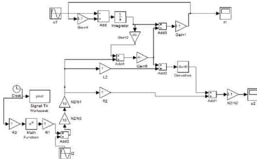
Слика 5.1.2.2.: Модел у коме делује синусна периодичне и аperiодична компоненте струје
