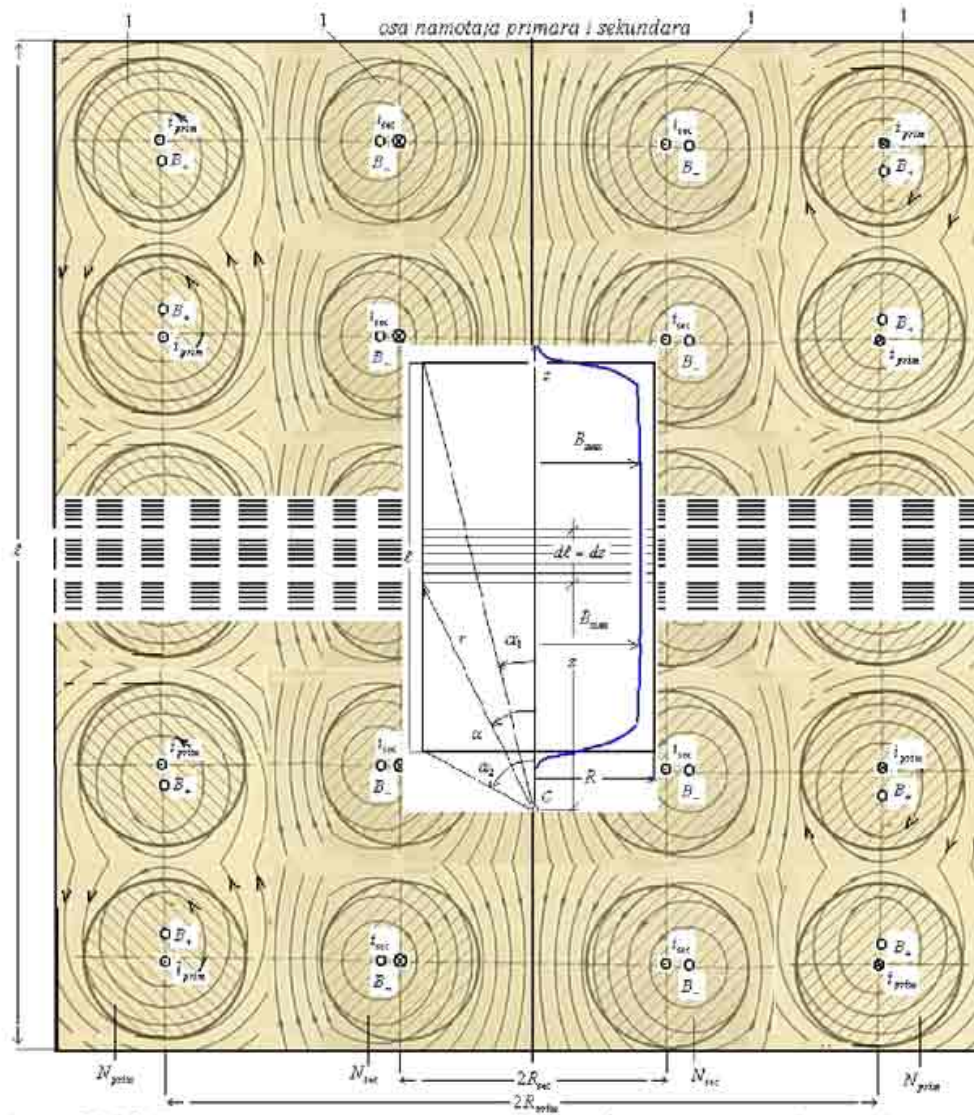
Слика 2.1.1.3. Индукција и квазистационарно поље струје i једног намотаја [примар/секундар] дужине (\lambda) полупречника R (R = R_{prim}) / (R = R_{sec}) i густо намотаних навојака N (N = N_{prim}) / (N = N_{sec}) .
