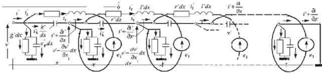
Слика 2.1.3.2. а). Подужни и попречни параметри еквивалентне шеме j тог навојка намотаја примара/секундара трансформатора, б) развијена шема по x оси са j навојком у намотаја примара/секундара трансформатора.
