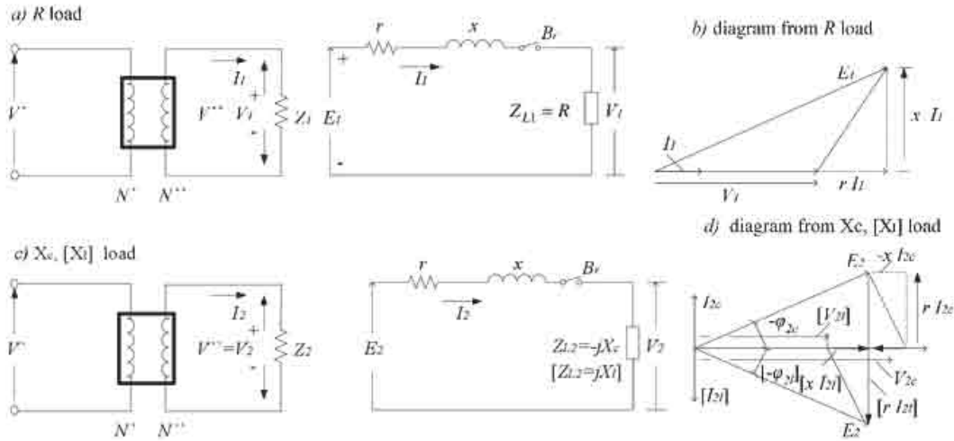
Слика 4.5.3.1. Шема и векторски дијаграм: а) за активно оптерећење R , б) векторски дијаграм за активно оптерећење R , в) реактивно X_c ( X_l ) оптерећење, д) векторски дијаграм за X_c ( X_l ) оптерећење.
