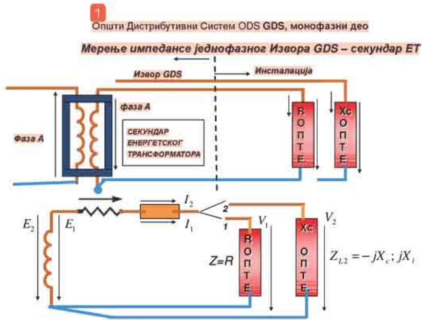
Слика 4.5.2.2. а) Мерење импедансе секундара 3- фазног Т, б) мерење импедансе секундара 1- фазног Т
