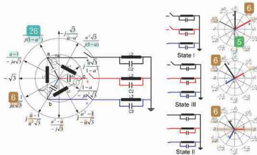
Слика. 4.3.2. Енергетски трансформатор са трополним прекидачем, еквивалентни дијаграм и State 0, I, II, III прелазни процеси на прекидачу према реактору
