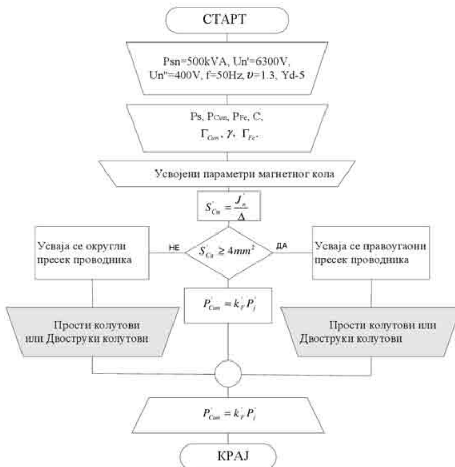
Слика 5.4.1.2. Итеративни поступак прорачуна намотаја високог напона
