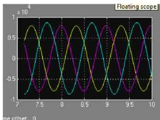
Слика.3.5.4. Графичка демонстрација струја магнетног неоптерећеног енергетског трансформатора Y\delta-11 , који је алгоритмом описан у моделу.
