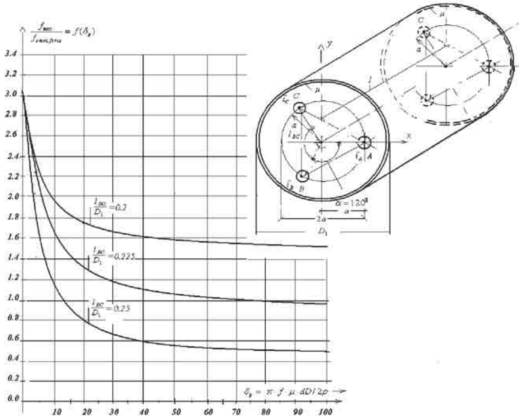
Слика 1.7.1. Зависности \frac{f_{\max}}{f_{\text{otot. force}}} = f(\delta_\rho) од фактора \delta_\rho = \pi \cdot f \cdot \mu \cdot \frac{dD}{2\rho_{el}} , омотача цилиндричног геометријског облика.
