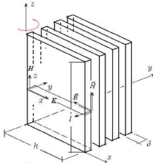
Слика 1.4.1. Величине које одређују равнског електромагнетног таласа у једном "листу" стуба језгра трансформатора
