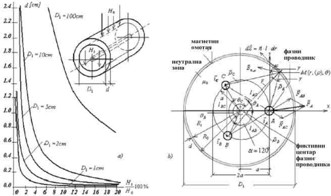
Слика 1.5.3.а.и б. Дијаграми зависности дебљина цилиндричних омотача d од слабљења утицаја спољног поља h_{i,pu} , параметри кривих су D_1 [22]
