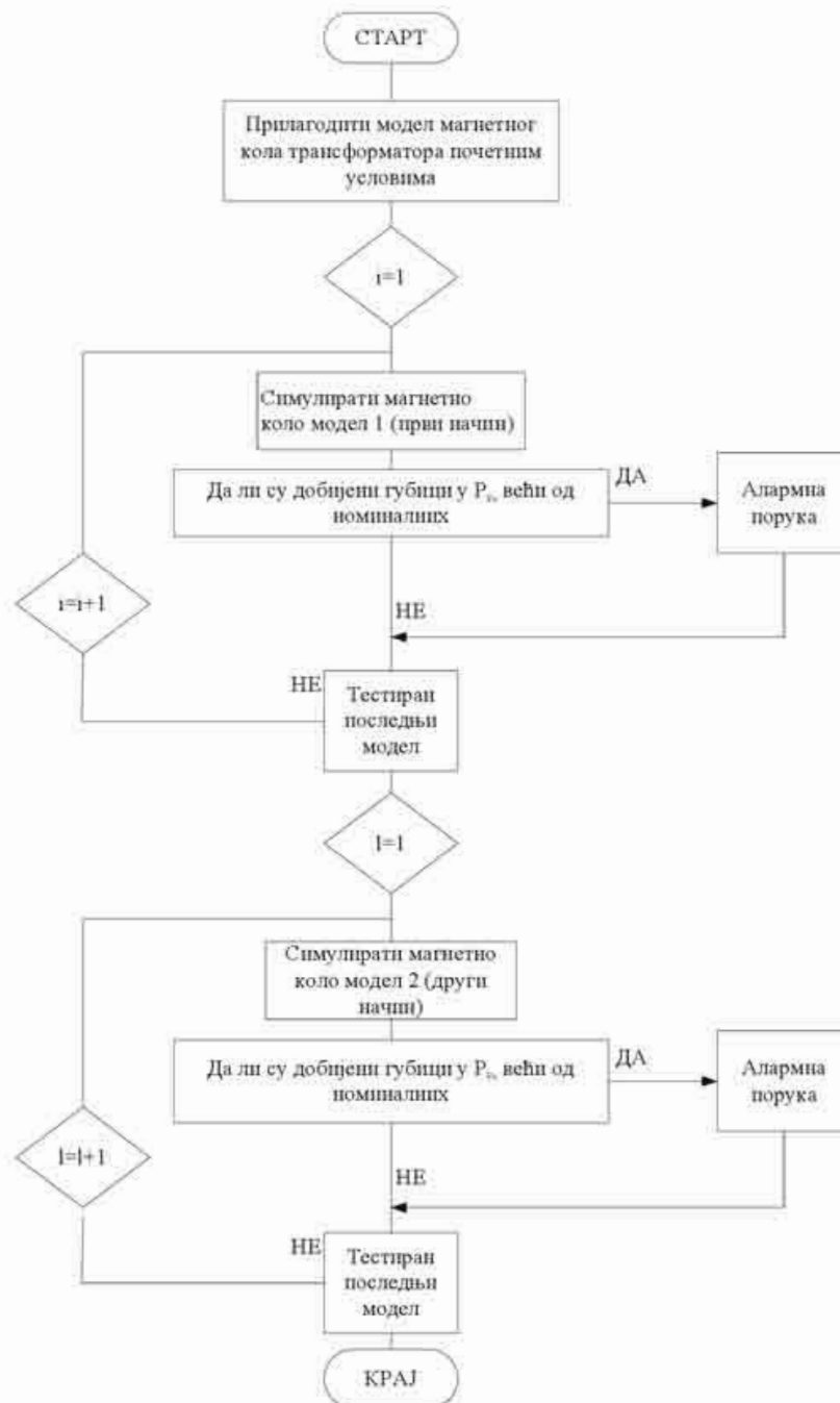
Слика 5.3.1.1. Итеративни поступак прорачуна магнетног кола трансформатора
