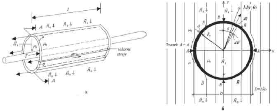
Слика 1.5.2. Струја у проводницима и расподела повратне струје у омотачу истакнутих магнетних параметара
