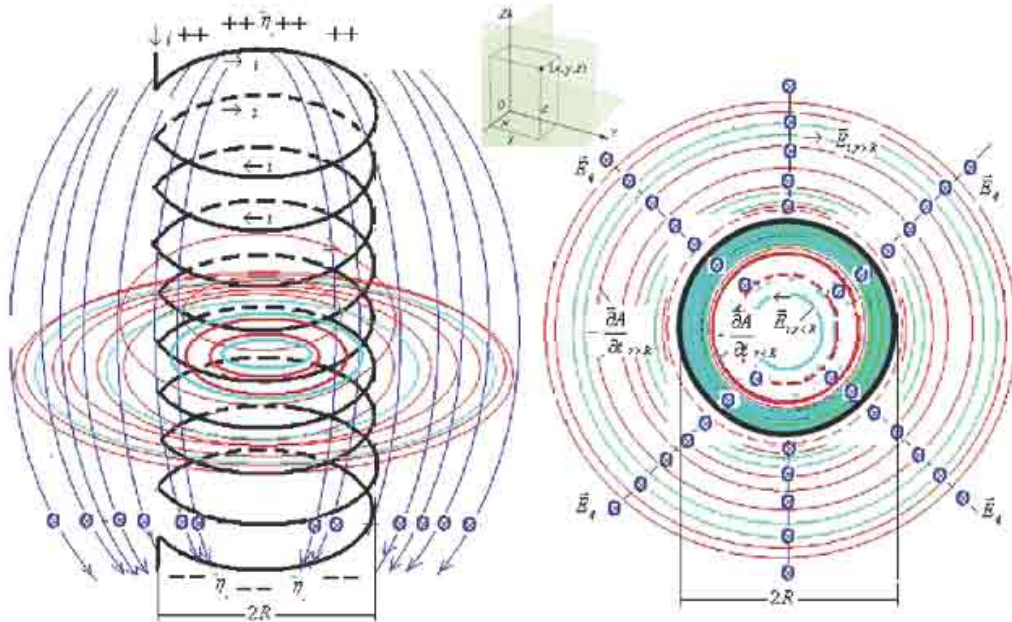
Слика 2.1.1.4.: Магнетски вектор потенцијали, квазистационарно поље и поље електростатичких оптерећења које ствара струја i једног намотаја [примар/секундар] дужине (l) полупречника (R)
