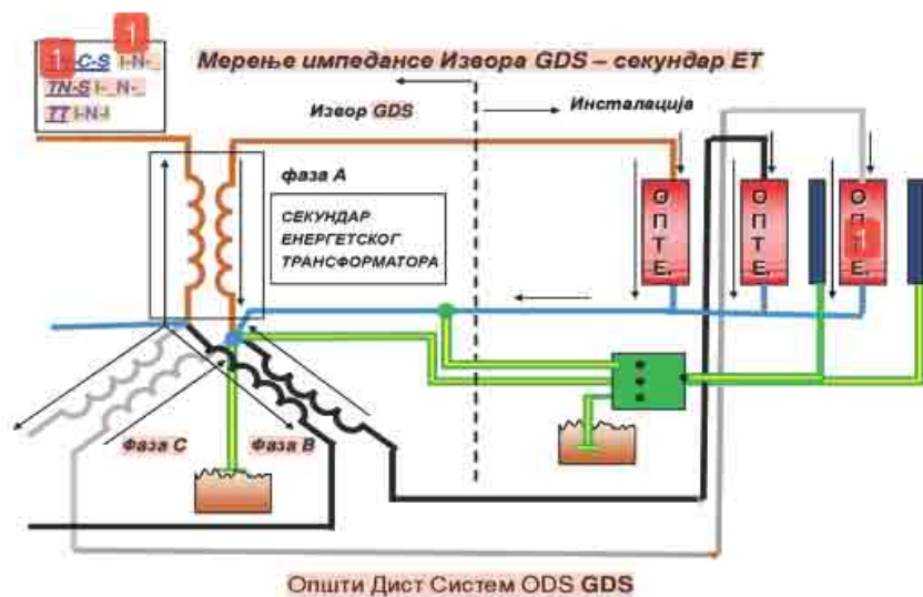
Слика 4.5.2.1. Мерење импедансе код енергетског трансформатора
