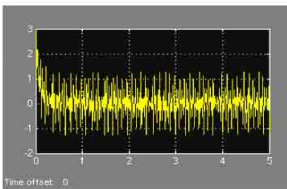
Слика 5.1.2.5. Флуks за максималне вредности напона 200V
