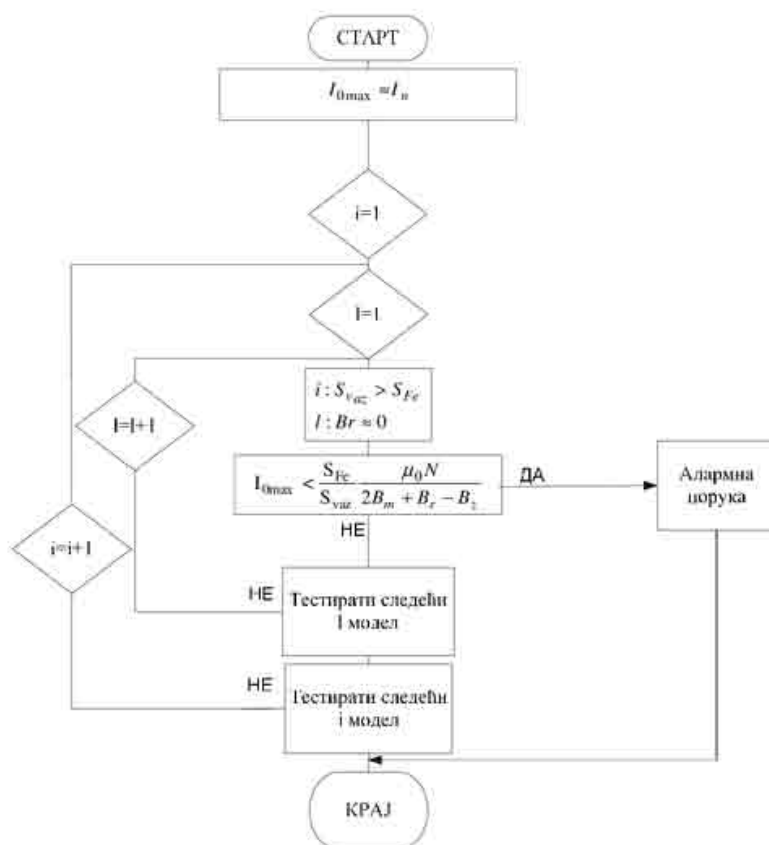
Слика 5.2.1.3. Итеративни поступак прорачуна струје магнећења
