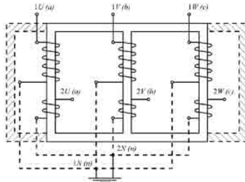
Слика 5.1.3. Електрично и магнетно коло трансформатора.
