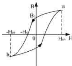
Слика 5.1.7. Хистерезисни циклус
