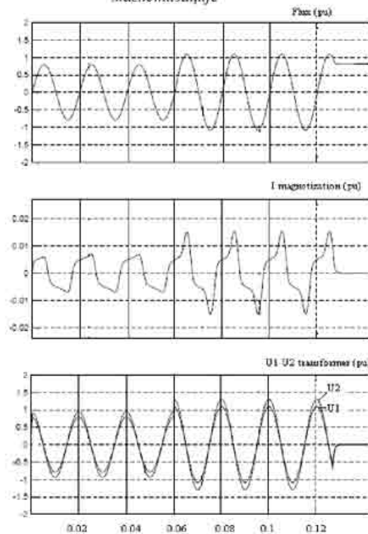
Слика 3.3.2. Резултати симулације бр.1.: Дијаграм флукса, струје магнетезања и напона примара и секундара.
