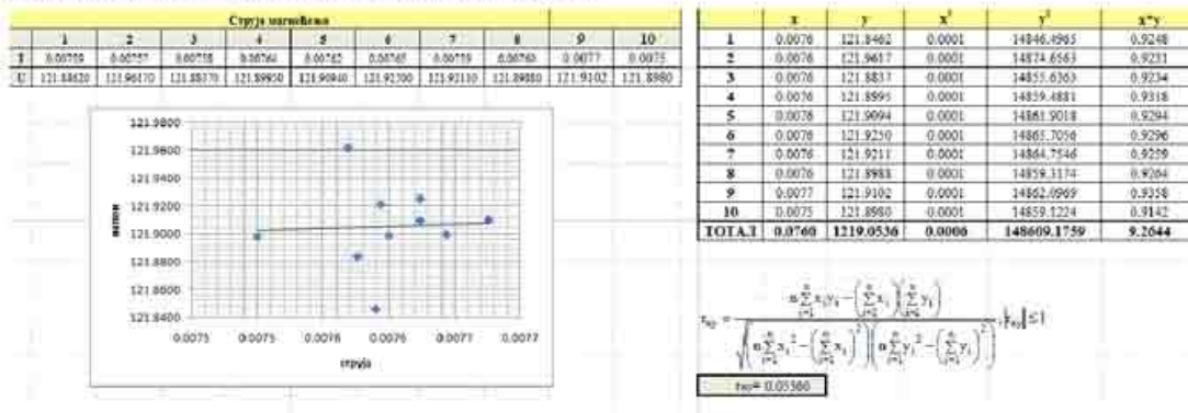
Слика5.2.2.4. Коефицијент корелације, безначајна корелација
