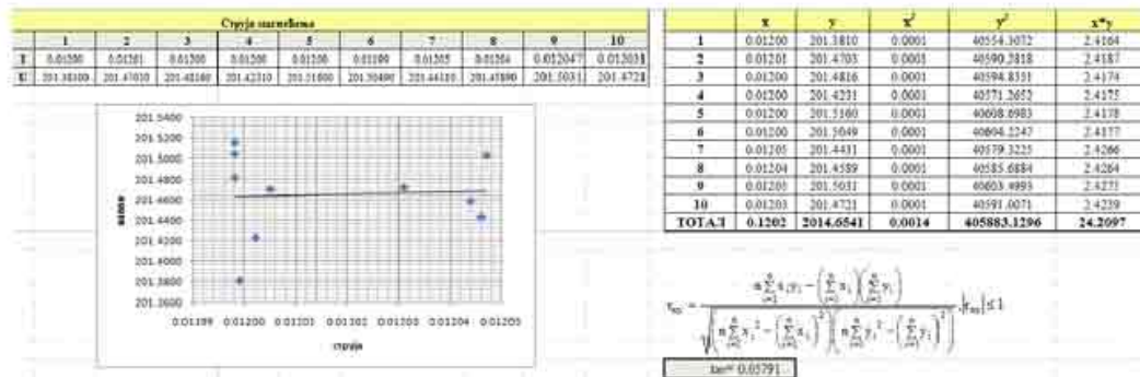
Слика 5.2.2.7. Коефицијент корелације, безначајна корелација
