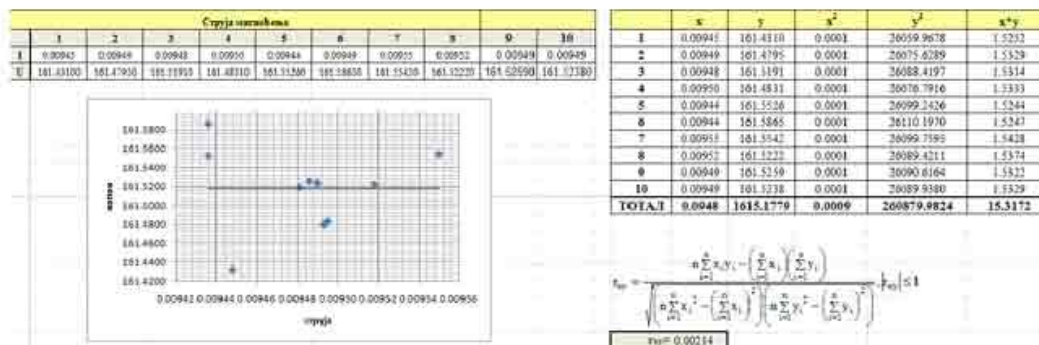
Слика 5.2.2.6. Коефицијент корелације, безначајна корелација
