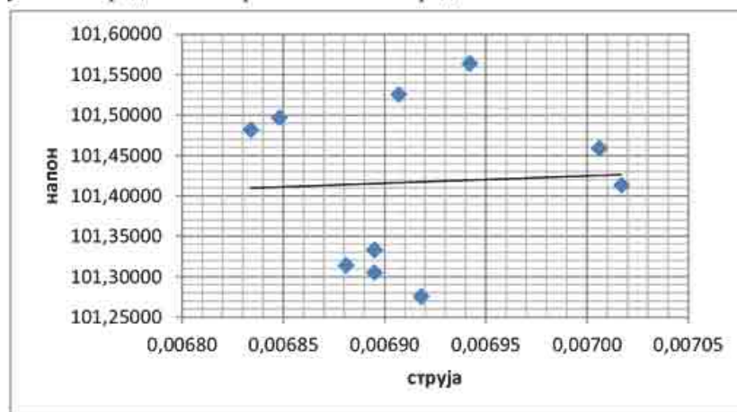
Слика 5.2.2.3. Дијаграм расипања
