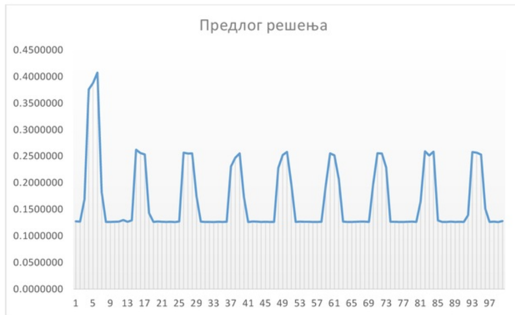
Слика 66. Време извршавања скрипте заштићене предложеним решењем
