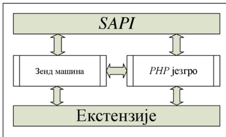
Слика 41. Архитектура PHP
