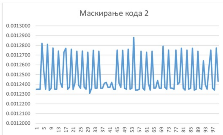
Слика 69. Време извршавања скрипте заштићене маскирањем кода решењем 2
