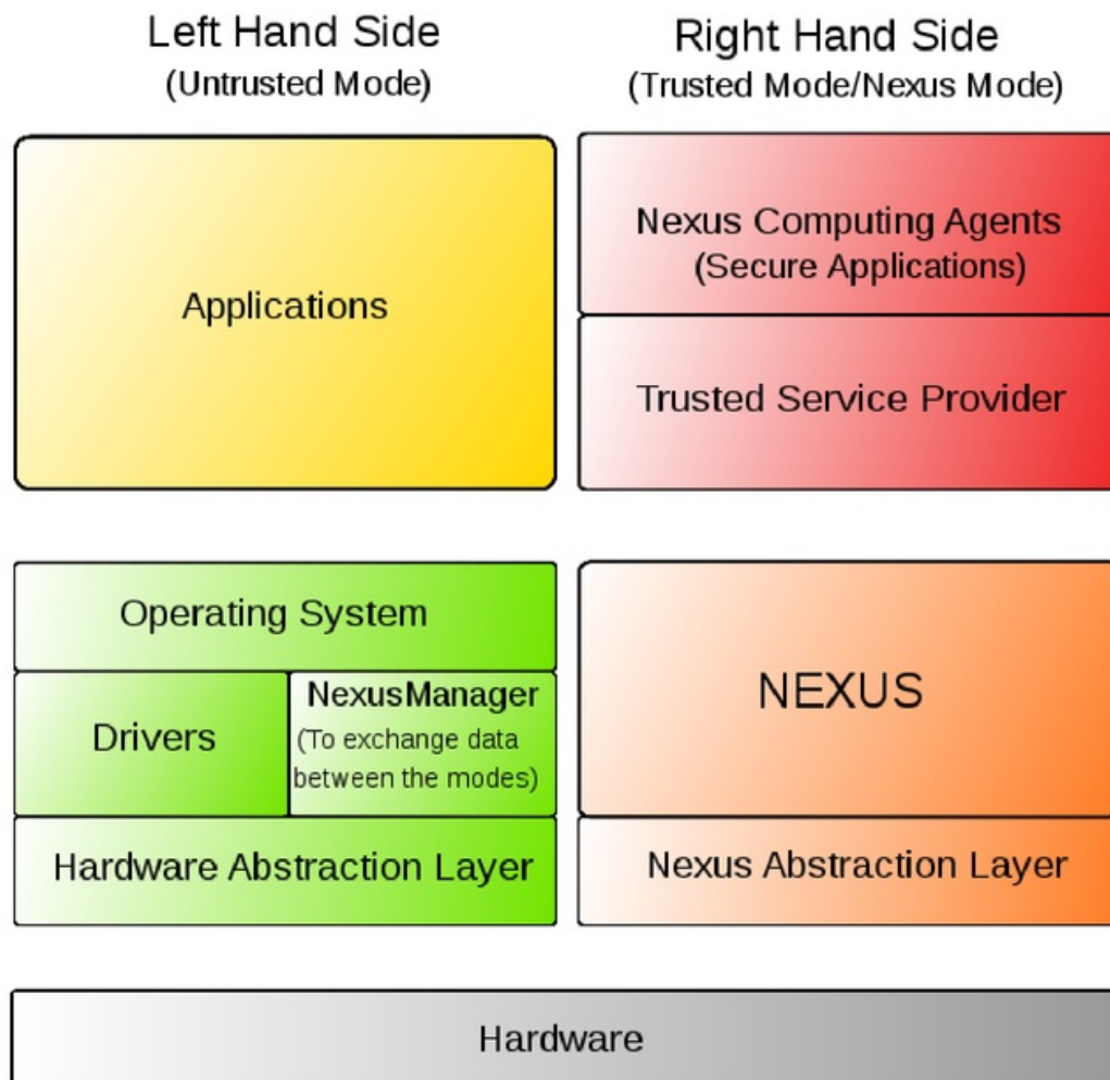
Слика 40. Сигурна рачунарска основа нове генерације (енгл. Next Generation Secure Computing Base ) [70]
