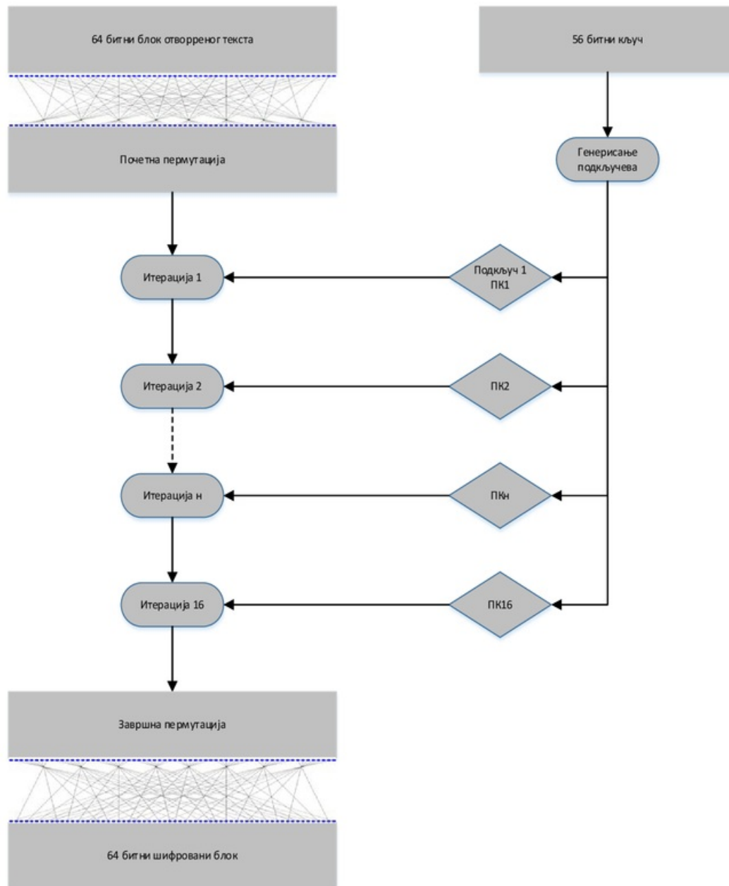
Слика 8. Шифровање блока ДЕС
