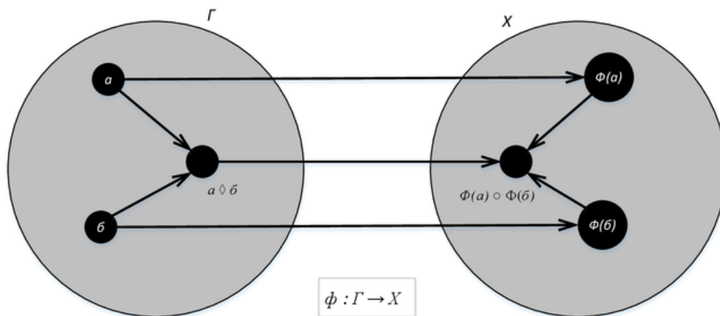
Слика 19. Хомоморфизам група
