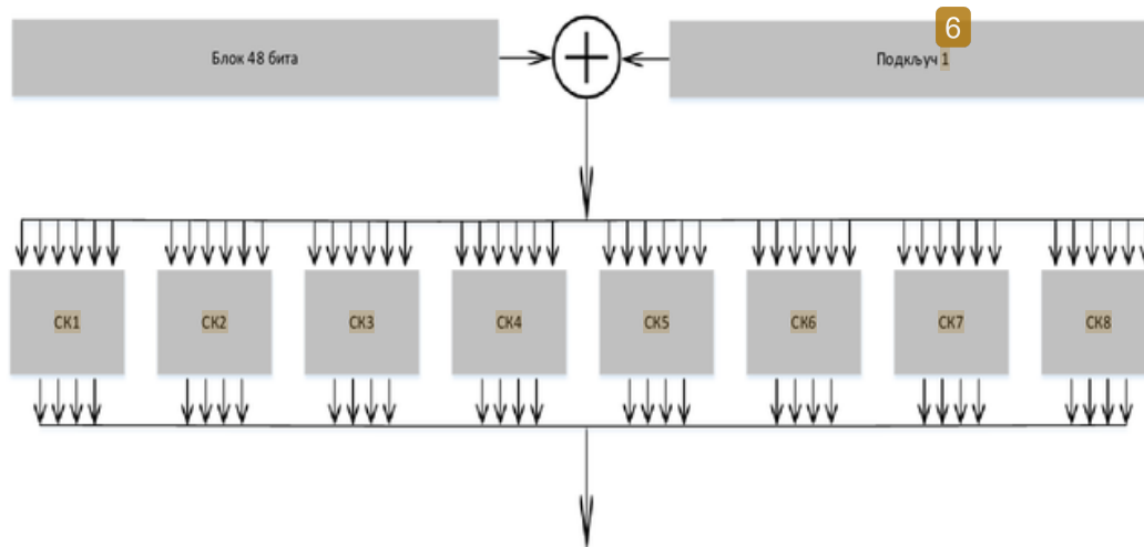
Слика 10. Операције с-кутија
