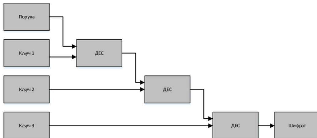
Слика 11. Приказ реализације троструки DES
