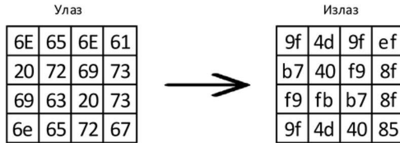
Слика 14. Приказ функције замене употребом с-кутије
