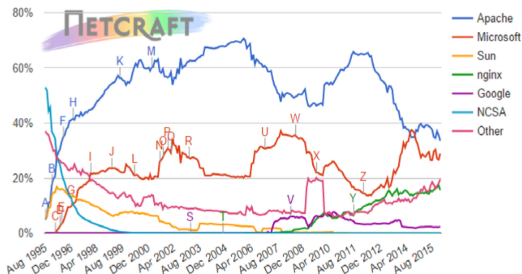
Слика 27. Учешће различитих Веб сервера
