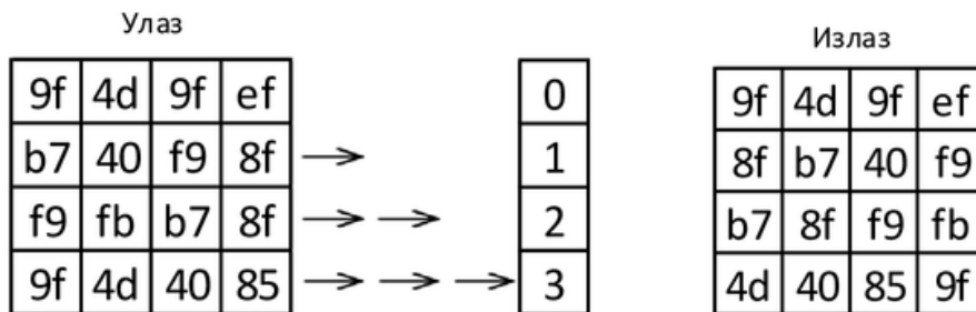
Слика 15. Приказ функције померања редова
