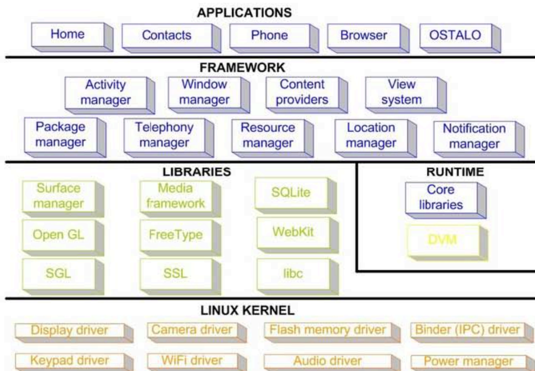
Слика бр. 8.: Андроид анатомија.
