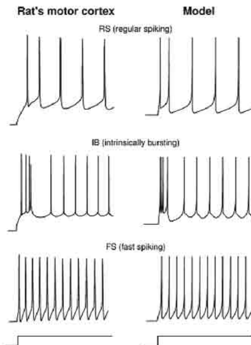
Slika 17: Izhikevich-ev „Simple model“ može da reprodukuje povorke impulsa veoma bliske stvarnim elektrofiziološkim impulsima različitih tipova neurona u motornom korteksu pacova (preuzeto iz [146]).
