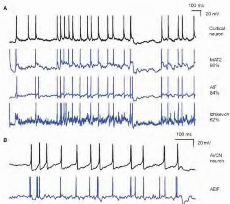
Slika 18: Poređenje kvaliteta nekih modela neurona (preuzeto iz [147]). (A) Stvarni elektrofiziološki signal kortikalnog neurona i simulirani odziv nekoliko popularnih naprednijih modela (B) Elektrofiziološki signal AVCN neurona (Anteroventral cochlear nucleus neuron) i simulirani odziv AEIF modela („Adaptive Exponential Integrate-and-Fire“, Brette i Gerstner, 2005. [141]).
