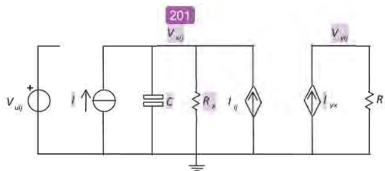
Slika 27: Originalna CNM ćelija, prema modelu Chua i Yang ([21]).
