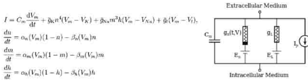
Slika 15: Hodgkin–Huxley model. Matematički model i ekvivalentno električno kolo membrane (preuzeto iz [139]).
