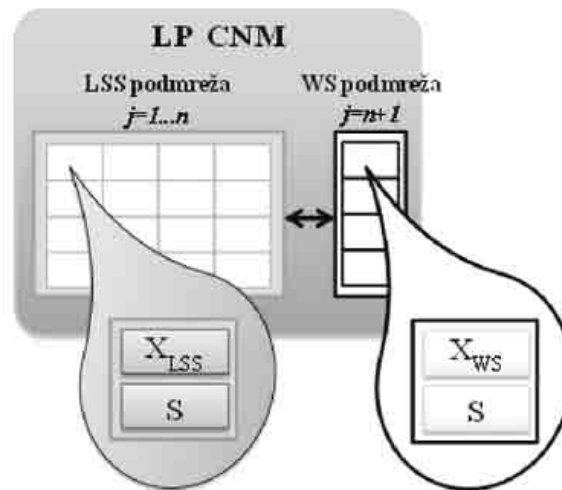
Slika 31: Topološka arhitektura LPS CNM. Podmreža LSS sa leve strane (siva) sastoji se od identičnih modula tipa LSS (Linear System Solver CNM) dok se podmreža na desnoj strani (bela) sastoji od modula slične topologije ali sa različitom x -čelijom. I jedni i drugi moduli imaju istu unutrašnju topologiju – sastoje se od dve ćelije ( x i S tipa).
