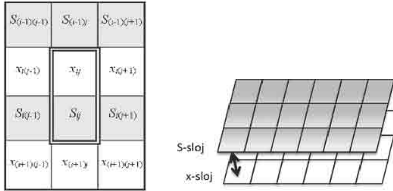
Slika 29: Raspored ćelija CNM mreže za rešavanje sistema linearnih algebarskih jednačina (LSS CNM). Po jedna korespondentna (i, j) x i S ćelija čine „modul“. Ovakva topologija se može predstaviti i kao dvoslojna mreža.
